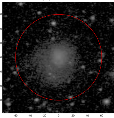
LEDA: pa,inc= 1.0 35.6
