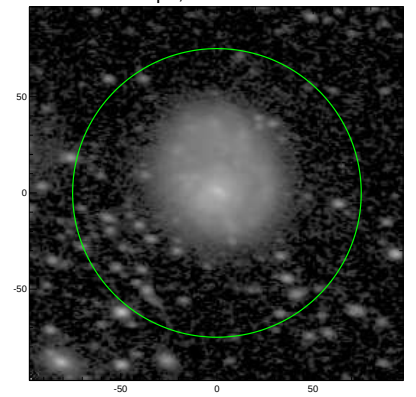
S4G: pa,inc= -3.8 48.2
