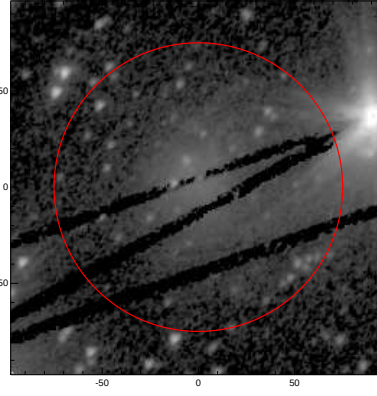
LEDA: pa,inc= 51.4 42.0
