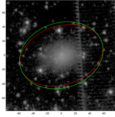
ESO486-021
