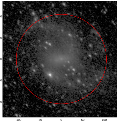
LEDA: pa,inc= 136.8 46.8
