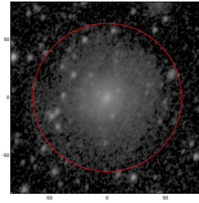
LEDA: pa,inc= 62.1 41.0
