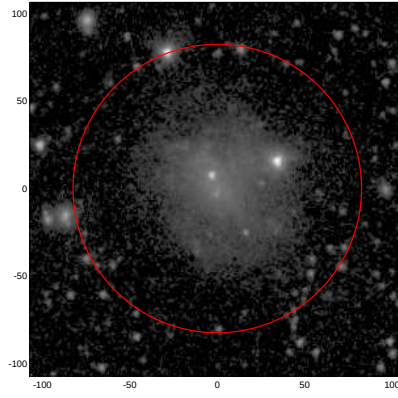
LEDA: pa,inc= 999.0 17.7
