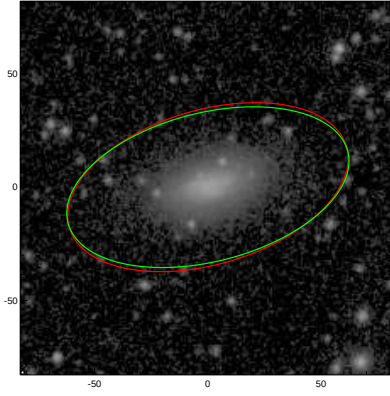
ESO603-031
