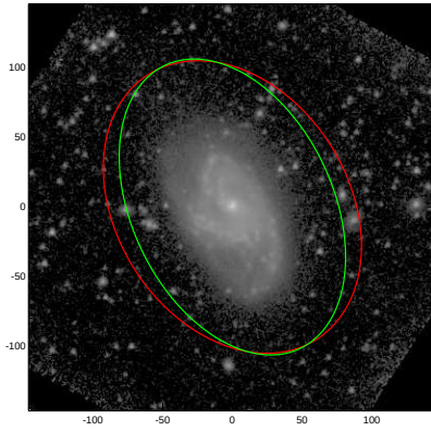
ESO342-050
