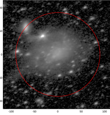
LEDA: pa,inc= 22.6 50.0
