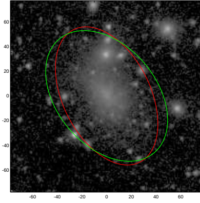
ESO549-002
