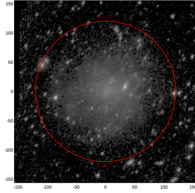
LEDA: pa,inc= 60.3 43.6
