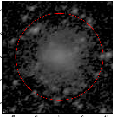
LEDA: pa,inc= 33.3 44.9
