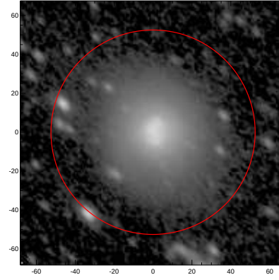
LEDA: pa,inc= 134.7 54.7
