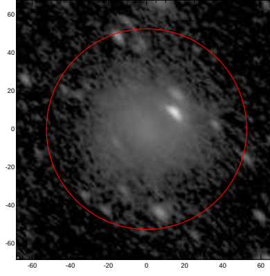
LEDA: pa,inc= 136.1 59.0
