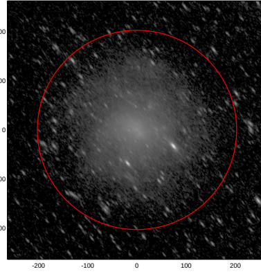
LEDA: pa,inc= 129.3 67.6
