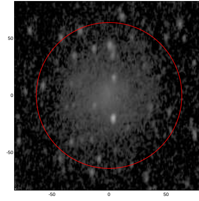
LEDA: pa,inc= 86.6 55.1
