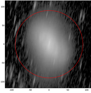
LEDA: pa,inc= 78.8 80.2
