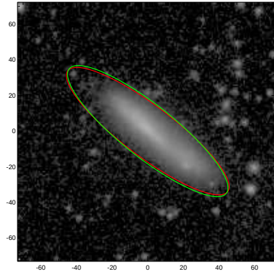
ESO479-025
