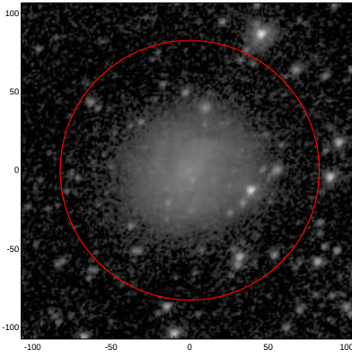
LEDA: pa,inc= 40.3 34.3
