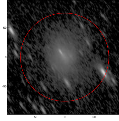
LEDA: pa,inc= 121.7 71.9
