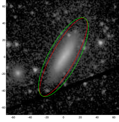
ESO576-008
