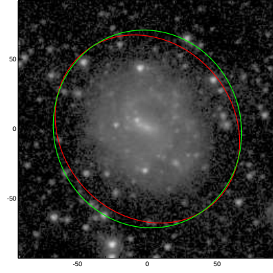
ESO026-001
