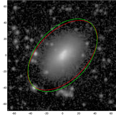
ESO402-030
