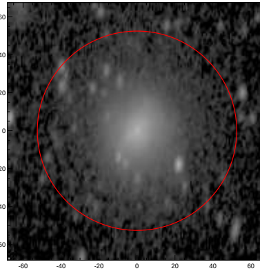
LEDA: pa,inc= 83.1 57.5
