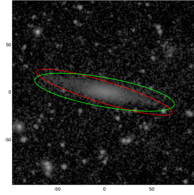
ESO482-005
