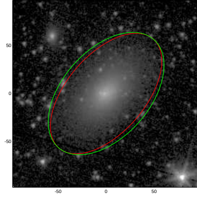
ESO483-013
