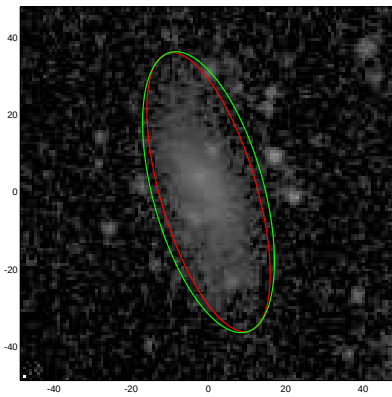
ESO504-010
