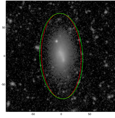
ESO358-051
