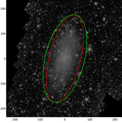
ESO300-014
