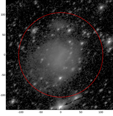
LEDA: pa,inc= 40.8 49.7
