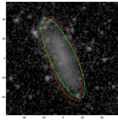
ESO476-010
