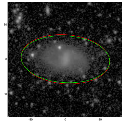
ESO548-025
