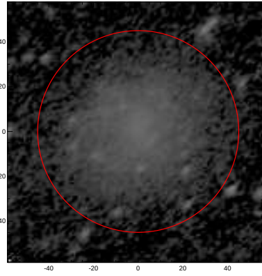
LEDA: pa,inc= 39.2 53.4
