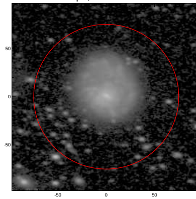
LEDA: pa,inc= 177.9 49.7
