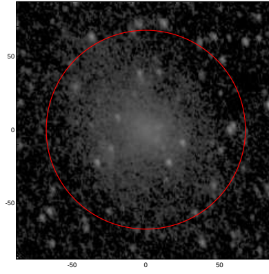
LEDA: pa,inc= 109.8 40.0
