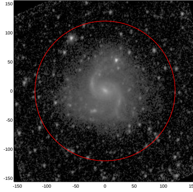
LEDA: pa,inc= 72.1 34.3
