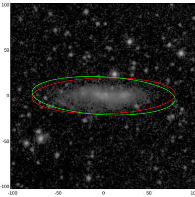
ESO602-003
