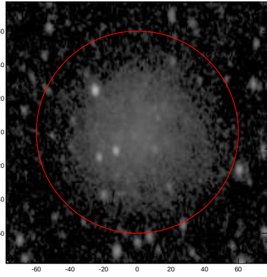
LEDA: pa,inc= 97.7 45.3
