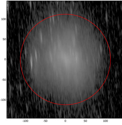
LEDA: pa,inc= 95.0 81.8
