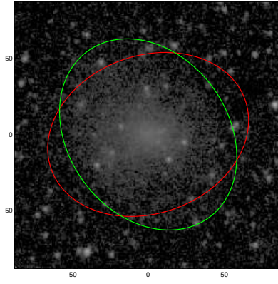
ESO545-016
