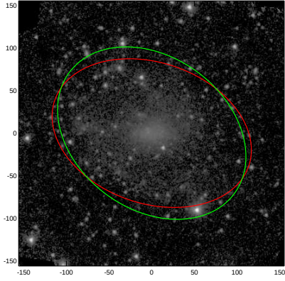
ESO305-009
