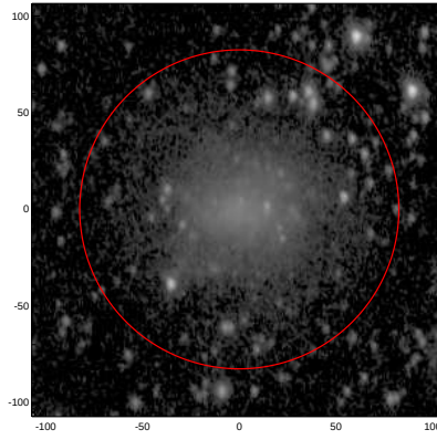
LEDA: pa,inc= 97.7 44.7
