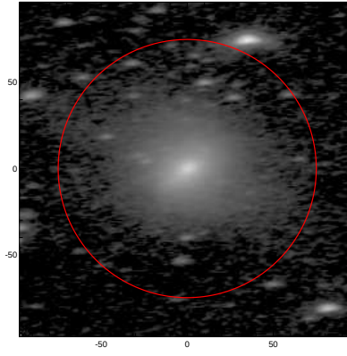
LEDA: pa,inc= 4.4 68.4
