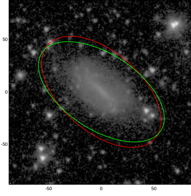
ESO443-085
