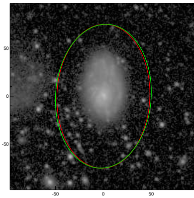
ESO510-058
