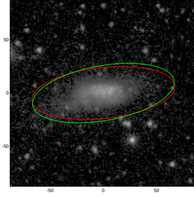
ESO361-019
