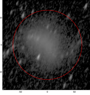
LEDA: pa,inc= 67.1 65.1
