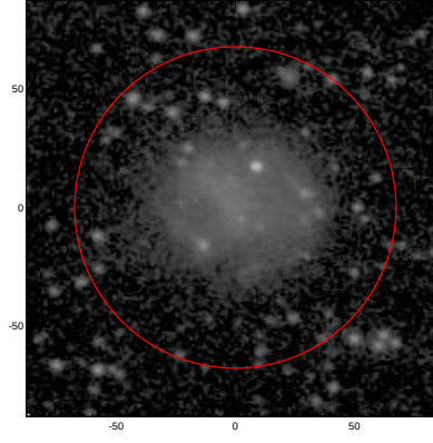
LEDA: pa,inc= 162.9 33.5
