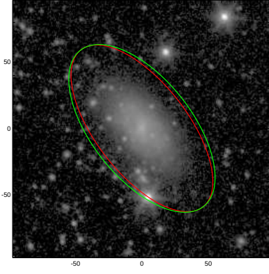
ESO572-018
