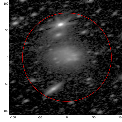
LEDA: pa,inc= 17.5 60.6
