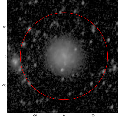
LEDA: pa,inc= 74.7 40.8
