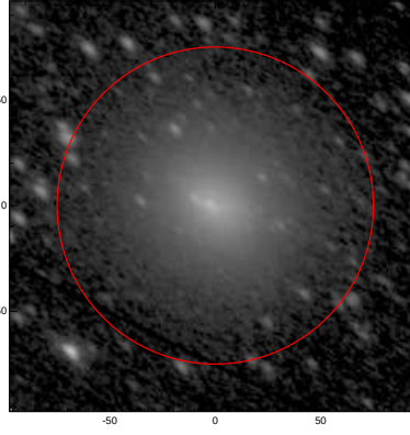
LEDA: pa,inc= 139.0 57.1
