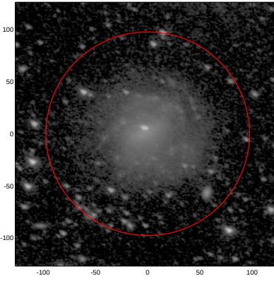
LEDA: pa,inc= 157.0 46.4
