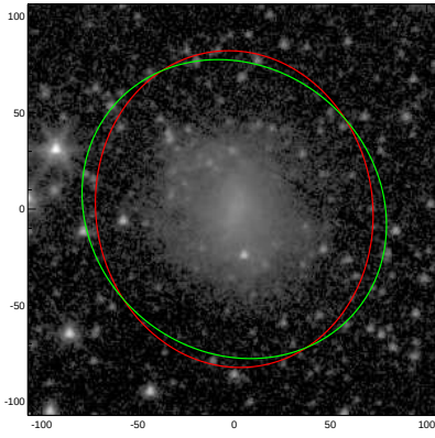
ESO287-037
