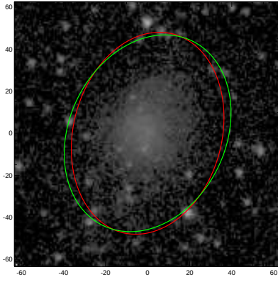
ESO504-024
