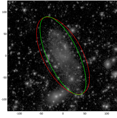
ESO119-016
