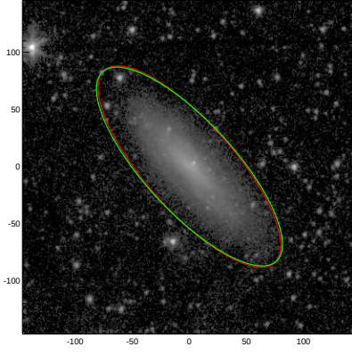
ESO481-018
