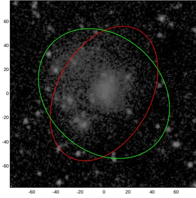
ESO539-007
