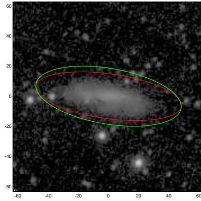
ESO402-025
