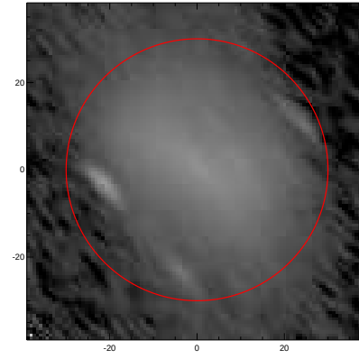
LEDA: pa,inc= 132.9 71.0
