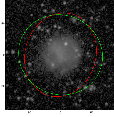
ESO288-013
