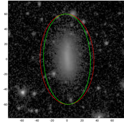
ESO419-013
