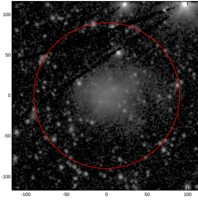
LEDA: pa,inc= 999.0 13.4
