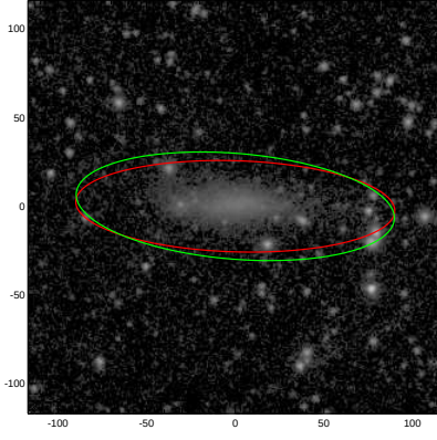
ESO249-027
