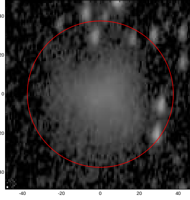
LEDA: pa,inc= 85.4 60.7
