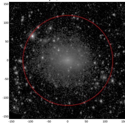
LEDA: pa,inc= 999.0 24.5
