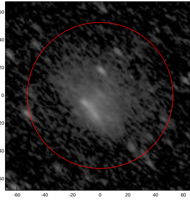
LEDA: pa,inc= 137.1 64.1
