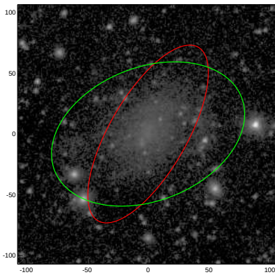
ESO145-025
