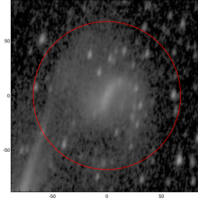
LEDA: pa,inc= 79.8 57.7
