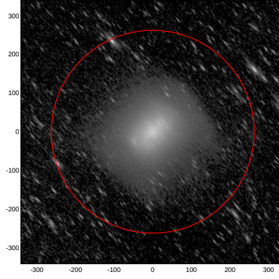
LEDA: pa,inc= 131.6 73.0
