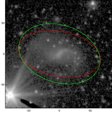
ESO340-042
