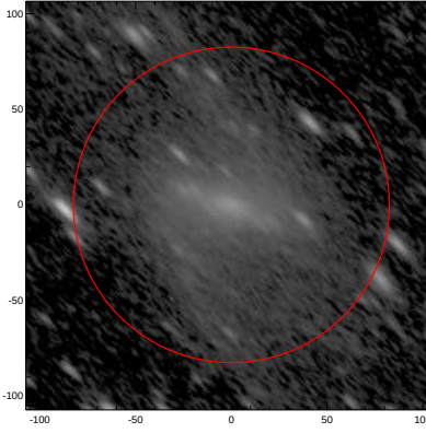
LEDA: pa,inc= 135.4 71.1
