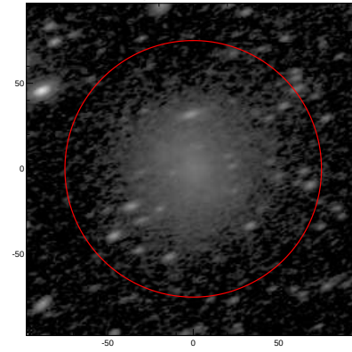
LEDA: pa,inc= 21.2 58.3
