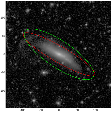
ESO545-005
