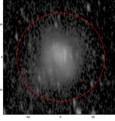
LEDA: pa,inc= 96.1 69.2
