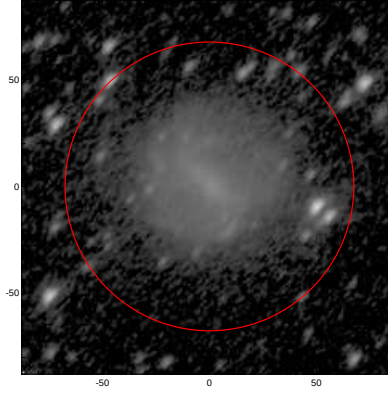
LEDA: pa,inc= 49.0 55.8
