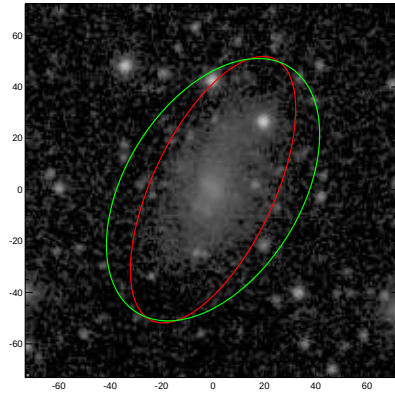
ESO403-031
