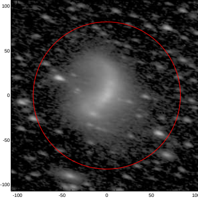
LEDA: pa,inc= 162.5 64.2
