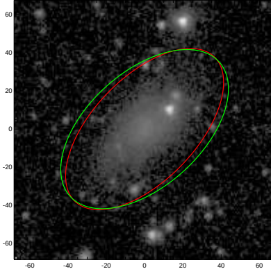
ESO548-082
