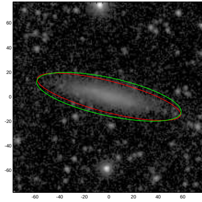
ESO356-018
