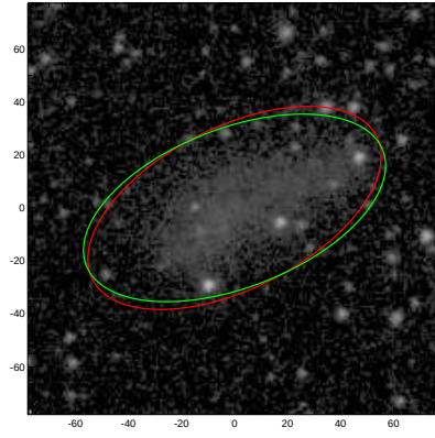
ESO120-021
