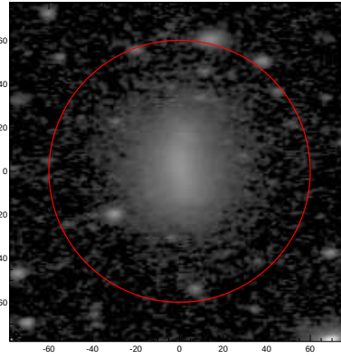
LEDA: pa,inc= 1.9 53.5
