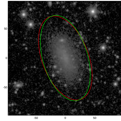
ESO359-029
