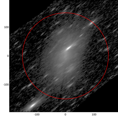
LEDA: pa,inc= 38.8 76.3
