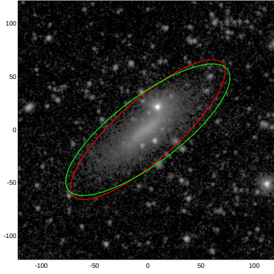
ESO359-003
