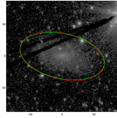
ESO508-007
