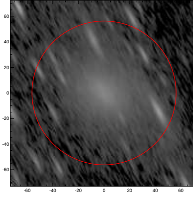
LEDA: pa,inc= 117.8 76.5
