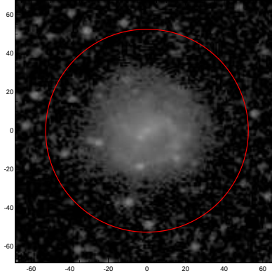
LEDA: pa,inc= 177.5 31.7
