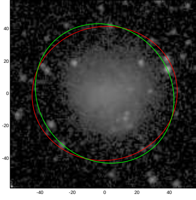
ESO359-031
