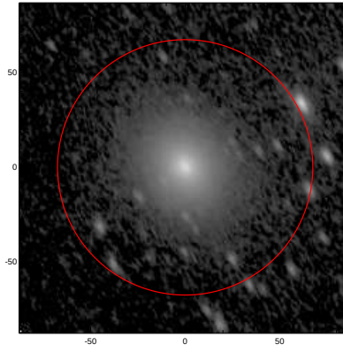
LEDA: pa,inc= 121.3 59.8
