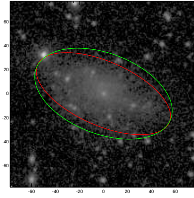
ESO406-042
