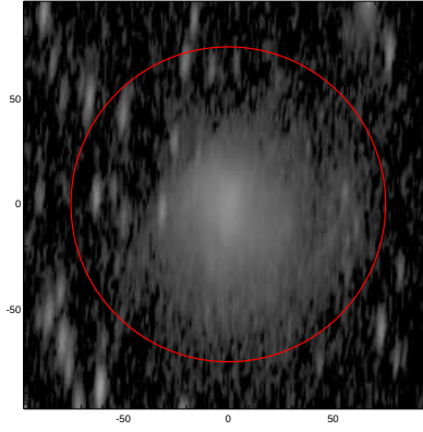
LEDA: pa,inc= 86.2 77.0
