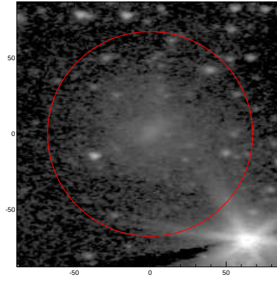
LEDA: pa,inc= 0.2 50.6
