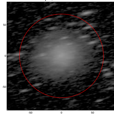
LEDA: pa,inc= 12.5 74.8
