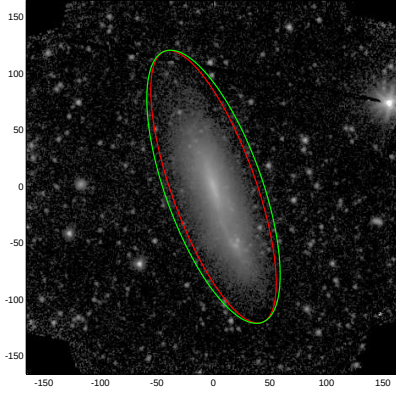
ESO423-002
