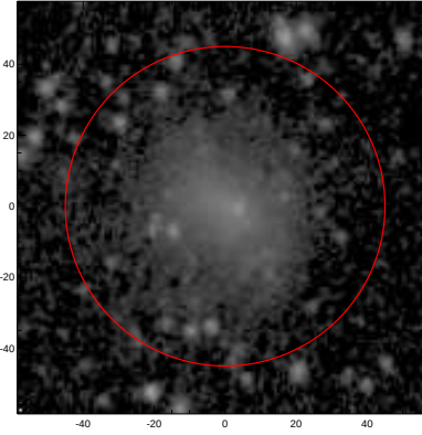
LEDA: pa,inc= 999.0 23.9
