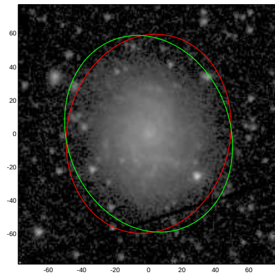
ESO580-030
