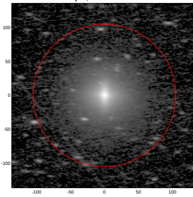
LEDA: pa,inc= 176.7 63.5
