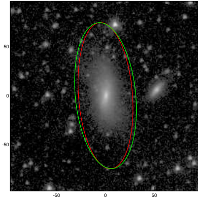
ESO462-031
