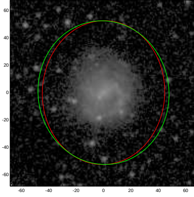
ESO238-018
