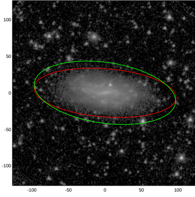
ESO285-048
