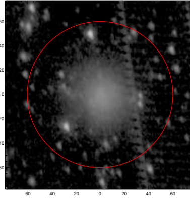
LEDA: pa,inc= 107.9 46.7
