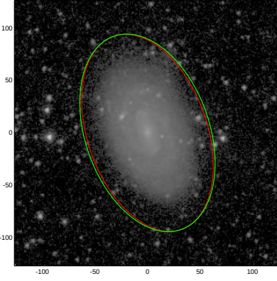
ESO549-018
