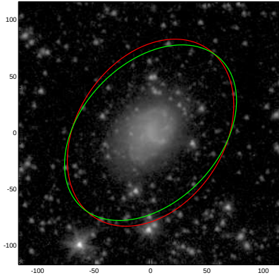
ESO418-008
