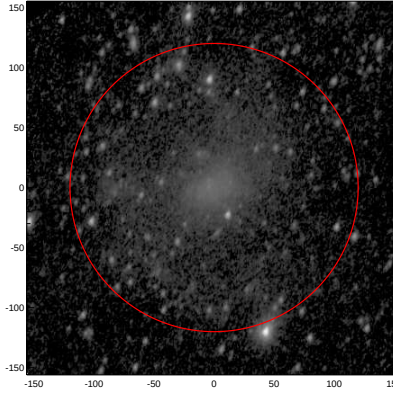
LEDA: pa,inc= 71.3 46.5
