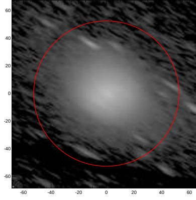
LEDA: pa,inc= 150.8 74.7
