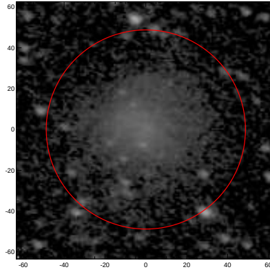
LEDA: pa,inc= 165.7 43.6
