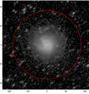
LEDA: pa,inc= 42.2 52.2
