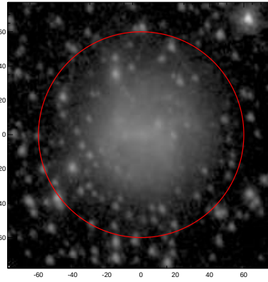
LEDA: pa,inc= 106.9 32.9
