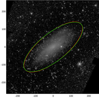
ESO550-024
