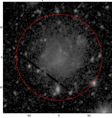
LEDA: pa,inc= 52.6 29.0
