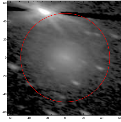
LEDA: pa,inc= 159.8 67.7
