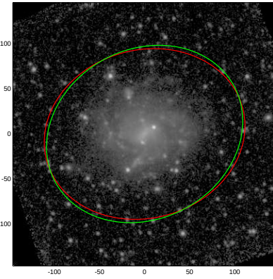
ESO445-089
