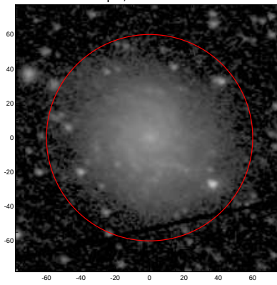
LEDA: pa,inc= 167.9 35.6
