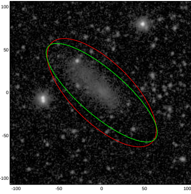
ESO469-008
