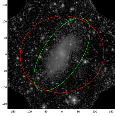
ESO012-010
