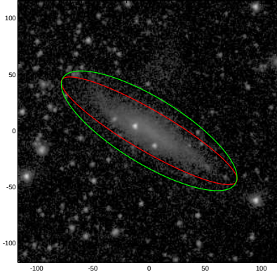
ESO550-005
