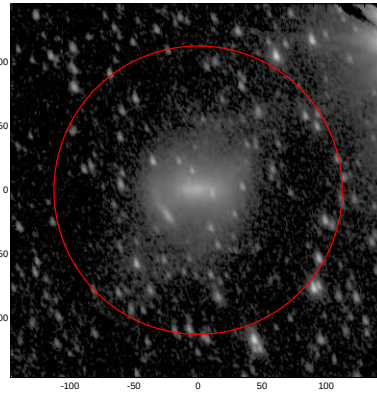
LEDA: pa,inc= 112.4 54.9
