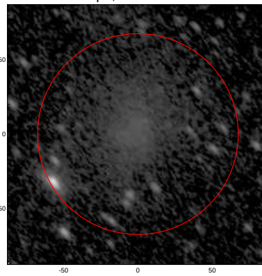
LEDA: pa,inc= 133.4 59.5
