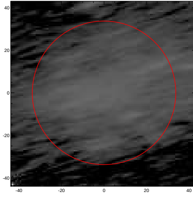
LEDA: pa,inc= 14.3 77.4
