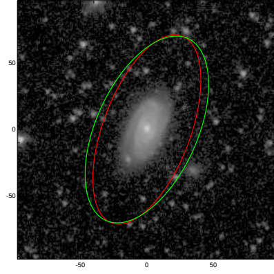
ESO576-001
