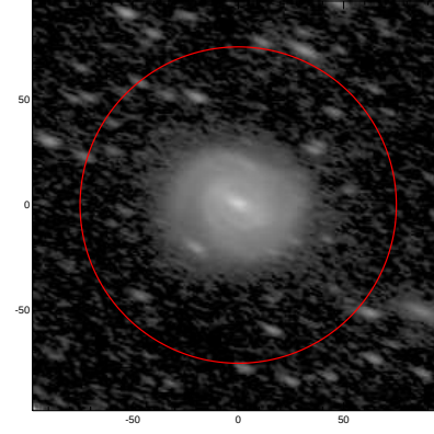
LEDA: pa,inc= 159.2 64.0
