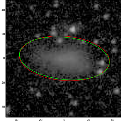
ESO236-039
