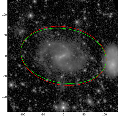
ESO510-059
