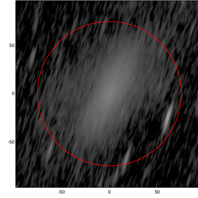
LEDA: pa,inc= 73.1 81.3
