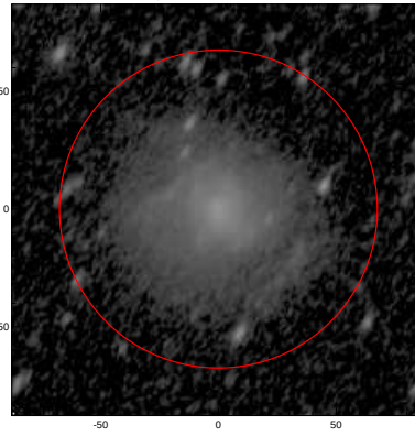
LEDA: pa,inc= 60.1 57.0
