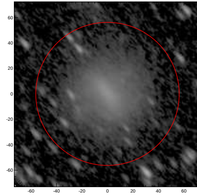
LEDA: pa,inc= 130.7 63.7
