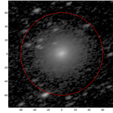
LEDA: pa,inc= 21.2 62.5
