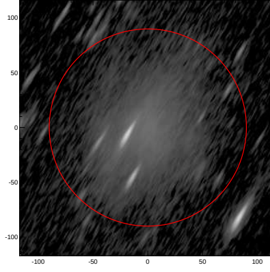
LEDA: pa,inc= 59.8 78.4
