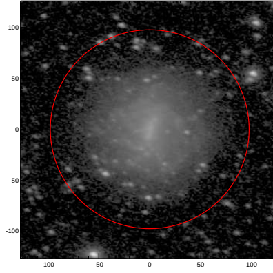
LEDA: pa,inc= 167.6 49.4
