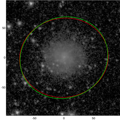
ESO576-017
