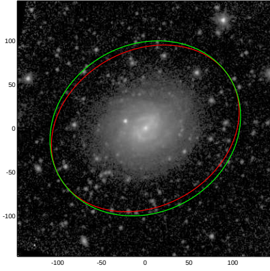
ESO404-012
