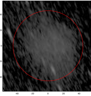
LEDA: pa,inc= 113.1 74.2
