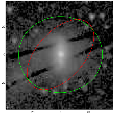
ESO509-026
