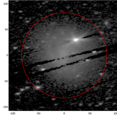
LEDA: pa,inc= 8.6 56.8
