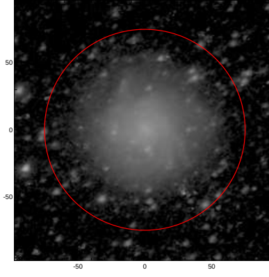
LEDA: pa,inc= 28.6 40.7
