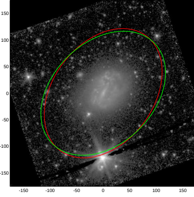
ESO576-032
