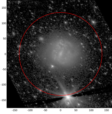
LEDA: pa,inc= 142.9 45.6
