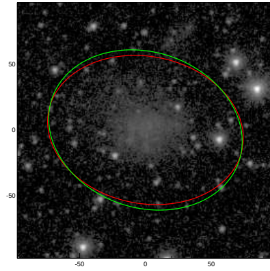
ESO159-025
