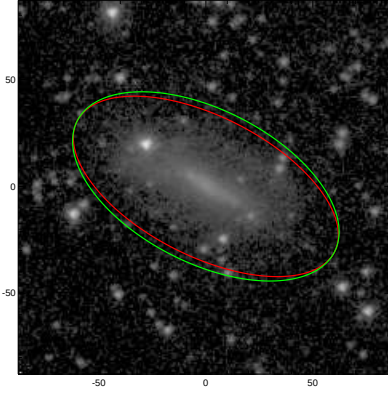
ESO048-017
