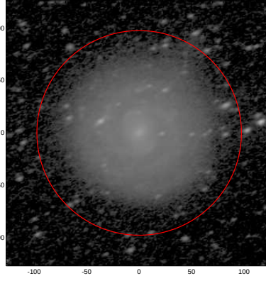
LEDA: pa,inc= 19.3 54.3
