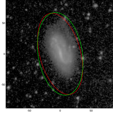
ESO404-003
