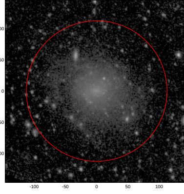
LEDA: pa,inc= 121.2 33.9
