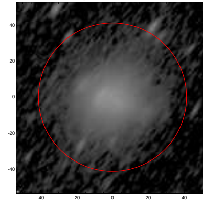
LEDA: pa,inc= 54.3 67.6
