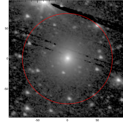
LEDA: pa,inc= 157.0 43.2
