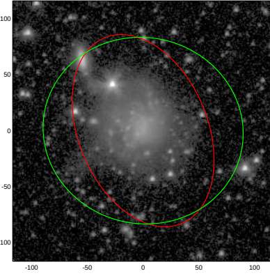
ESO234-049
