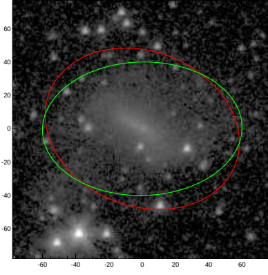
ESO234-043
