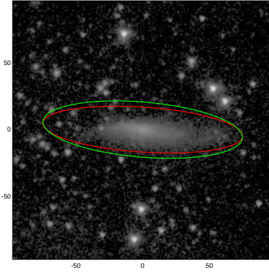
ESO444-033
