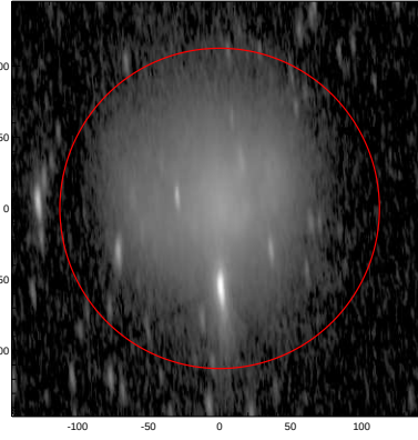
LEDA: pa,inc= 94.0 77.3
