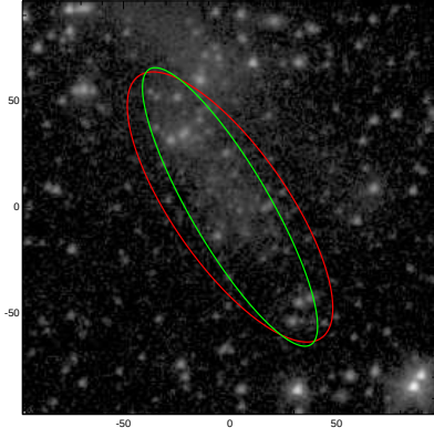
ESO540-031
