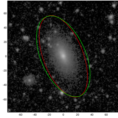
ESO548-023
