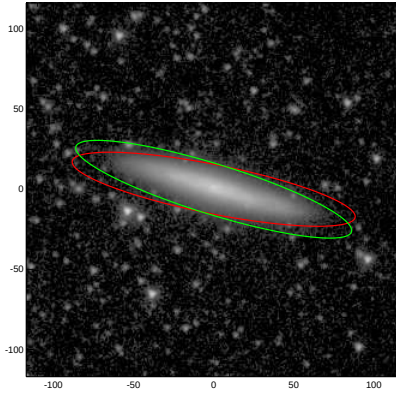
ESO580-029
