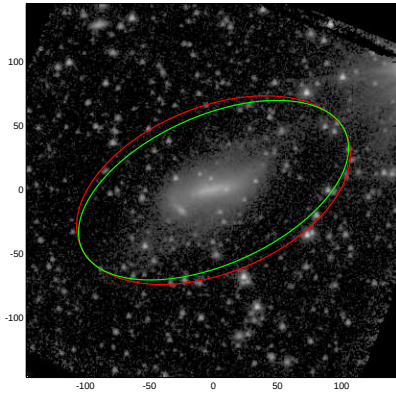
ESO340-017
