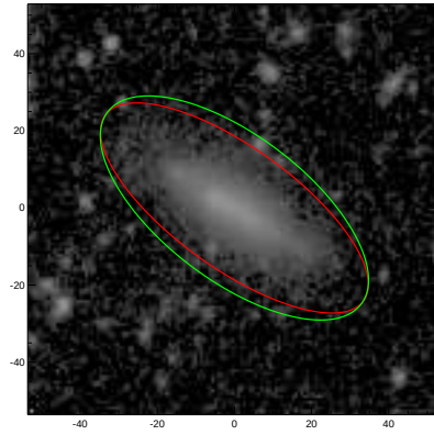
ESO482-013
