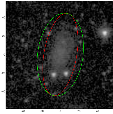
ESO249-026
