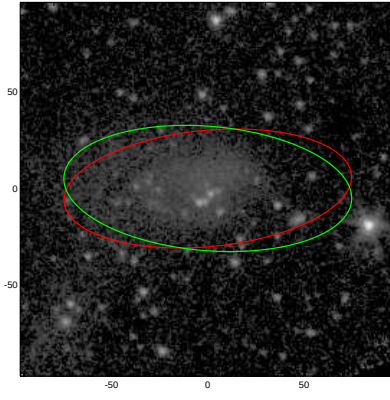
ESO576-059
