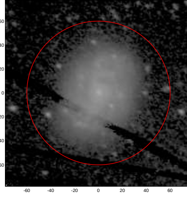
LEDA: pa,inc= 153.2 41.7
