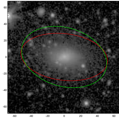
ESO570-019
