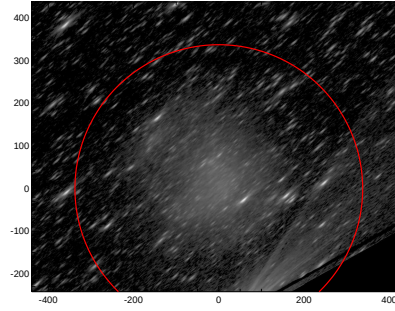
LEDA: pa,inc= 40.2 76.5
