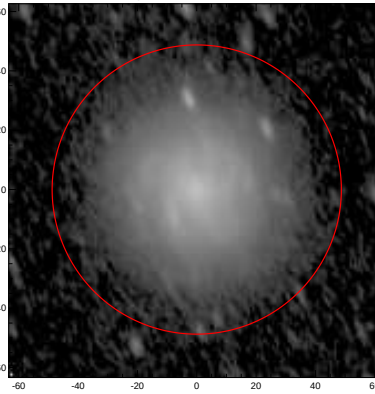
LEDA: pa,inc= 113.6 60.5
