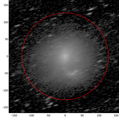
LEDA: pa,inc= 19.8 73.1
