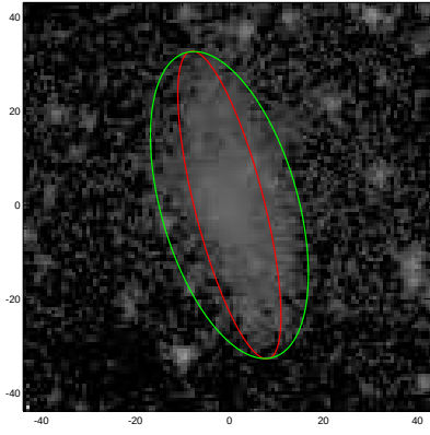
ESO507-065
