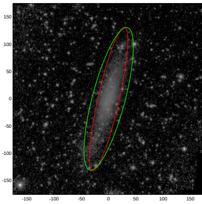
ESO481-014
