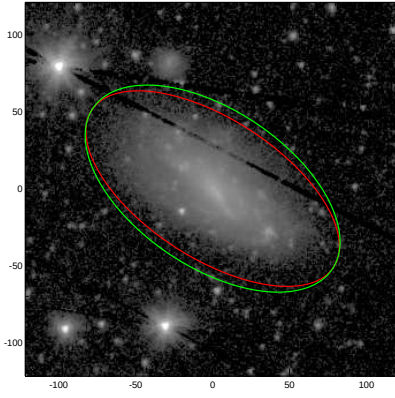
ESO479-004
