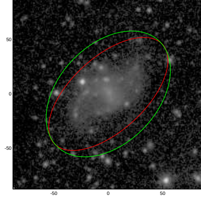
ESO532-022
