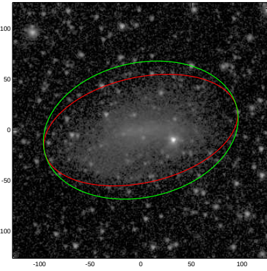
ESO572-030
