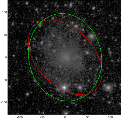
ESO150-005
