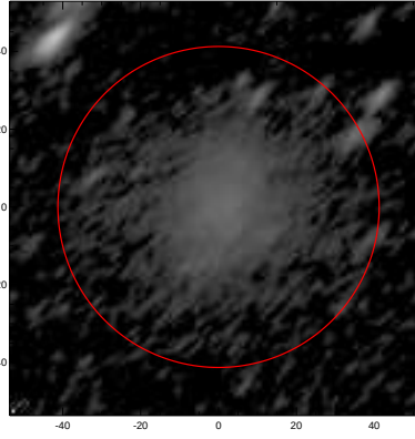
LEDA: pa,inc= 45.5 66.0
