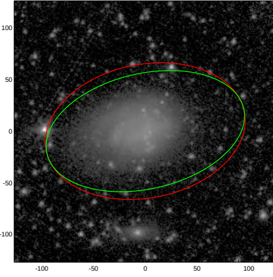
ESO544-030
