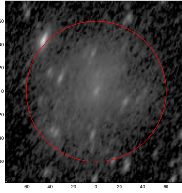
LEDA: pa,inc= 66.5 63.5
