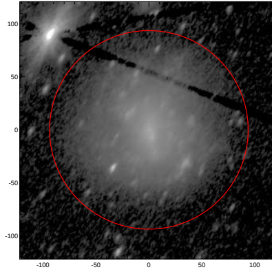
LEDA: pa,inc= 57.0 61.2
