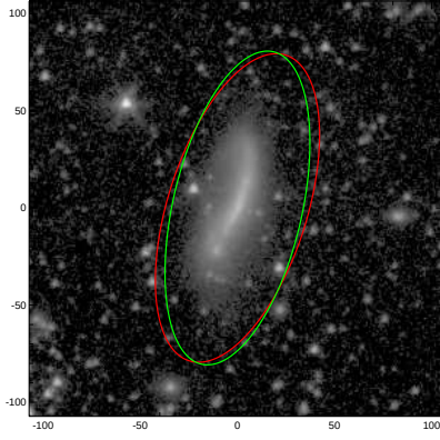
ESO342-013
