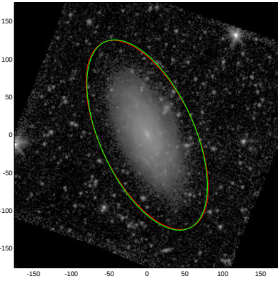
ESO541-004
