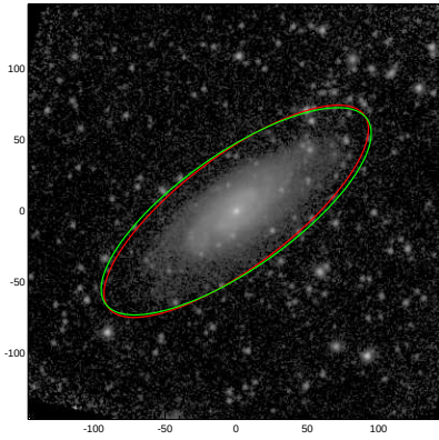
ESO404-027
