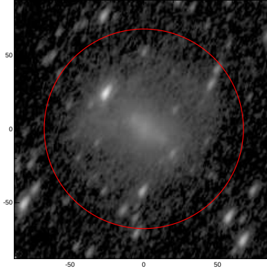
LEDA: pa,inc= 63.1 61.1
