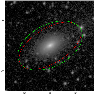
ESO466-036
