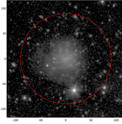
LEDA: pa,inc= 999.0 23.6
