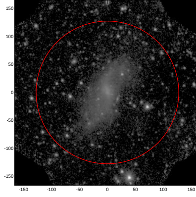
LEDA: pa,inc= 999.0 24.2
