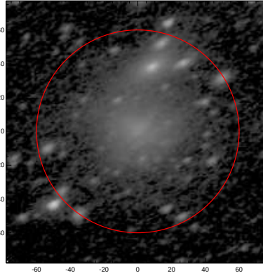
LEDA: pa,inc= 26.5 53.8
