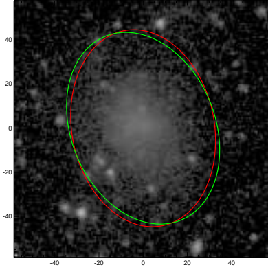
ESO422-005
