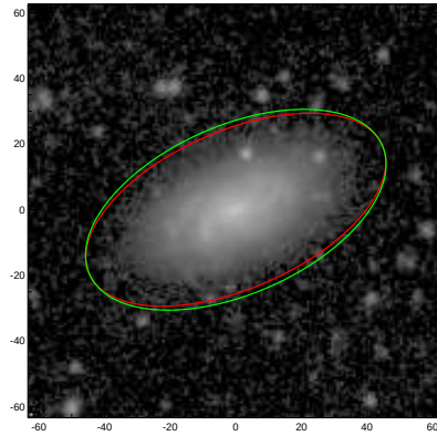
ESO533-028
