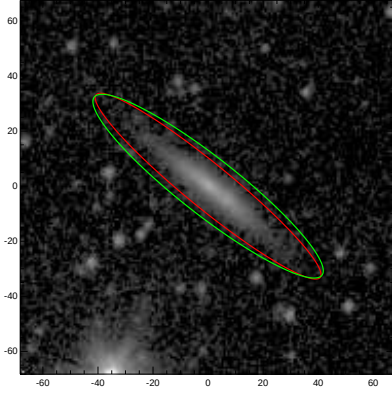
ESO536-003
