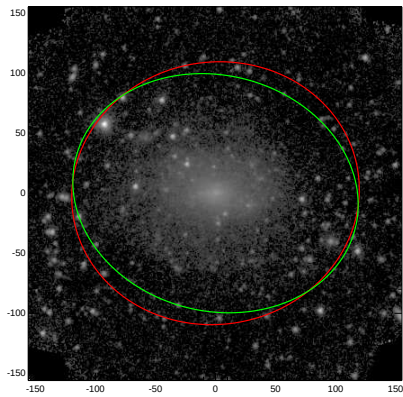
ESO422-041
