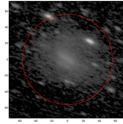
LEDA: pa,inc= 154.7 65.1
