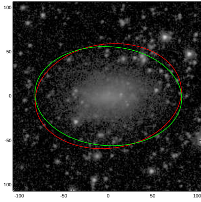
ESO120-012
