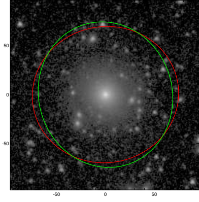
ESO440-037
