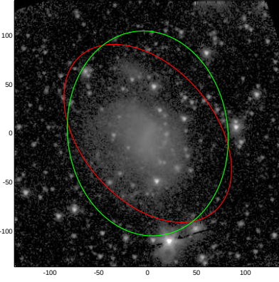
ESO440-046
