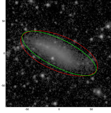
ESO305-017
