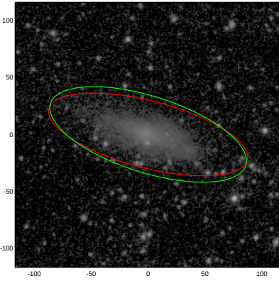
ESO601-025
