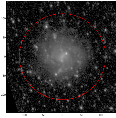
LEDA: pa,inc= 105.0 34.1
