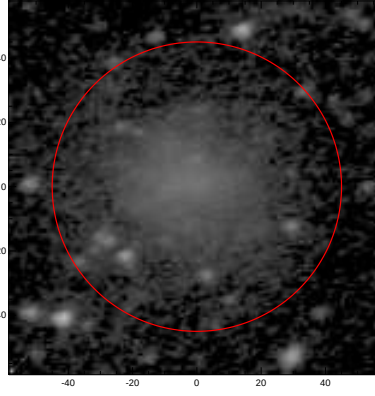
LEDA: pa,inc= 11.1 44.3
