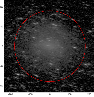
LEDA: pa,inc= 166.0 69.7
