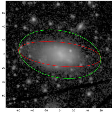
ESO441-017
