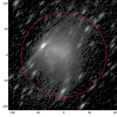
LEDA: pa,inc= 48.6 68.9
