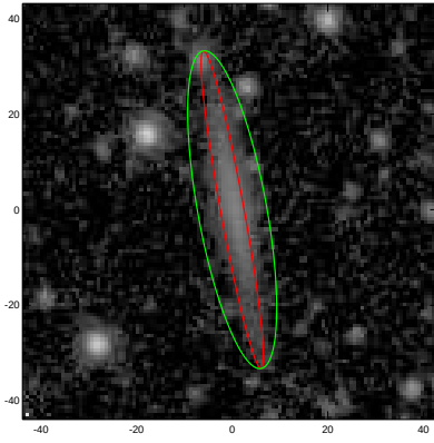
ESO506-018
