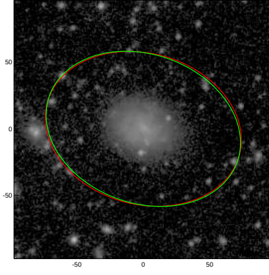
ESO602-030
