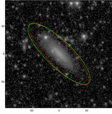
ESO572-022
