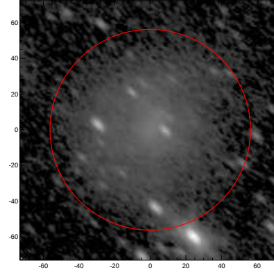
LEDA: pa,inc= 137.9 59.6
