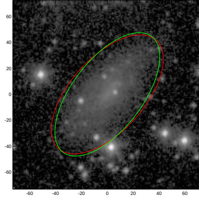
ESO400-025
