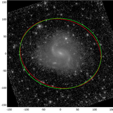
ESO508-024
