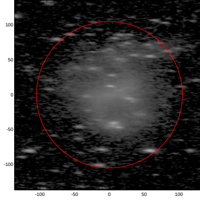
LEDA: pa,inc= 177.6 74.2
