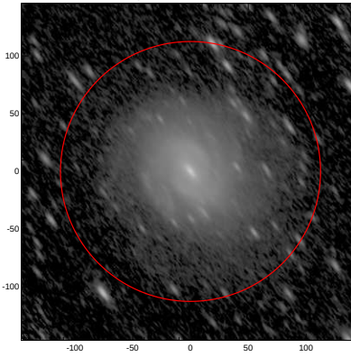
LEDA: pa,inc= 127.0 69.7
