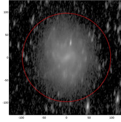
LEDA: pa,inc= 85.7 70.3
