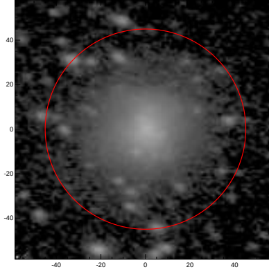
LEDA: pa,inc= 167.6 48.6
