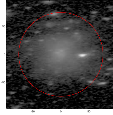
LEDA: pa,inc= 6.2 68.0
