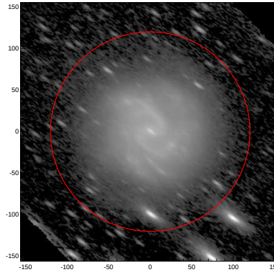
LEDA: pa,inc= 144.7 70.1
