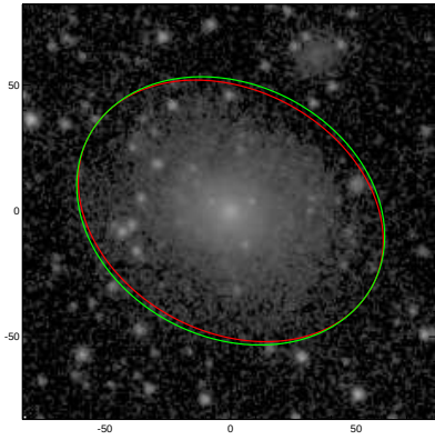
ESO440-049
