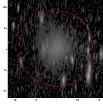
LEDA: pa,inc= 88.2 73.4
