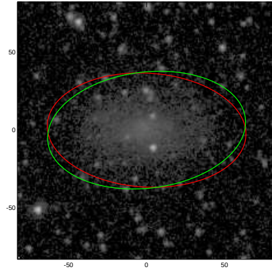
ESO480-025
