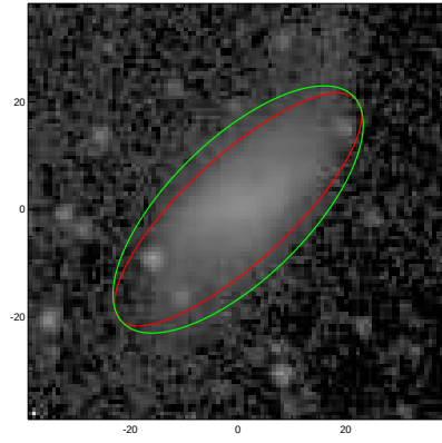
ESO548-016
