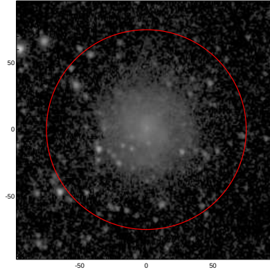
LEDA: pa,inc= 999.0 27.2
