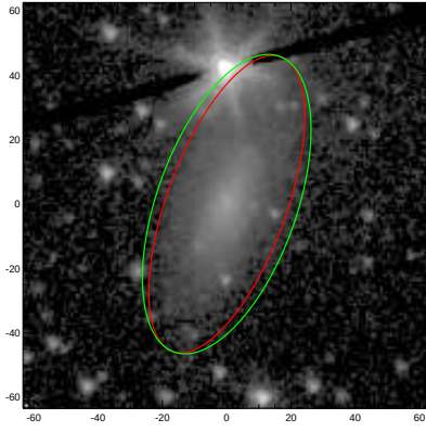
ESO582-004
