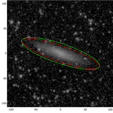
ESO572-049
