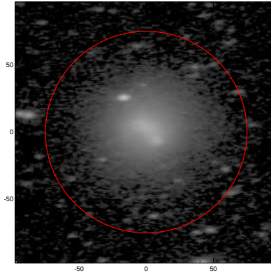
LEDA: pa,inc= 2.3 62.3
