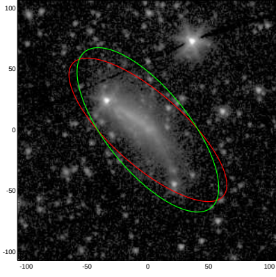
ESO508-019
