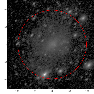
LEDA: pa,inc= 43.9 49.9
