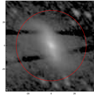
LEDA: pa,inc= 138.0 55.8
