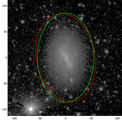
ESO482-035
