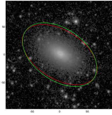
ESO358-025
