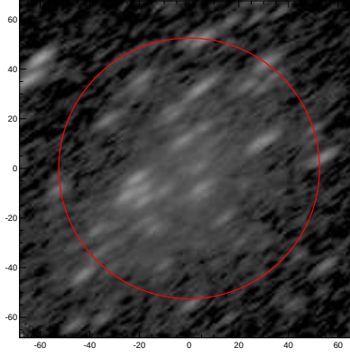
LEDA: pa,inc= 35.9 70.4
