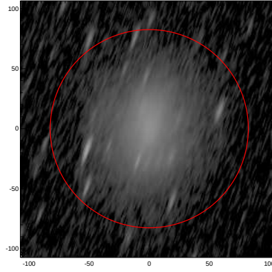
LEDA: pa,inc= 71.1 78.9
