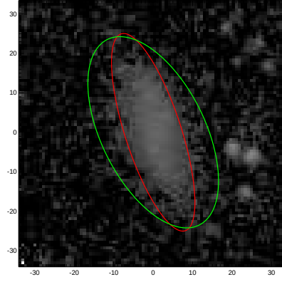
ESO359-022
