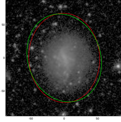
ESO079-007
