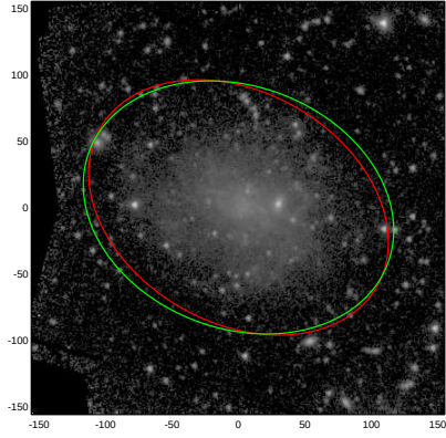
ESO421-019
