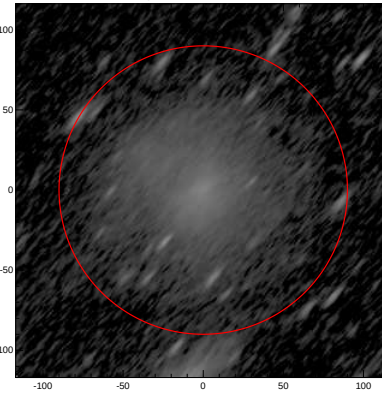
LEDA: pa,inc= 48.4 74.2
