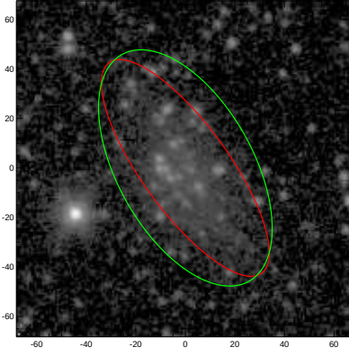
ESO444-078
