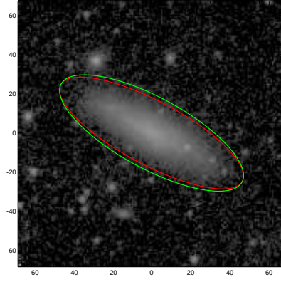
ESO482-011
