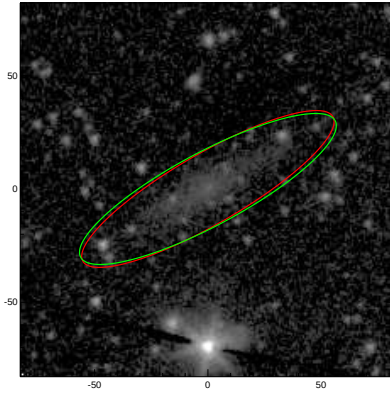
ESO410-012
