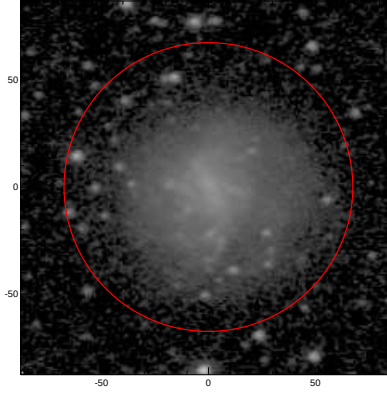
LEDA: pa,inc= 2.6 38.1
