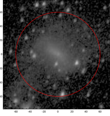
LEDA: pa,inc= 68.8 39.2
