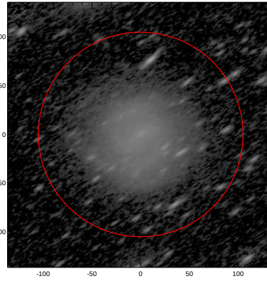
LEDA: pa,inc= 33.0 67.7
