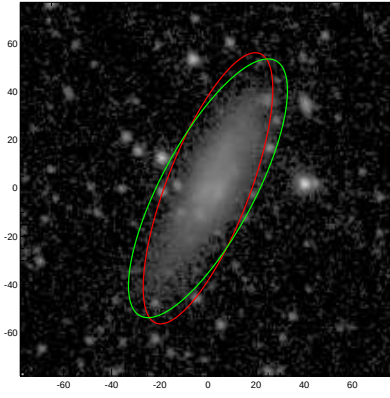
ESO441-014
