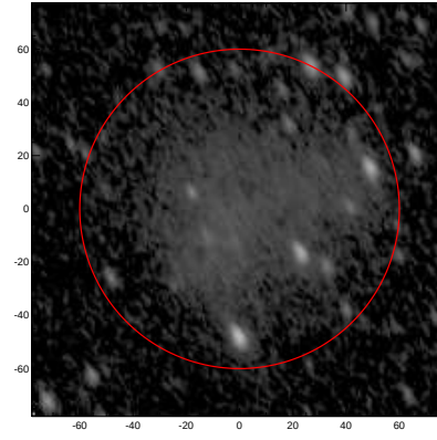
LEDA: pa,inc= 116.7 59.5
