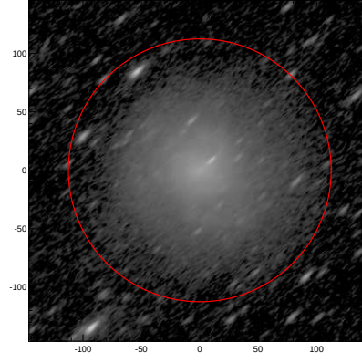
LEDA: pa,inc= 41.5 69.9
