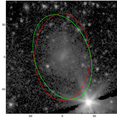
ESO506-029
