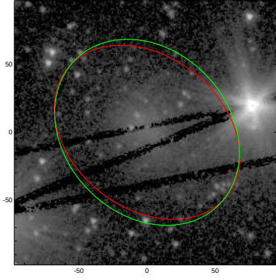
ESO501-079
