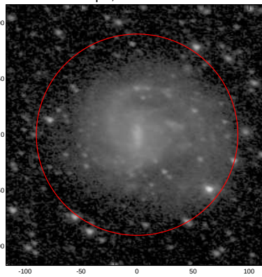
LEDA: pa,inc= 166.6 42.6
