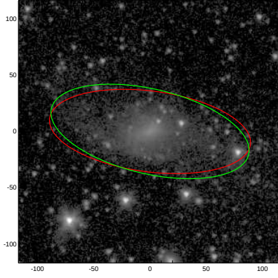
ESO440-004
