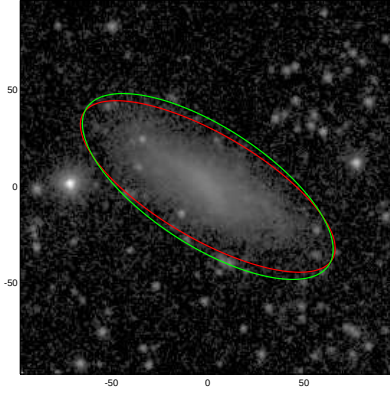
ESO298-015
