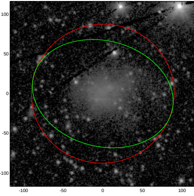
ESO505-002
