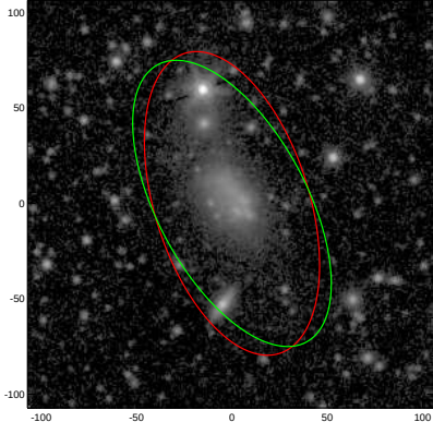
ESO572-034
