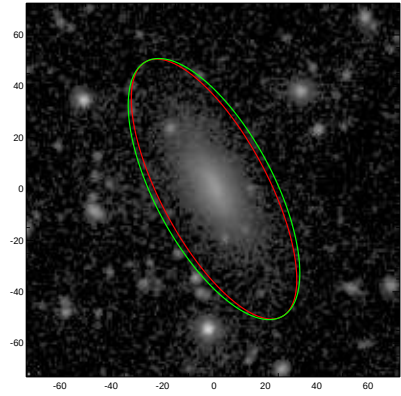
ESO357-025
