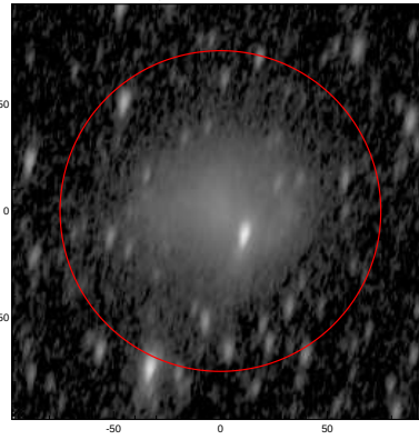
LEDA: pa,inc= 77.6 66.3
