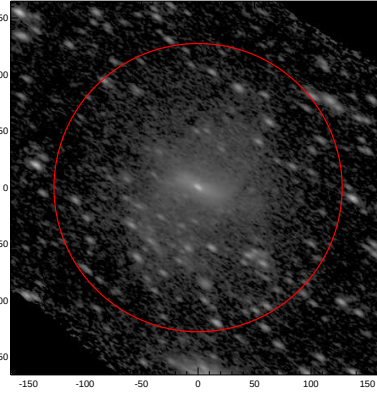
LEDA: pa,inc= 146.7 63.4
