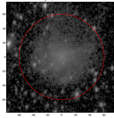
LEDA: pa,inc= 82.9 42.4
