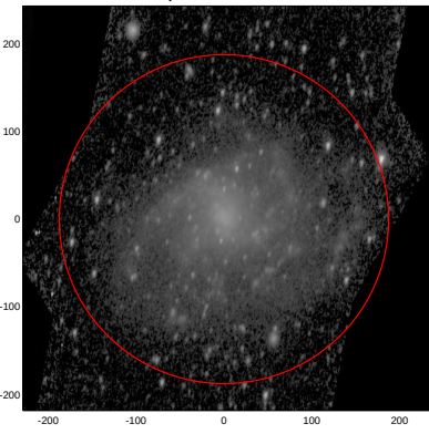
LEDA: pa,inc= 81.7 56.0
