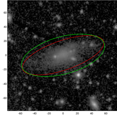
ESO532-014
