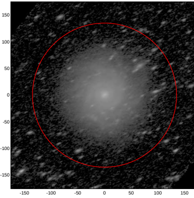
LEDA: pa,inc= 25.4 62.5
