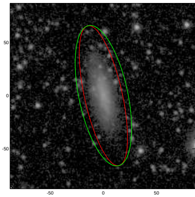
ESO505-008
