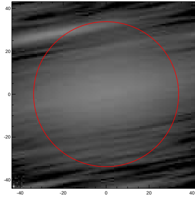
LEDA: pa,inc= 10.3 85.8
