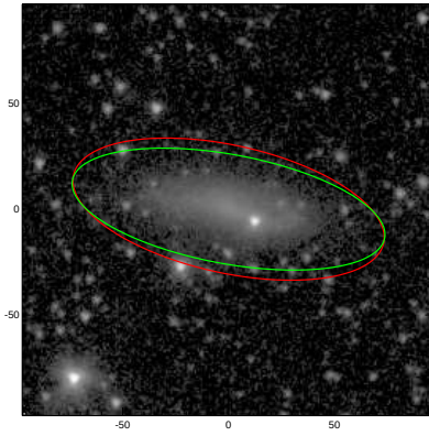
ESO502-016
