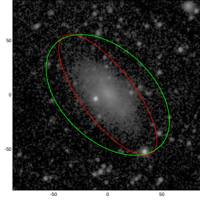
ESO403-024
