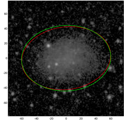
ESO358-005
