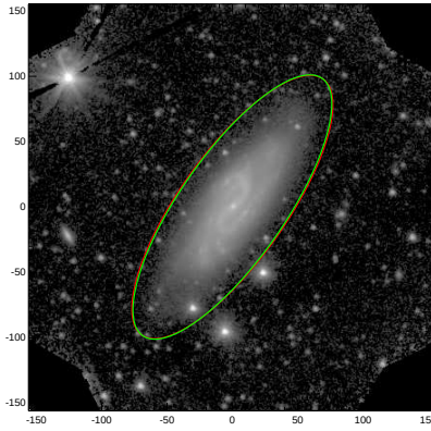
ESO027-008
