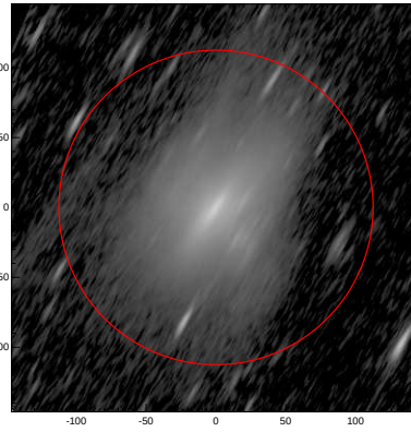
LEDA: pa,inc= 60.2 78.8
