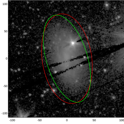
ESO438-017
