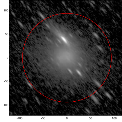
LEDA: pa,inc= 131.5 72.4
