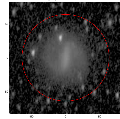
LEDA: pa,inc= 85.6 56.5
