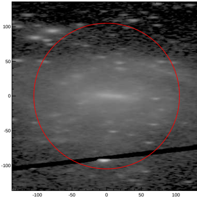
LEDA: pa,inc= 0.2 74.0
