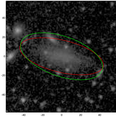
ESO502-023
