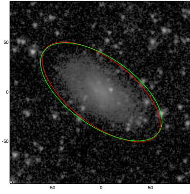
ESO508-051
