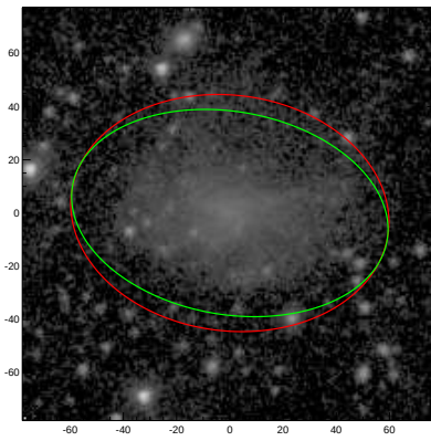
ESO358-054
