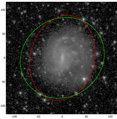
ESO443-069
