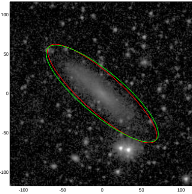
ESO302-009
