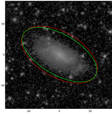
ESO237-052
