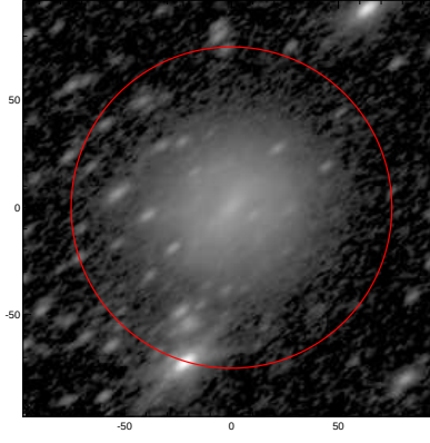
LEDA: pa,inc= 37.8 62.6
