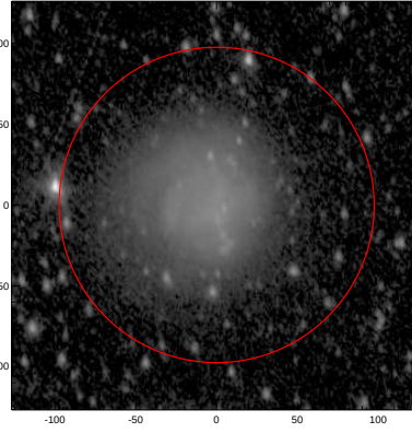
LEDA: pa,inc= 101.0 48.5
