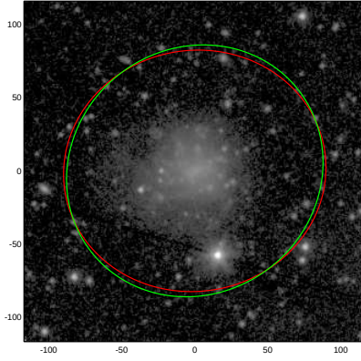
ESO341-032
