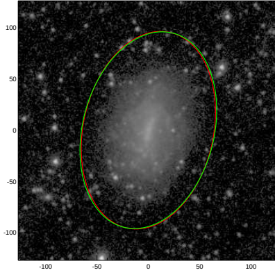
ESO013-016
