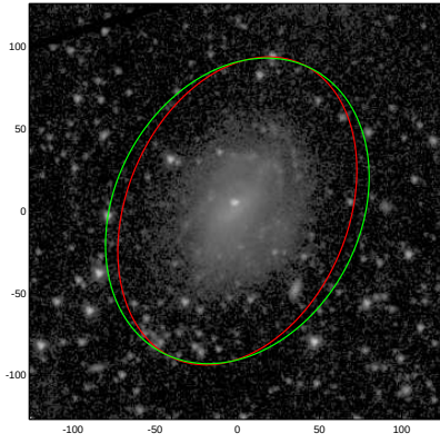
ESO580-022
