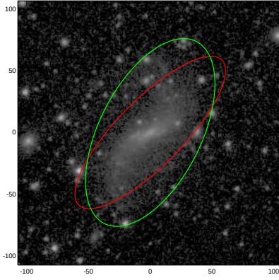
ESO289-026
