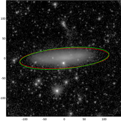
ESO361-015
