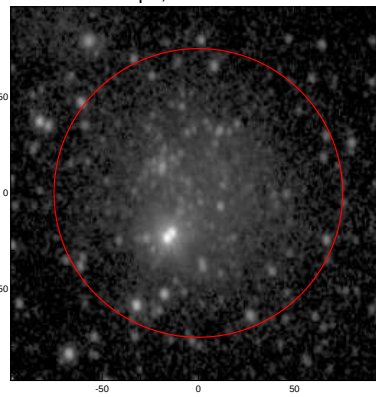
LEDA: pa,inc= 999.0 33.5
