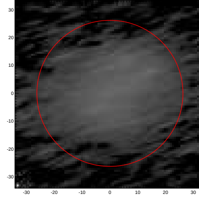
LEDA: pa,inc= 18.0 74.3
