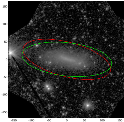
ESO085-014
