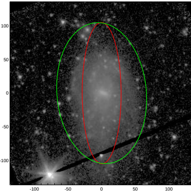
ESO576-050
