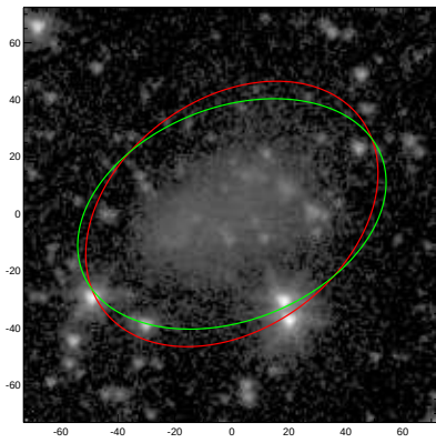
ESO508-015
