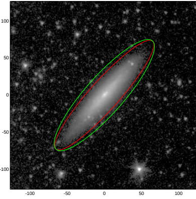
ESO509-074
