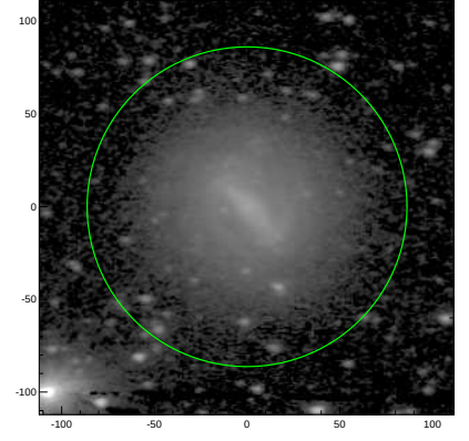
S4G: pa,inc= 0.7 50.7
