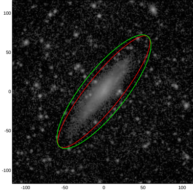
ESO289-048
