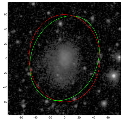
ESO358-015
