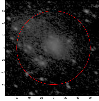
LEDA: pa,inc= 151.2 49.6
