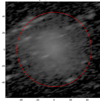
LEDA: pa,inc= 18.7 70.5
