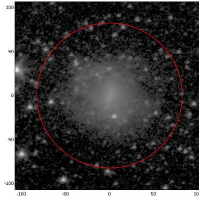
LEDA: pa,inc= 8.5 29.4
