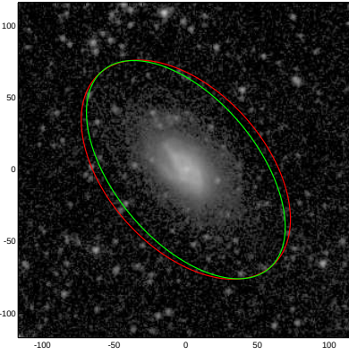
ESO407-014
