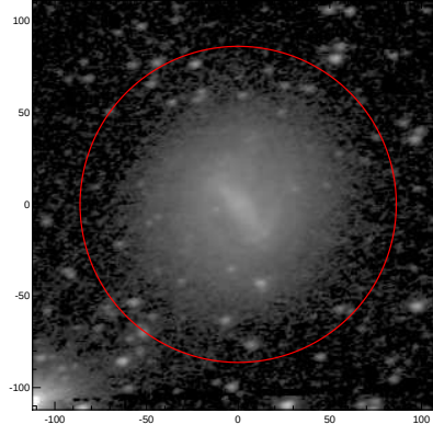
LEDA: pa,inc= 10.2 49.2
