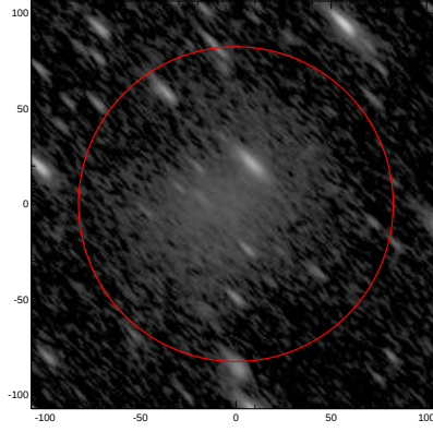
LEDA: pa,inc= 135.1 71.6
