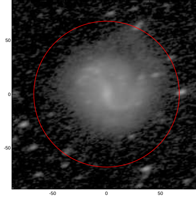
LEDA: pa,inc= 15.2 60.8
