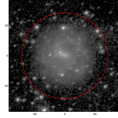
LEDA: pa,inc= 41.1 29.9
