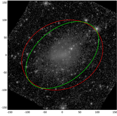
ESO357-012
