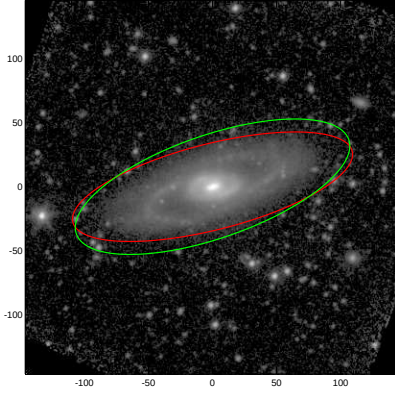
ESO402-026
