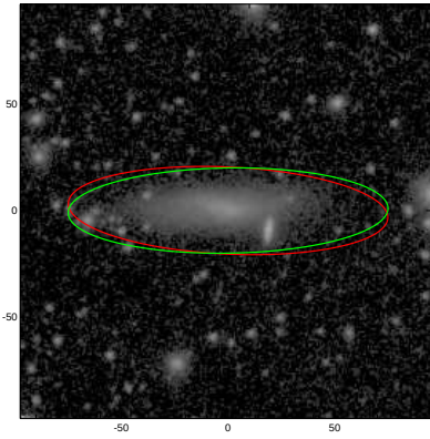
ESO291-024
