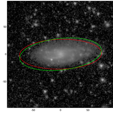
ESO576-003
