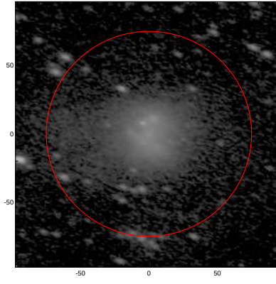
LEDA: pa,inc= 160.7 57.8
