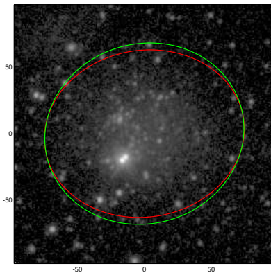
ESO407-018
