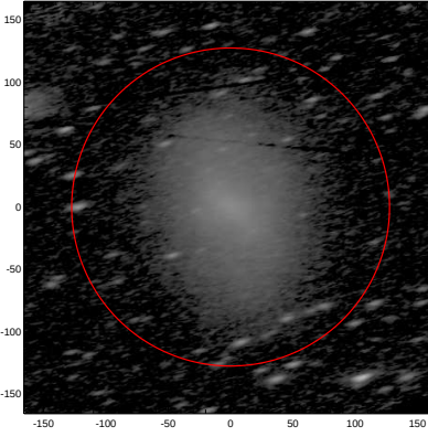
LEDA: pa,inc= 14.8 71.1
