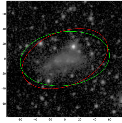
ESO601-031
