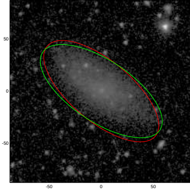
ESO545-002
