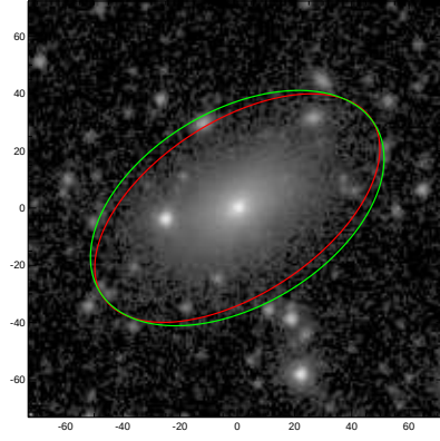
ESO286-044
