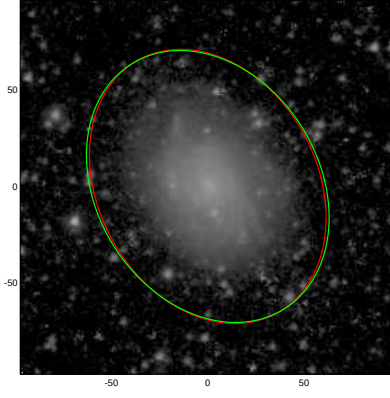
ESO420-009
