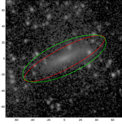
ESO572-024
