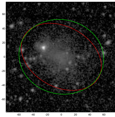
ESO547-020
