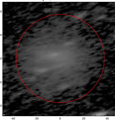
LEDA: pa,inc= 16.4 70.6
