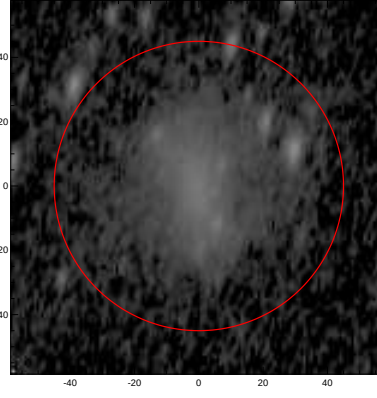
LEDA: pa,inc= 79.7 62.8
