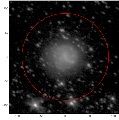
LEDA: pa,inc= 145.9 43.9
