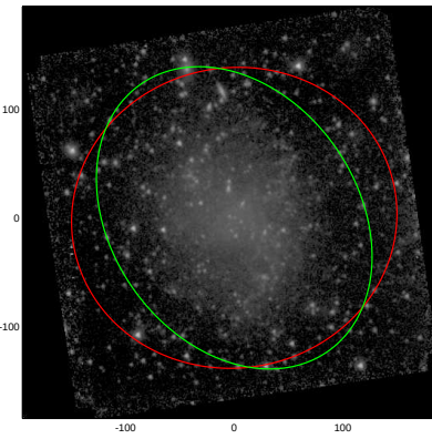
ESO362-009
