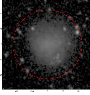
LEDA: pa,inc= 999.0 23.0
