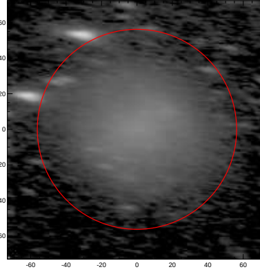
LEDA: pa,inc= 172.6 72.6
