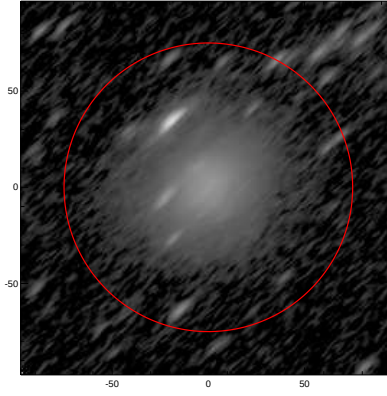
LEDA: pa,inc= 43.8 73.1
