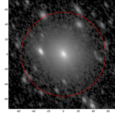
LEDA: pa,inc= 123.4 57.5
