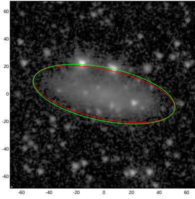
ESO505-009
