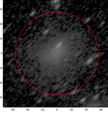
LEDA: pa,inc= 42.1 65.2
