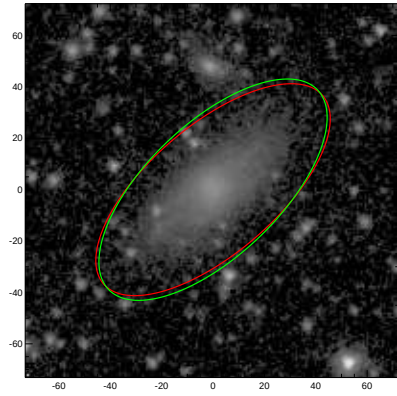
ESO508-034
