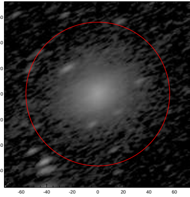
LEDA: pa,inc= 28.0 68.2
