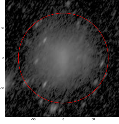
LEDA: pa,inc= 59.7 68.7
