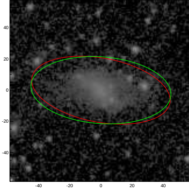
ESO541-005
