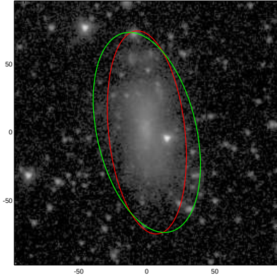
ESO440-044
