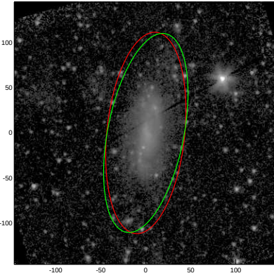
ESO442-013
