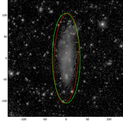
ESO362-019
