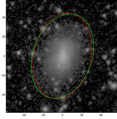
ESO249-008
