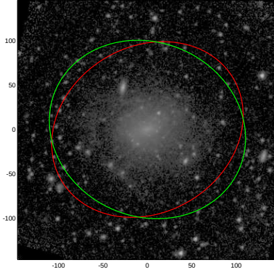
ESO345-046
