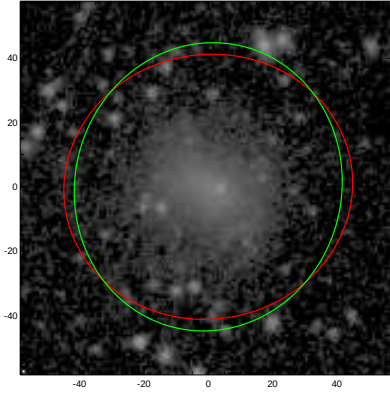
ESO298-023
