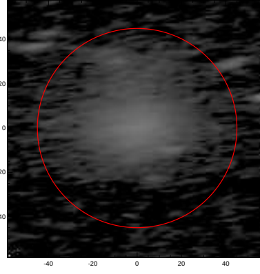
LEDA: pa,inc= 6.0 75.7
