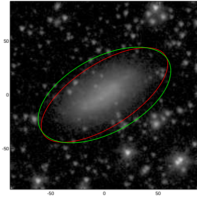
ESO503-022
