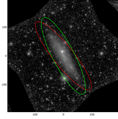
ESO149-001
