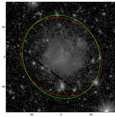
ESO410-018
