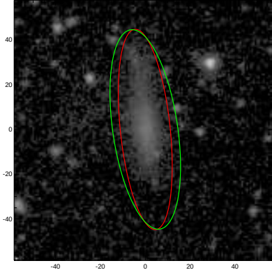
ESO302-021
