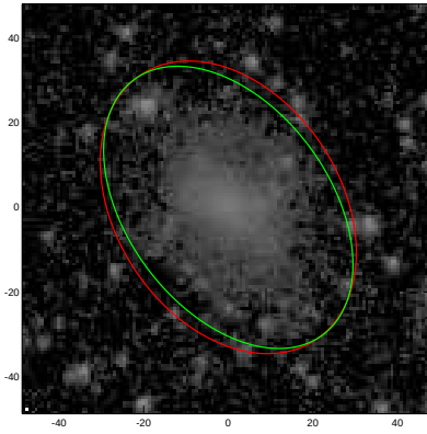
ESO549-035
