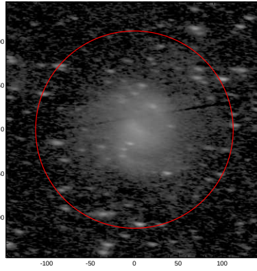
LEDA: pa,inc= 174.1 67.4
