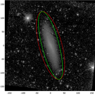
ESO248-002
