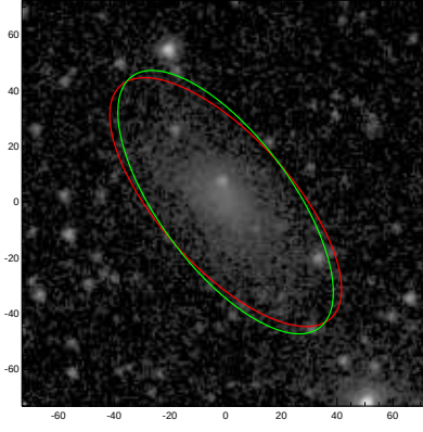
ESO486-003
