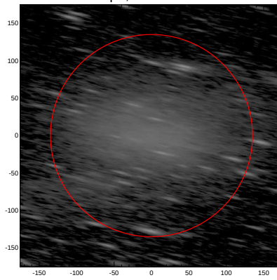
LEDA: pa,inc= 167.4 81.8
