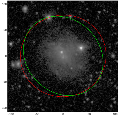
ESO548-005
