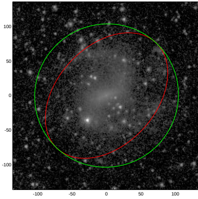
ESO485-021
