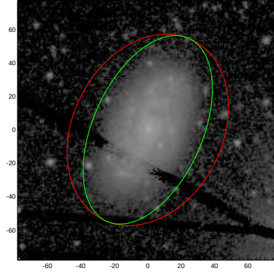
ESO355-026
