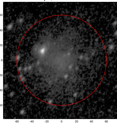
LEDA: pa,inc= 61.3 44.7
