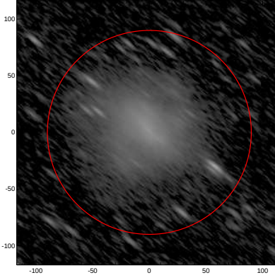
LEDA: pa,inc= 141.1 76.2
