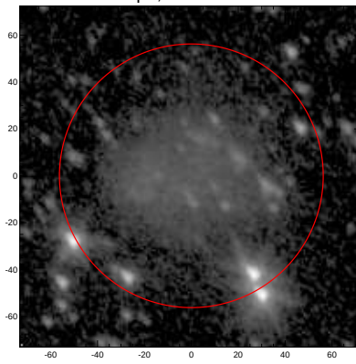
LEDA: pa,inc= 126.2 44.1
