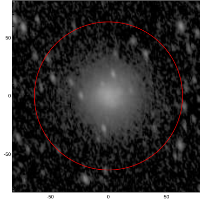
LEDA: pa,inc= 106.3 57.7
