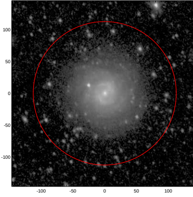
LEDA: pa,inc= 119.5 37.9
