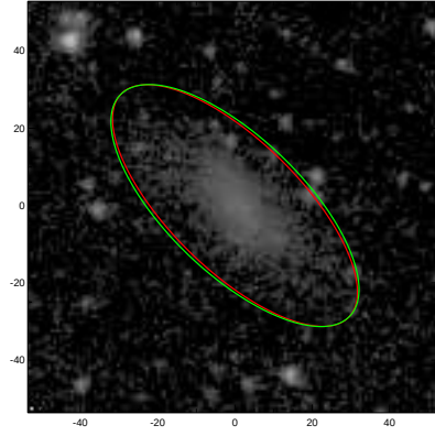
ESO483-008
