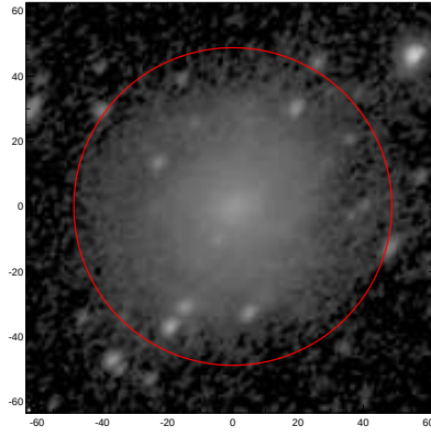
LEDA: pa,inc= 46.3 44.4
