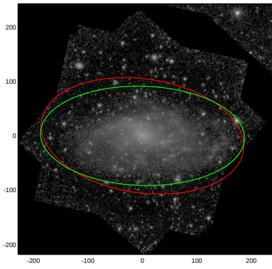
ESO054-021
