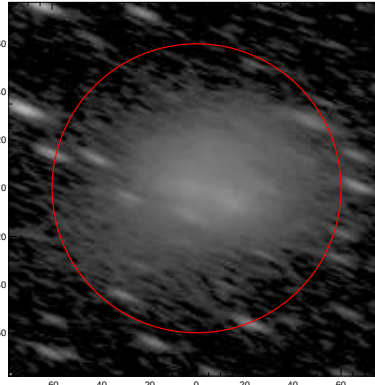
LEDA: pa,inc= 158.9 73.4
