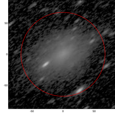
LEDA: pa,inc= 37.3 68.7
