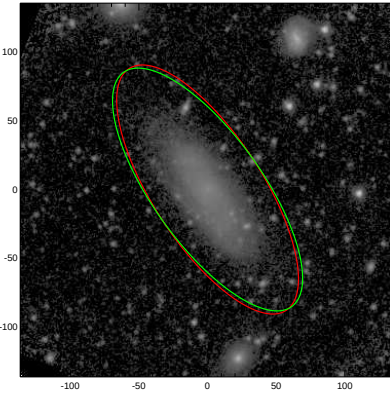
ESO407-009
