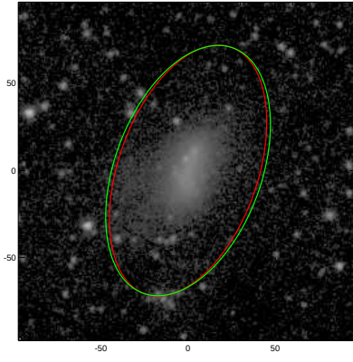
ESO358-020
