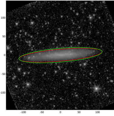
ESO508-011
