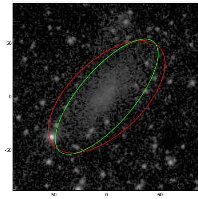
ESO420-006
