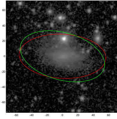
ESO408-012
