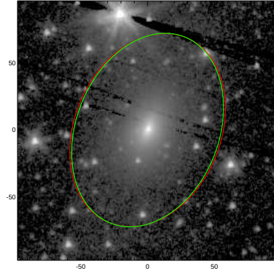
ESO399-025
