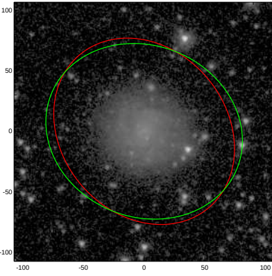
ESO504-028
