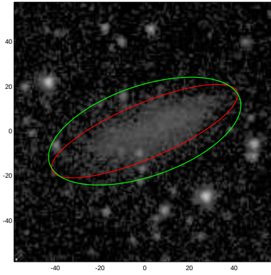
ESO546-034
