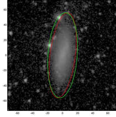
ESO551-031
