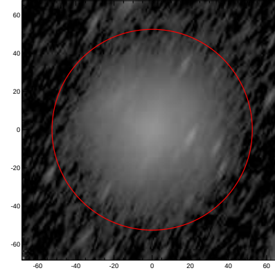
LEDA: pa,inc= 62.0 72.0
