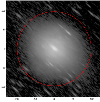
LEDA: pa,inc= 138.2 78.3
