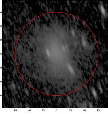
LEDA: pa,inc= 109.1 69.9
