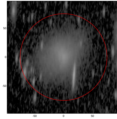
LEDA: pa,inc= 87.3 74.2
