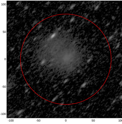
LEDA: pa,inc= 45.3 64.6
