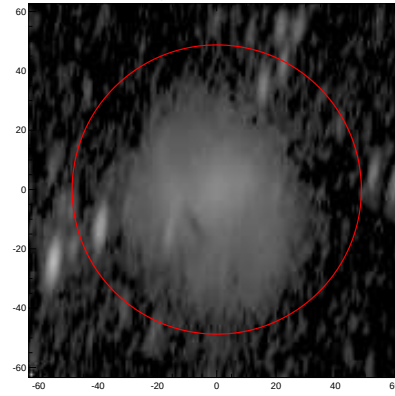
LEDA: pa,inc= 82.2 72.2
