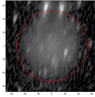
LEDA: pa,inc= 77.8 70.2
