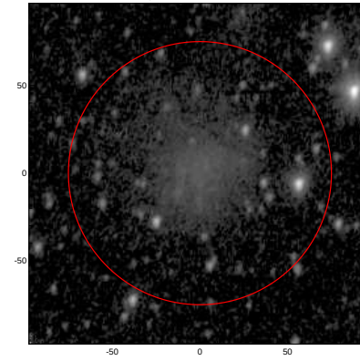
LEDA: pa,inc= 79.1 41.9
