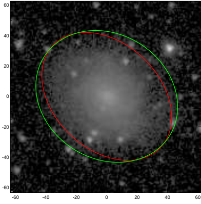
ESO502-020
