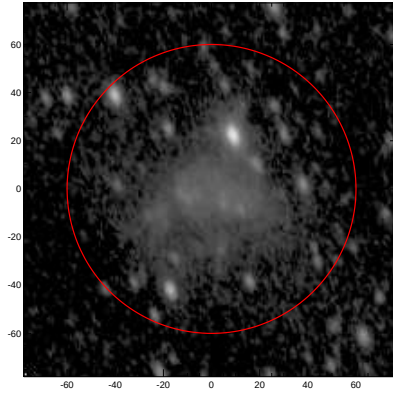
LEDA: pa,inc= 112.0 53.0
