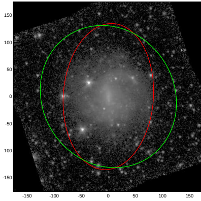
ESO440-011
