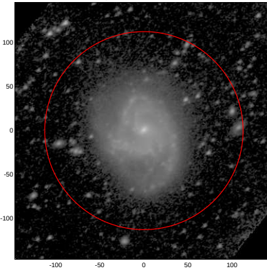
LEDA: pa,inc= 32.4 42.3
