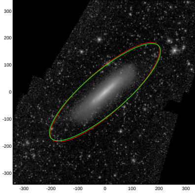
ESO358-063
