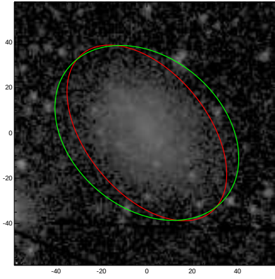
ESO547-005
