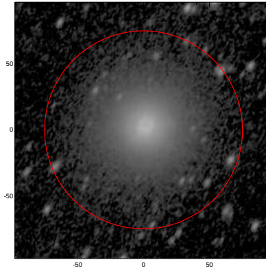
LEDA: pa,inc= 58.2 54.4
