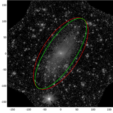
ESO347-029
