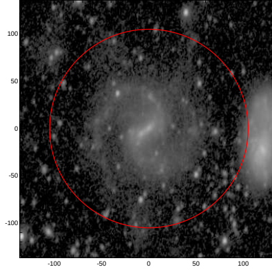
LEDA: pa,inc= 80.8 47.5
