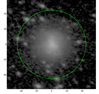
S4G: pa,inc= -19.1 47.3
