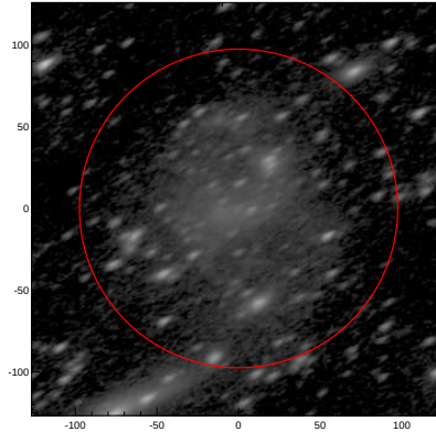
LEDA: pa,inc= 28.0 62.7
