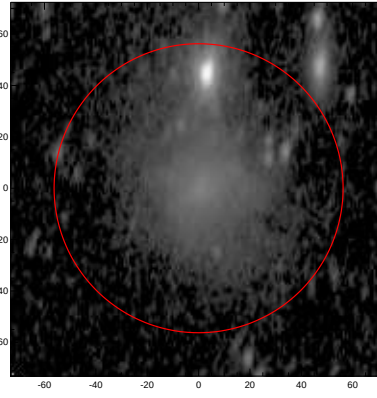
LEDA: pa,inc= 87.0 59.3
