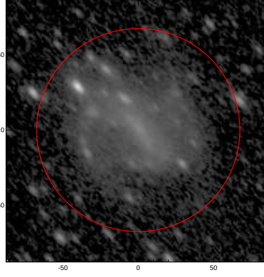
LEDA: pa,inc= 132.5 59.8
