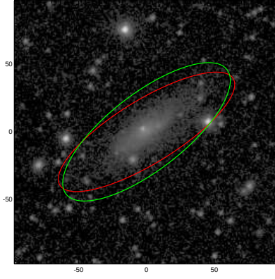
ESO404-017
