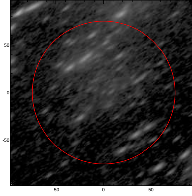
LEDA: pa,inc= 34.8 68.9
