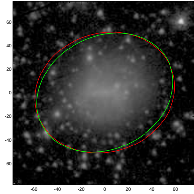
ESO418-009
