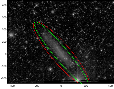
ESO154-023
