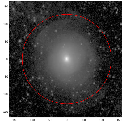
LEDA: pa,inc= 999.0 23.0
