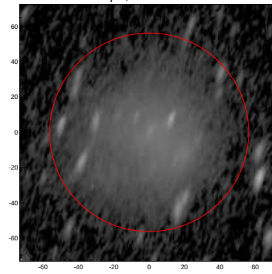
LEDA: pa,inc= 71.9 67.8
