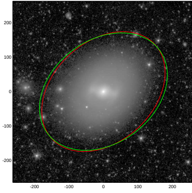
NGC0936
