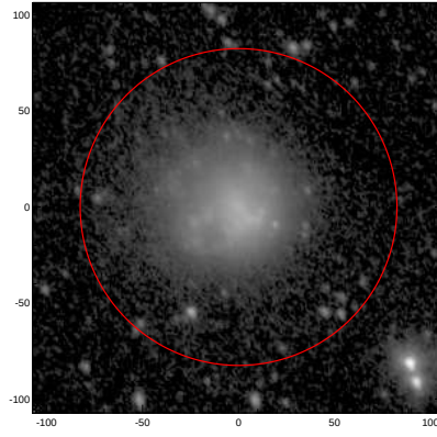
LEDA: pa,inc= 120.7 42.2
