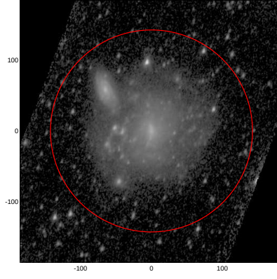
LEDA: pa,inc= 71.7 48.6
