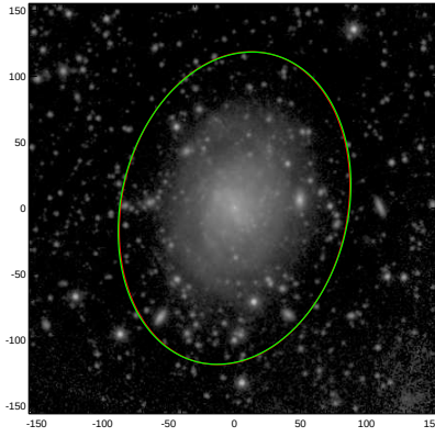
NGC0941
