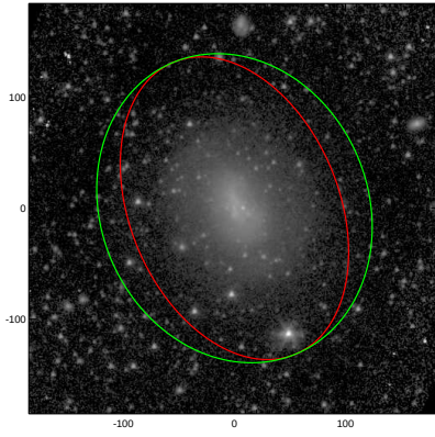
NGC0014
