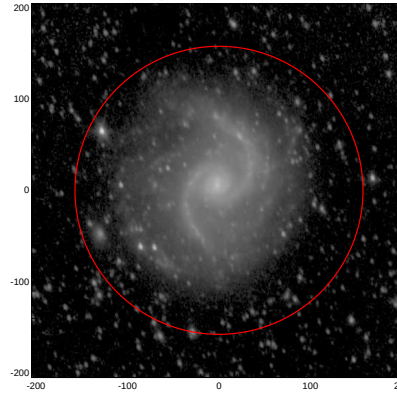
LEDA: pa,inc= 108.7 48.1
