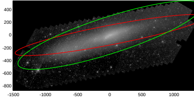
NGC0055
