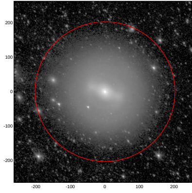
LEDA: pa,inc= 132.4 44.1
