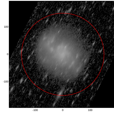
LEDA: pa,inc= 60.1 71.5
