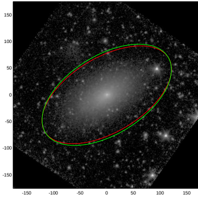
NGC0059
