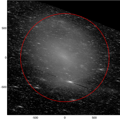
LEDA: pa,inc= 166.8 73.6
