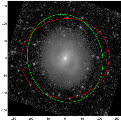
NGC0718
