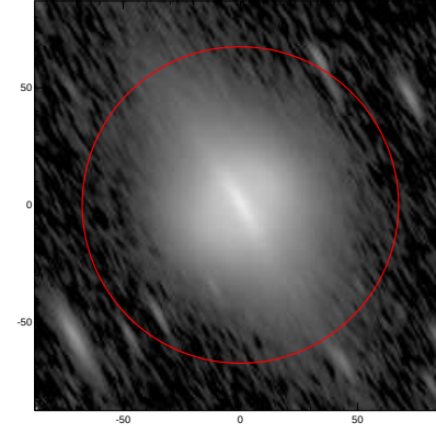
LEDA: pa,inc= 120.0 77.1
