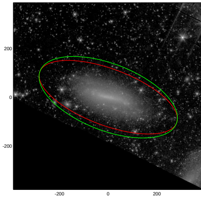
NGC0672
