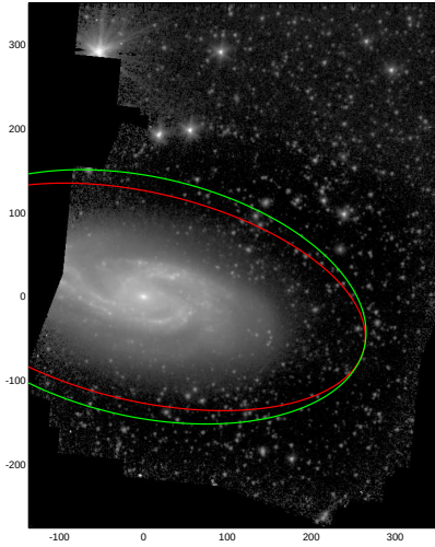
NGC0908
