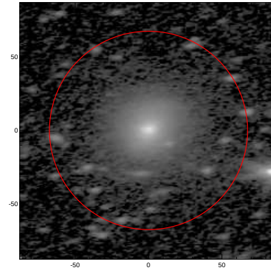
LEDA: pa,inc= 7.0 63.3
