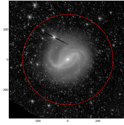
LEDA: pa,inc= 118.6 34.7
