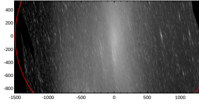
LEDA: pa,inc= 100.9 84.1
