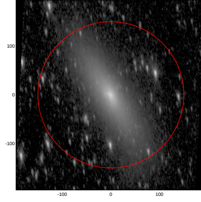
LEDA: pa,inc= 999.0 68.4
