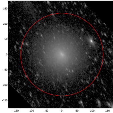
LEDA: pa,inc= 120.8 58.7
