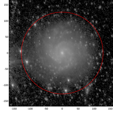
LEDA: pa,inc= 105.0 44.4
