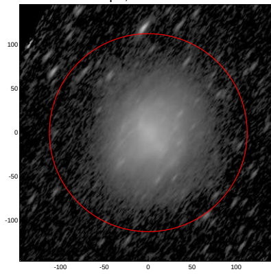
LEDA: pa,inc= 52.3 71.8
