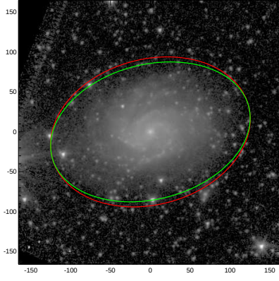
NGC0514
