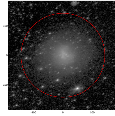
LEDA: pa,inc= 22.7 48.6
