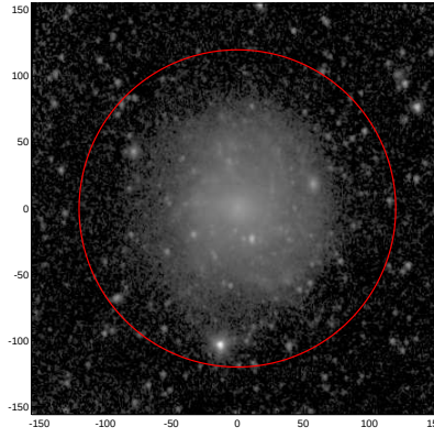
LEDA: pa,inc= 999.0 27.5
