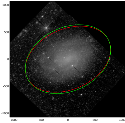
NGC0300
