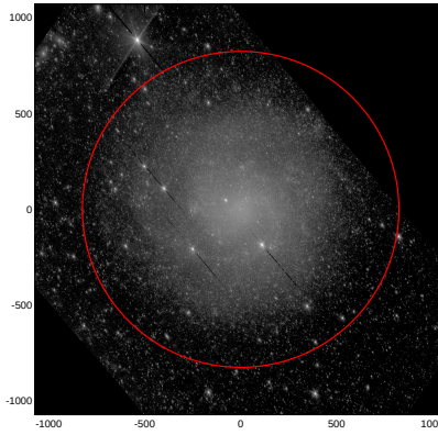
LEDA: pa,inc= 114.3 47.7
