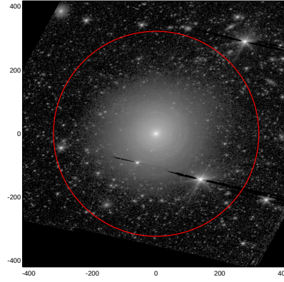
LEDA: pa,inc= 11.5 43.4
