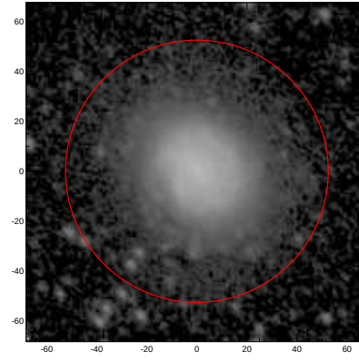
LEDA: pa,inc= 134.9 38.9
