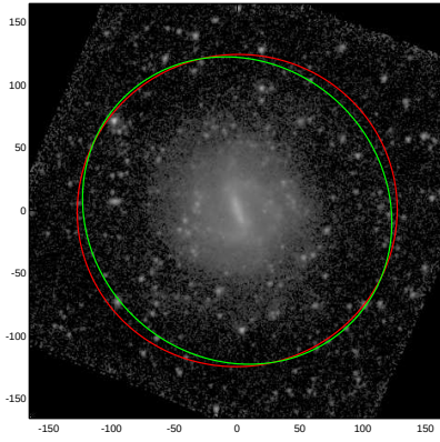
NGC0600
