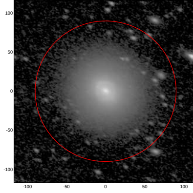
LEDA: pa,inc= 153.3 54.7
