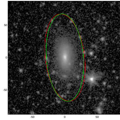
NGC0814
