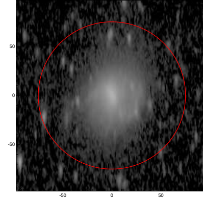
LEDA: pa,inc= 91.7 70.8
