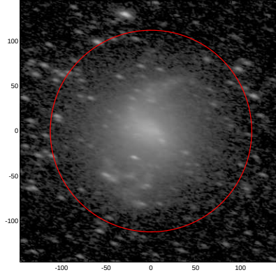
LEDA: pa,inc= 162.3 63.1
