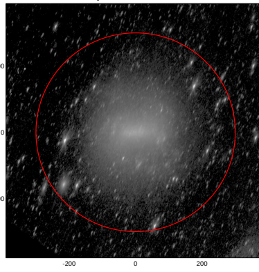
LEDA: pa,inc= 69.5 67.3
