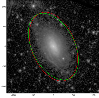
NGC0658
