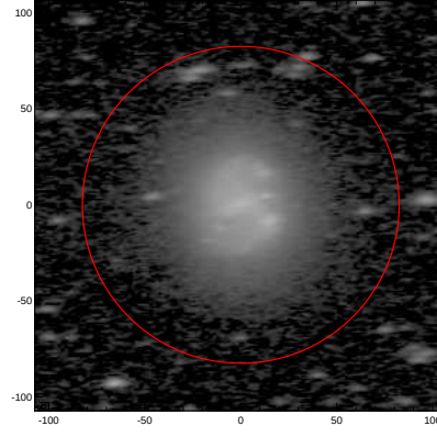
LEDA: pa,inc= 2.7 68.2
