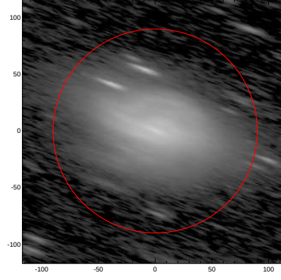
LEDA: pa,inc= 160.0 80.3
