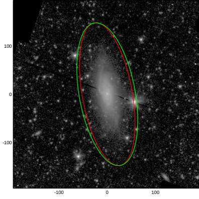
NGC0803
