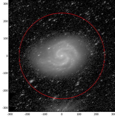
LEDA: pa,inc= 28.1 59.1
