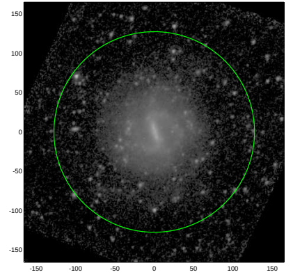
S4G: pa,inc= 47.1 22.4
