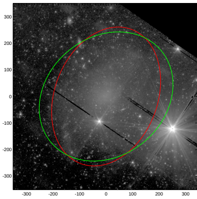
NGC0045
