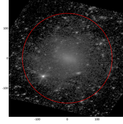
LEDA: pa,inc= 8.0 49.0
