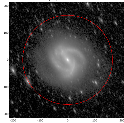
LEDA: pa,inc= 117.0 63.1
