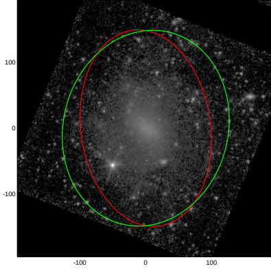
NGC0337A
