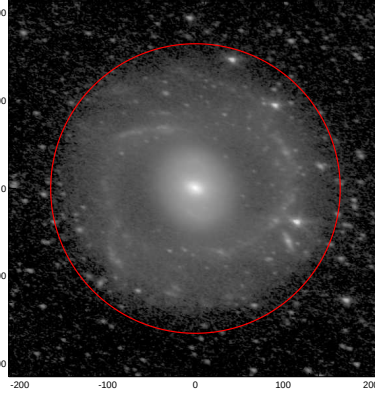
LEDA: pa,inc= 163.0 52.6
