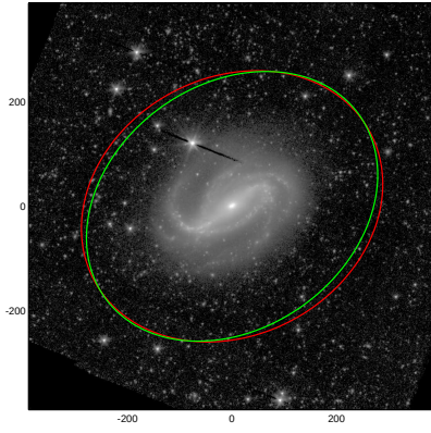
NGC0613
