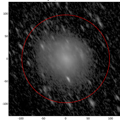
LEDA: pa,inc= 122.2 69.6
