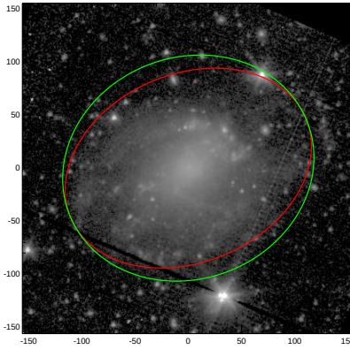
NGC0428
