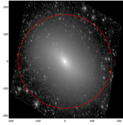
LEDA: pa,inc= 104.5 48.5
