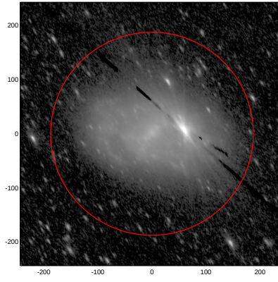
LEDA: pa,inc= 123.4 66.4
