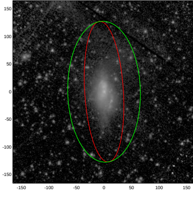
NGC0178
