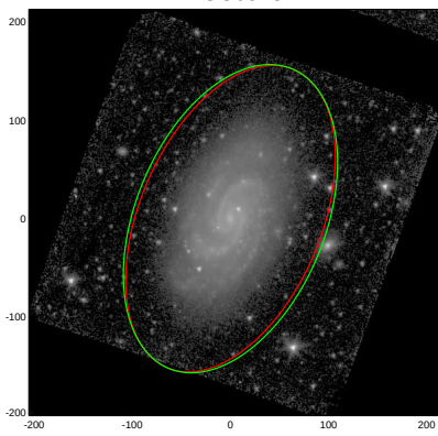
NGC0918
