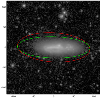
NGC0907
