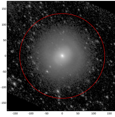
LEDA: pa,inc= 132.7 49.4
