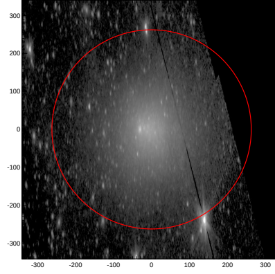
LEDA: pa,inc= 91.9 71.8
