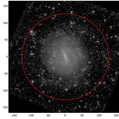
LEDA: pa,inc= 999.0 12.8
