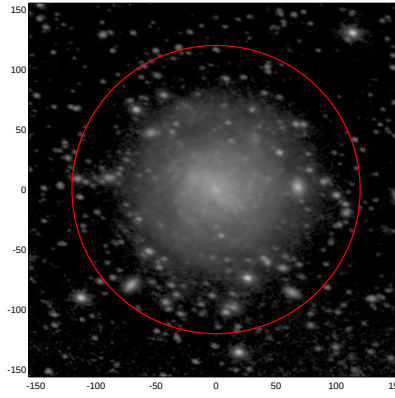
LEDA: pa,inc= 167.4 44.5
