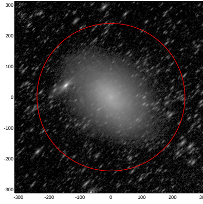
LEDA: pa,inc= 44.2 67.1
