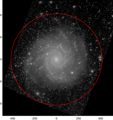
LEDA: pa,inc= 999.0 19.3
