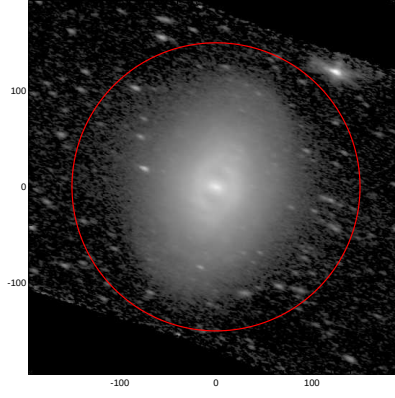
LEDA: pa,inc= 160.0 64.7
