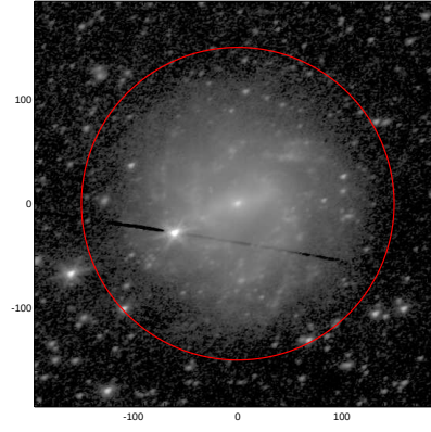
LEDA: pa,inc= 24.0 46.4
