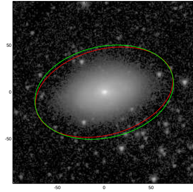
NGC0063
