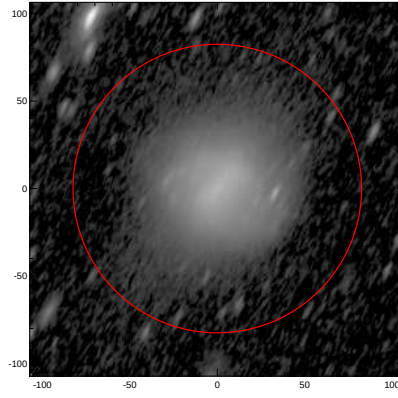
LEDA: pa,inc= 62.5 68.1
