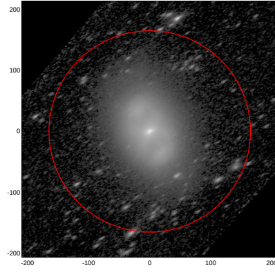
LEDA: pa,inc= 30.6 64.4
