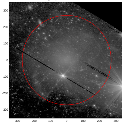
LEDA: pa,inc= 158.7 44.1
