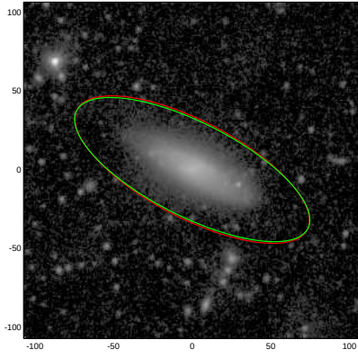
NGC0131
