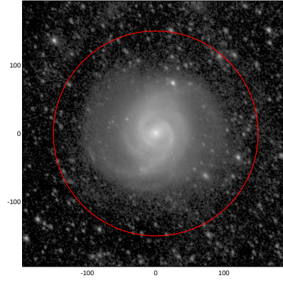
LEDA: pa,inc= 128.6 41.6
