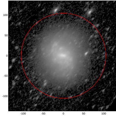
LEDA: pa,inc= 48.9 60.3
