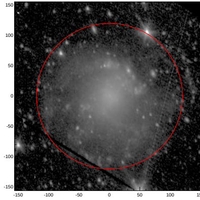
LEDA: pa,inc= 113.2 42.4
