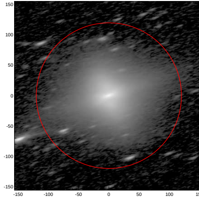
LEDA: pa,inc= 17.9 74.0
