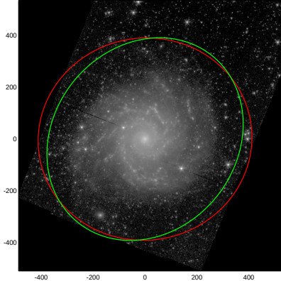
NGC0628
