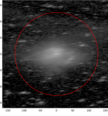
LEDA: pa,inc= 3.5 74.0
