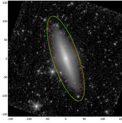
NGC0955
