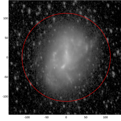
LEDA: pa,inc= 999.0 49.7
