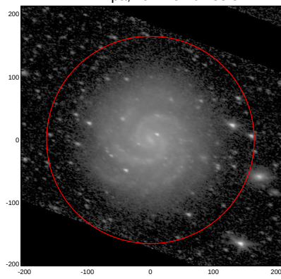
LEDA: pa,inc= 157.0 55.9
