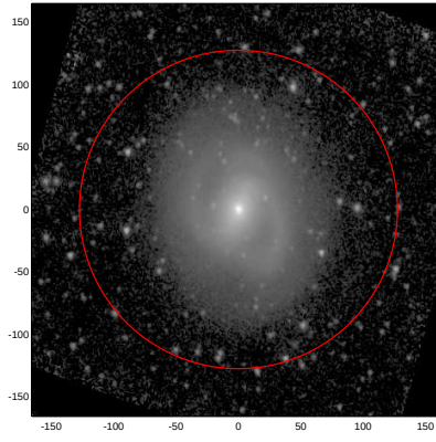
LEDA: pa,inc= 999.0 26.4
