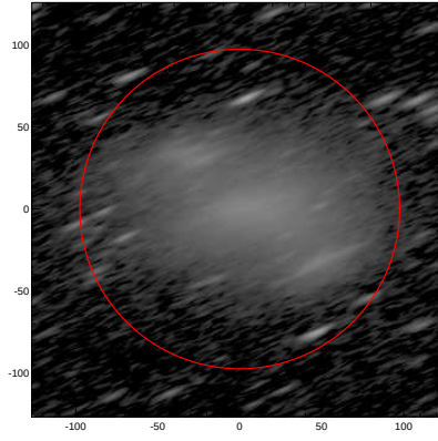
LEDA: pa,inc= 23.2 77.6
