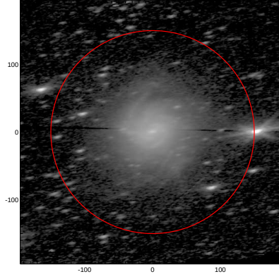
LEDA: pa,inc= 10.2 69.8
