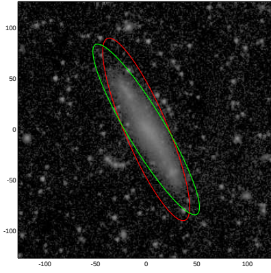
NGC0007
