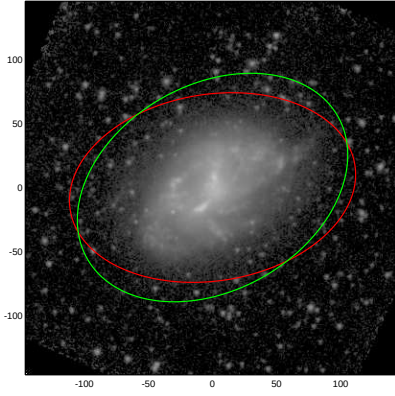
NGC0337
