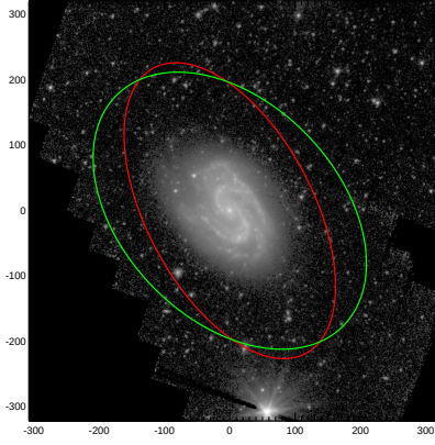
NGC0157
