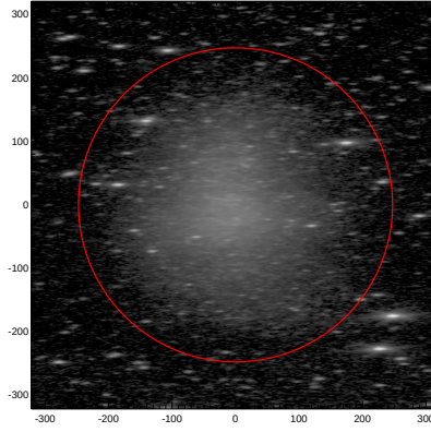
LEDA: pa,inc= 1.0 75.2
