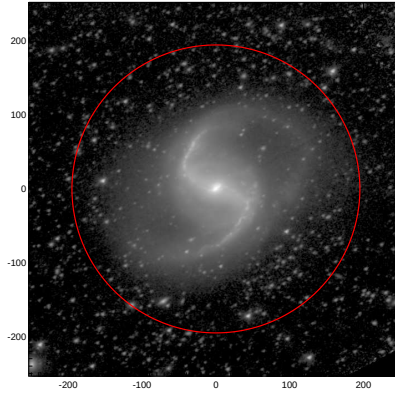
LEDA: pa,inc= 28.1 36.4
