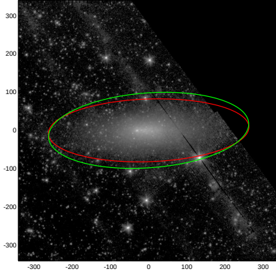
NGC0625
