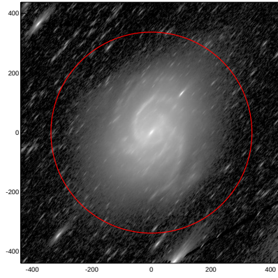
LEDA: pa,inc= 49.9 77.7
