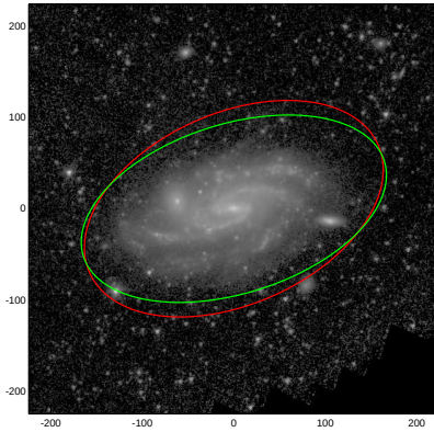
NGC0578
