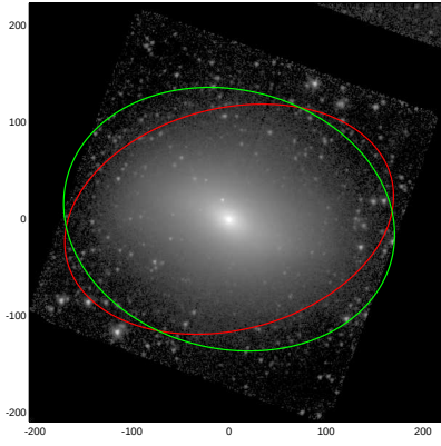
NGC0584
