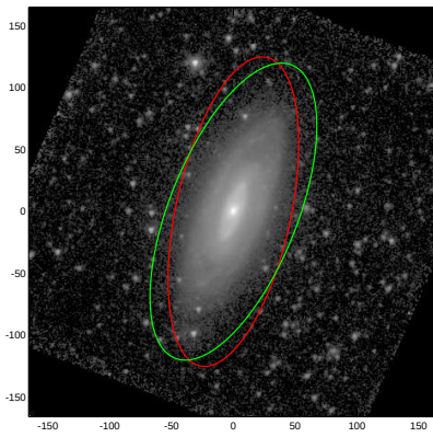
NGC0615
