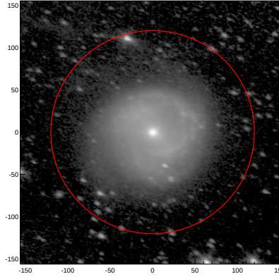
LEDA: pa,inc= 155.6 55.5
