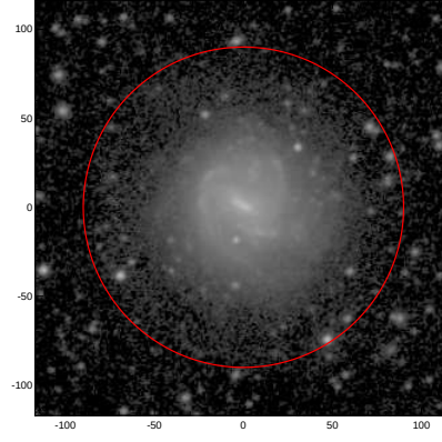
LEDA: pa,inc= 6.5 25.4
