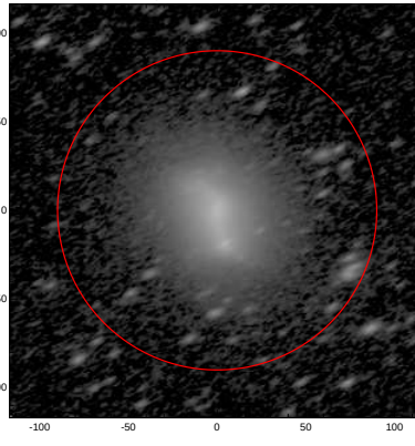
LEDA: pa,inc= 27.0 62.3
