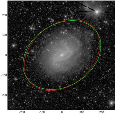
NGC1187
