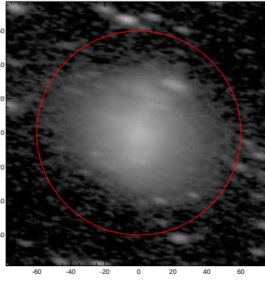
LEDA: pa,inc= 167.1 67.5
