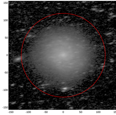
LEDA: pa,inc= 8.6 65.8
