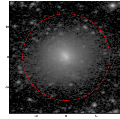
LEDA: pa,inc= 2.5 45.7
