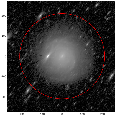
LEDA: pa,inc= 53.5 69.6
