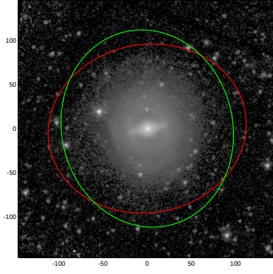
NGC1015
