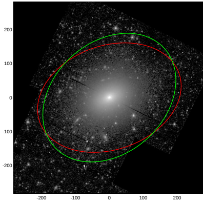
NGC1052
