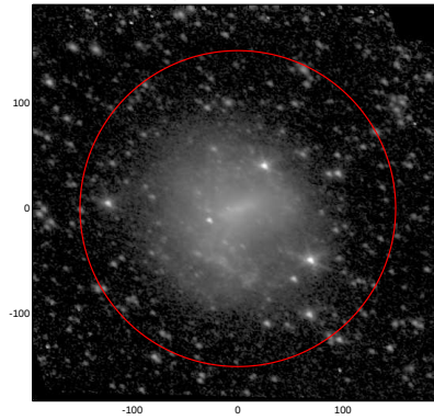
LEDA: pa,inc= 151.3 43.4
