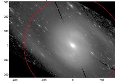
LEDA: pa,inc= 136.0 70.2
