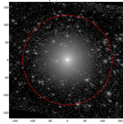
LEDA: pa,inc= 172.1 43.0
