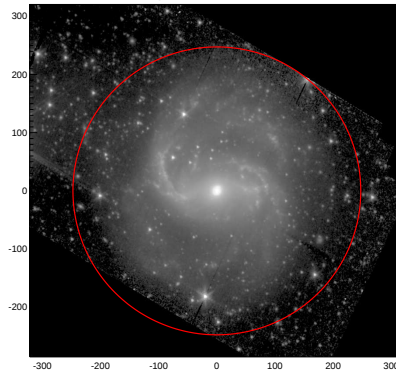
LEDA: pa,inc= 999.0 27.2
