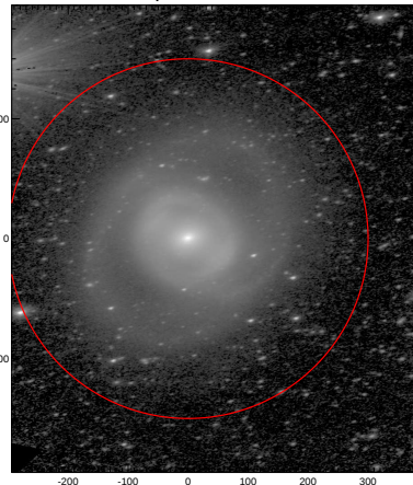
LEDA: pa,inc= 10.7 59.8
