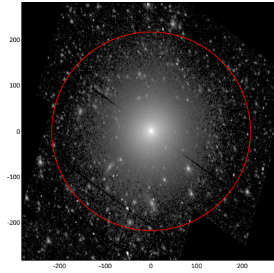
LEDA: pa,inc= 109.0 45.2
