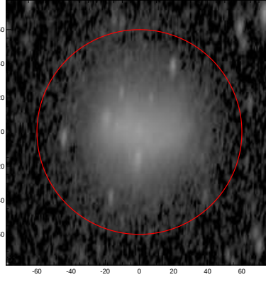
LEDA: pa,inc= 85.2 68.9
