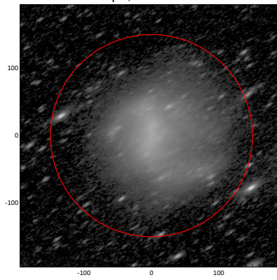
LEDA: pa,inc= 31.9 67.9
