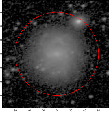
LEDA: pa,inc= 20.5 42.7
