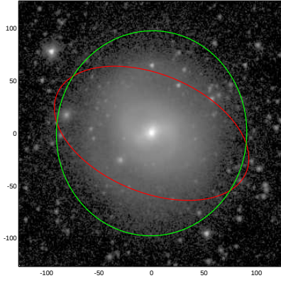
NGC1022
