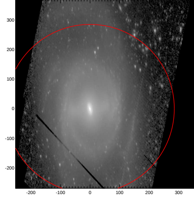
LEDA: pa,inc= 95.1 61.4
