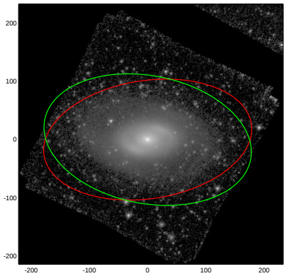
NGC1079
