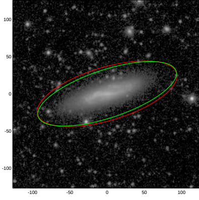
NGC1519
