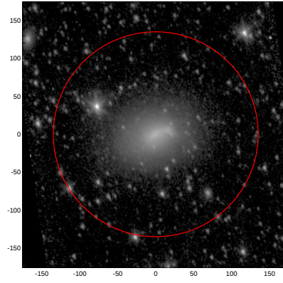
LEDA: pa,inc= 111.7 41.6
