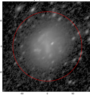
LEDA: pa,inc= 44.7 57.5
