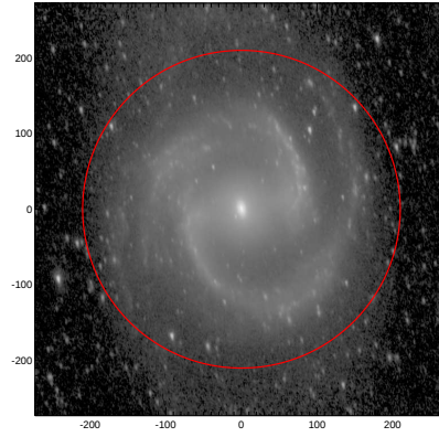
LEDA: pa,inc= 101.3 59.1
