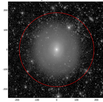
LEDA: pa,inc= 999.0 23.9
