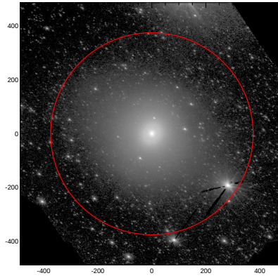
LEDA: pa,inc= 150.1 46.7
