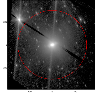
LEDA: pa,inc= 107.3 54.5
