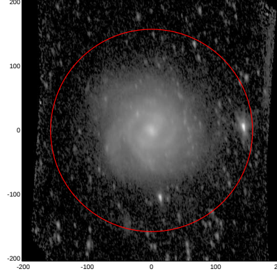
LEDA: pa,inc= 101.0 63.9
