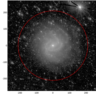
LEDA: pa,inc= 129.1 43.2
