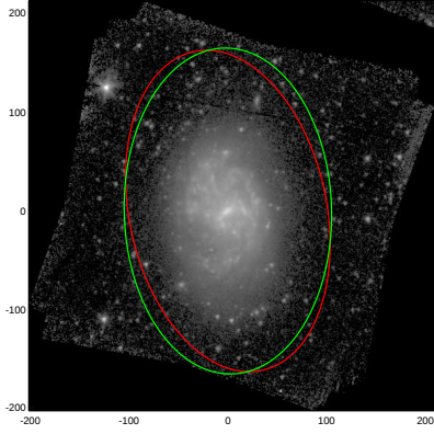
NGC1087
