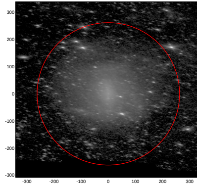
LEDA: pa,inc= 168.9 67.9
