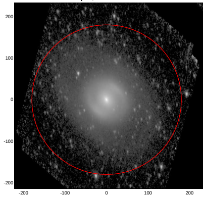
LEDA: pa,inc= 98.6 55.7
