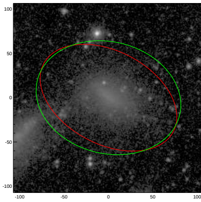
NGC1326A
