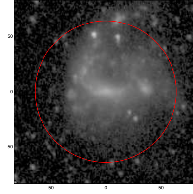
LEDA: pa,inc= 109.3 33.7
