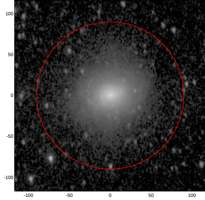
LEDA: pa,inc= 99.0 46.2
