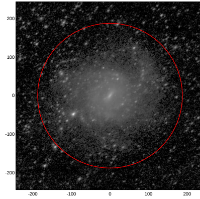
LEDA: pa,inc= 38.1 47.0
