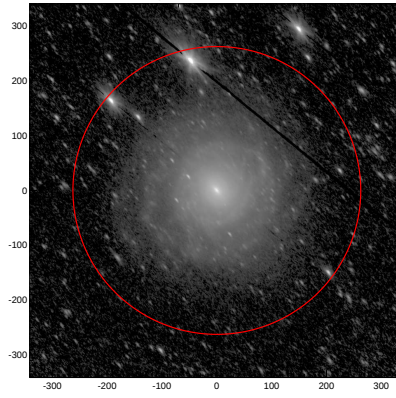
LEDA: pa,inc= 130.4 64.0
