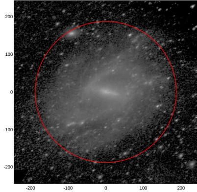
LEDA: pa,inc= 31.6 50.9
