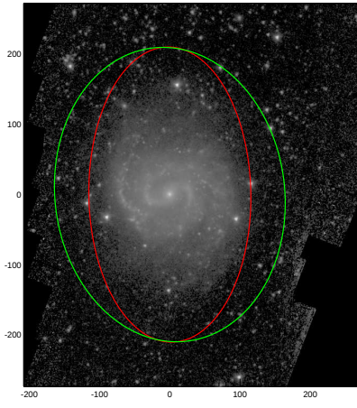
NGC1042
