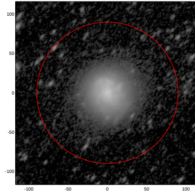
LEDA: pa,inc= 48.8 56.4
