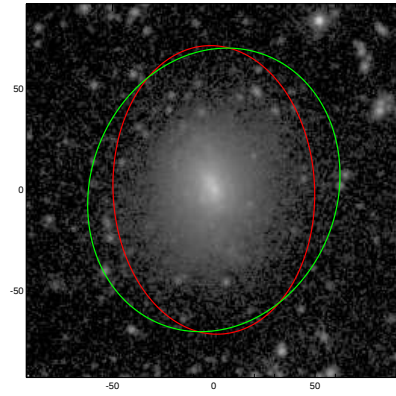
NGC1036
