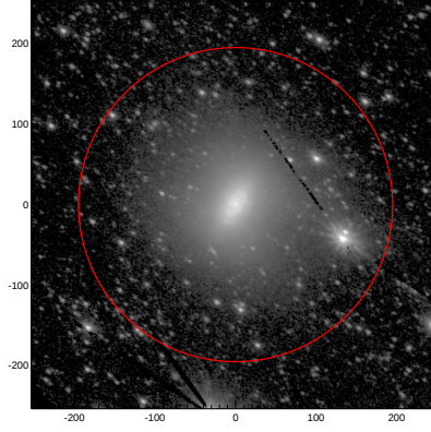
LEDA: pa,inc= 142.9 47.8
