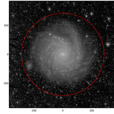
LEDA: pa,inc= 100.8 31.9
