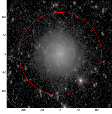
LEDA: pa,inc= 97.6 41.7
