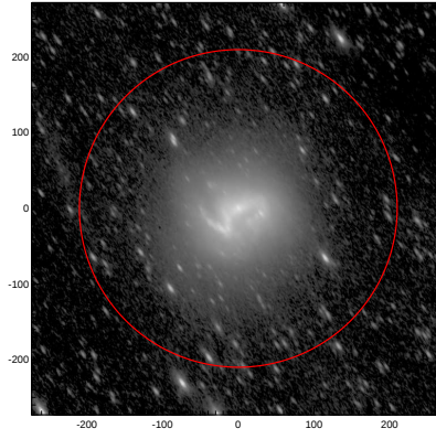
LEDA: pa,inc= 123.5 66.3
