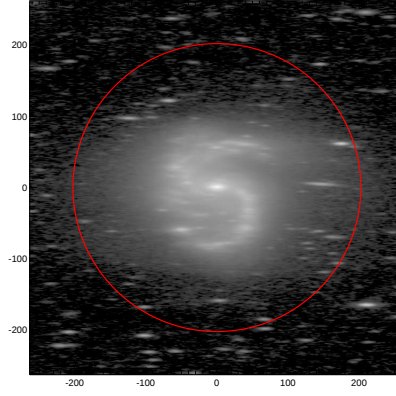
LEDA: pa,inc= 179.6 77.7
