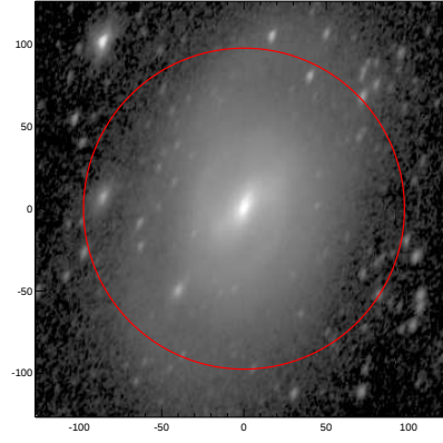
LEDA: pa,inc= 67.6 54.9
