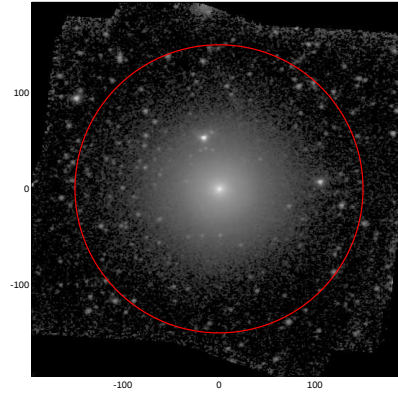
LEDA: pa,inc= 5.5 33.1
