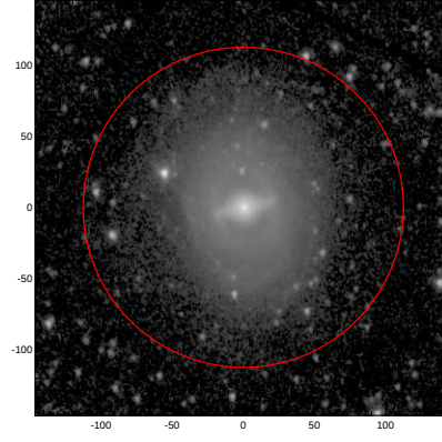
LEDA: pa,inc= 999.0 32.1
