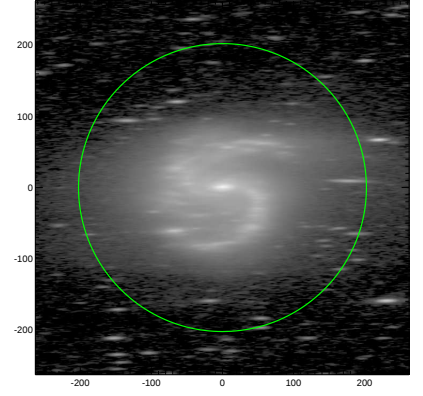
S4G: pa,inc= 1.4 79.8
