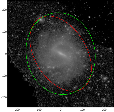
NGC1073
