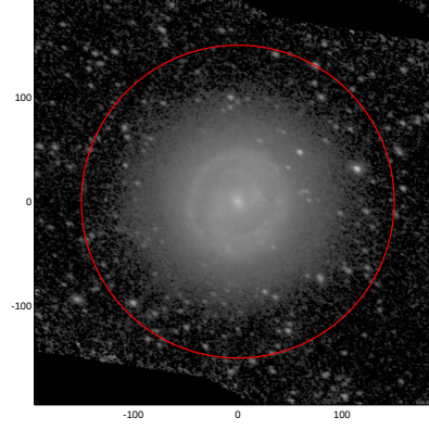
LEDA: pa,inc= 152.2 45.5
