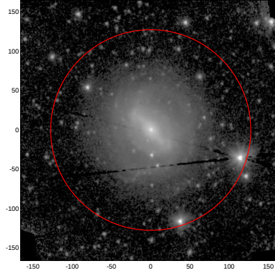
LEDA: pa,inc= 999.0 16.8
