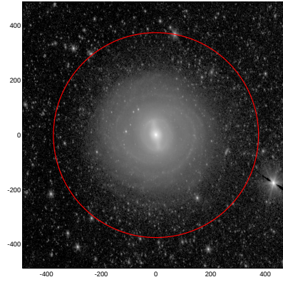
LEDA: pa,inc= 100.3 45.1
