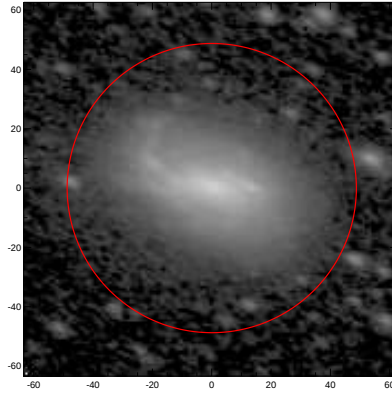
LEDA: pa,inc= 158.6 54.6
