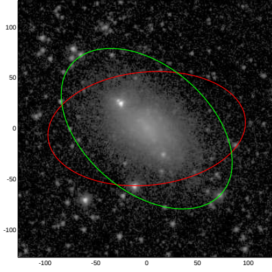
NGC1051
