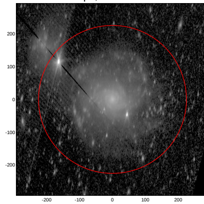
LEDA: pa,inc= 84.8 66.0
