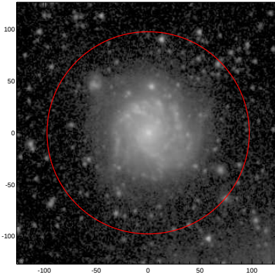
LEDA: pa,inc= 999.0 20.4
