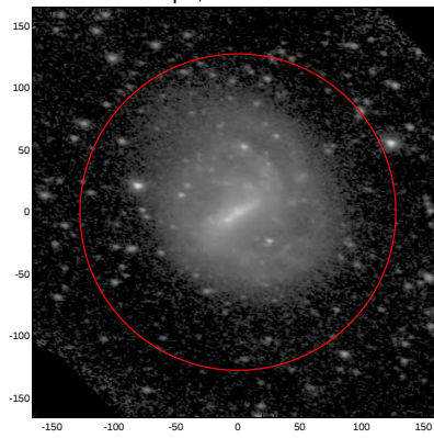
LEDA: pa,inc= 165.5 47.2
