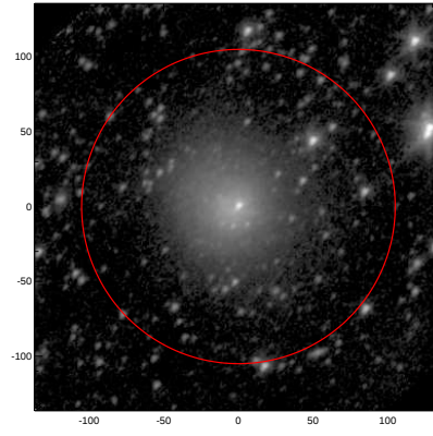
LEDA: pa,inc= 53.1 39.7
