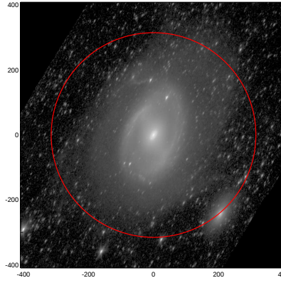
LEDA: pa,inc= 63.1 61.5
