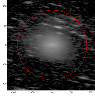
LEDA: pa,inc= 169.9 77.7
