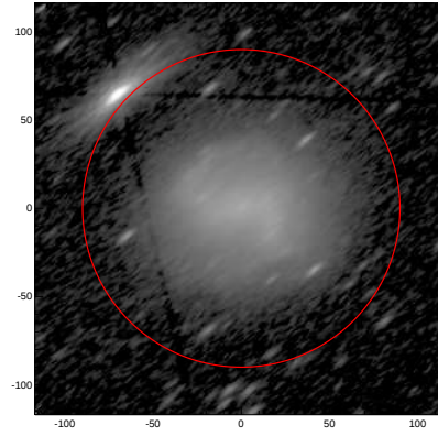
LEDA: pa,inc= 38.8 70.2
