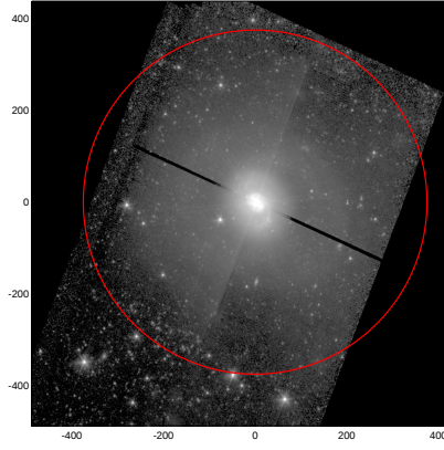
LEDA: pa,inc= 999.0 23.3
