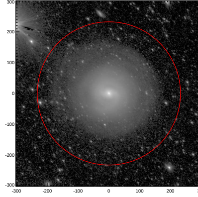
LEDA: pa,inc= 134.5 48.1
