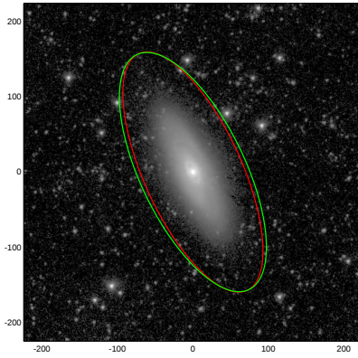
NGC1386
