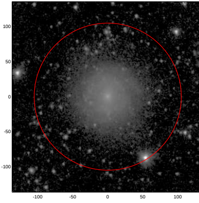
LEDA: pa,inc= 999.0 20.7
