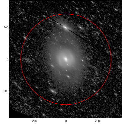
LEDA: pa,inc= 141.2 66.1
