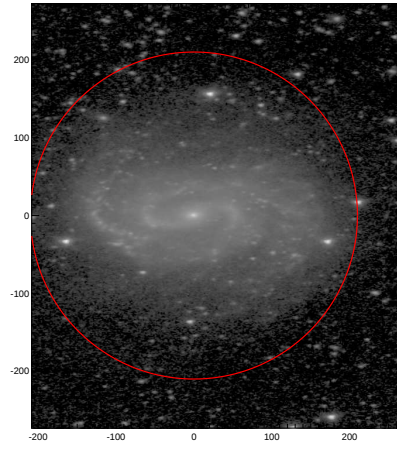
LEDA: pa,inc= 0.9 56.7
