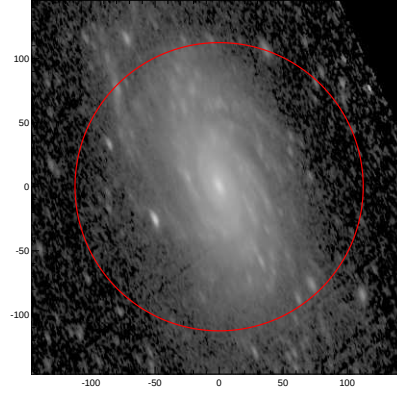
LEDA: pa,inc= 111.3 64.7
