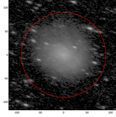
LEDA: pa,inc= 162.4 64.6
