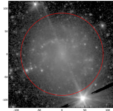
LEDA: pa,inc= 999.0 20.4
