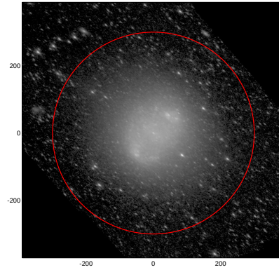
LEDA: pa,inc= 143.0 58.6
