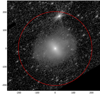
LEDA: pa,inc= 38.0 57.7
