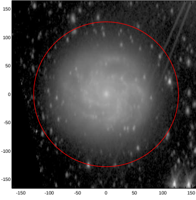
LEDA: pa,inc= 88.3 58.7
