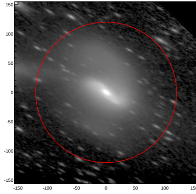
LEDA: pa,inc= 152.2 69.9
