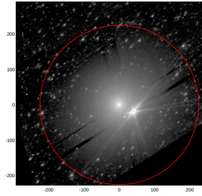
LEDA: pa,inc= 44.0 52.2
