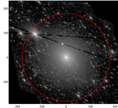
LEDA: pa,inc= 137.5 56.0
