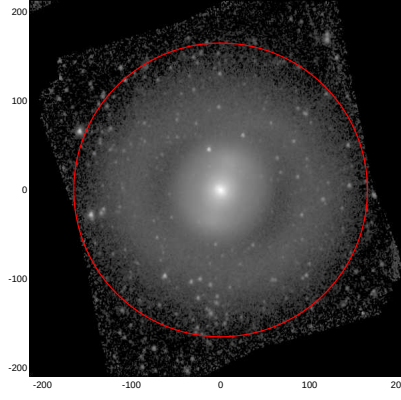
LEDA: pa,inc= 85.0 29.4
