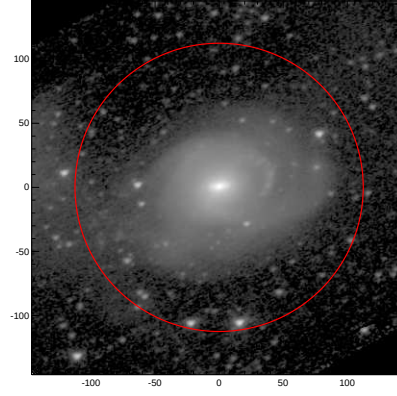
LEDA: pa,inc= 20.0 42.2
