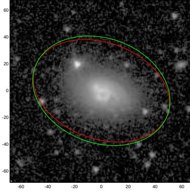
NGC2731
