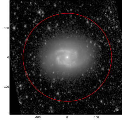
LEDA: pa,inc= 97.0 41.6
