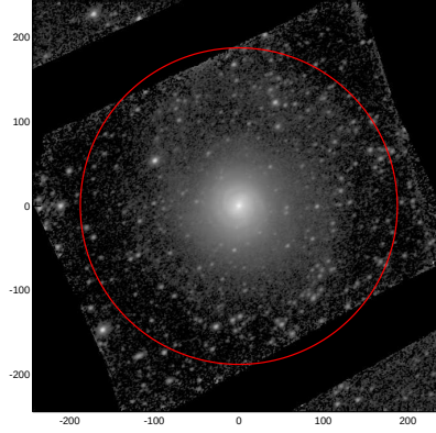
LEDA: pa,inc= 35.3 41.6
