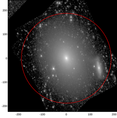
LEDA: pa,inc= 999.0 36.7
