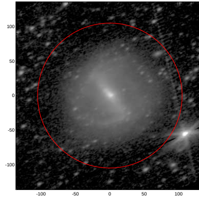
LEDA: pa,inc= 28.4 54.8
