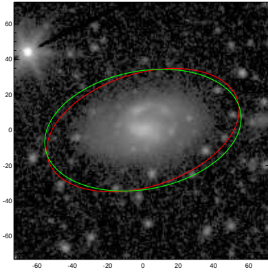
NGC3876
