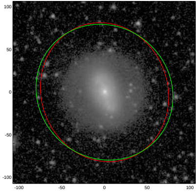
NGC3380
