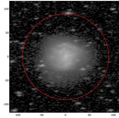
LEDA: pa,inc= 6.2 63.8
