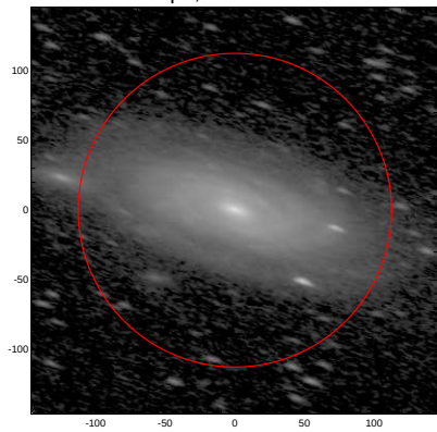
LEDA: pa,inc= 162.6 69.5
