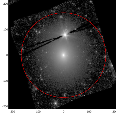
LEDA: pa,inc= 999.0 23.6
