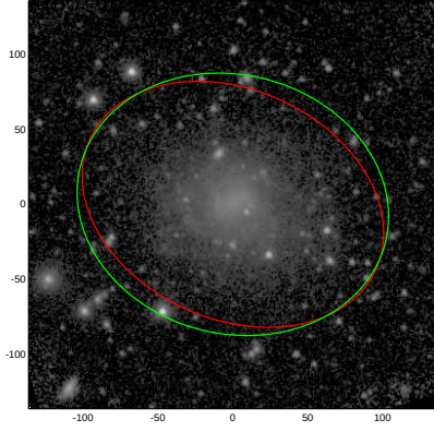
NGC3795A
