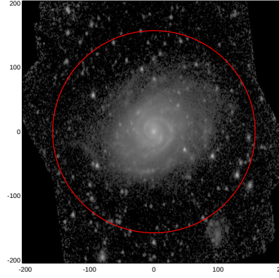
LEDA: pa,inc= 89.5 45.8
