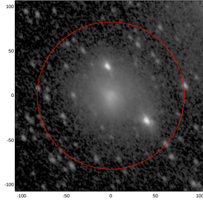
LEDA: pa,inc= 126.9 51.9
