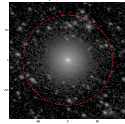
LEDA: pa,inc= 157.2 38.8
