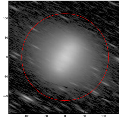
LEDA: pa,inc= 152.0 80.4
