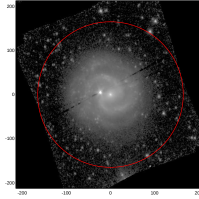
LEDA: pa,inc= 999.0 30.8
