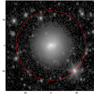
LEDA: pa,inc= 89.2 31.2
