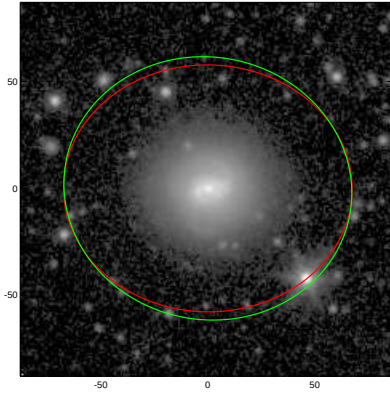
NGC3730
