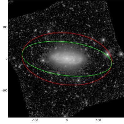
NGC3813
