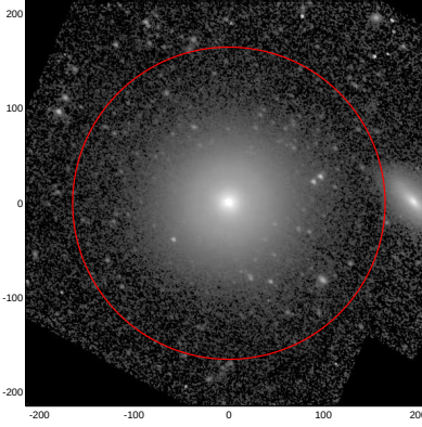
LEDA: pa,inc= 138.3 35.4
