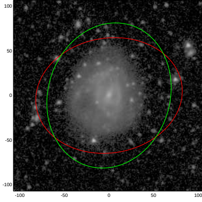
NGC3061
