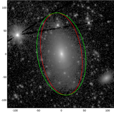
NGC3468
