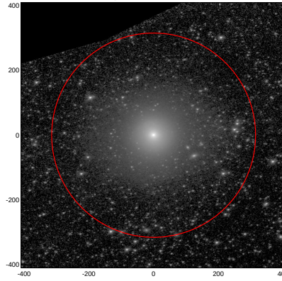
LEDA: pa,inc= 11.4 43.6
