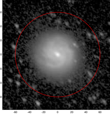
LEDA: pa,inc= 133.4 49.1
