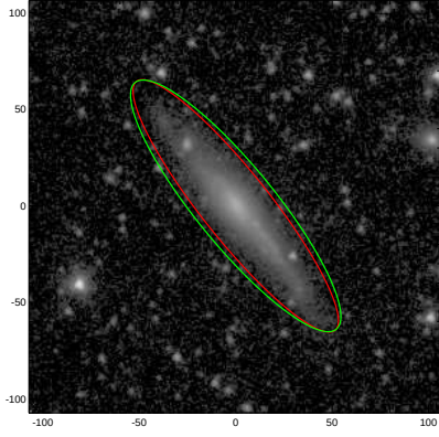
NGC3118
