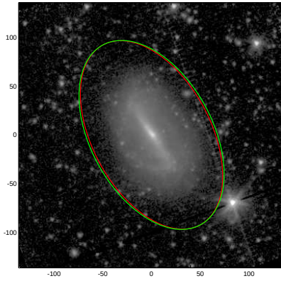
NGC3049
