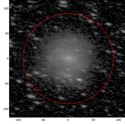
LEDA: pa,inc= 166.3 60.8
