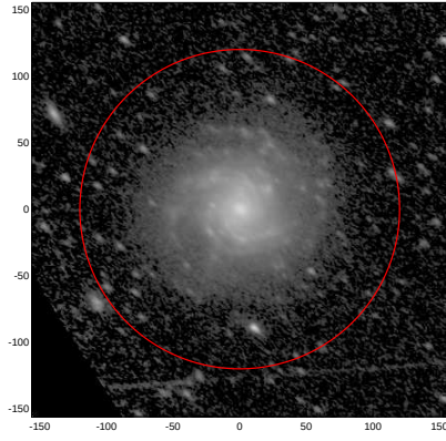
LEDA: pa,inc= 143.5 54.5
