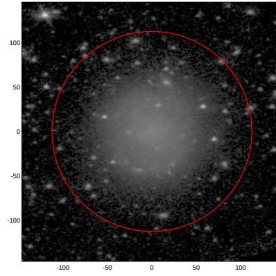
LEDA: pa,inc= 3.0 42.4
