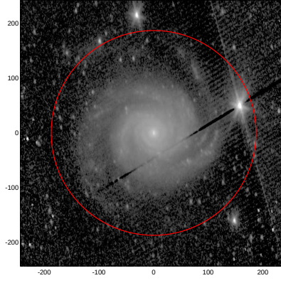
LEDA: pa,inc= 97.0 54.7
