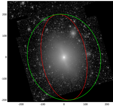
NGC3414
