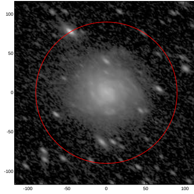
LEDA: pa,inc= 143.3 61.3
