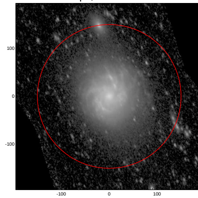
LEDA: pa,inc= 114.4 54.3
