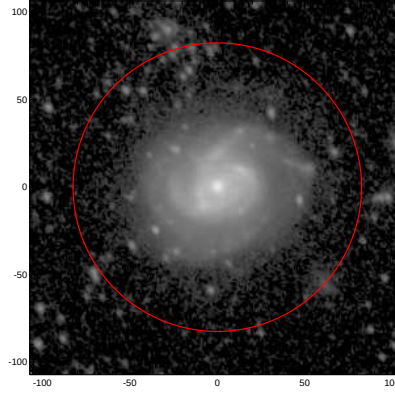
LEDA: pa,inc= 120.5 35.4
