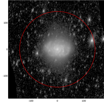
LEDA: pa,inc= 84.0 54.9
