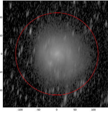
LEDA: pa,inc= 82.7 74.2
