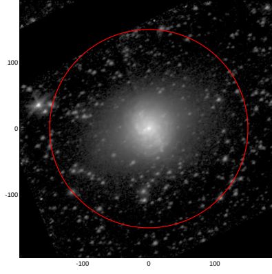
LEDA: pa,inc= 31.8 45.8
