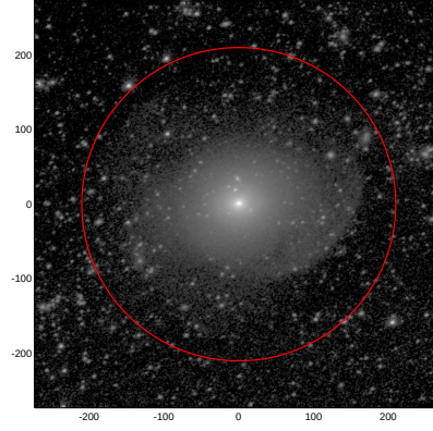
LEDA: pa,inc= 25.0 37.8
