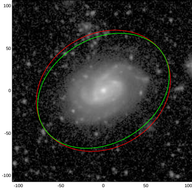
NGC3888
