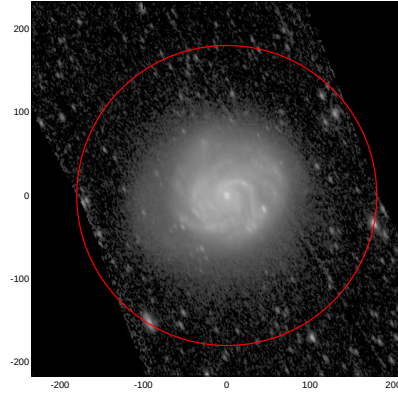
LEDA: pa,inc= 117.7 58.7
