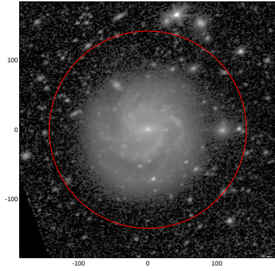
LEDA: pa,inc= 22.7 40.7
