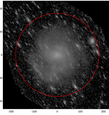
LEDA: pa,inc= 128.0 67.8
