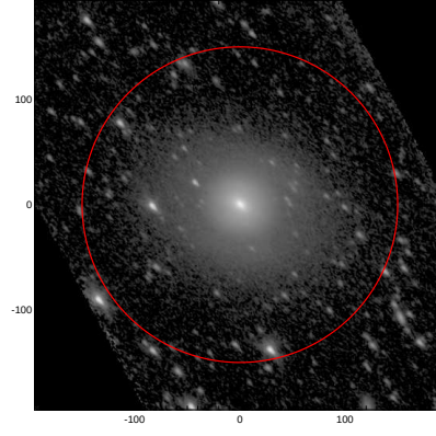
LEDA: pa,inc= 134.7 56.2
