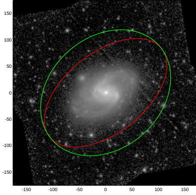
NGC3583
