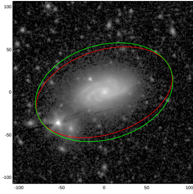
NGC3021
