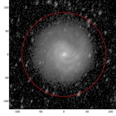
LEDA: pa,inc= 63.3 55.4
