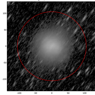
LEDA: pa,inc= 54.5 74.8
