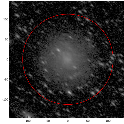
LEDA: pa,inc= 143.0 59.8
