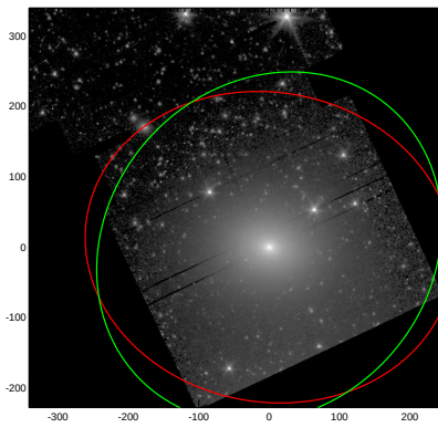
NGC3608
