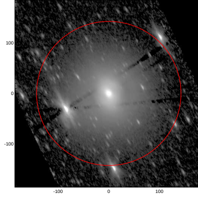
LEDA: pa,inc= 119.7 66.1
