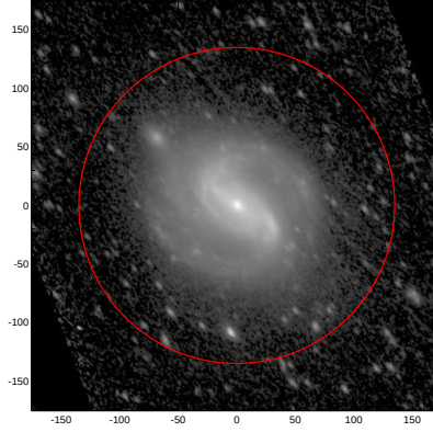
LEDA: pa,inc= 128.3 55.7
