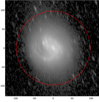
LEDA: pa,inc= 104.3 71.3
