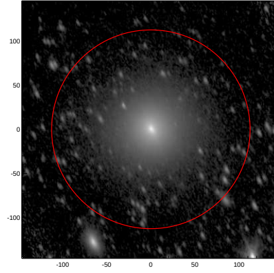
LEDA: pa,inc= 114.1 58.2
