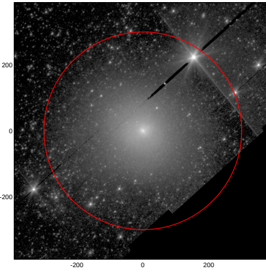
LEDA: pa,inc= 49.8 34.1
