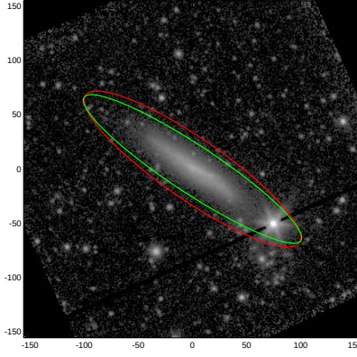
NGC3526
