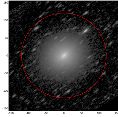
LEDA: pa,inc= 39.3 70.0
