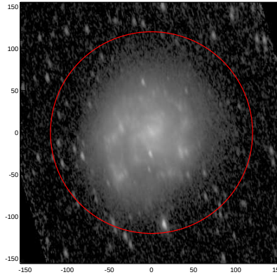
LEDA: pa,inc= 102.9 63.8
