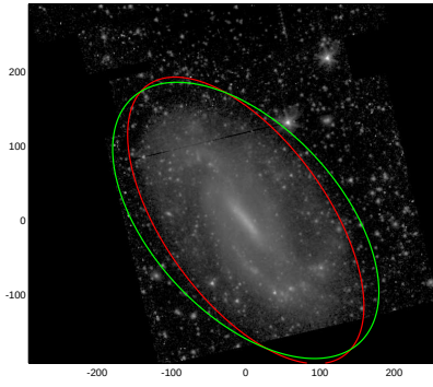
NGC3319
