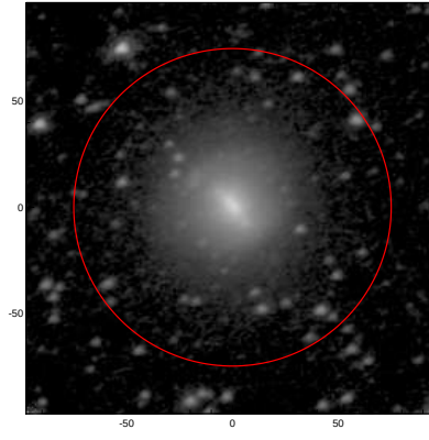
LEDA: pa,inc= 22.3 42.9
