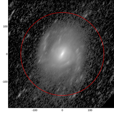
LEDA: pa,inc= 57.8 73.3
