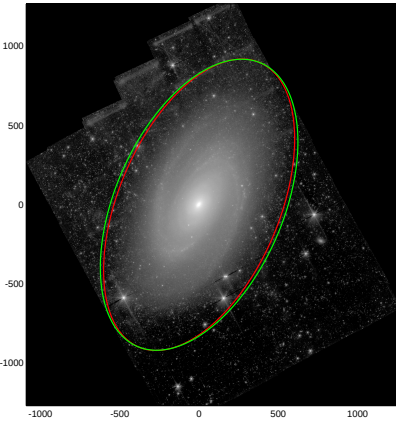
NGC3031
