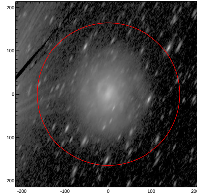
LEDA: pa,inc= 64.1 73.2
