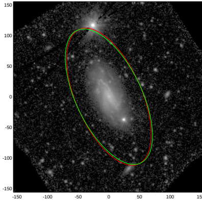
NGC3320
