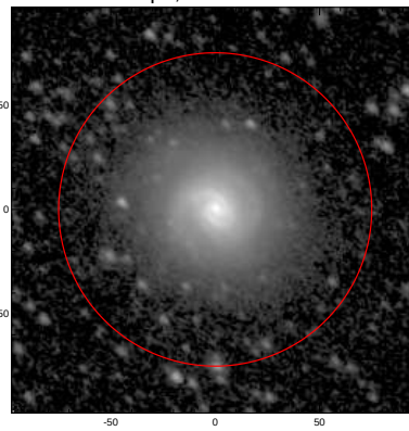
LEDA: pa,inc= 140.8 40.0
