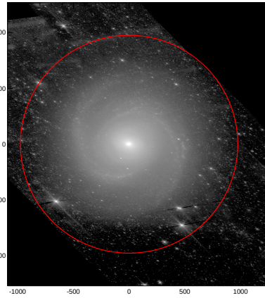
LEDA: pa,inc= 157.0 58.7
