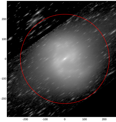
LEDA: pa,inc= 35.8 76.7
