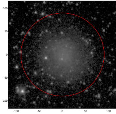
LEDA: pa,inc= 999.0 16.4
