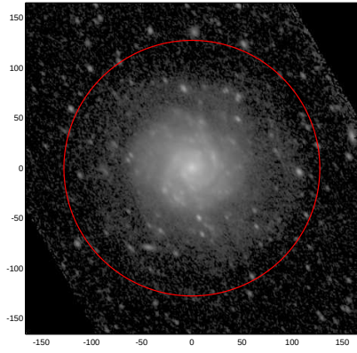
LEDA: pa,inc= 126.2 49.0
