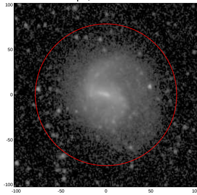
LEDA: pa,inc= 999.0 25.4
