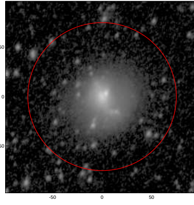
LEDA: pa,inc= 65.3 44.0
