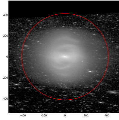
LEDA: pa,inc= 173.0 75.1
