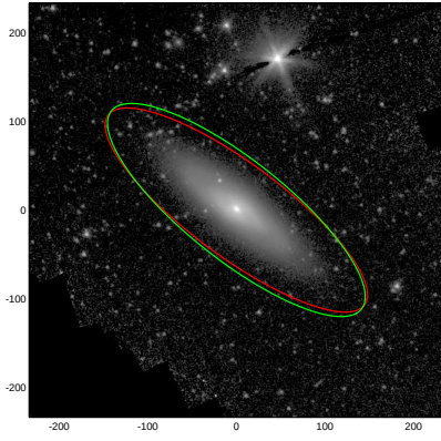
NGC3301
