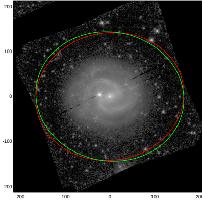
NGC3507
