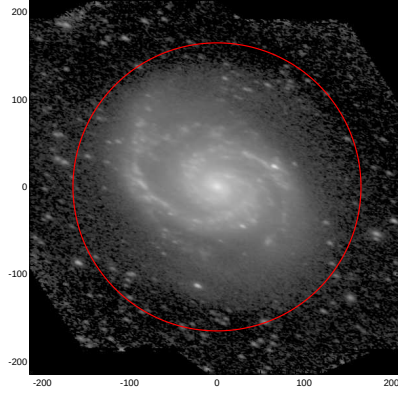
LEDA: pa,inc= 159.3 57.9
