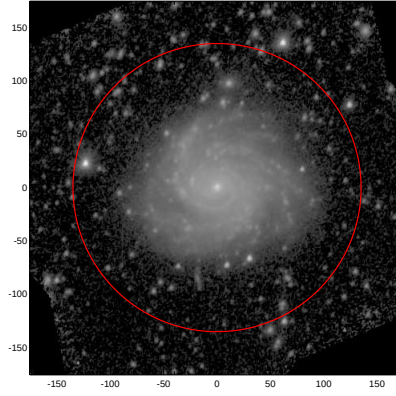
LEDA: pa,inc= 68.2 34.5
