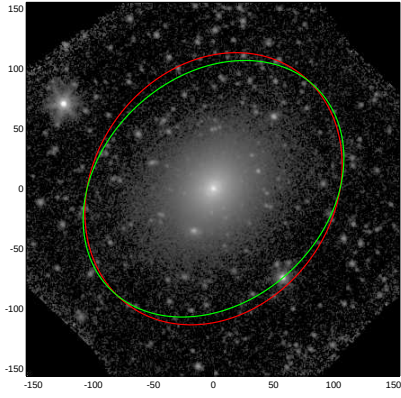
NGC3182
