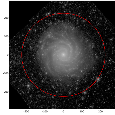
LEDA: pa,inc= 999.0 13.9
