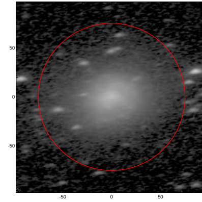
LEDA: pa,inc= 9.5 66.1
