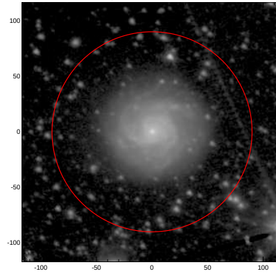
LEDA: pa,inc= 151.2 30.3
