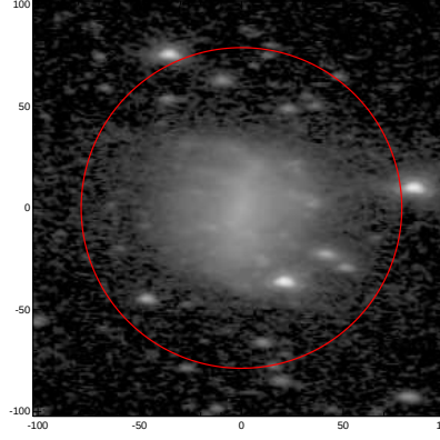
LEDA: pa,inc= 177.5 58.9
