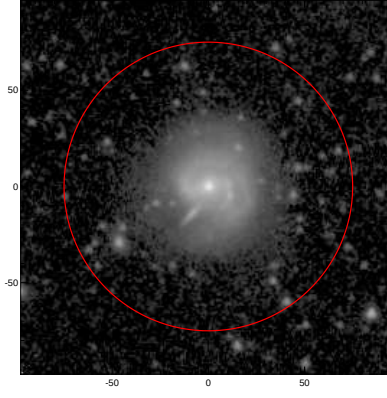
LEDA: pa,inc= 999.0 18.1
