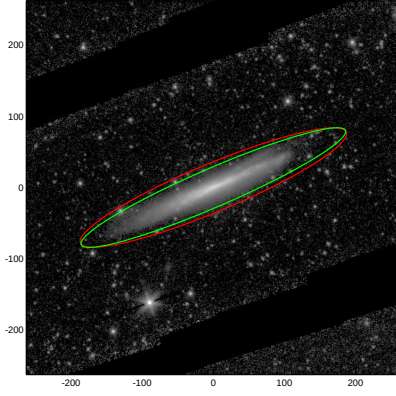
NGC3044
