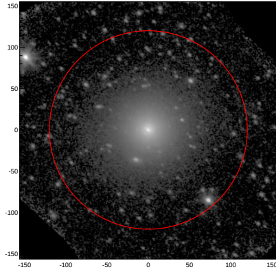
LEDA: pa,inc= 143.9 33.9
