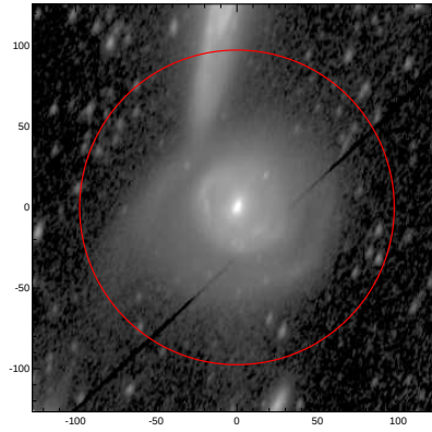
LEDA: pa,inc= 70.7 59.1
