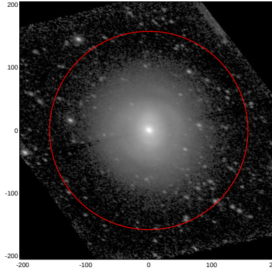
LEDA: pa,inc= 156.3 48.9
