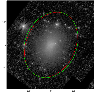
NGC3738
