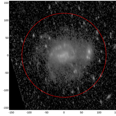
LEDA: pa,inc= 99.4 56.9
