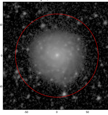
LEDA: pa,inc= 67.5 28.7
