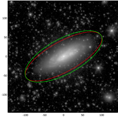
NGC3437
