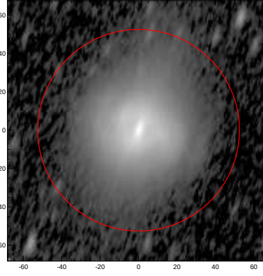
LEDA: pa,inc= 70.7 68.1
