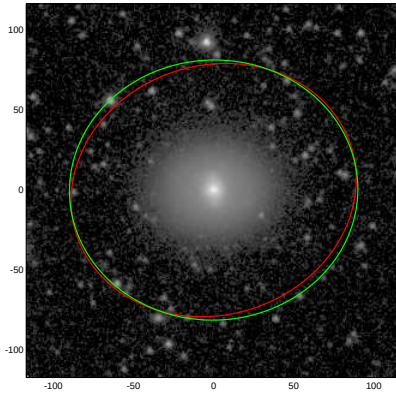
NGC3266
