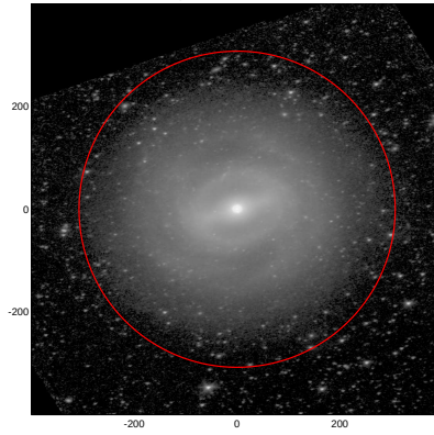
LEDA: pa,inc= 9.9 52.0
