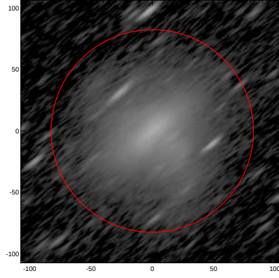
LEDA: pa,inc= 38.6 77.7
