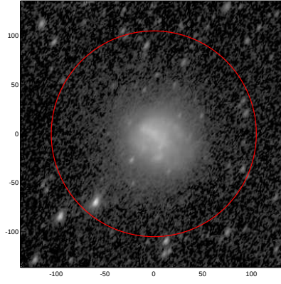
LEDA: pa,inc= 59.2 57.9
