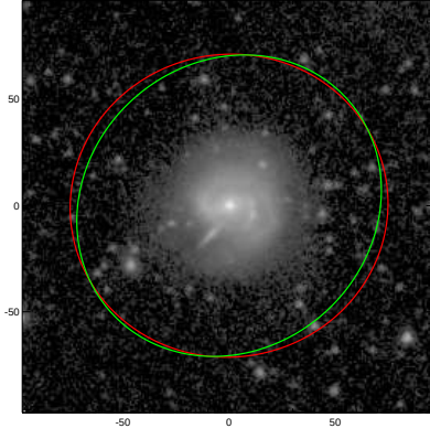
NGC3066
