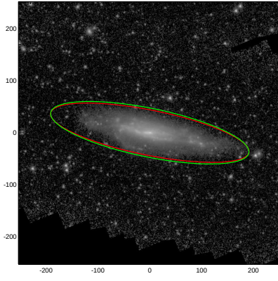
NGC3003
