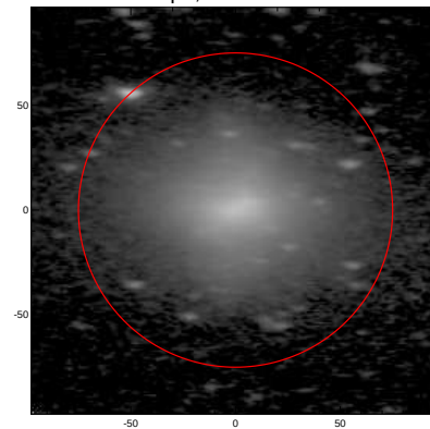
LEDA: pa,inc= 178.1 65.2
