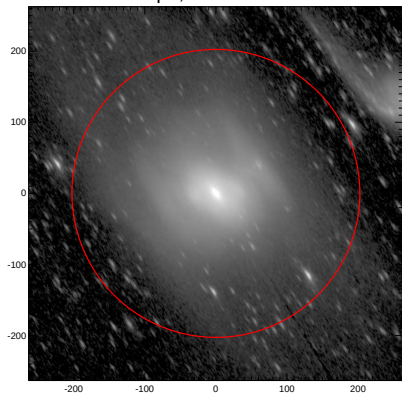
LEDA: pa,inc= 123.2 70.4
