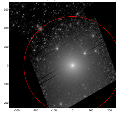
LEDA: pa,inc= 80.0 33.1
