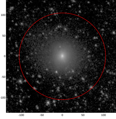
LEDA: pa,inc= 121.3 26.7
