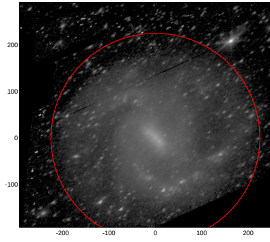
LEDA: pa,inc= 36.0 60.9
