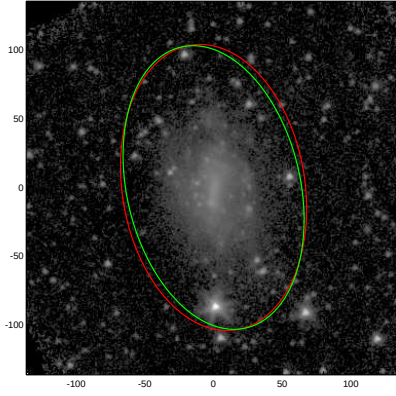
NGC3057
