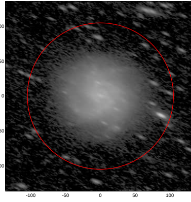
LEDA: pa,inc= 155.0 69.7
