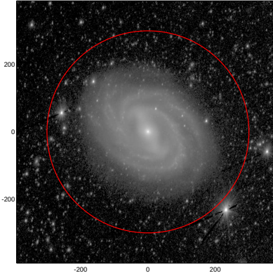
LEDA: pa,inc= 77.5 45.7
