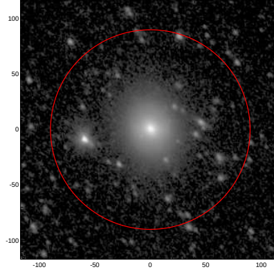
LEDA: pa,inc= 125.0 38.9
