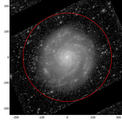
LEDA: pa,inc= 31.5 47.0
