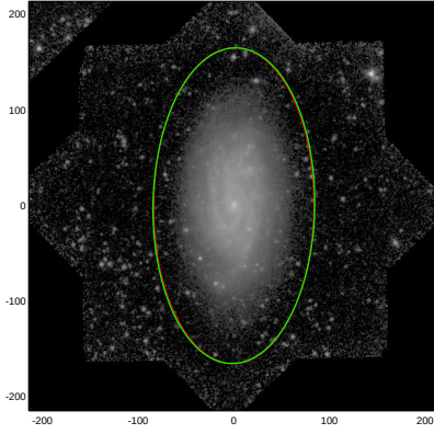
NGC3756
