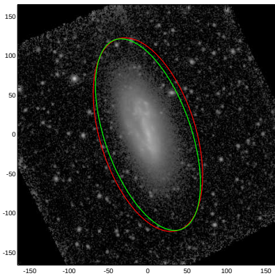
NGC3287
