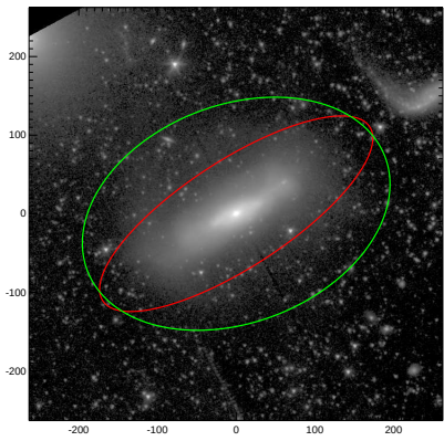
NGC3190
