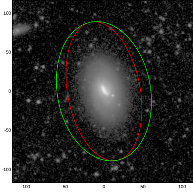
NGC3471
