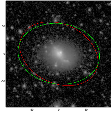
NGC3353
