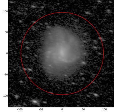
LEDA: pa,inc= 164.4 59.0
