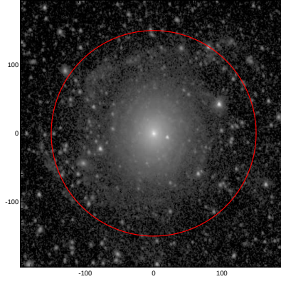
LEDA: pa,inc= 999.0 31.2
