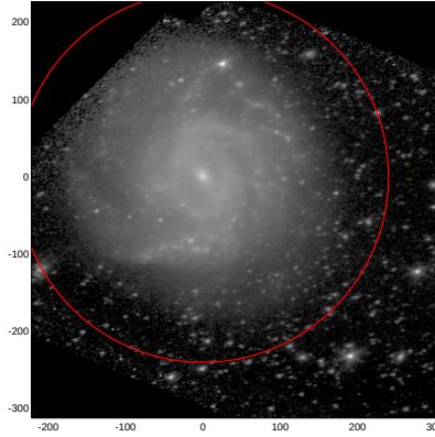
LEDA: pa,inc= 13.5 47.8
