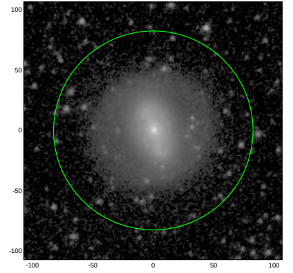
S4G: pa,inc= 47.4 20.8
