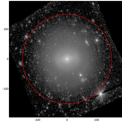
LEDA: pa,inc= 98.2 28.7
