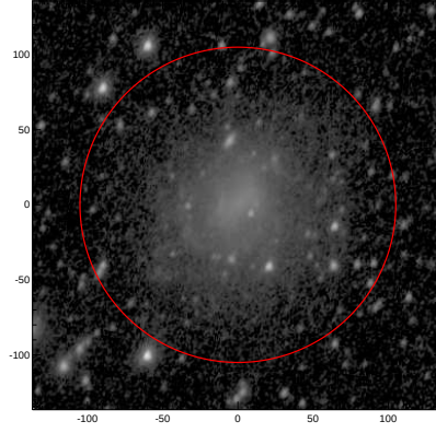
LEDA: pa,inc= 65.7 43.2
