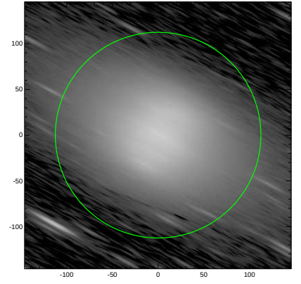
S4G: pa,inc= 151.9 84.1
