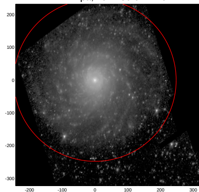
LEDA: pa,inc= 80.0 44.9
