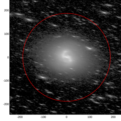
LEDA: pa,inc= 166.3 73.1
