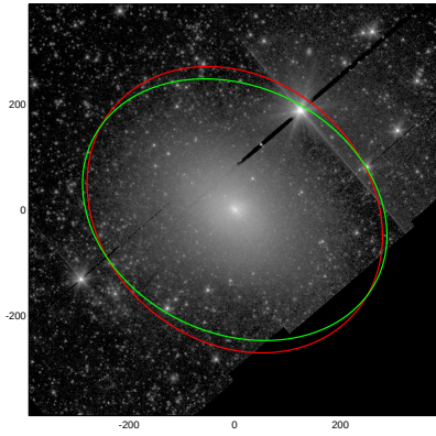
NGC3077
