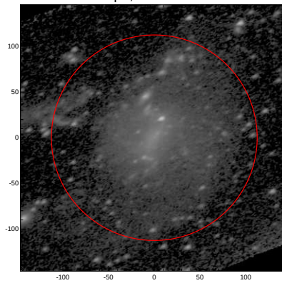
LEDA: pa,inc= 25.6 54.9
