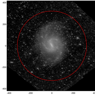
LEDA: pa,inc= 166.4 46.0
