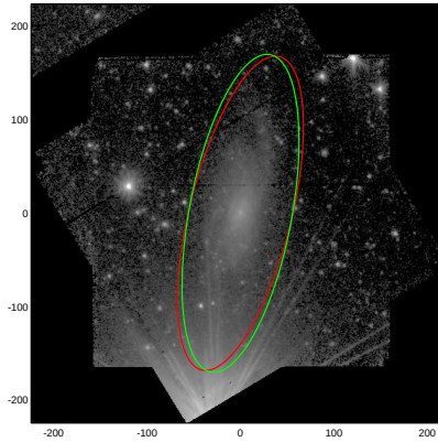
NGC3733
