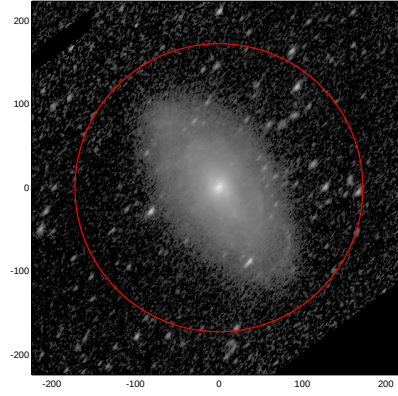
LEDA: pa,inc= 51.9 61.4
