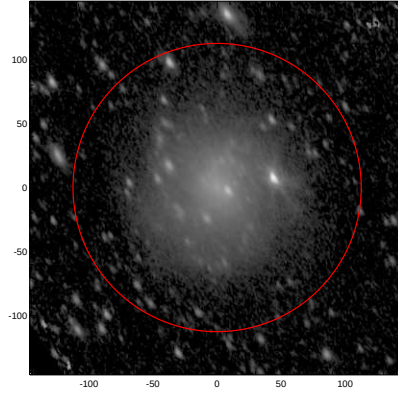
LEDA: pa,inc= 116.0 56.5
