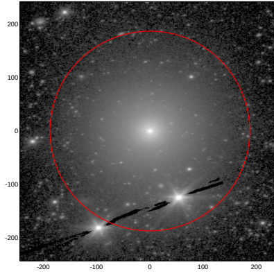
LEDA: pa,inc= 10.0 44.0
