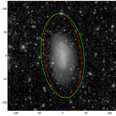
NGC3547
