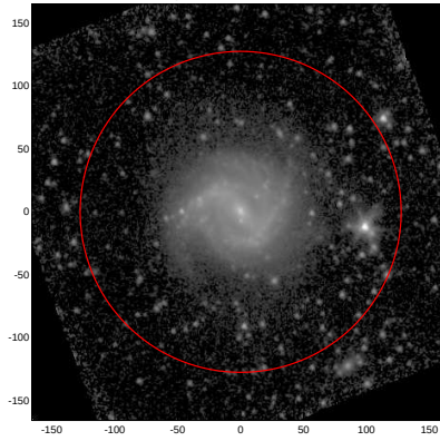
LEDA: pa,inc= 999.0 19.3
