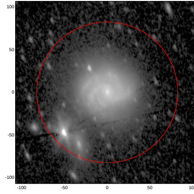
LEDA: pa,inc= 108.3 53.5
