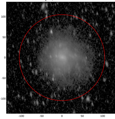
LEDA: pa,inc= 97.5 60.7
