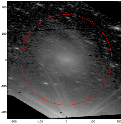
LEDA: pa,inc= 166.0 71.6
