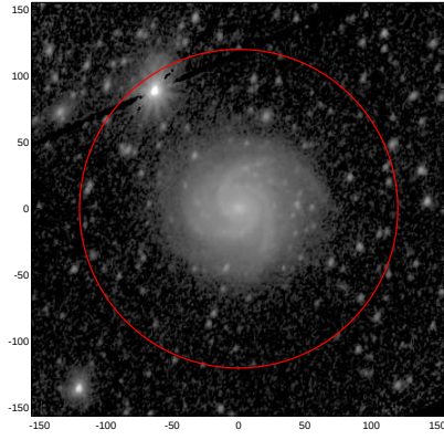
LEDA: pa,inc= 68.1 43.3
