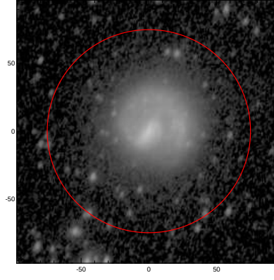
LEDA: pa,inc= 70.2 48.6
