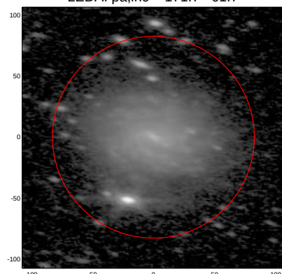
LEDA: pa,inc= 171.7 61.7
