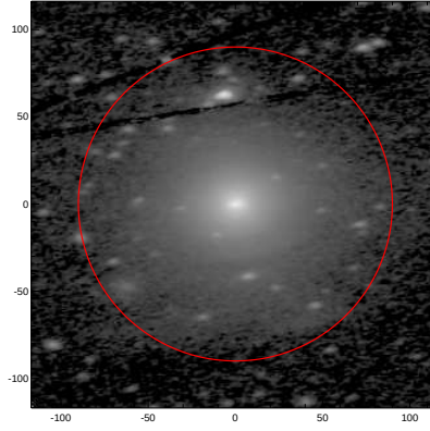
LEDA: pa,inc= 8.7 61.0
