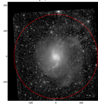
LEDA: pa,inc= 999.0 15.5
