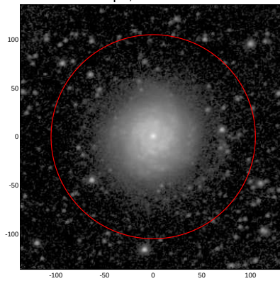
LEDA: pa,inc= 25.1 29.0
