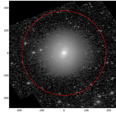
LEDA: pa,inc= 10.0 48.3
