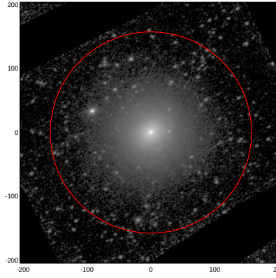
LEDA: pa,inc= 29.0 41.1
