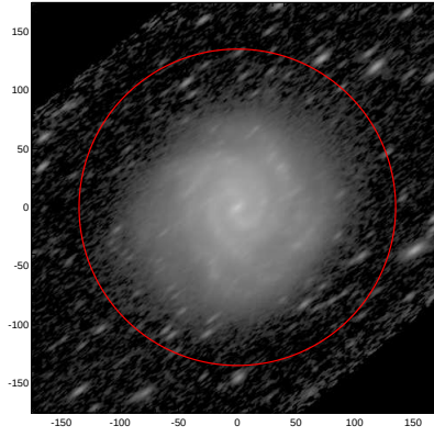
LEDA: pa,inc= 38.5 71.0
