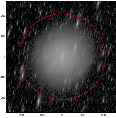
LEDA: pa,inc= 76.2 77.1
