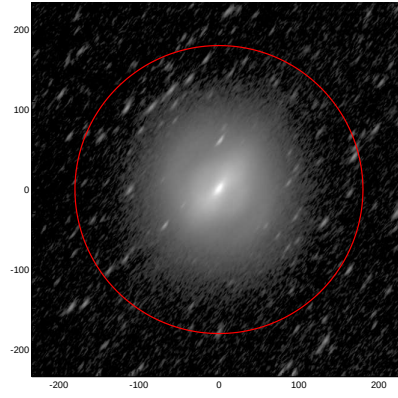
LEDA: pa,inc= 53.5 73.0
