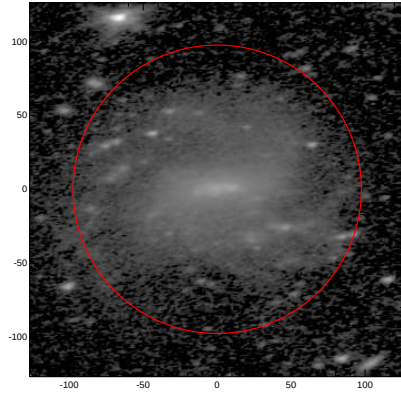
LEDA: pa,inc= 9.4 59.5
