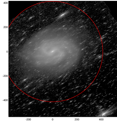
LEDA: pa,inc= 32.2 73.4
