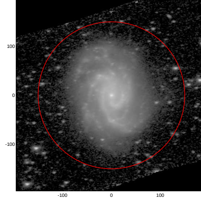
LEDA: pa,inc= 6.5 54.5
