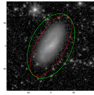
NGC3752
