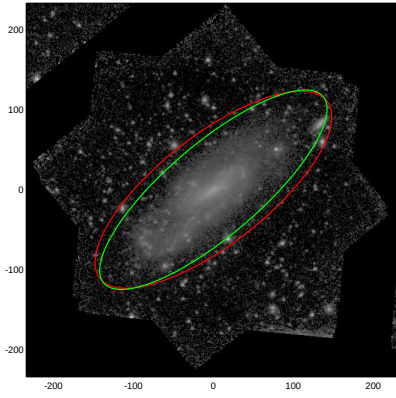
NGC3027
