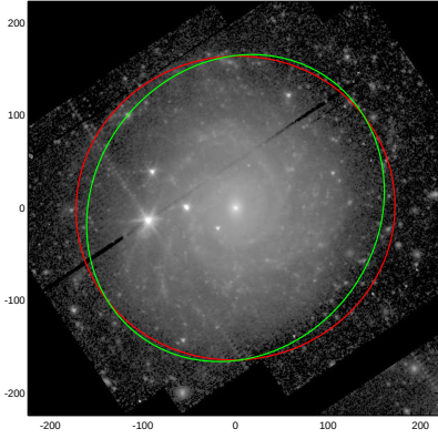
NGC3344
