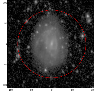
LEDA: pa,inc= 999.0 38.8
