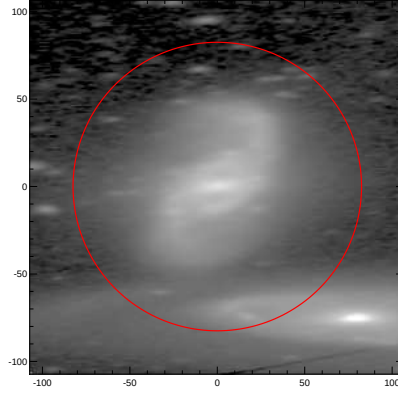
LEDA: pa,inc= 3.2 73.2
