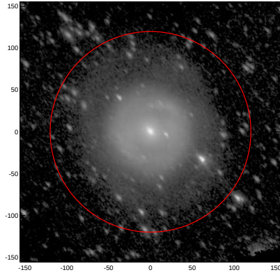
LEDA: pa,inc= 130.9 55.1
