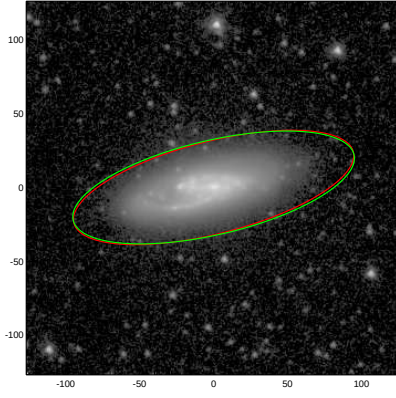
NGC3067
