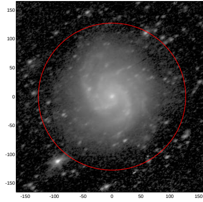
LEDA: pa,inc= 32.3 56.1
