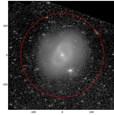
LEDA: pa,inc= 180.0 43.7
