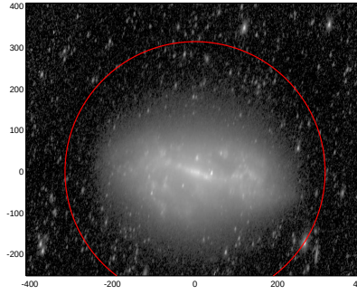
LEDA: pa,inc= 78.8 65.4
