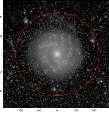
LEDA: pa,inc= 118.0 33.9
