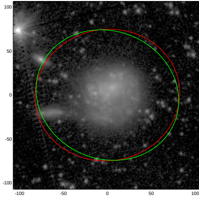
NGC3445
