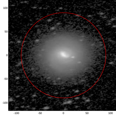
LEDA: pa,inc= 10.5 59.0
