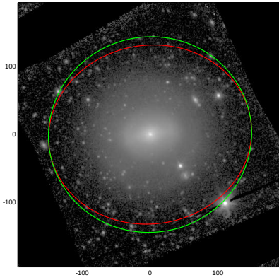
NGC3892
