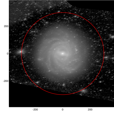
LEDA: pa,inc= 12.5 59.4
