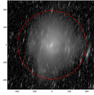
LEDA: pa,inc= 78.8 77.1
