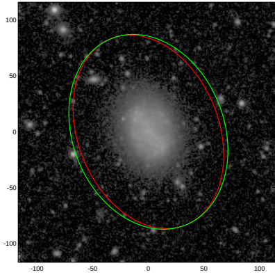
NGC3691
