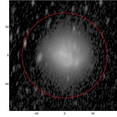
LEDA: pa,inc= 81.4 68.6
