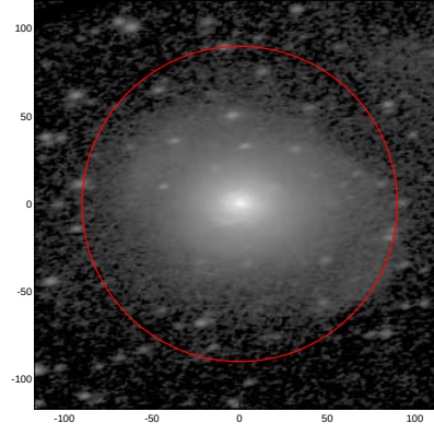
LEDA: pa,inc= 10.5 57.5
