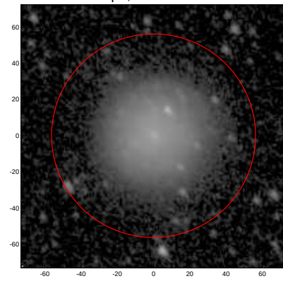
LEDA: pa,inc= 126.7 37.8
