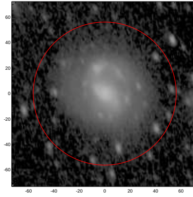
LEDA: pa,inc= 107.6 55.4
