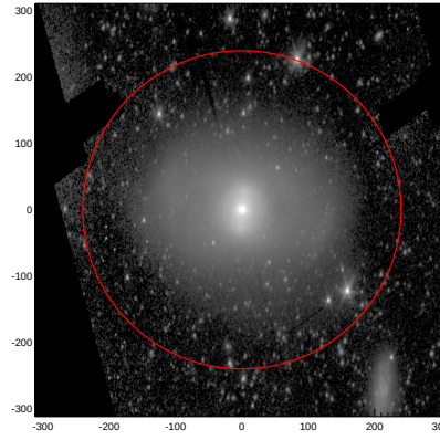
LEDA: pa,inc= 87.3 50.8
