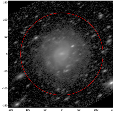
LEDA: pa,inc= 29.3 61.1
