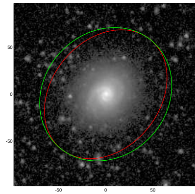
NGC3177
