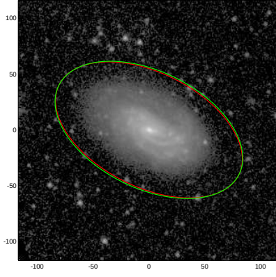
NGC3055
