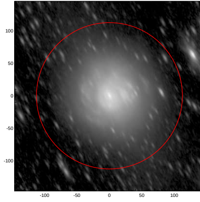
LEDA: pa,inc= 118.8 69.5
