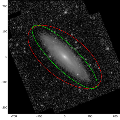
NGC3254
