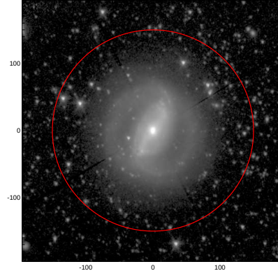
LEDA: pa,inc= 999.0 25.1
