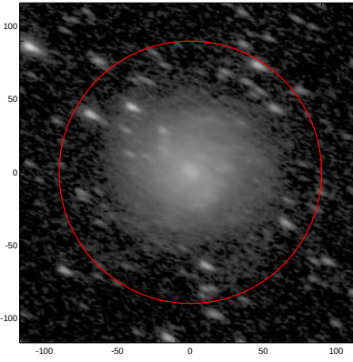
LEDA: pa,inc= 154.0 62.9
