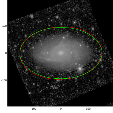
NGC3041
