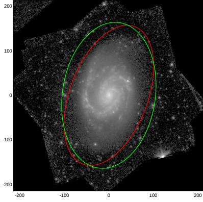
NGC3893
