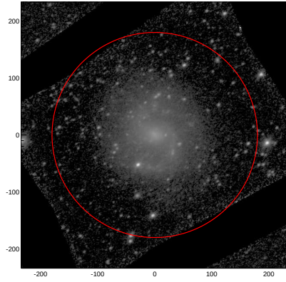
LEDA: pa,inc= 36.5 42.0
