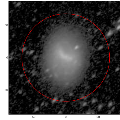
LEDA: pa,inc= 45.0 54.8
