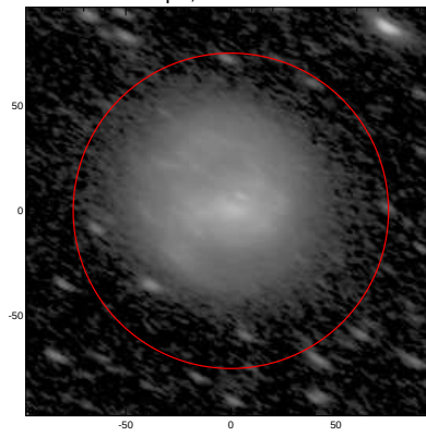
LEDA: pa,inc= 150.0 65.2
