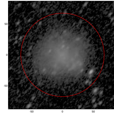
LEDA: pa,inc= 51.0 59.2
