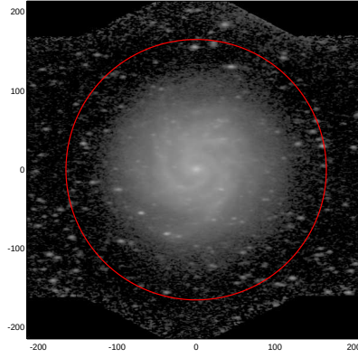
LEDA: pa,inc= 179.6 59.5
