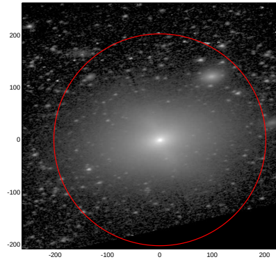
LEDA: pa,inc= 9.4 59.1
