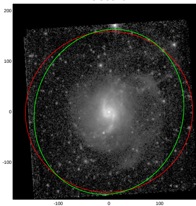
NGC3310
