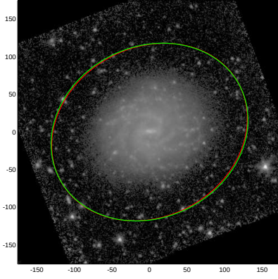
NGC3346
