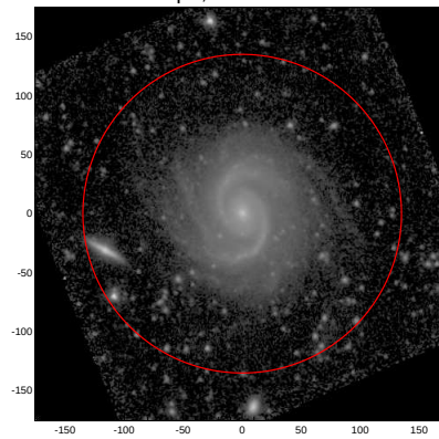
LEDA: pa,inc= 999.0 17.3
