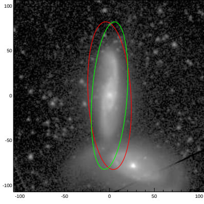
NGC3788
