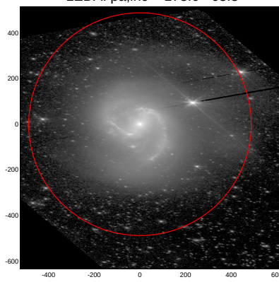
LEDA: pa,inc= 173.0 63.3
