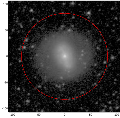
LEDA: pa,inc= 20.0 26.2
