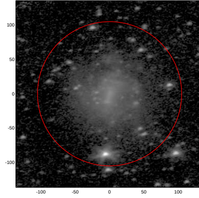
LEDA: pa,inc= 9.1 50.7
