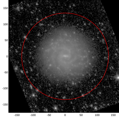
LEDA: pa,inc= 118.6 33.5
