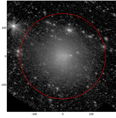
LEDA: pa,inc= 155.0 44.1
