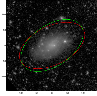
NGC3794
