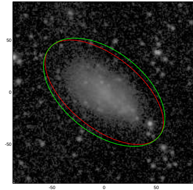
NGC3589
