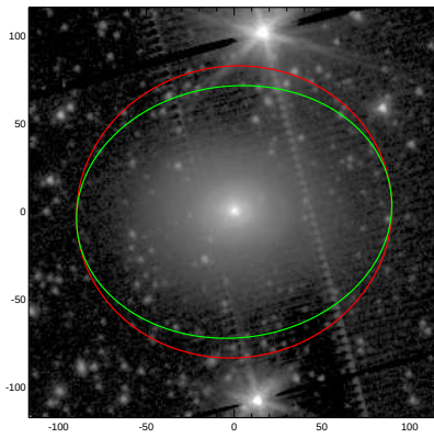
NGC3032
