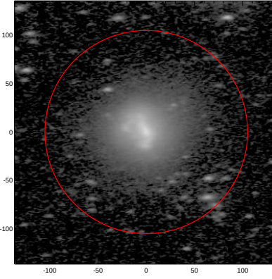
LEDA: pa,inc= 3.3 63.7
