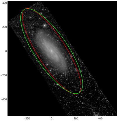
NGC3198
