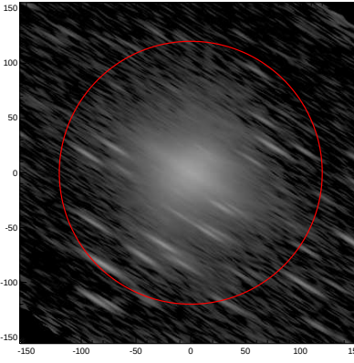
LEDA: pa,inc= 148.4 82.6
