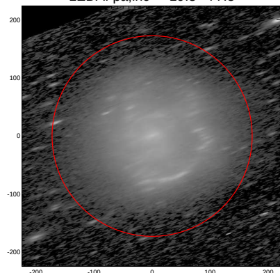
LEDA: pa,inc= 19.8 77.5
