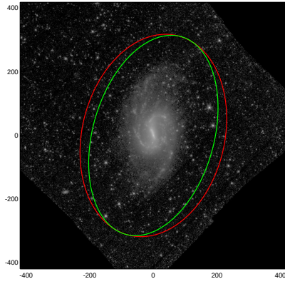
NGC3359
