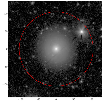
LEDA: pa,inc= 999.0 17.3
