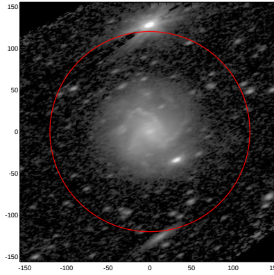
LEDA: pa,inc= 23.8 63.4
