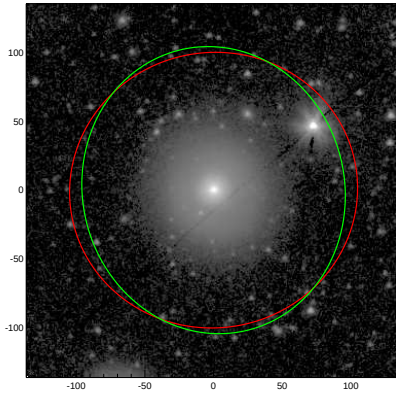
NGC3065
