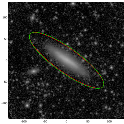
NGC3795
