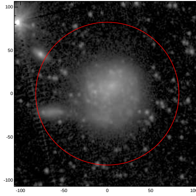
LEDA: pa,inc= 999.0 25.1
