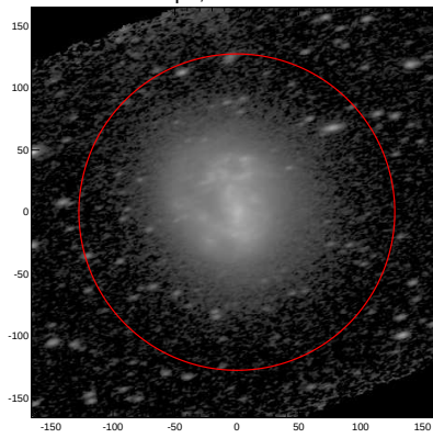
LEDA: pa,inc= 17.5 61.5
