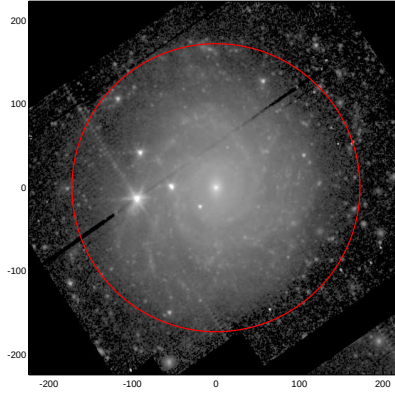
LEDA: pa,inc= 999.0 18.1
