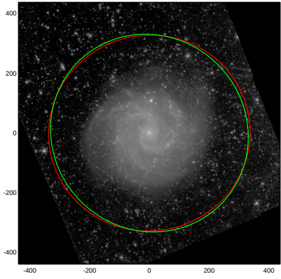
NGC3184
