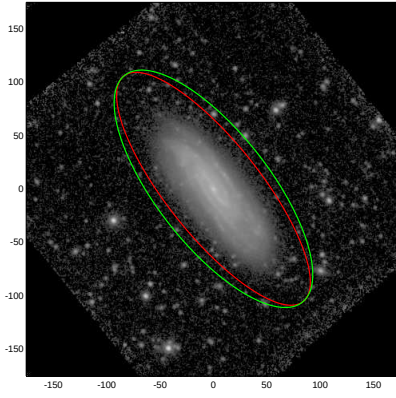
NGC3549
