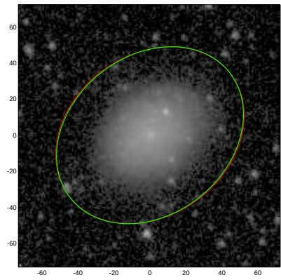
NGC3213
