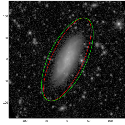
NGC3361
