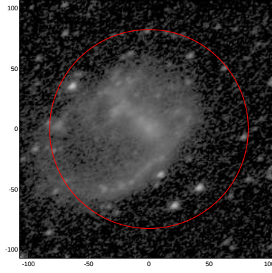
LEDA: pa,inc= 33.5 49.8
