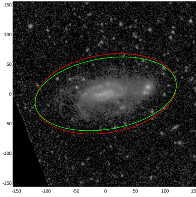
NGC3020
