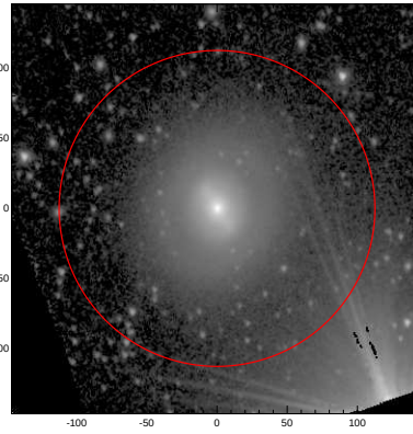
LEDA: pa,inc= 999.0 29.2
