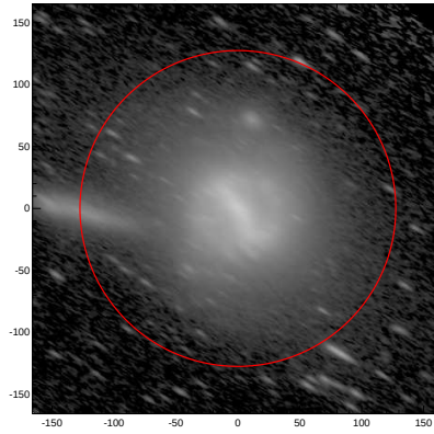
LEDA: pa,inc= 149.4 71.7
