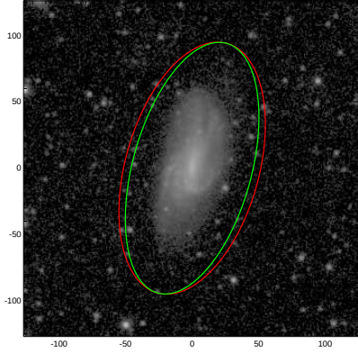
NGC3153
