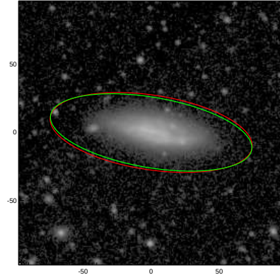
NGC3043
