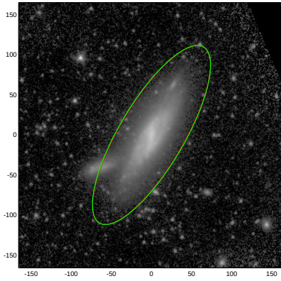
NGC3769
