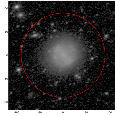
LEDA: pa,inc= 22.0 45.3
