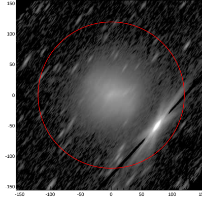
LEDA: pa,inc= 55.4 76.4
