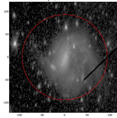
LEDA: pa,inc= 87.1 58.9
