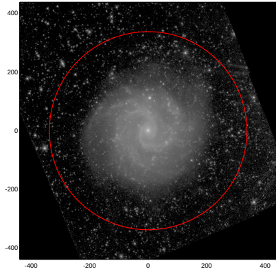
LEDA: pa,inc= 999.0 13.9
