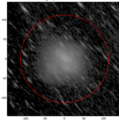
LEDA: pa,inc= 131.0 75.8
