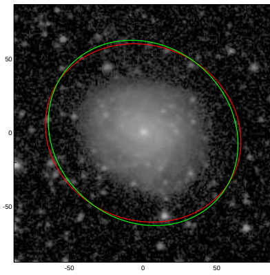
NGC3364
