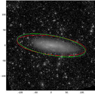
NGC3026
