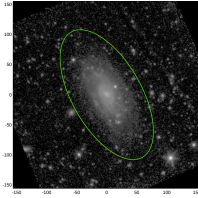
NGC3321
