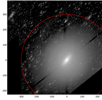
LEDA: pa,inc= 53.0 63.1
