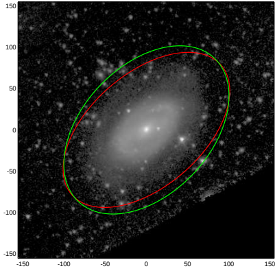
NGC3185
