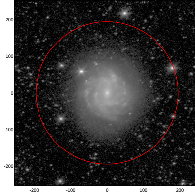
LEDA: pa,inc= 9.5 38.1
