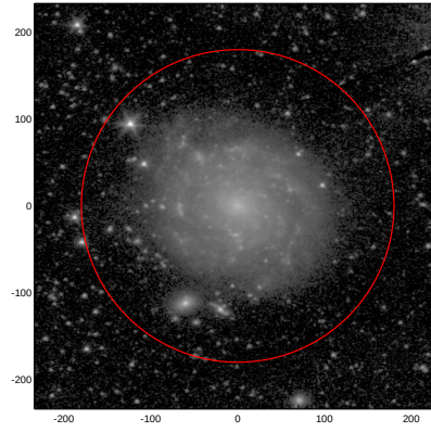
LEDA: pa,inc= 1.7 31.4
