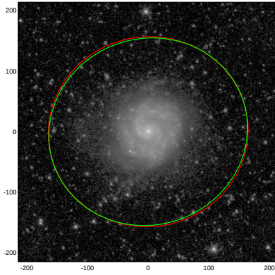
NGC3596
