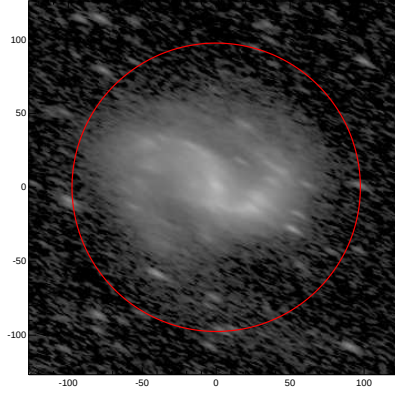
LEDA: pa,inc= 154.1 71.9
