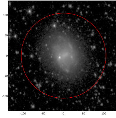
LEDA: pa,inc= 999.0 31.4
