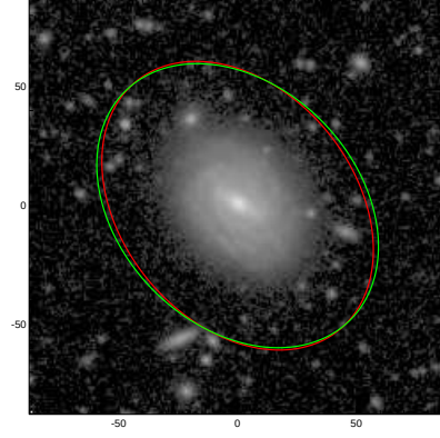
NGC4067
