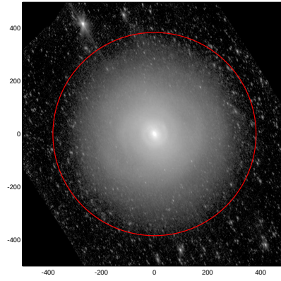
LEDA: pa,inc= 113.5 59.5
