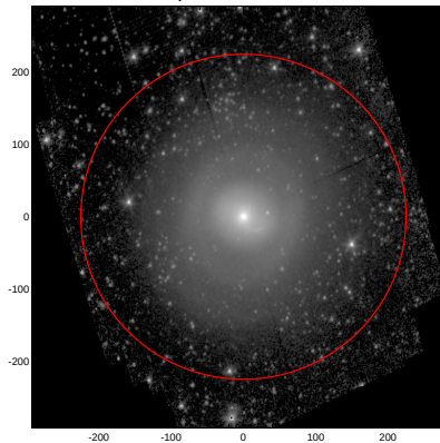
LEDA: pa,inc= 78.5 32.1
