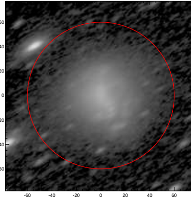
LEDA: pa,inc= 33.3 65.9
