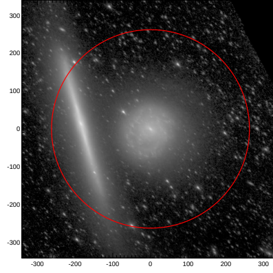
LEDA: pa,inc= 135.7 56.6
