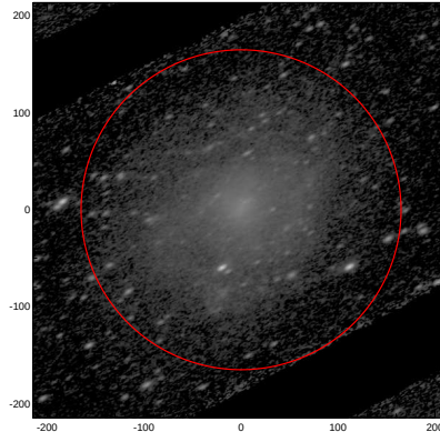
LEDA: pa,inc= 30.1 61.5
