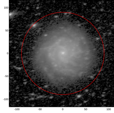
LEDA: pa,inc= 15.0 54.6
