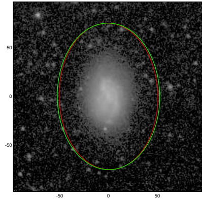
NGC4470
