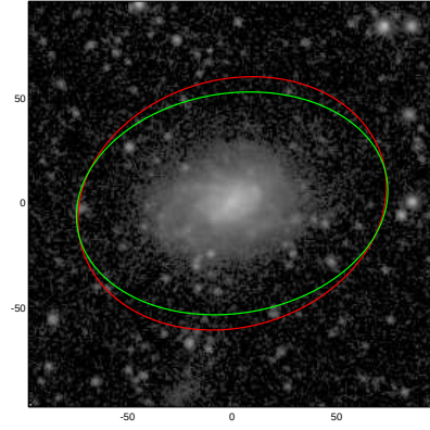
NGC4961
