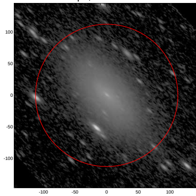
LEDA: pa,inc= 139.1 69.2
