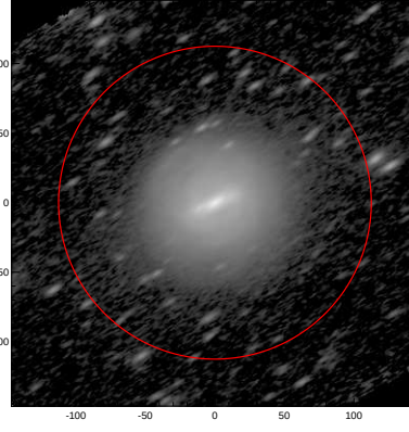
LEDA: pa,inc= 32.2 69.5
