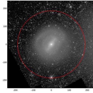
LEDA: pa,inc= 999.0 15.9
