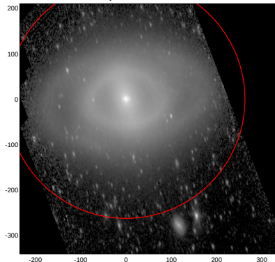
LEDA: pa,inc= 101.7 62.1
