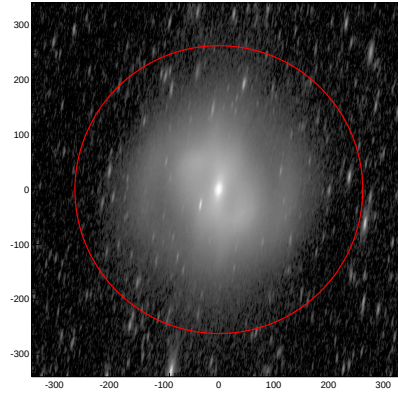
LEDA: pa,inc= 81.0 77.4
