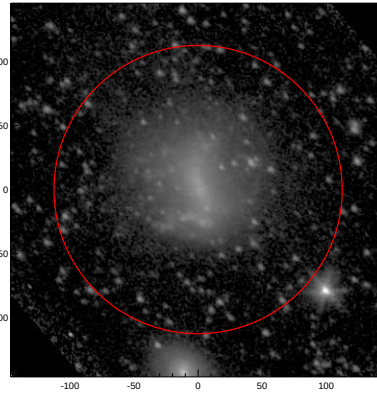
LEDA: pa,inc= 135.9 37.6
