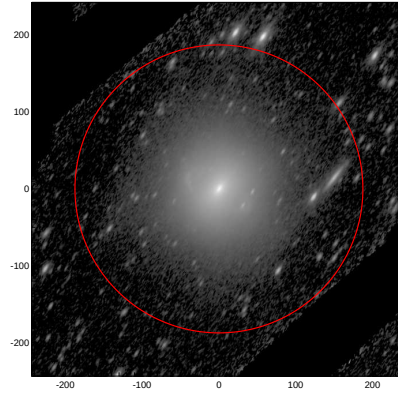
LEDA: pa,inc= 56.3 66.3
