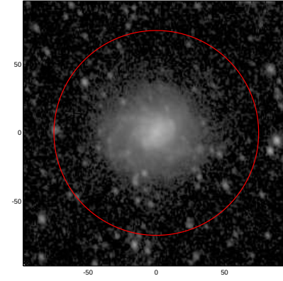
LEDA: pa,inc= 106.6 37.9
