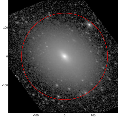
LEDA: pa,inc= 143.0 46.2
