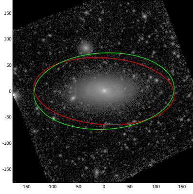
NGC4309
