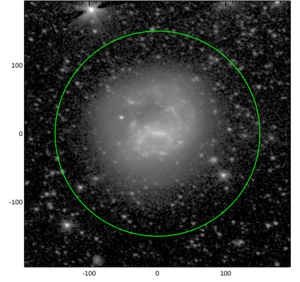
S4G: pa,inc= -9.2 35.9
