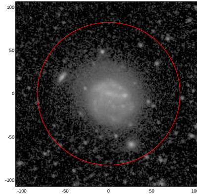
LEDA: pa,inc= 999.0 15.5
