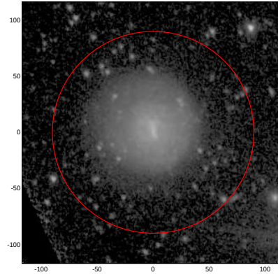
LEDA: pa,inc= 112.2 29.0
