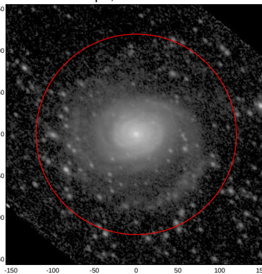
LEDA: pa,inc= 131.6 43.2
