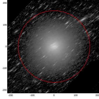
LEDA: pa,inc= 39.8 74.4
