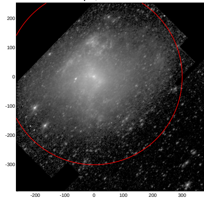
LEDA: pa,inc= 46.5 54.4
