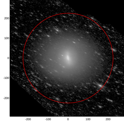
LEDA: pa,inc= 151.7 66.1
