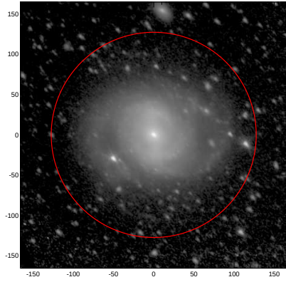
LEDA: pa,inc= 136.6 49.0
