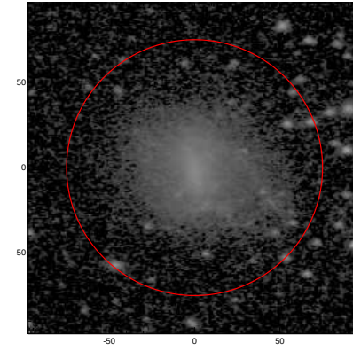
LEDA: pa,inc= 179.7 43.9
