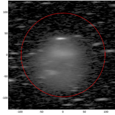
LEDA: pa,inc= 2.0 76.6
