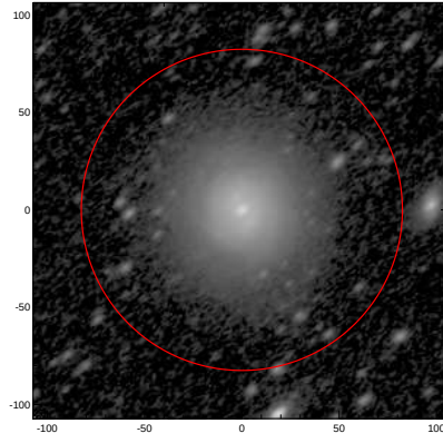
LEDA: pa,inc= 39.7 56.8
