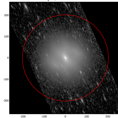
LEDA: pa,inc= 115.7 70.9
