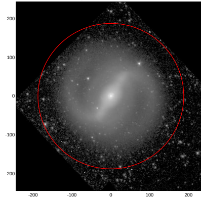
LEDA: pa,inc= 999.0 15.5
