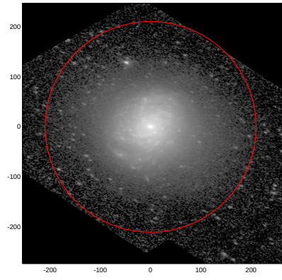
LEDA: pa,inc= 164.5 54.9
