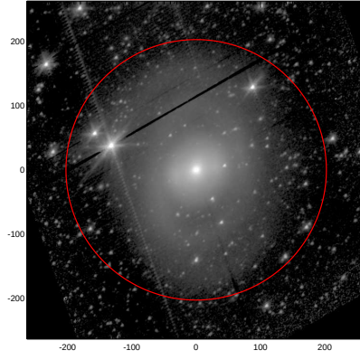
LEDA: pa,inc= 45.0 42.0
