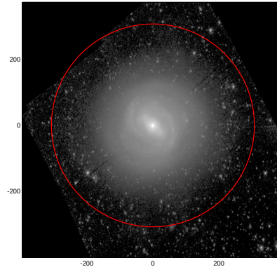
LEDA: pa,inc= 88.8 40.0
