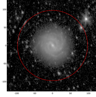
LEDA: pa,inc= 99.9 44.3
