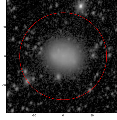
LEDA: pa,inc= 64.9 39.6
