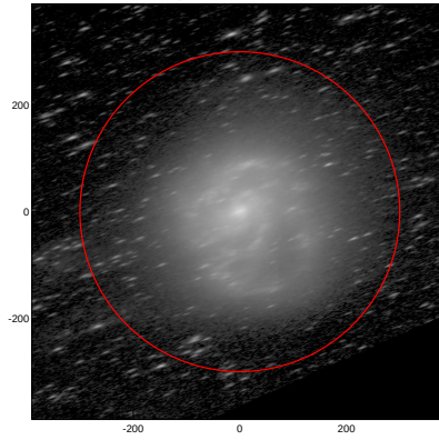
LEDA: pa,inc= 20.0 75.4
