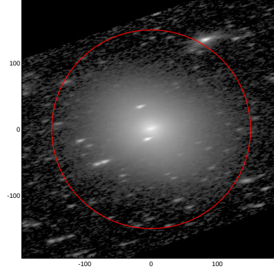
LEDA: pa,inc= 16.2 71.1
