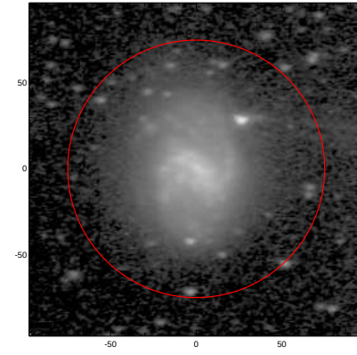
LEDA: pa,inc= 2.5 51.5
