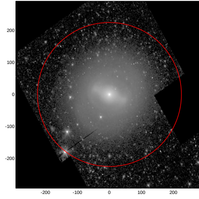
LEDA: pa,inc= 999.0 32.9
