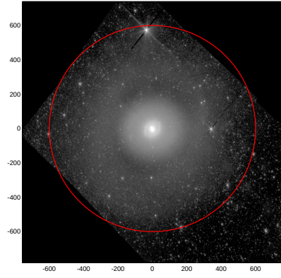
LEDA: pa,inc= 105.0 30.3
