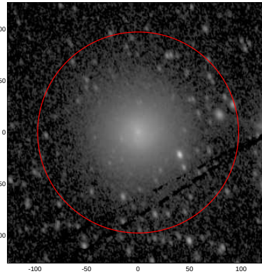
LEDA: pa,inc= 107.6 47.0
