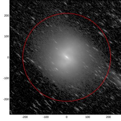
LEDA: pa,inc= 140.3 74.9
