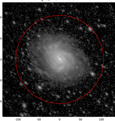
LEDA: pa,inc= 135.9 49.2
