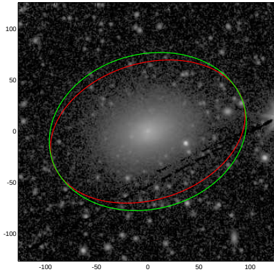
NGC4506
