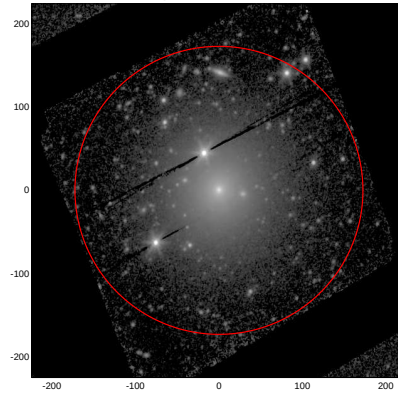
LEDA: pa,inc= 64.5 27.5
