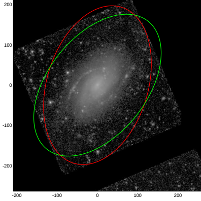
NGC4504
