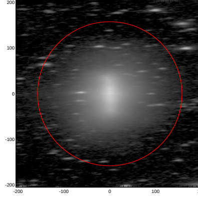
LEDA: pa,inc= 2.7 78.4
