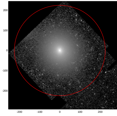
LEDA: pa,inc= 999.0 11.6
