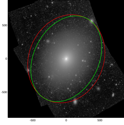
NGC4472
