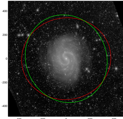
NGC4535
