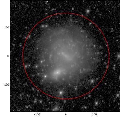
LEDA: pa,inc= 67.5 34.5
