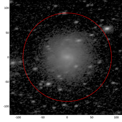
LEDA: pa,inc= 13.6 52.7
