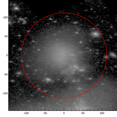
LEDA: pa,inc= 179.7 48.3
