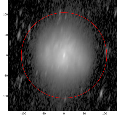
LEDA: pa,inc= 77.3 75.2
