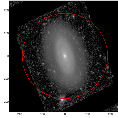
LEDA: pa,inc= 999.0 34.9
