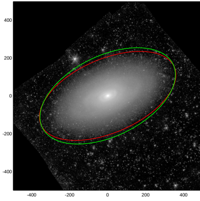
NGC4826
