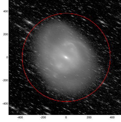
LEDA: pa,inc= 151.8 76.1
