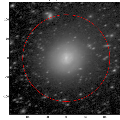
LEDA: pa,inc= 21.9 49.8
