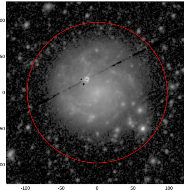
LEDA: pa,inc= 58.5 28.0
