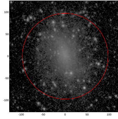
LEDA: pa,inc= 999.0 22.1
