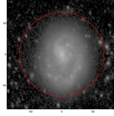
LEDA: pa,inc= 999.0 41.0
