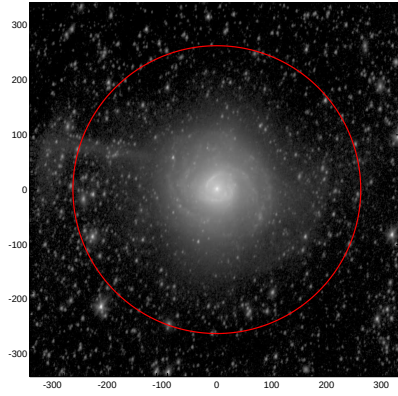
LEDA: pa,inc= 76.8 48.2
