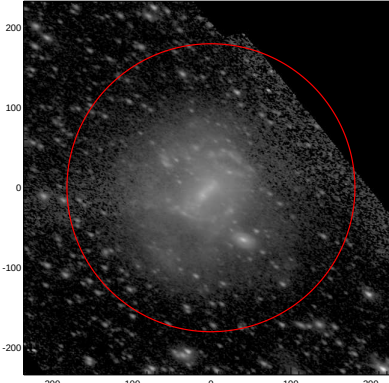
LEDA: pa,inc= 151.2 54.6
