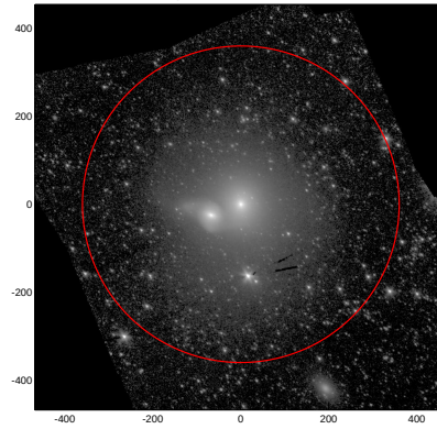
LEDA: pa,inc= 136.4 37.9
