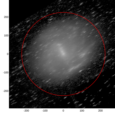
LEDA: pa,inc= 32.0 74.5
