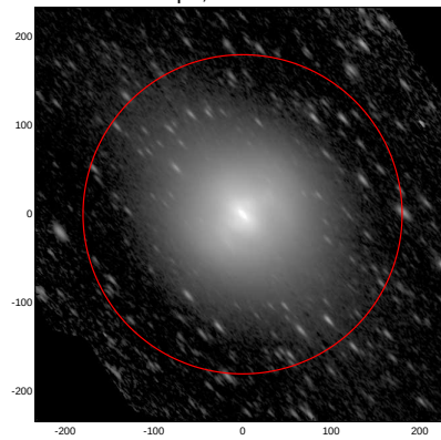
LEDA: pa,inc= 132.0 70.5
