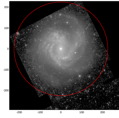
LEDA: pa,inc= 999.0 17.7
