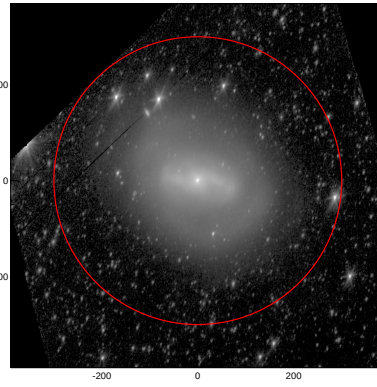
LEDA: pa,inc= 72.0 53.4
