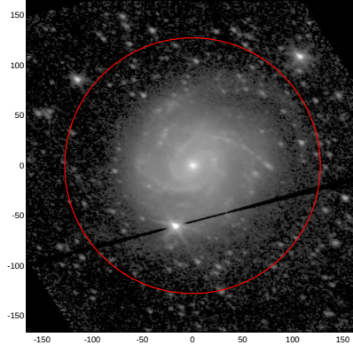
LEDA: pa,inc= 155.3 43.2
