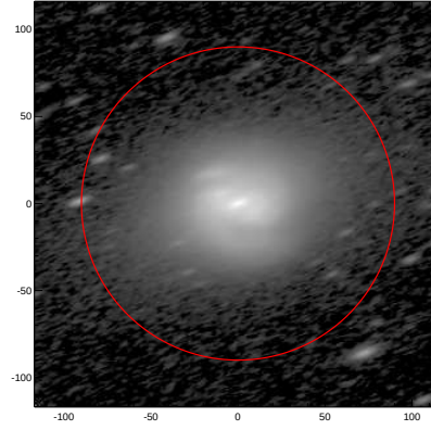
LEDA: pa,inc= 21.0 70.2
