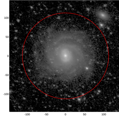
LEDA: pa,inc= 153.4 37.1
