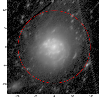
LEDA: pa,inc= 51.6 59.1
