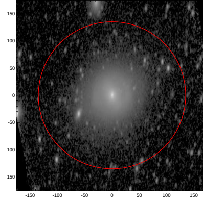
LEDA: pa,inc= 86.3 61.7
