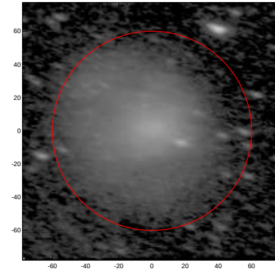
LEDA: pa,inc= 165.4 63.7
