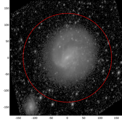
LEDA: pa,inc= 73.5 42.2
