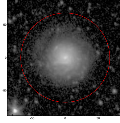
LEDA: pa,inc= 104.5 35.3
