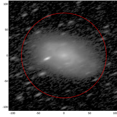
LEDA: pa,inc= 24.1 69.9
