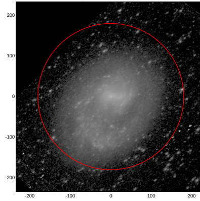
LEDA: pa,inc= 40.2 50.1
