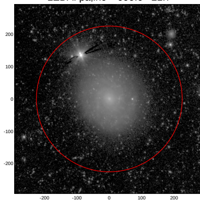
LEDA: pa,inc= 999.0 21.7
