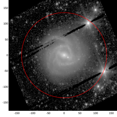
LEDA: pa,inc= 78.0 25.6
