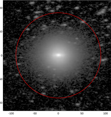
LEDA: pa,inc= 5.0 57.5
