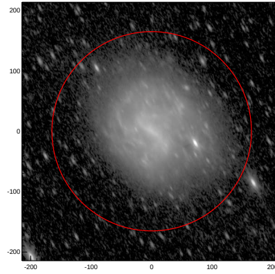
LEDA: pa,inc= 118.3 66.3
