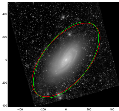
NGC4501
