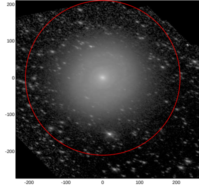
LEDA: pa,inc= 159.7 57.9
