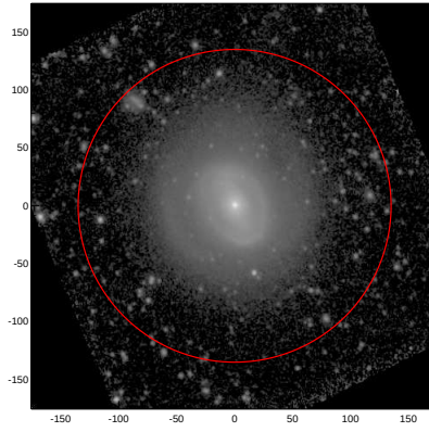
LEDA: pa,inc= 999.0 23.3
