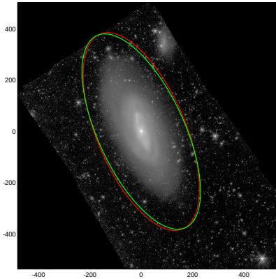
NGC4569
