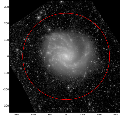
LEDA: pa,inc= 999.0 19.6
