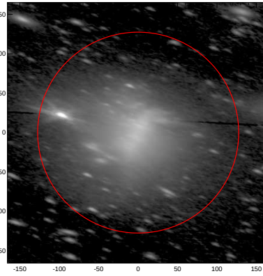
LEDA: pa,inc= 161.8 69.4
