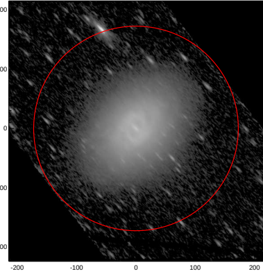
LEDA: pa,inc= 133.2 71.5
