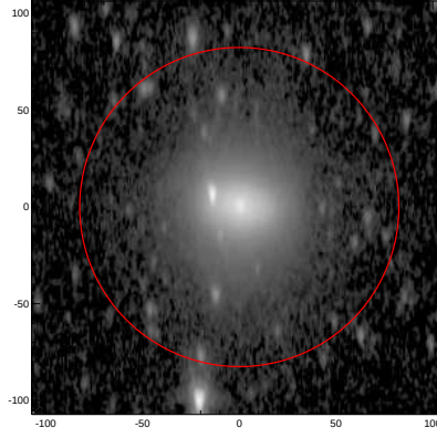
LEDA: pa,inc= 91.0 64.4
