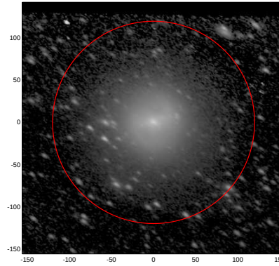
LEDA: pa,inc= 147.7 58.3
