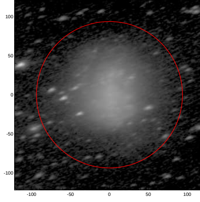
LEDA: pa,inc= 19.6 64.0
