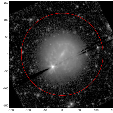
LEDA: pa,inc= 999.0 18.5
