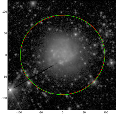
NGC4299
