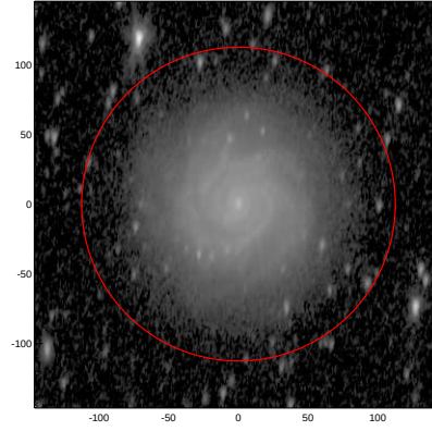
LEDA: pa,inc= 84.3 62.7
