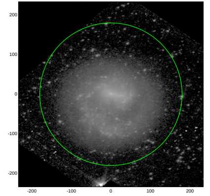
S4G: pa,inc= 13.3 42.0
