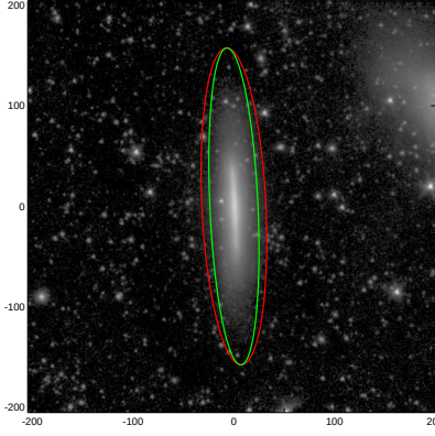
NGC4607
