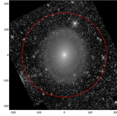
LEDA: pa,inc= 999.0 22.7
