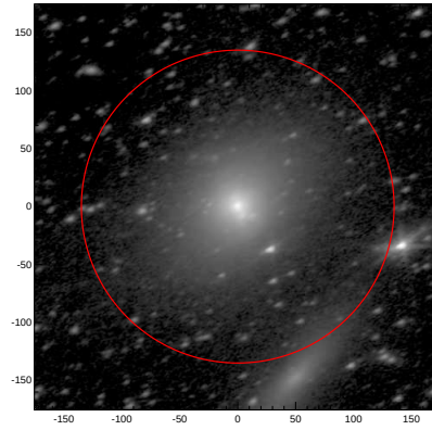
LEDA: pa,inc= 24.0 57.6
