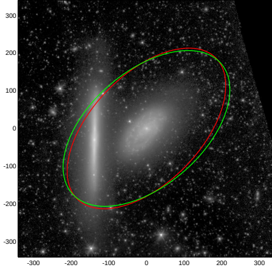
NGC4298
