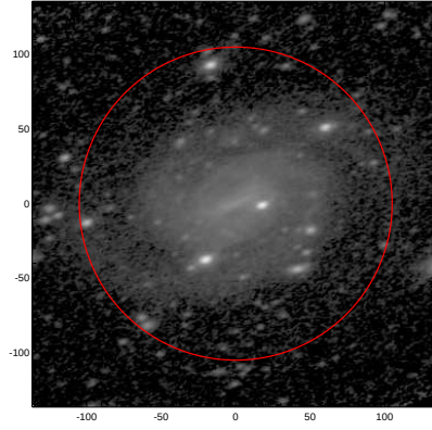
LEDA: pa,inc= 19.0 52.9
