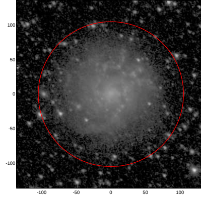
LEDA: pa,inc= 141.7 34.5
