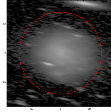
LEDA: pa,inc= 167.2 76.1
