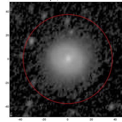
LEDA: pa,inc= 64.5 48.9
