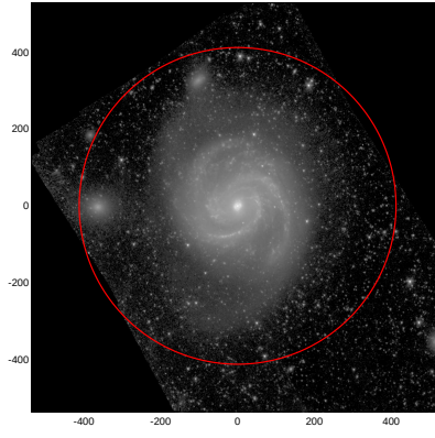
LEDA: pa,inc= 999.0 22.7
