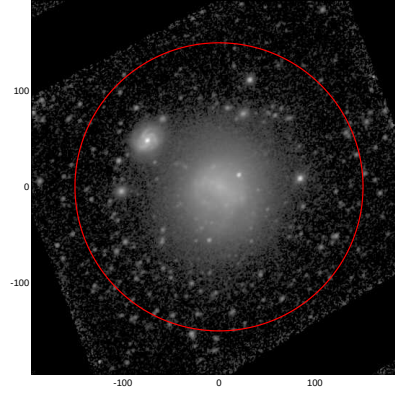
LEDA: pa,inc= 44.9 33.5
