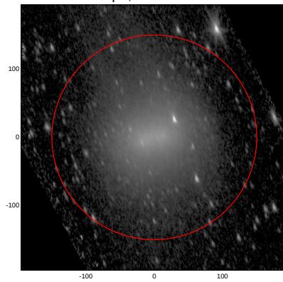
LEDA: pa,inc= 108.0 63.4
