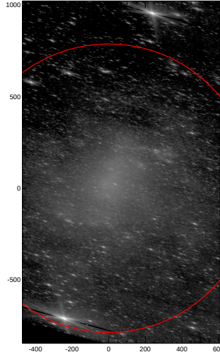
LEDA: pa,inc= 162.0 73.0
