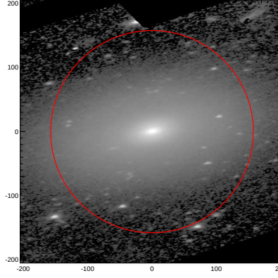
LEDA: pa,inc= 10.3 65.4
