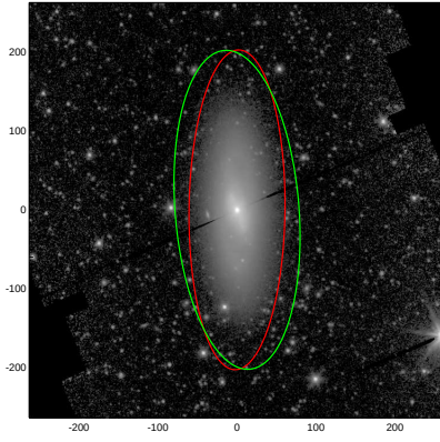
NGC4818
