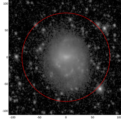
LEDA: pa,inc= 999.0 27.7
