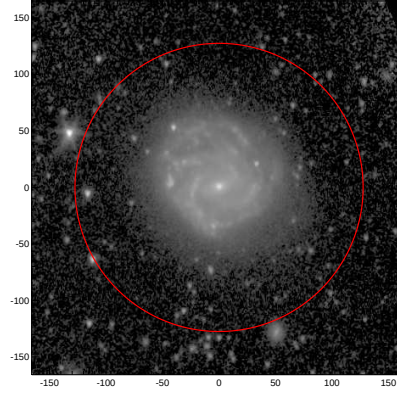
LEDA: pa,inc= 87.5 35.3
