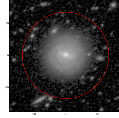
LEDA: pa,inc= 39.4 43.6
