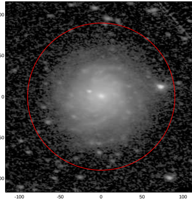
LEDA: pa,inc= 173.3 53.0
