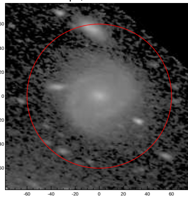
LEDA: pa,inc= 162.4 57.3
