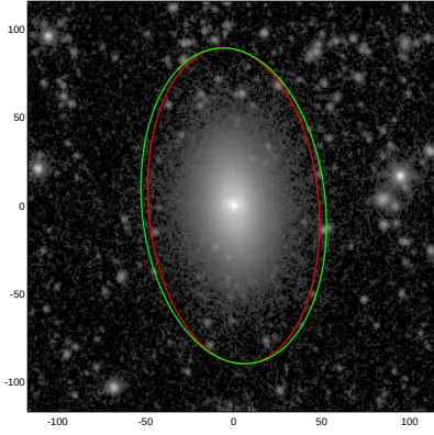
NGC4528
