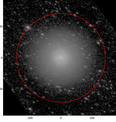
LEDA: pa,inc= 155.4 49.3
