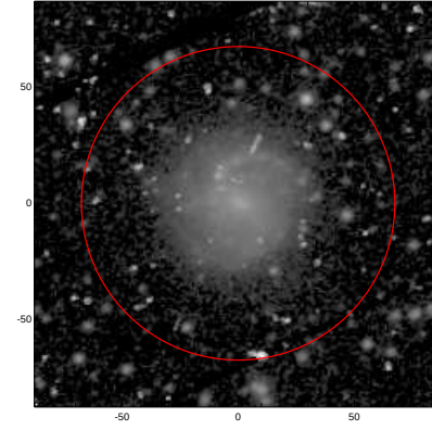
LEDA: pa,inc= 21.5 25.9
