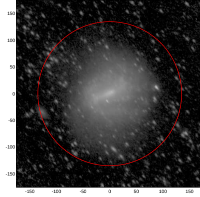
LEDA: pa,inc= 132.0 56.0
