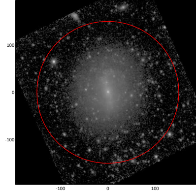
LEDA: pa,inc= 999.0 21.1
