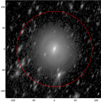
LEDA: pa,inc= 65.4 61.3
