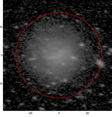
LEDA: pa,inc= 174.6 58.8
