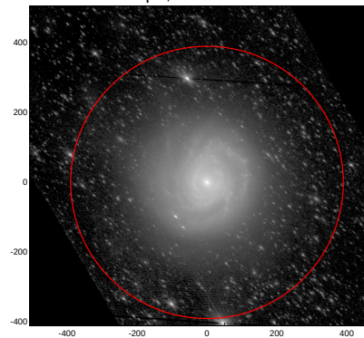
LEDA: pa,inc= 138.8 59.6
