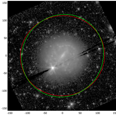
NGC4900
