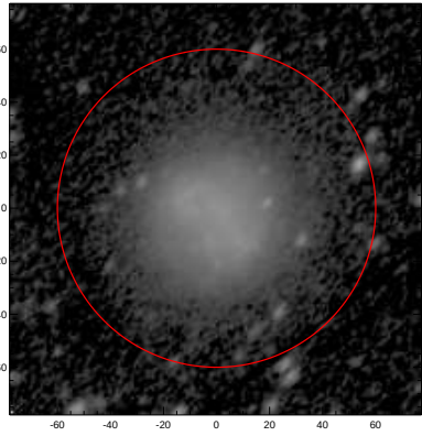
LEDA: pa,inc= 50.7 51.5
