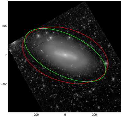
NGC4293
