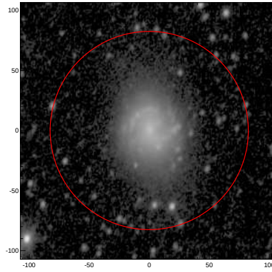
LEDA: pa,inc= 73.0 40.5
