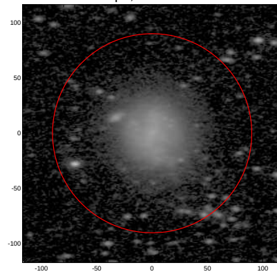
LEDA: pa,inc= 2.9 54.7
