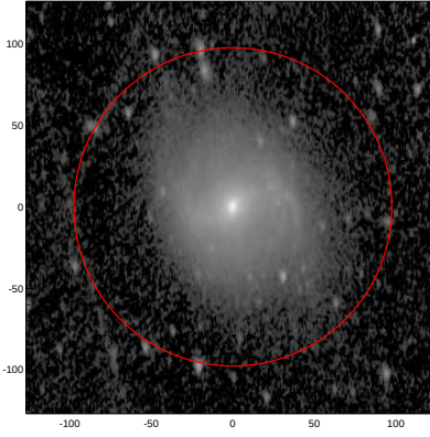
LEDA: pa,inc= 92.4 57.4
