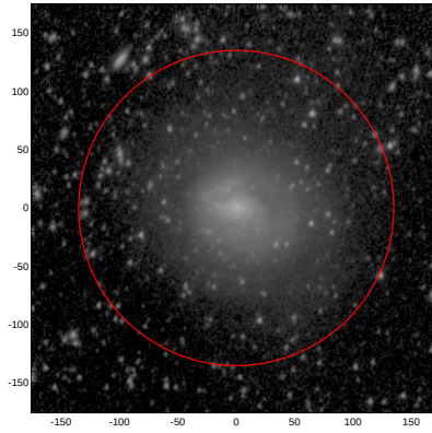
LEDA: pa,inc= 71.9 35.8
