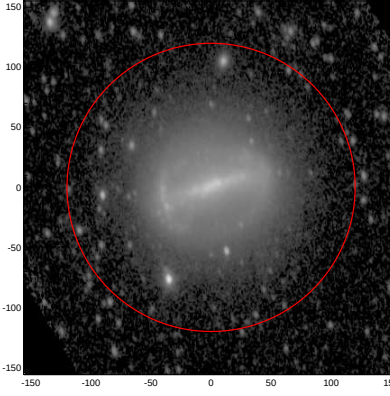
LEDA: pa,inc= 96.0 48.3
