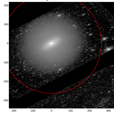
LEDA: pa,inc= 22.0 62.0
