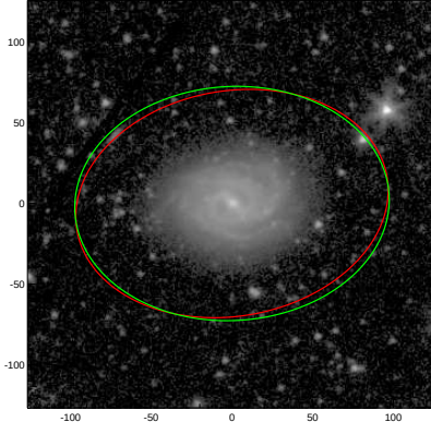
NGC4210
