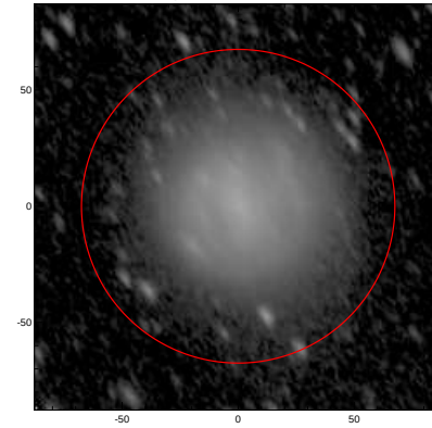
LEDA: pa,inc= 120.5 61.7
