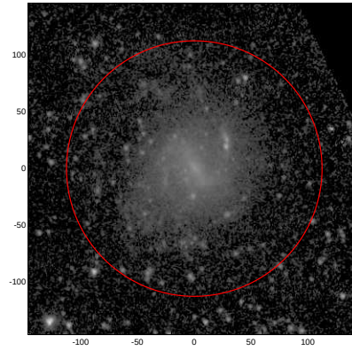
LEDA: pa,inc= 999.0 23.3
