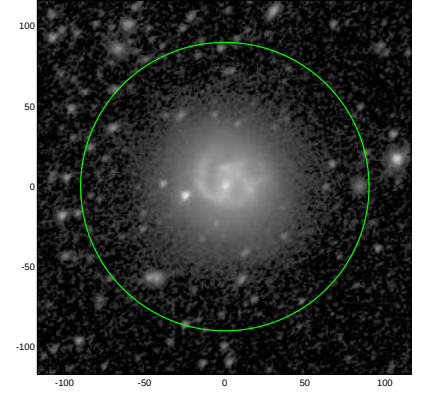
S4G: pa,inc= 38.4 39.2
