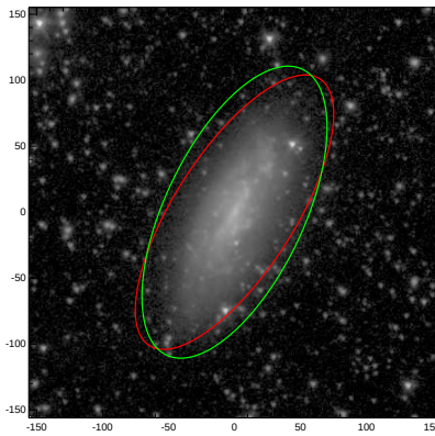
NGC4294
