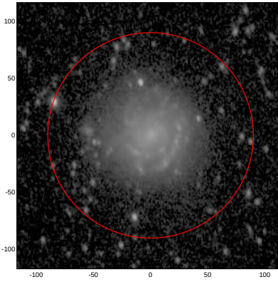
LEDA: pa,inc= 98.7 42.2
