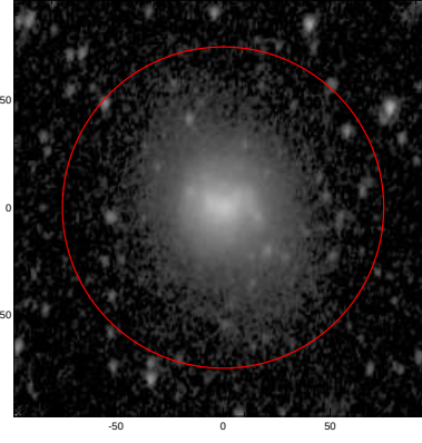
LEDA: pa,inc= 80.0 45.6
