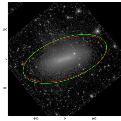
NGC4248
