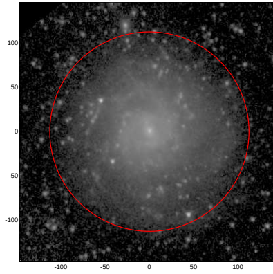
LEDA: pa,inc= 999.0 21.7
