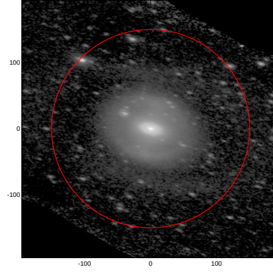
LEDA: pa,inc= 165.3 59.9
