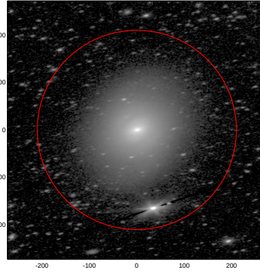
LEDA: pa,inc= 11.3 62.9
