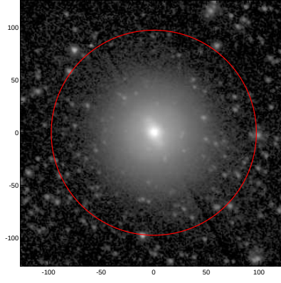
LEDA: pa,inc= 145.0 29.0
