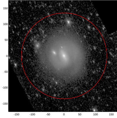
LEDA: pa,inc= 115.7 49.0
