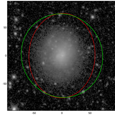
NGC4032
