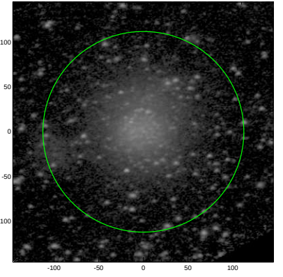
S4G: pa,inc= 10.6 45.2
