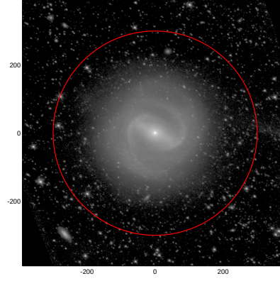
LEDA: pa,inc= 150.0 35.4
