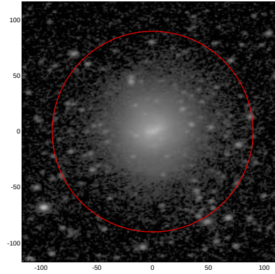
LEDA: pa,inc= 8.8 46.5
