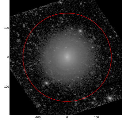
LEDA: pa,inc= 163.4 41.6
