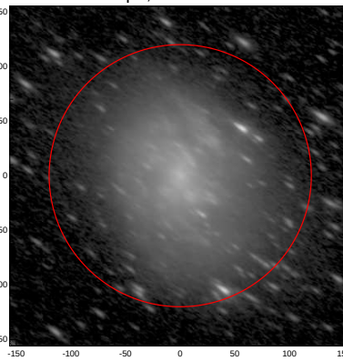
LEDA: pa,inc= 147.4 67.7
