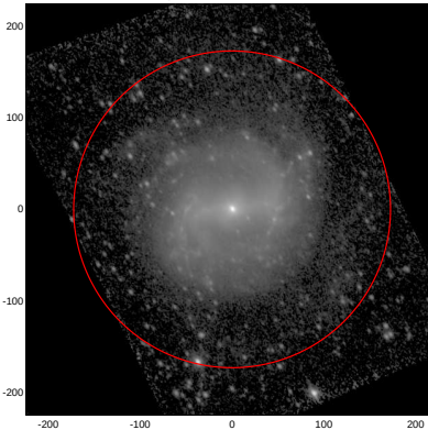
LEDA: pa,inc= 123.7 43.2
