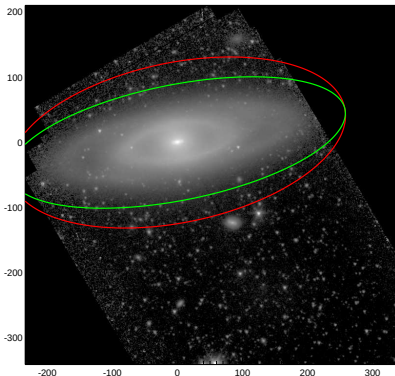
NGC4274
