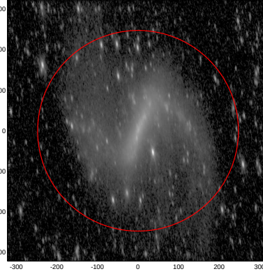
LEDA: pa,inc= 97.2 70.2
