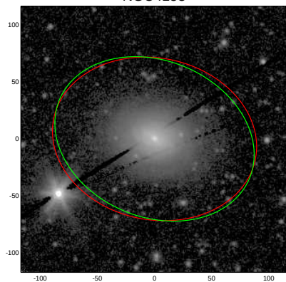
NGC4158
