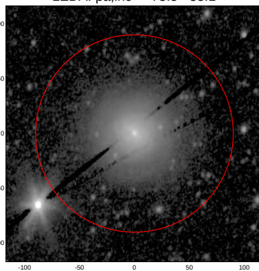
LEDA: pa,inc= 78.5 38.1
