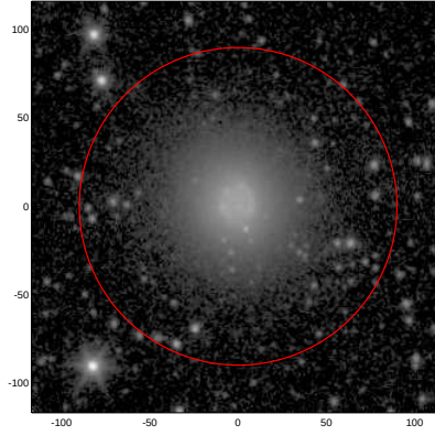
LEDA: pa,inc= 999.0 15.0
