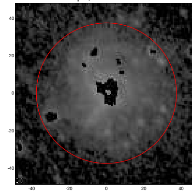
LEDA: pa,inc= 120.7 40.2
