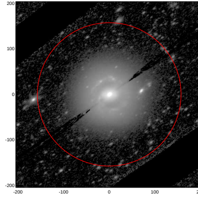
LEDA: pa,inc= 38.0 55.3
