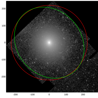
NGC4278
