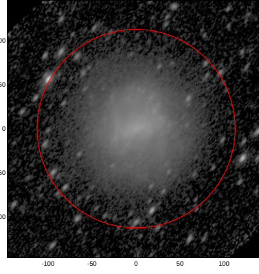
LEDA: pa,inc= 52.4 59.0
