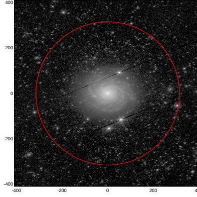
LEDA: pa,inc= 16.9 45.5
