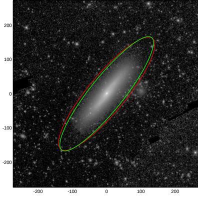
NGC4313
