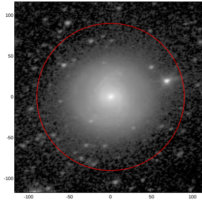
LEDA: pa,inc= 19.4 45.1
