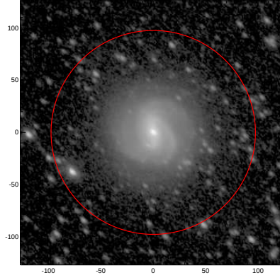
LEDA: pa,inc= 133.3 49.0
