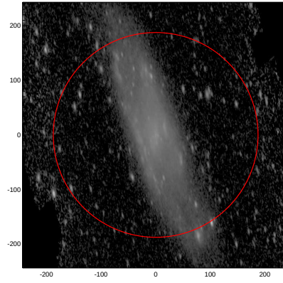
LEDA: pa,inc= 999.0 66.4
