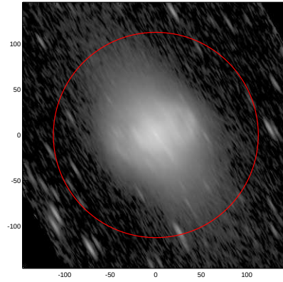
LEDA: pa,inc= 120.3 78.0
