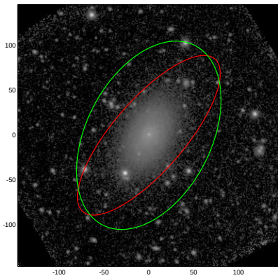
NGC4286
