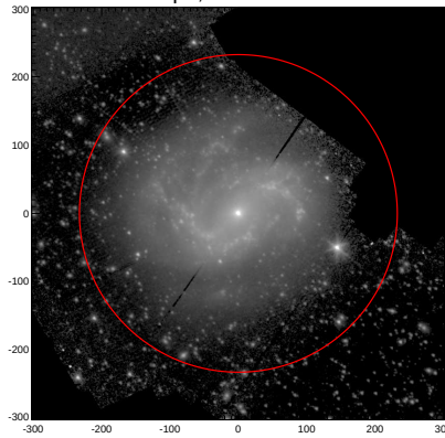
LEDA: pa,inc= 135.0 29.4
