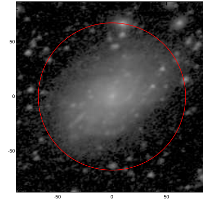
LEDA: pa,inc= 24.9 43.3
