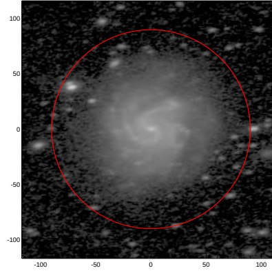
LEDA: pa,inc= 9.7 55.8
