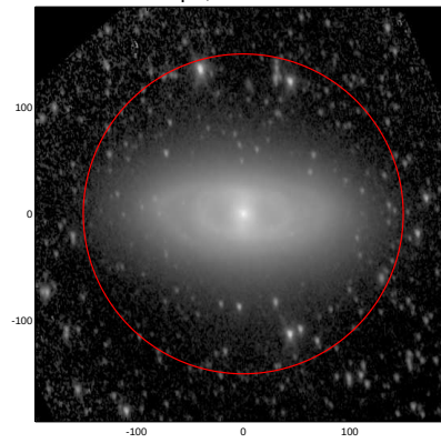
LEDA: pa,inc= 97.9 49.2
