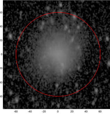
LEDA: pa,inc= 91.3 46.2
