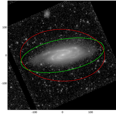
NGC4602
