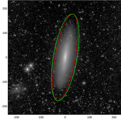
NGC4312
