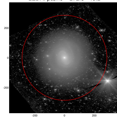
LEDA: pa,inc= 172.3 46.2
