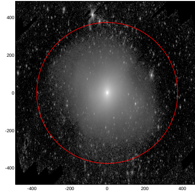
LEDA: pa,inc= 88.1 61.8
