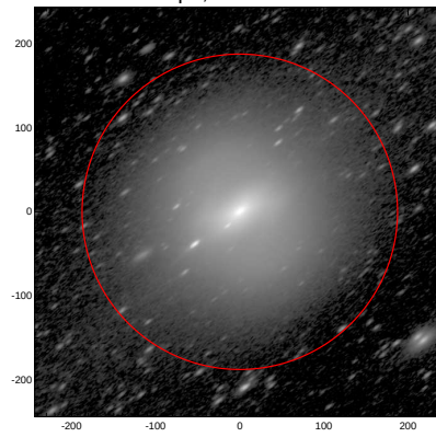
LEDA: pa,inc= 38.3 68.3
