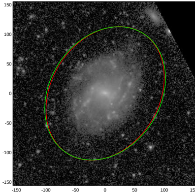
NGC4519
