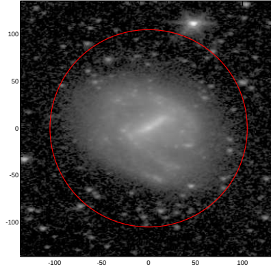
LEDA: pa,inc= 2.6 51.4
