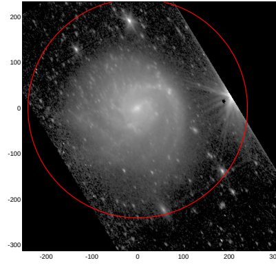
LEDA: pa,inc= 121.2 58.2
