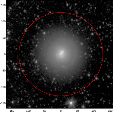
LEDA: pa,inc= 999.0 17.7
