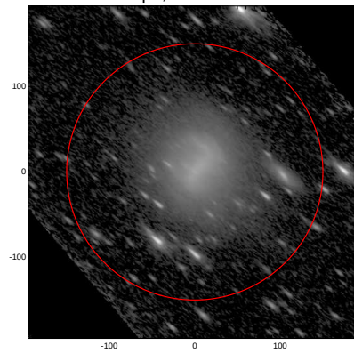
LEDA: pa,inc= 141.1 69.1
