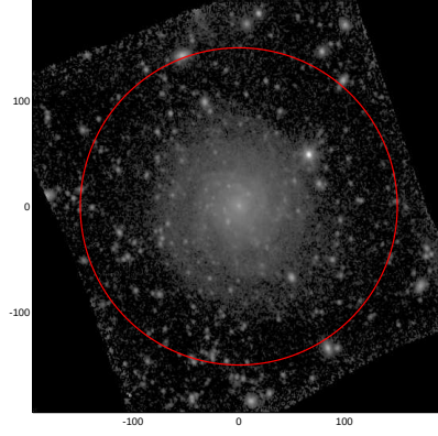
LEDA: pa,inc= 999.0 26.2
