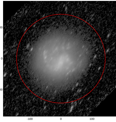
LEDA: pa,inc= 58.5 67.4
