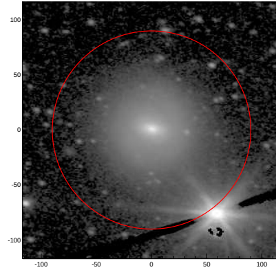
LEDA: pa,inc= 173.2 44.9
