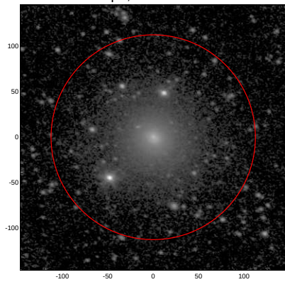
LEDA: pa,inc= 167.4 34.9
