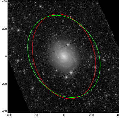
NGC4030
