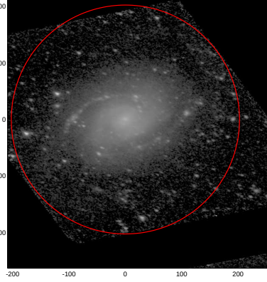
LEDA: pa,inc= 163.0 51.7
