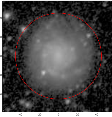
LEDA: pa,inc= 51.6 32.1
