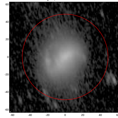
LEDA: pa,inc= 104.4 65.6
