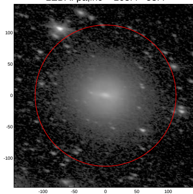
LEDA: pa,inc= 163.4 58.4
