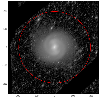
LEDA: pa,inc= 59.1 62.7
