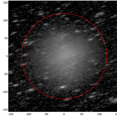
LEDA: pa,inc= 15.4 69.6
