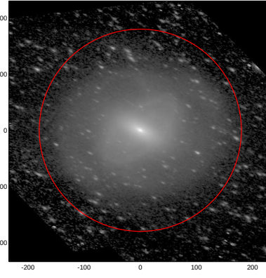
LEDA: pa,inc= 155.9 60.9
