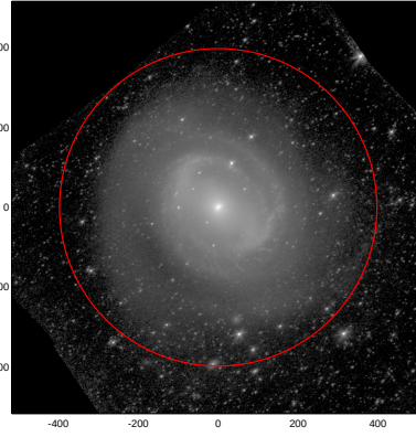
LEDA: pa,inc= 36.0 43.0
