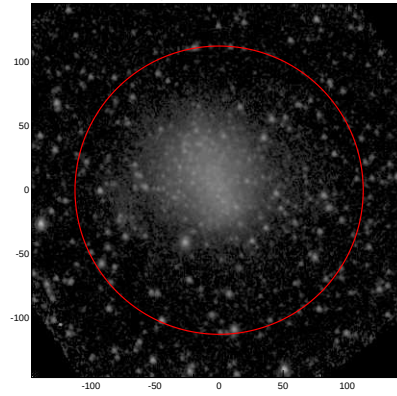
LEDA: pa,inc= 999.0 22.1
