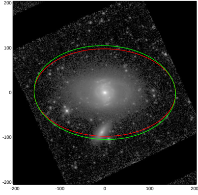
NGC4045
