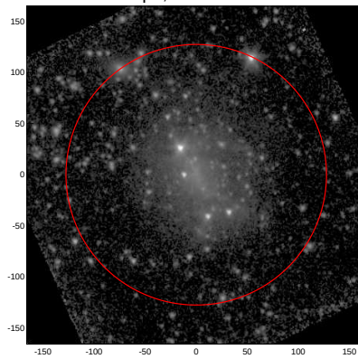
LEDA: pa,inc= 999.0 22.7
