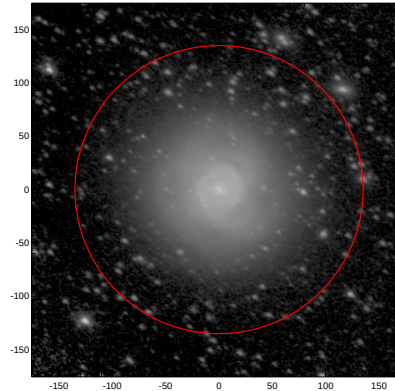
LEDA: pa,inc= 153.4 47.1
