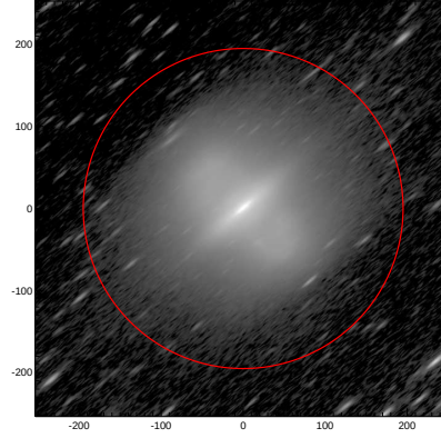
LEDA: pa,inc= 40.7 78.8
