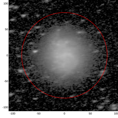
LEDA: pa,inc= 9.5 60.9
