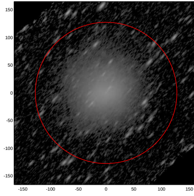
LEDA: pa,inc= 49.0 70.7
