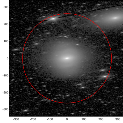
LEDA: pa,inc= 7.7 70.1
