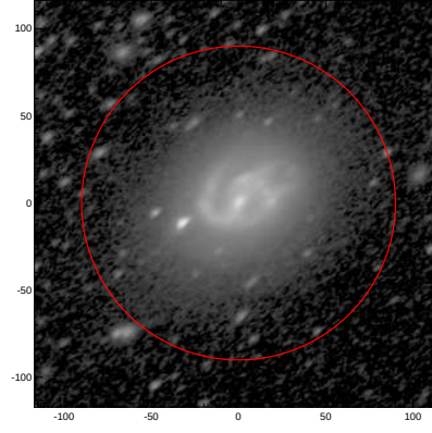
LEDA: pa,inc= 38.7 56.2
