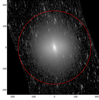
LEDA: pa,inc= 99.5 68.9
