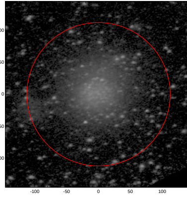
LEDA: pa,inc= 11.8 47.5
