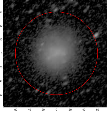
LEDA: pa,inc= 43.9 58.6
