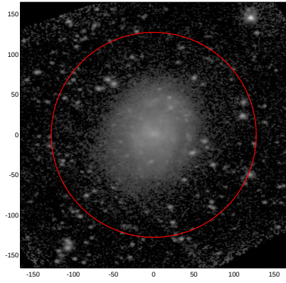
LEDA: pa,inc= 3.0 43.9
