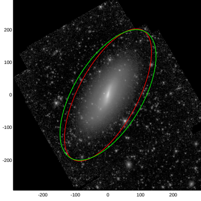
NGC4064
