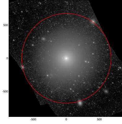
LEDA: pa,inc= 157.1 34.9
