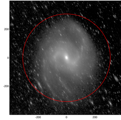
LEDA: pa,inc= 118.5 68.9
