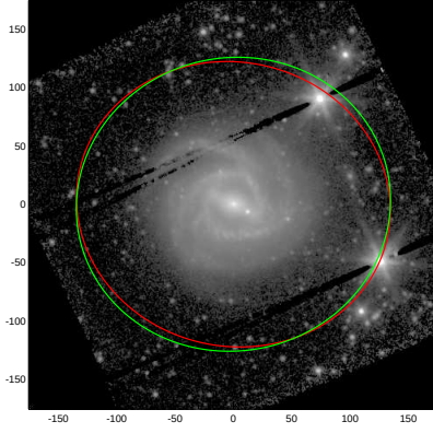
NGC4902
