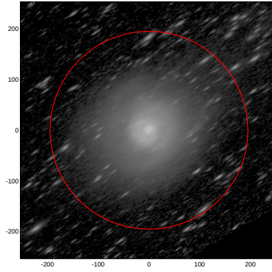
LEDA: pa,inc= 34.9 75.0
