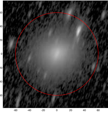
LEDA: pa,inc= 71.0 71.6
