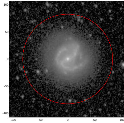
LEDA: pa,inc= 999.0 25.9
