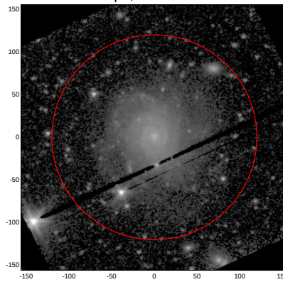
LEDA: pa,inc= 15.3 25.9
