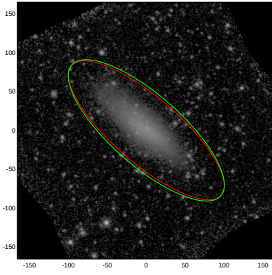
NGC4562
