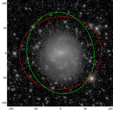
NGC4276
