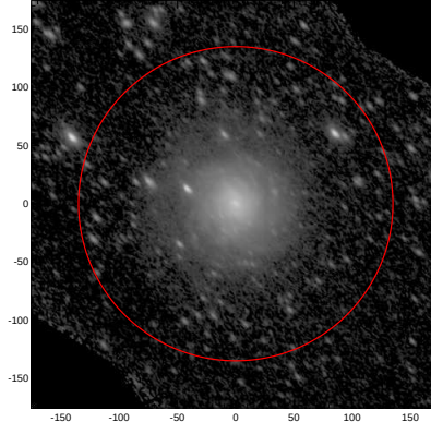
LEDA: pa,inc= 132.8 57.3
