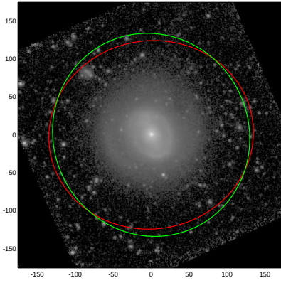
NGC4454
