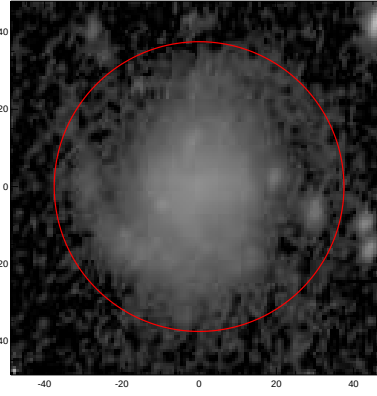
LEDA: pa,inc= 70.6 50.2
