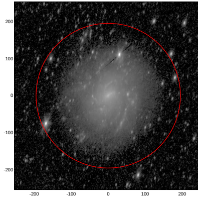
LEDA: pa,inc= 74.2 56.8
