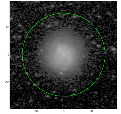
S4G: pa,inc= 0.7 45.6
