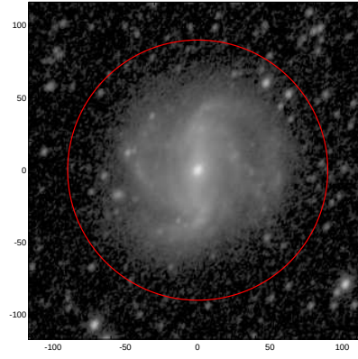
LEDA: pa,inc= 58.7 45.1
