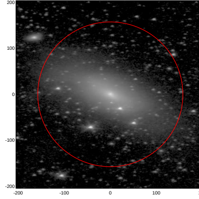
LEDA: pa,inc= 1.6 56.5
