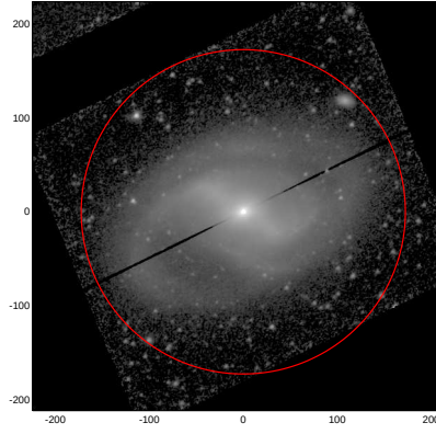
LEDA: pa,inc= 37.9 31.9
