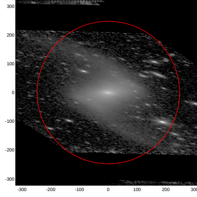
LEDA: pa,inc= 166.9 74.1
