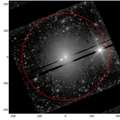
LEDA: pa,inc= 17.5 29.4
