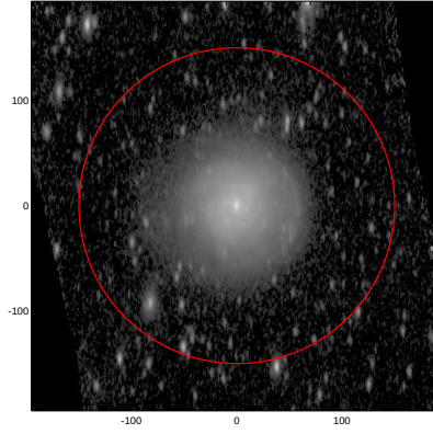
LEDA: pa,inc= 89.1 63.5
