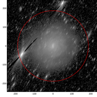
LEDA: pa,inc= 62.0 69.9
