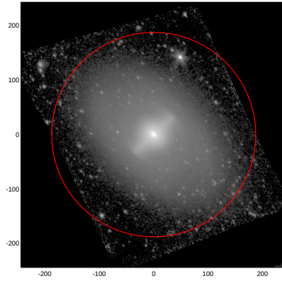
LEDA: pa,inc= 131.7 38.6
