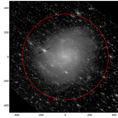
LEDA: pa,inc= 147.5 62.9
