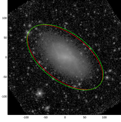
NGC4525
