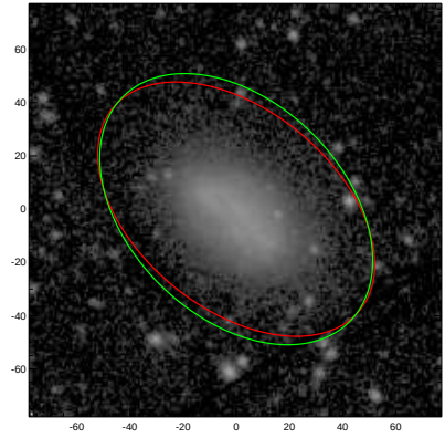
NGC4049
