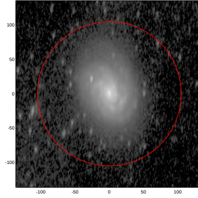
LEDA: pa,inc= 86.3 65.4
