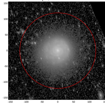
LEDA: pa,inc= 104.9 49.8
