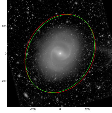
NGC4548
