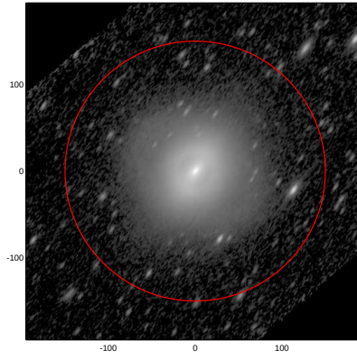
LEDA: pa,inc= 55.0 66.0
