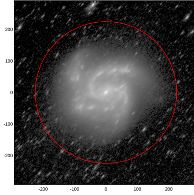
LEDA: pa,inc= 49.5 67.8
