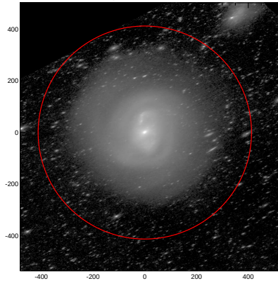
LEDA: pa,inc= 23.0 65.2
