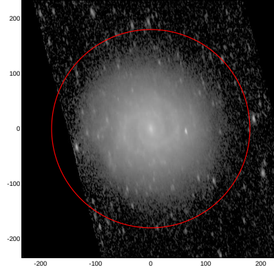
LEDA: pa,inc= 100.8 67.2
