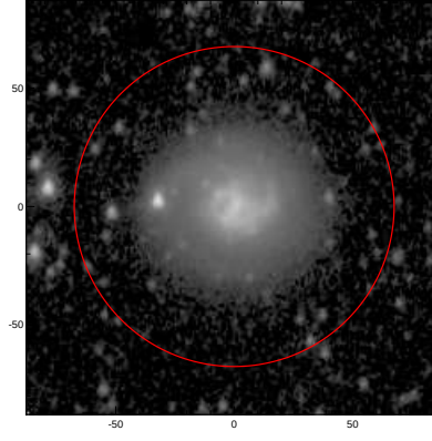
LEDA: pa,inc= 82.7 39.1
