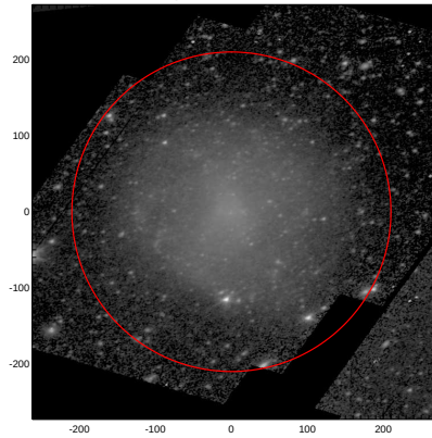
LEDA: pa,inc= 20.8 45.3
