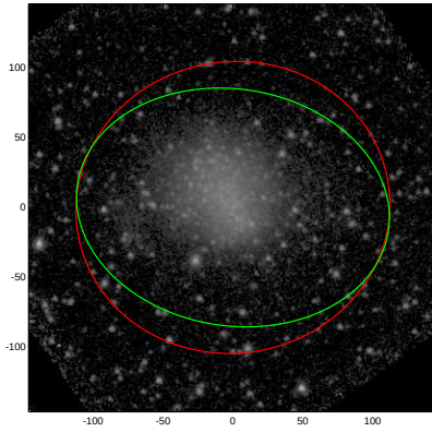
NGC4190
