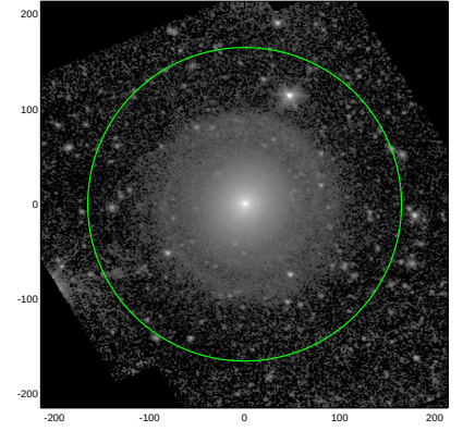
S4G: pa,inc= -9.2 32.4
