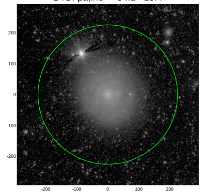
S4G: pa,inc= 84.1 19.4
