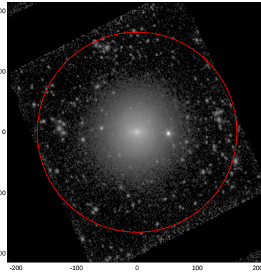
LEDA: pa,inc= 999.0 22.1
