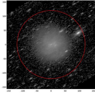
LEDA: pa,inc= 33.5 65.1
