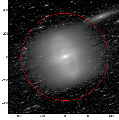
LEDA: pa,inc= 19.7 76.4
