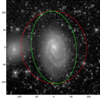
NGC4273
