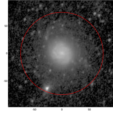
LEDA: pa,inc= 63.1 38.1
