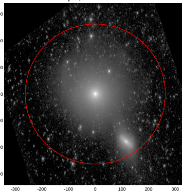
LEDA: pa,inc= 89.7 48.5
