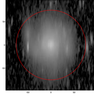
LEDA: pa,inc= 89.0 79.0
