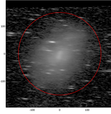
LEDA: pa,inc= 176.7 77.5
