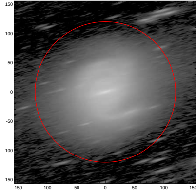
LEDA: pa,inc= 14.5 80.9
