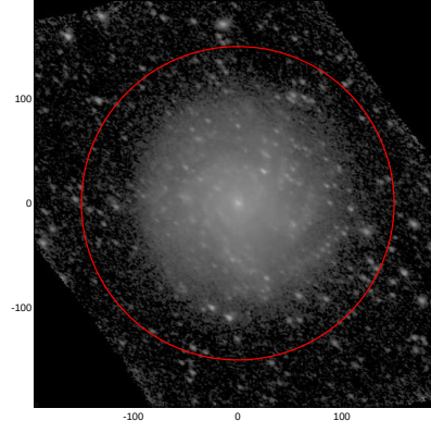
LEDA: pa,inc= 146.2 49.4
