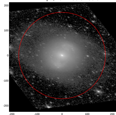
LEDA: pa,inc= 159.3 55.5
