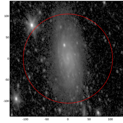
LEDA: pa,inc= 999.0 52.6
