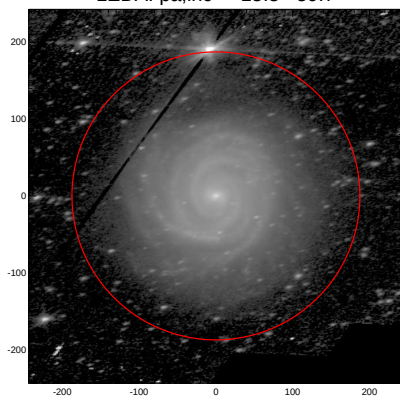
LEDA: pa,inc= 15.3 59.7
