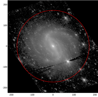
LEDA: pa,inc= 140.0 47.7
