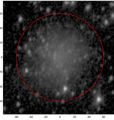
LEDA: pa,inc= 80.0 45.6
