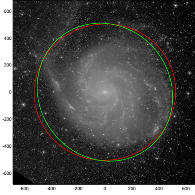
NGC5457
