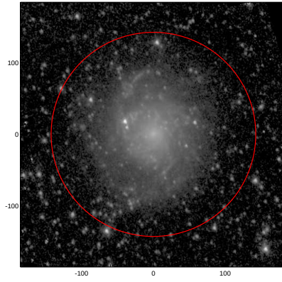
LEDA: pa,inc= 107.0 32.5
