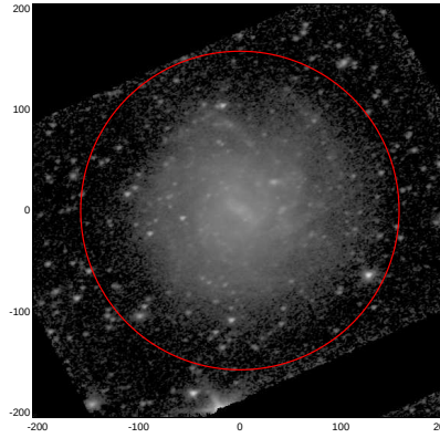
LEDA: pa,inc= 18.2 43.7
