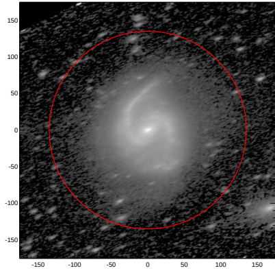
LEDA: pa,inc= 21.4 66.3
