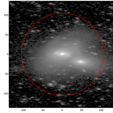
LEDA: pa,inc= 178.7 64.7
