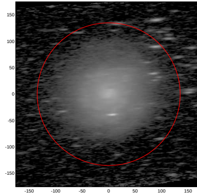
LEDA: pa,inc= 4.0 77.4
