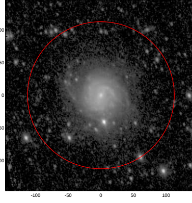
LEDA: pa,inc= 110.9 40.8
