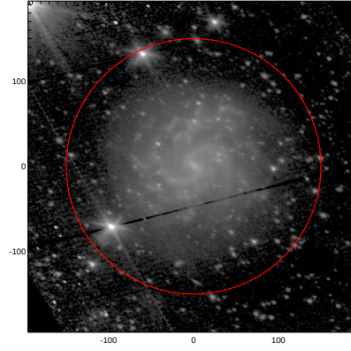
LEDA: pa,inc= 156.9 41.6
