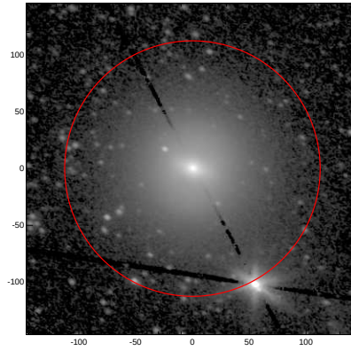
LEDA: pa,inc= 154.3 39.4
