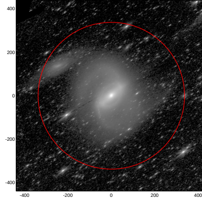
LEDA: pa,inc= 35.0 67.2
