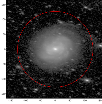
LEDA: pa,inc= 168.3 60.2
