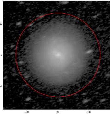
LEDA: pa,inc= 22.9 61.2
