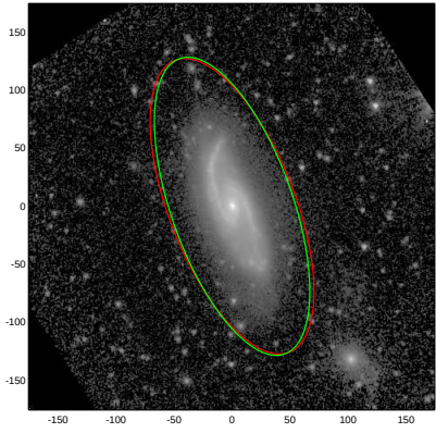
NGC5899
