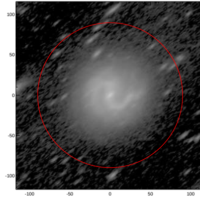
LEDA: pa,inc= 39.1 69.9
