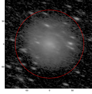
LEDA: pa,inc= 160.2 65.7
