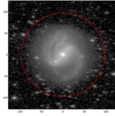
LEDA: pa,inc= 177.7 48.1
