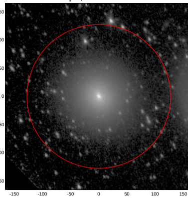
LEDA: pa,inc= 112.7 46.0
