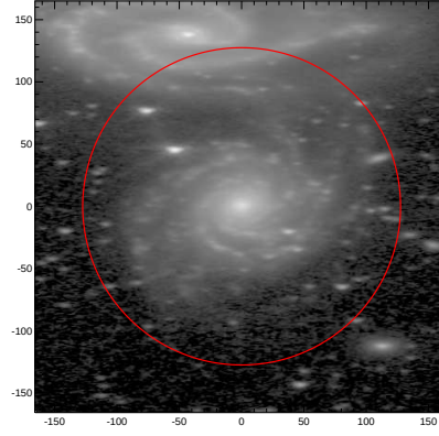
LEDA: pa,inc= 0.5 66.7
