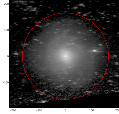
LEDA: pa,inc= 1.6 68.0
