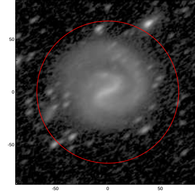
LEDA: pa,inc= 38.1 59.8
