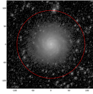
LEDA: pa,inc= 59.0 43.4
