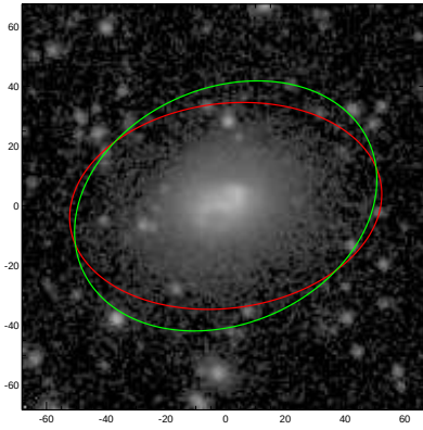
NGC5744
