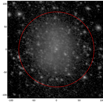
LEDA: pa,inc= 154.8 32.5
