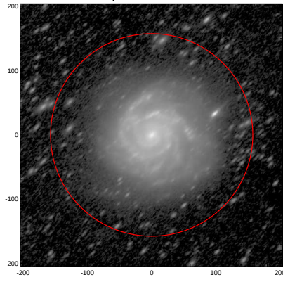
LEDA: pa,inc= 45.2 63.4
