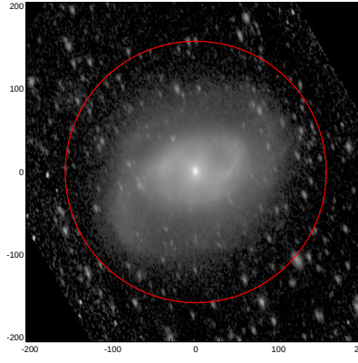
LEDA: pa,inc= 105.8 58.9
