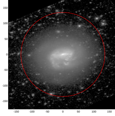
LEDA: pa,inc= 11.0 46.5
