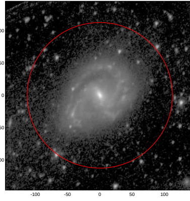
LEDA: pa,inc= 65.0 39.2
