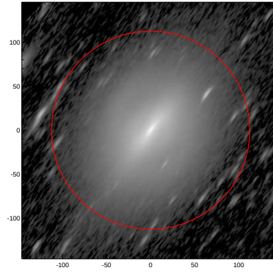
LEDA: pa,inc= 55.0 76.5
