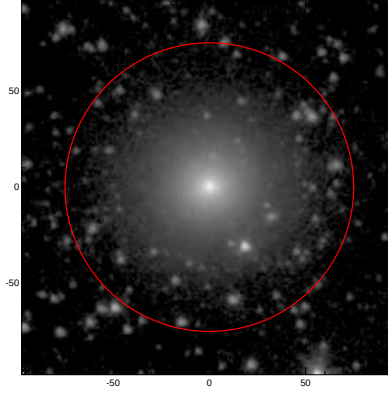
LEDA: pa,inc= 999.0 18.9
