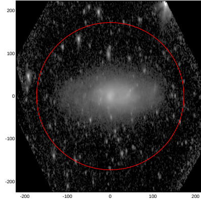
LEDA: pa,inc= 91.6 64.1
