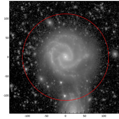
LEDA: pa,inc= 999.0 24.8
