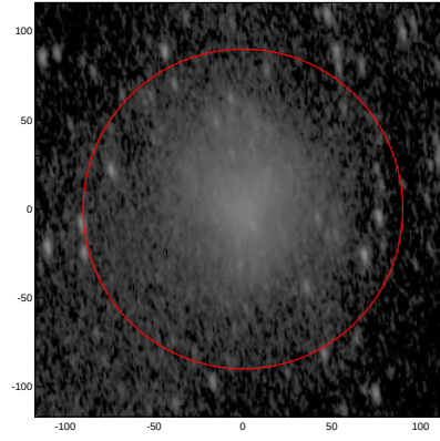
LEDA: pa,inc= 98.5 63.9
