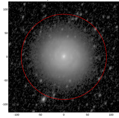
LEDA: pa,inc= 64.8 51.6
