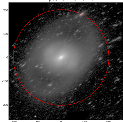
LEDA: pa,inc= 34.5 67.1
