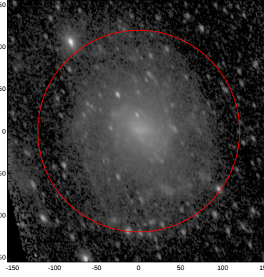
LEDA: pa,inc= 116.7 51.5
