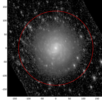
LEDA: pa,inc= 106.8 49.4
