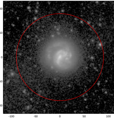
LEDA: pa,inc= 999.0 10.3
