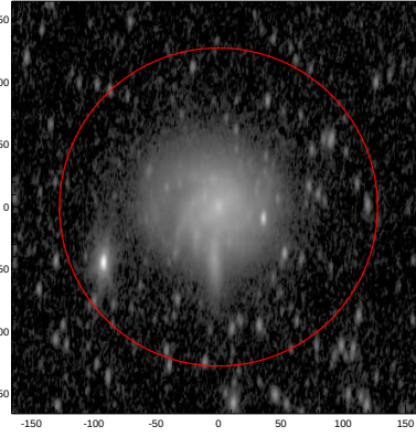
LEDA: pa,inc= 86.6 65.8
