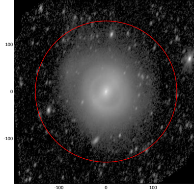
LEDA: pa,inc= 70.6 59.0
