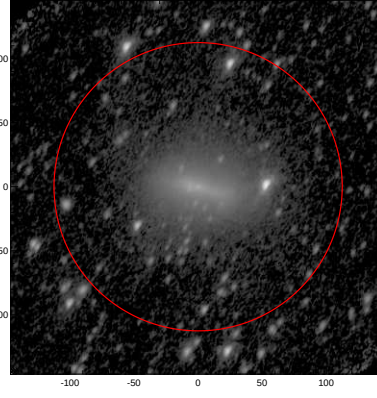
LEDA: pa,inc= 60.3 55.4
