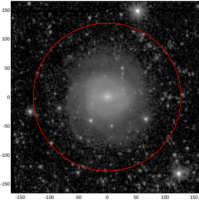
LEDA: pa,inc= 999.0 16.8
