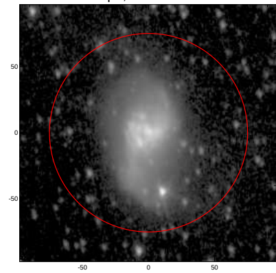
LEDA: pa,inc= 999.0 42.3
