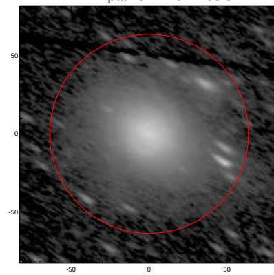
LEDA: pa,inc= 149.7 68.8
