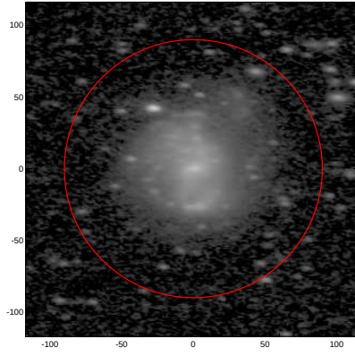
LEDA: pa,inc= 174.0 59.6
