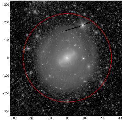
LEDA: pa,inc= 999.0 20.7
