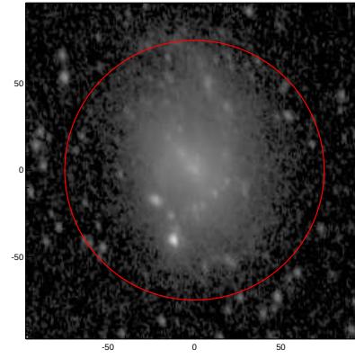
LEDA: pa,inc= 999.0 47.0
