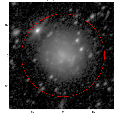
LEDA: pa,inc= 48.5 48.4
