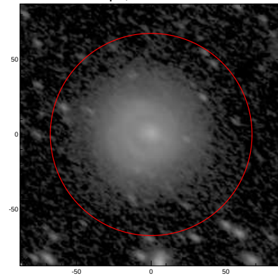
LEDA: pa,inc= 145.7 58.2
