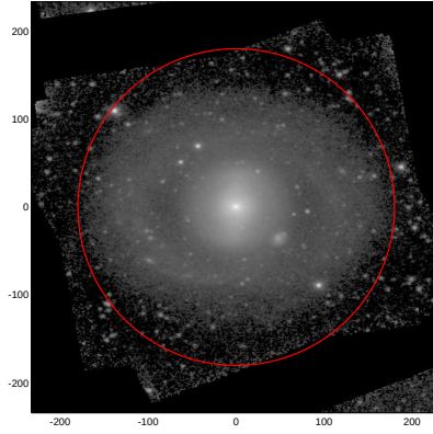
LEDA: pa,inc= 3.5 36.9
