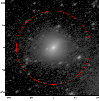
LEDA: pa,inc= 30.9 51.2
