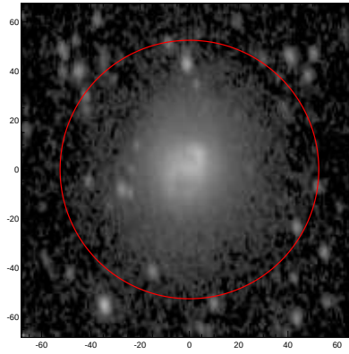
LEDA: pa,inc= 97.4 49.3
