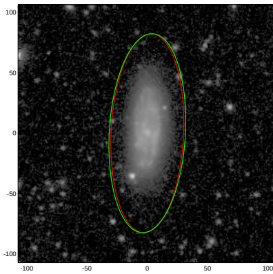
NGC5708
