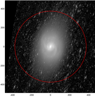
LEDA: pa,inc= 71.6 71.6
