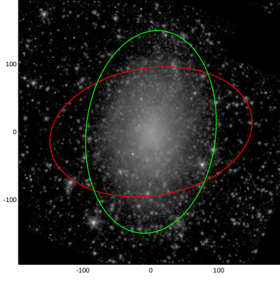
NGC5204
