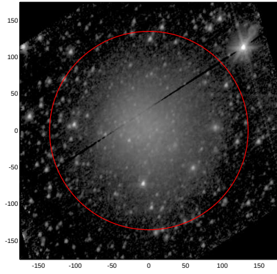
LEDA: pa,inc= 65.1 42.3
