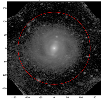
LEDA: pa,inc= 180.0 42.6
