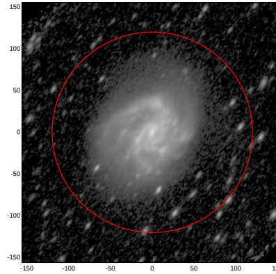
LEDA: pa,inc= 53.5 61.6
