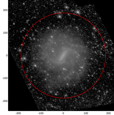
LEDA: pa,inc= 147.7 41.4
