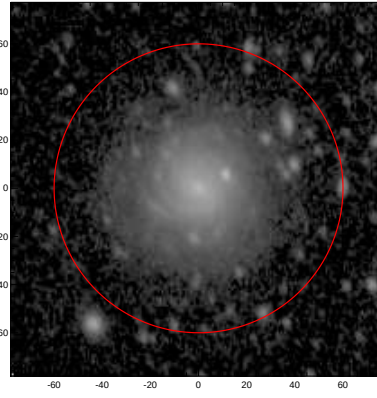
LEDA: pa,inc= 98.4 41.0
