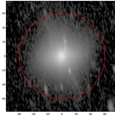
LEDA: pa,inc= 100.2 69.9
