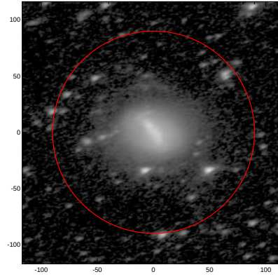
LEDA: pa,inc= 19.6 57.2
