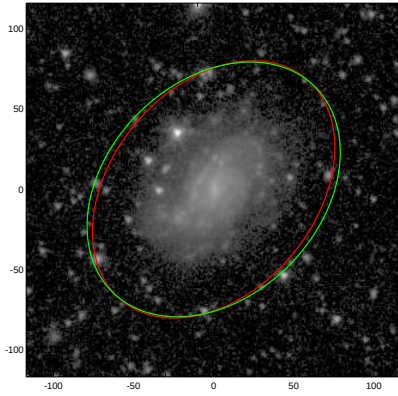
NGC5105
