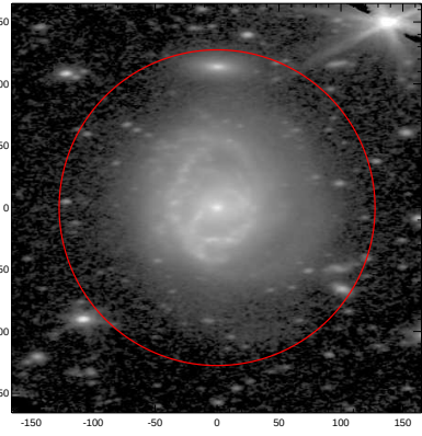
LEDA: pa,inc= 1.4 58.5
