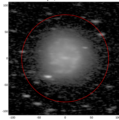
LEDA: pa,inc= 177.5 68.6
