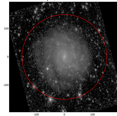
LEDA: pa,inc= 999.0 38.6
