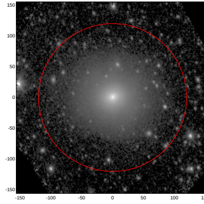
LEDA: pa,inc= 99.3 34.3
