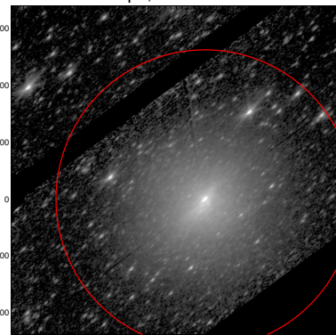
LEDA: pa,inc= 43.5 64.9
