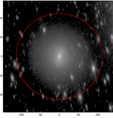
LEDA: pa,inc= 97.3 64.2
