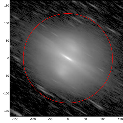
LEDA: pa,inc= 148.8 81.5
