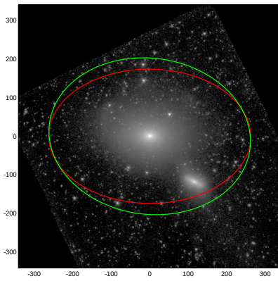
NGC5576
