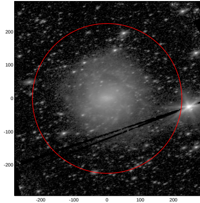
LEDA: pa,inc= 19.0 58.0
