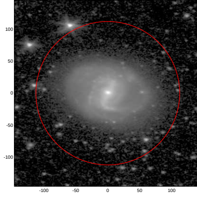
LEDA: pa,inc= 177.6 48.3
