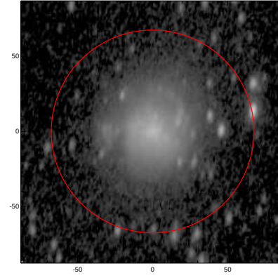
LEDA: pa,inc= 82.3 57.9
