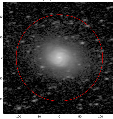
LEDA: pa,inc= 5.9 59.2
