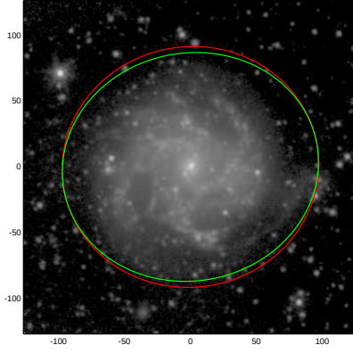
NGC5468
