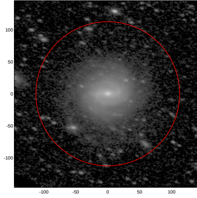
LEDA: pa,inc= 165.8 53.8
