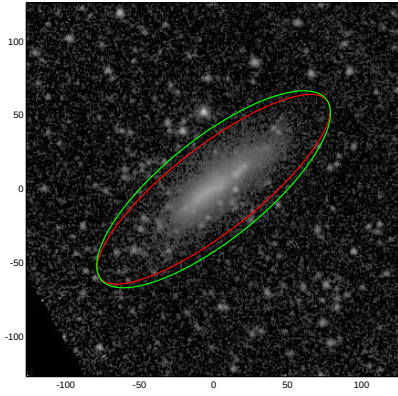
NGC5107
