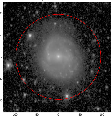
LEDA: pa,inc= 84.7 34.7
