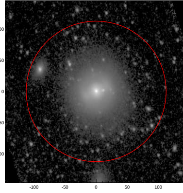
LEDA: pa,inc= 999.0 35.4
