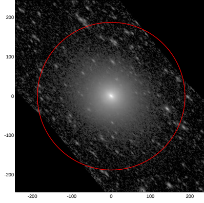
LEDA: pa,inc= 135.3 61.8
