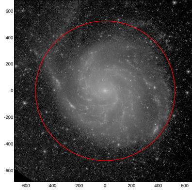
LEDA: pa,inc= 999.0 15.9
