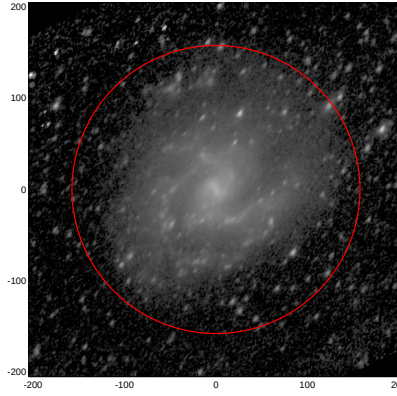
LEDA: pa,inc= 54.8 55.3
