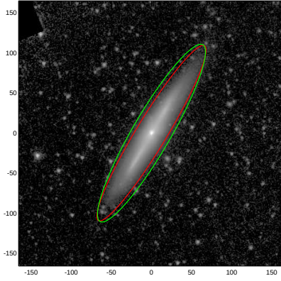
NGC5073
