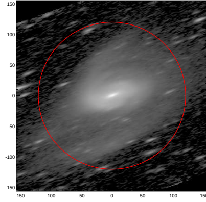
LEDA: pa,inc= 20.6 77.0
