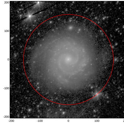
LEDA: pa,inc= 41.7 36.7
