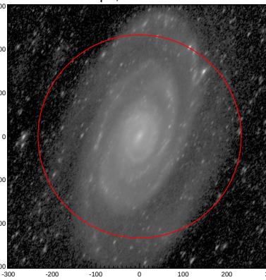
LEDA: pa,inc= 58.0 64.1
