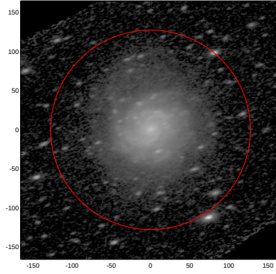
LEDA: pa,inc= 18.0 59.8
