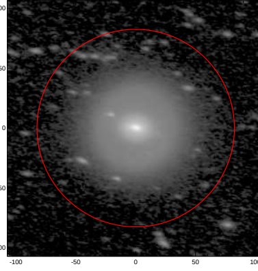
LEDA: pa,inc= 168.0 58.4
