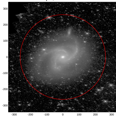
LEDA: pa,inc= 171.1 54.9
