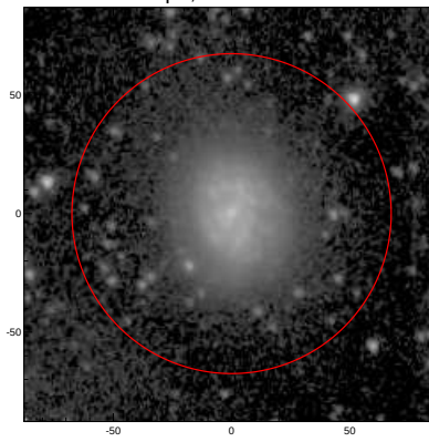
LEDA: pa,inc= 999.0 21.7
