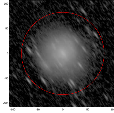
LEDA: pa,inc= 125.9 74.0
