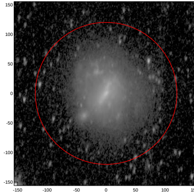
LEDA: pa,inc= 83.2 57.3
