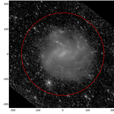
LEDA: pa,inc= 129.2 52.2
