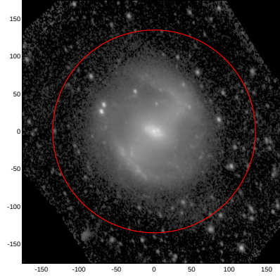
LEDA: pa,inc= 107.0 40.7
