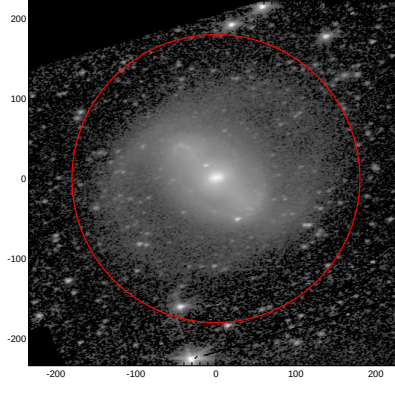
LEDA: pa,inc= 14.5 54.3
