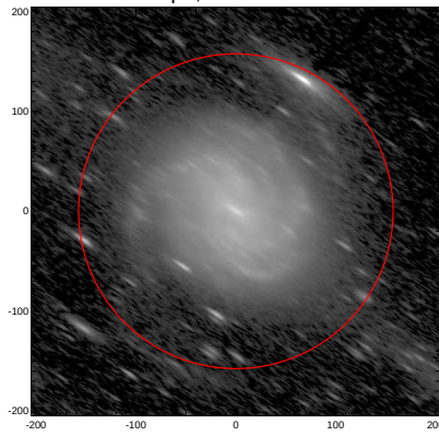
LEDA: pa,inc= 146.0 75.9
