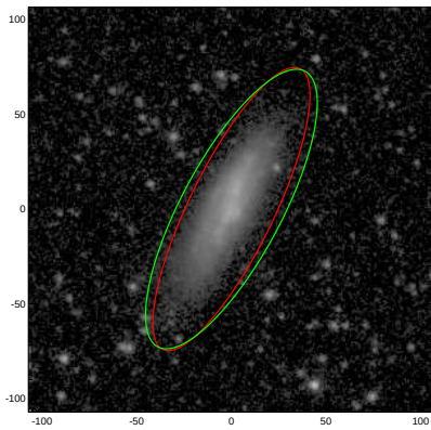
NGC5109
