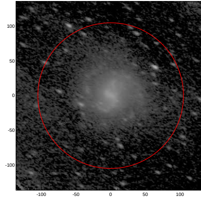
LEDA: pa,inc= 153.8 60.7
