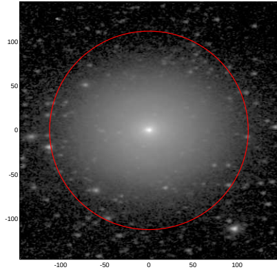
LEDA: pa,inc= 3.8 48.6
