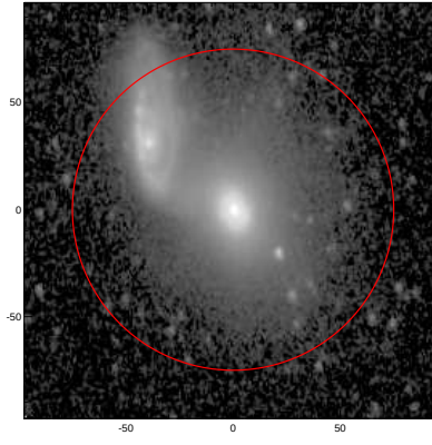
LEDA: pa,inc= 999.0 40.2
