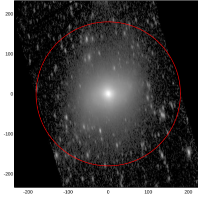
LEDA: pa,inc= 97.8 65.4
