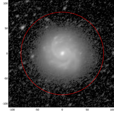
LEDA: pa,inc= 42.7 54.4
