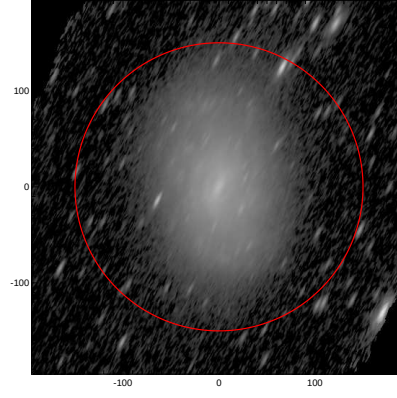
LEDA: pa,inc= 62.6 75.3
