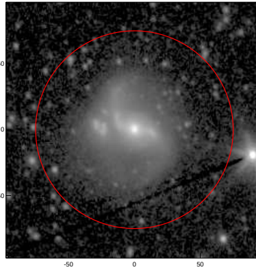
LEDA: pa,inc= 999.0 25.1
