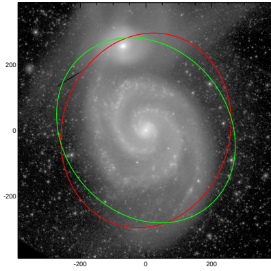
NGC5194
