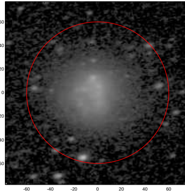
LEDA: pa,inc= 9.2 48.2
