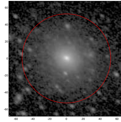
LEDA: pa,inc= 144.0 44.0
