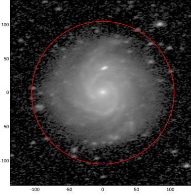
LEDA: pa,inc= 9.8 56.9
