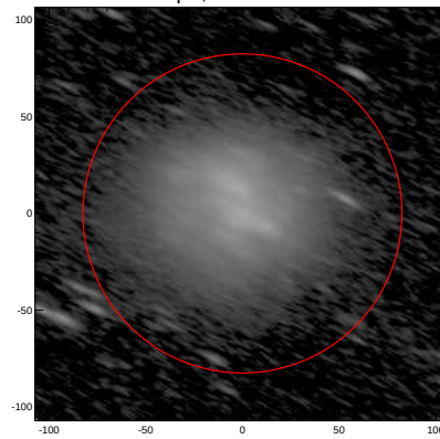
LEDA: pa,inc= 153.9 74.3
