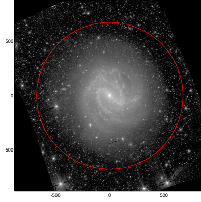
LEDA: pa,inc= 999.0 13.9
