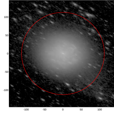
LEDA: pa,inc= 148.4 65.5
