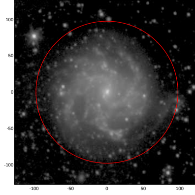
LEDA: pa,inc= 999.0 20.7
