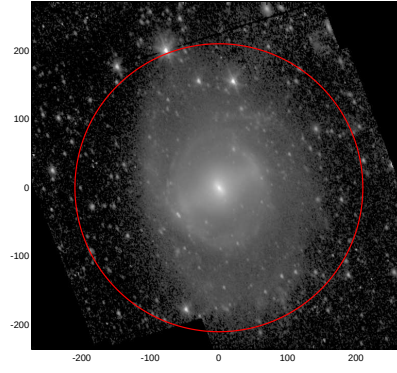
LEDA: pa,inc= 114.4 44.9
