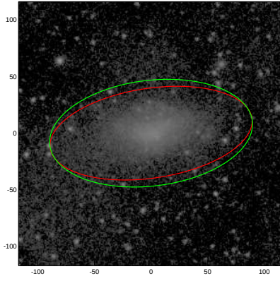
NGC5608
