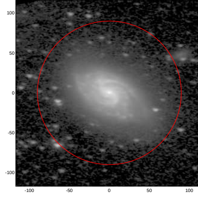
LEDA: pa,inc= 175.3 55.1
