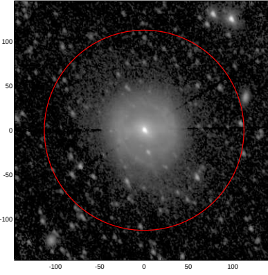
LEDA: pa,inc= 119.6 42.9
