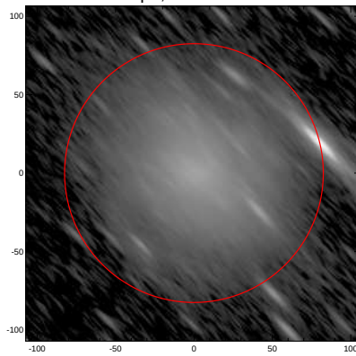
LEDA: pa,inc= 133.8 79.0
