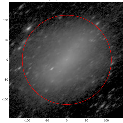
LEDA: pa,inc= 40.0 65.1
