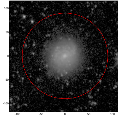
LEDA: pa,inc= 999.0 21.4
