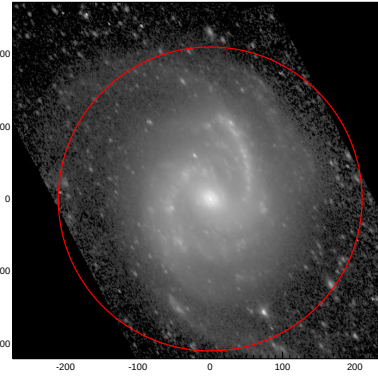
LEDA: pa,inc= 125.0 54.2
