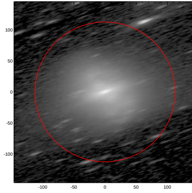
LEDA: pa,inc= 18.7 78.5
