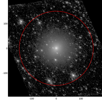
LEDA: pa,inc= 140.0 43.0
