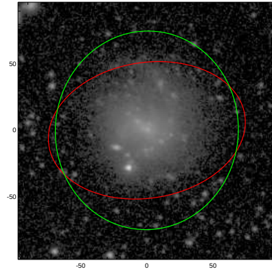
NGC5693
