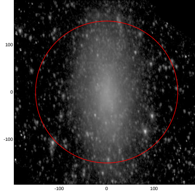
LEDA: pa,inc= 999.0 51.1
