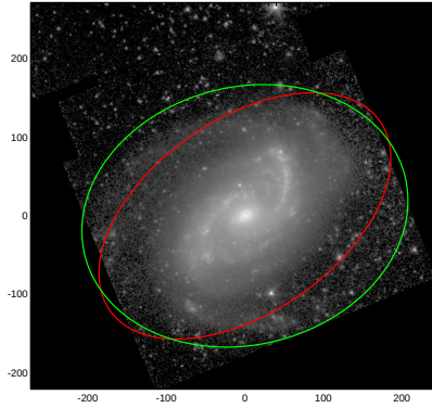
NGC5248
