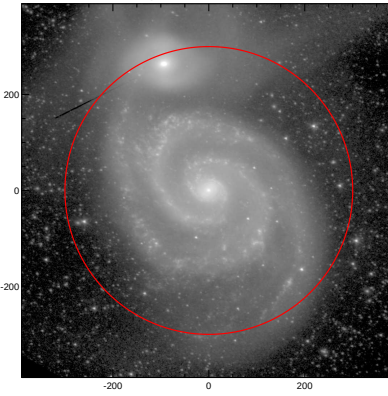
LEDA: pa,inc= 163.0 31.7
