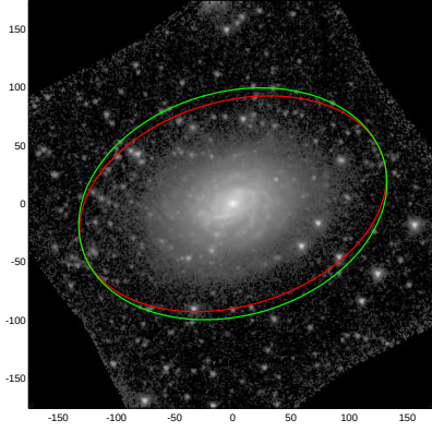
NGC5962
