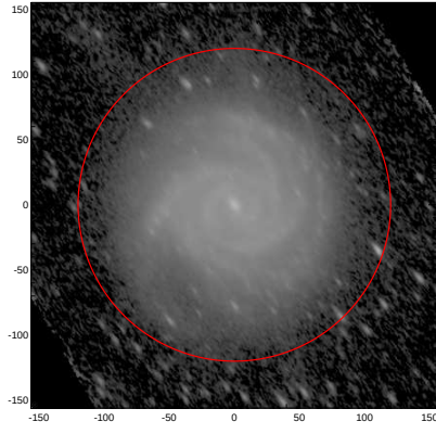
LEDA: pa,inc= 126.8 64.6
