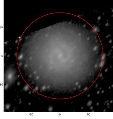
LEDA: pa,inc= 57.3 46.4
