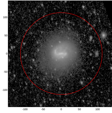
LEDA: pa,inc= 99.5 41.1
