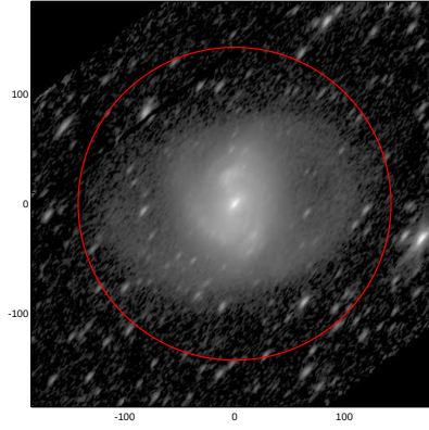
LEDA: pa,inc= 51.8 67.5
