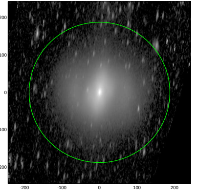
S4G: pa,inc= 84.1 74.4
