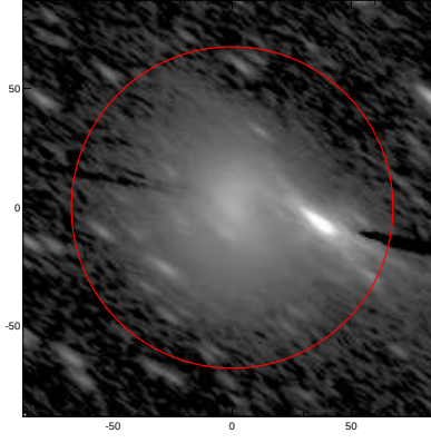
LEDA: pa,inc= 144.8 71.6
