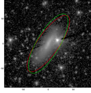
NGC5916A
