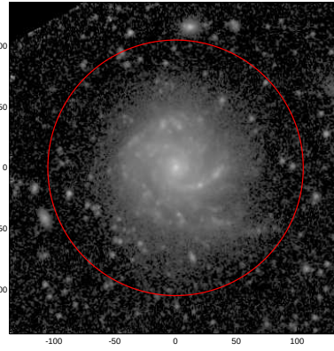
LEDA: pa,inc= 999.0 23.0
