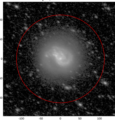
LEDA: pa,inc= 150.6 51.6
