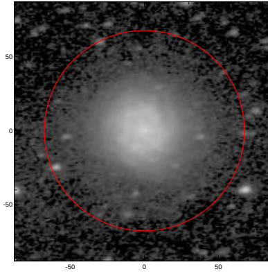
LEDA: pa,inc= 10.3 48.5
