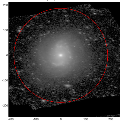
LEDA: pa,inc= 172.5 57.3
