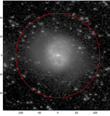
LEDA: pa,inc= 177.5 40.4
