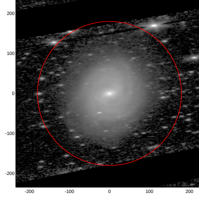
LEDA: pa,inc= 6.5 68.3
