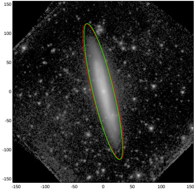
NGC5894
