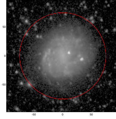
LEDA: pa,inc= 999.0 22.7
