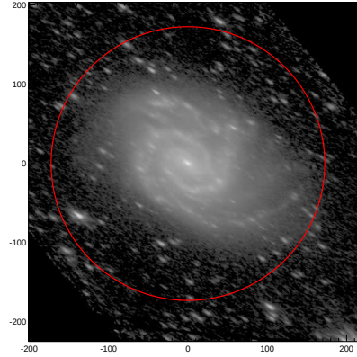
LEDA: pa,inc= 149.2 66.5
