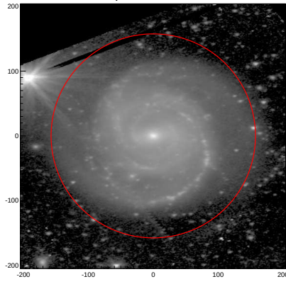
LEDA: pa,inc= 5.9 51.9
