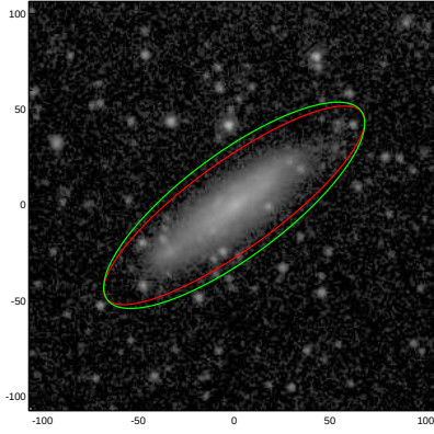
NGC5425
