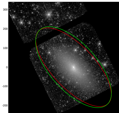
NGC5253
