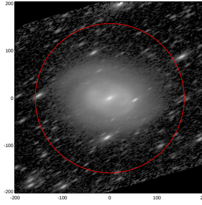
LEDA: pa,inc= 29.1 70.3
