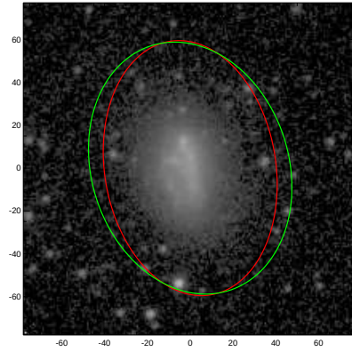
NGC5624
