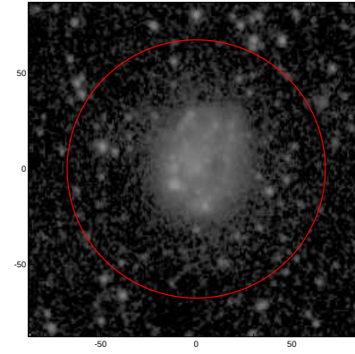
LEDA: pa,inc= 92.0 26.7
