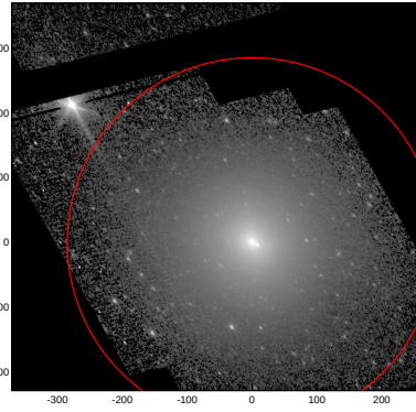
LEDA: pa,inc= 132.5 48.6
