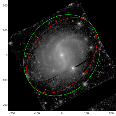
NGC5921
