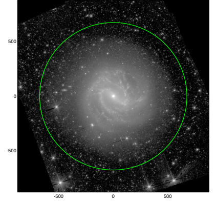
S4G: pa,inc= 4.1 19.2
