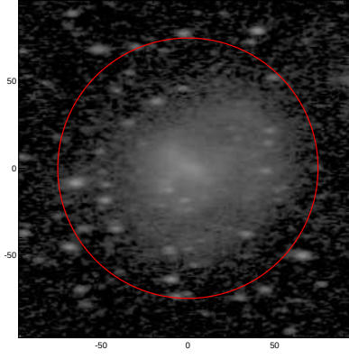
LEDA: pa,inc= 0.9 59.5
