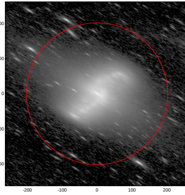
LEDA: pa,inc= 148.9 76.8
