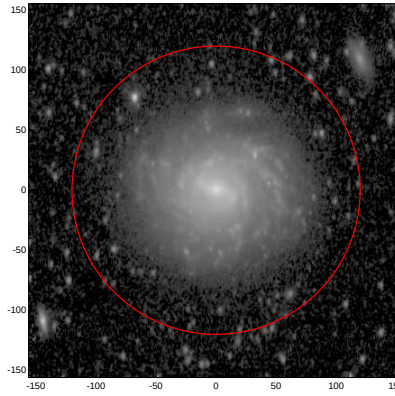
LEDA: pa,inc= 87.8 46.4
