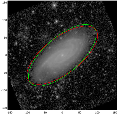
NGC5254
