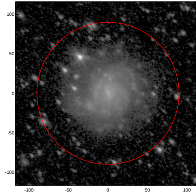
LEDA: pa,inc= 140.2 44.9
