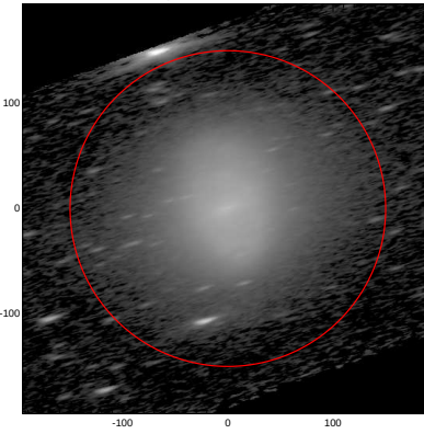
LEDA: pa,inc= 16.0 76.4
