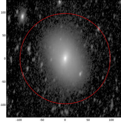
LEDA: pa,inc= 79.6 60.6
