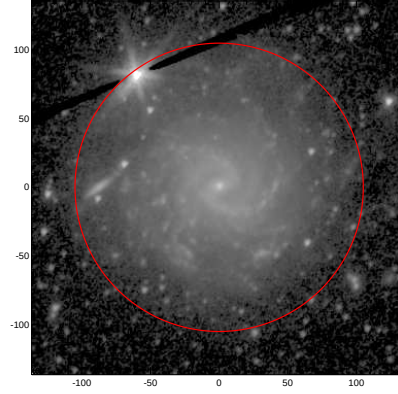
LEDA: pa,inc= 57.7 32.5
