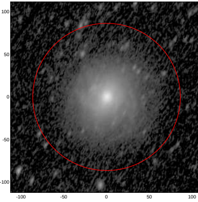
LEDA: pa,inc= 65.3 60.2
