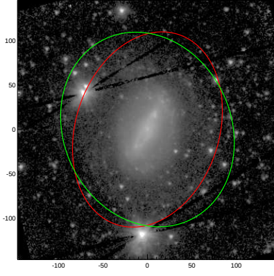
NGC6012
