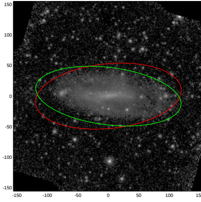
NGC6255
