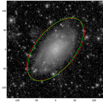
NGC6106
