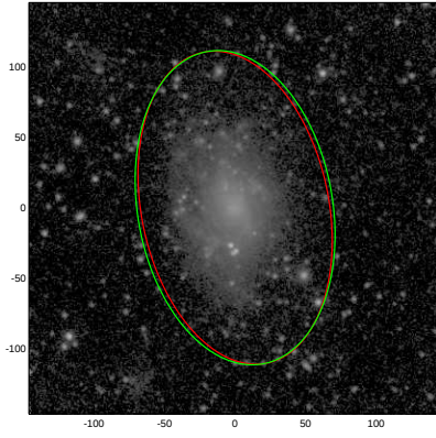
NGC6236
