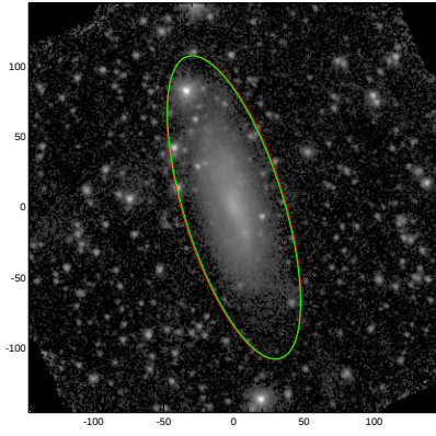
NGC6395
