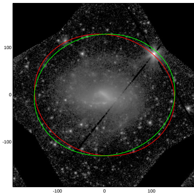
NGC6140
