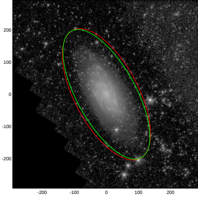
NGC6015
