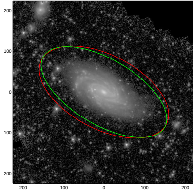
NGC6070
