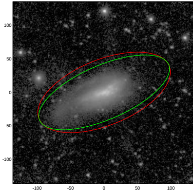
NGC6239
