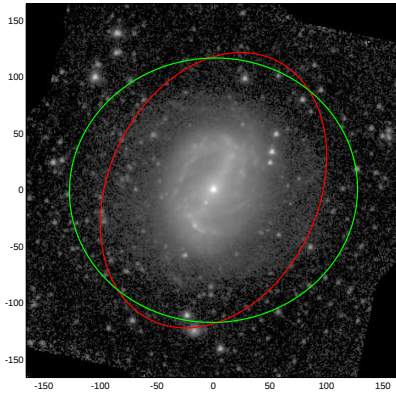
NGC6217
