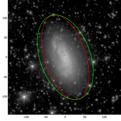
NGC6207
