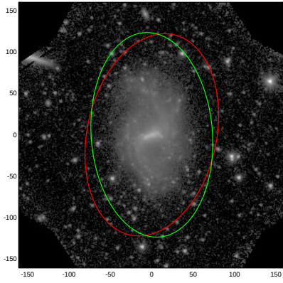
NGC6339
