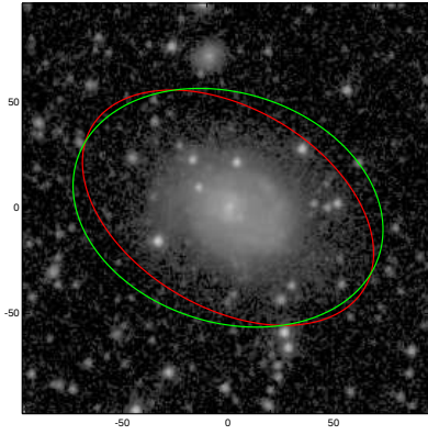
NGC6889
