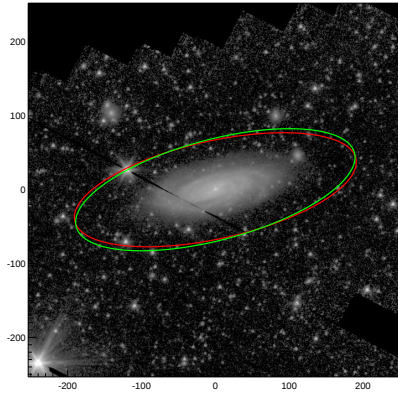
NGC6887
