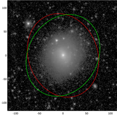
NGC6014
