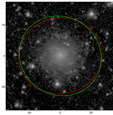
NGC6902B
