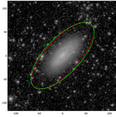
NGC7191
