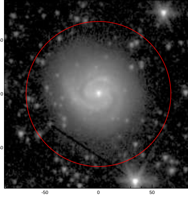
LEDA: pa,inc= 999.0 23.9
