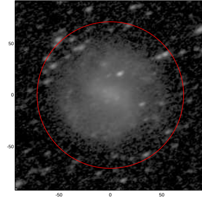
LEDA: pa,inc= 26.0 50.0
