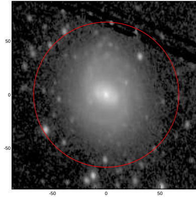
LEDA: pa,inc= 999.0 42.3
