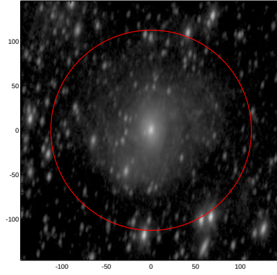
LEDA: pa,inc= 81.4 59.7
