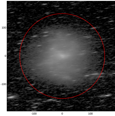
LEDA: pa,inc= 8.5 76.8
