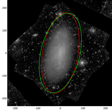
NGC7713
