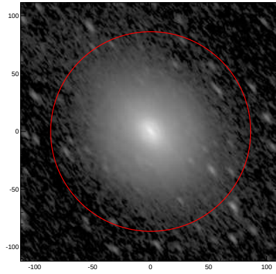
LEDA: pa,inc= 129.6 66.9
