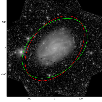
NGC7689
