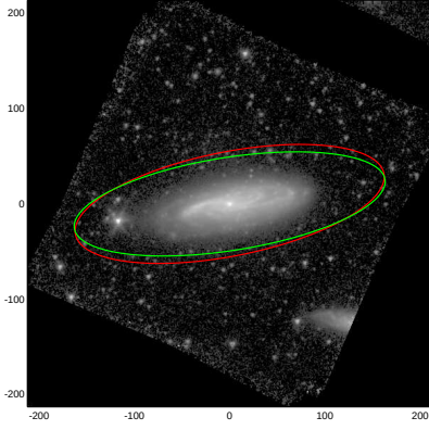
NGC7541
