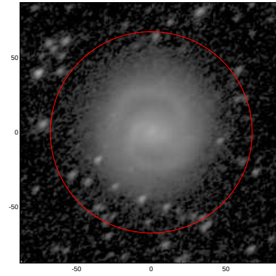
LEDA: pa,inc= 37.8 47.1
