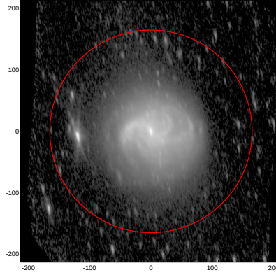
LEDA: pa,inc= 101.2 70.7
