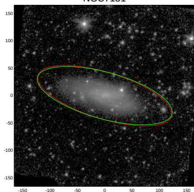
NGC7151
