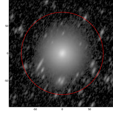
LEDA: pa,inc= 64.6 62.4
