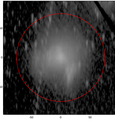
LEDA: pa,inc= 90.8 71.5
