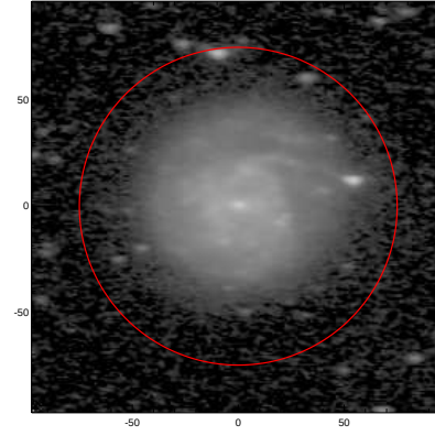
LEDA: pa,inc= 175.5 61.0
