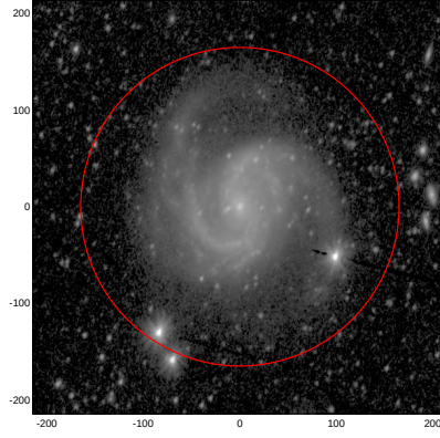
LEDA: pa,inc= 75.3 42.6
