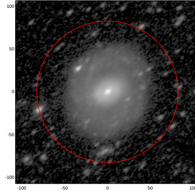
LEDA: pa,inc= 38.1 53.0
