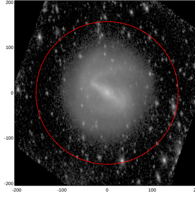
LEDA: pa,inc= 100.3 53.0
