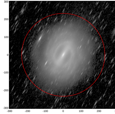
LEDA: pa,inc= 61.4 77.8
