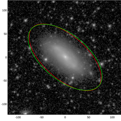
NGC7179
