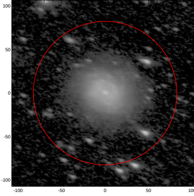
LEDA: pa,inc= 158.0 61.0
