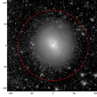
LEDA: pa,inc= 999.0 13.9
