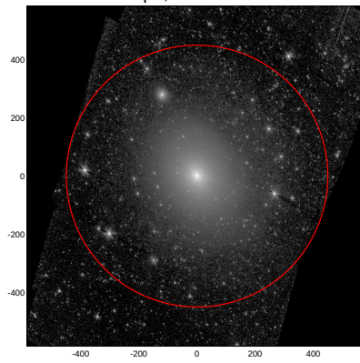
LEDA: pa,inc= 121.0 36.5
