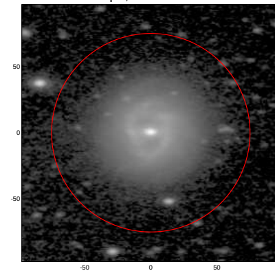
LEDA: pa,inc= 179.5 56.2
