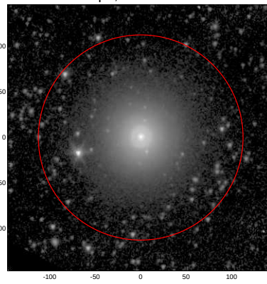
LEDA: pa,inc= 999.0 16.4
