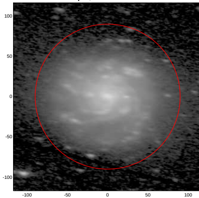
LEDA: pa,inc= 170.6 67.1
