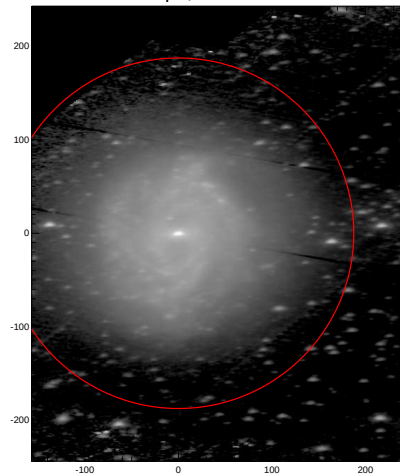
LEDA: pa,inc= 2.9 66.0
