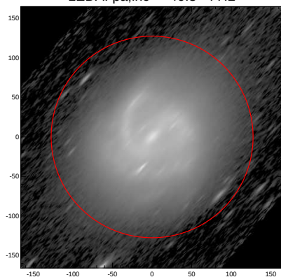
LEDA: pa,inc= 46.3 77.2
