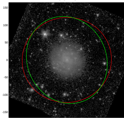
NGC7437
