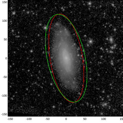
NGC7162
