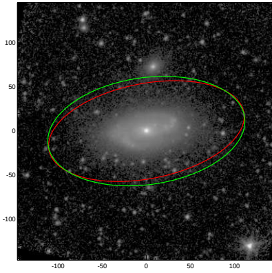
NGC7163
