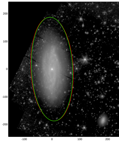
NGC7314
