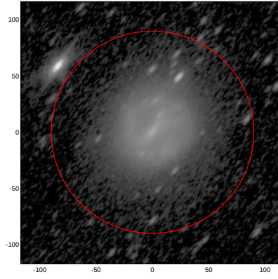
LEDA: pa,inc= 48.8 65.0
