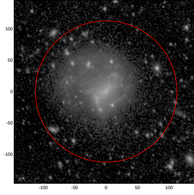
LEDA: pa,inc= 115.5 31.0
