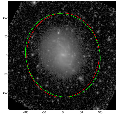
NGC7070
