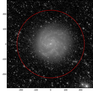
LEDA: pa,inc= 138.7 39.1
