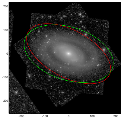
NGC7098
