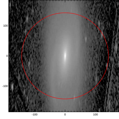
LEDA: pa,inc= 88.3 77.4
