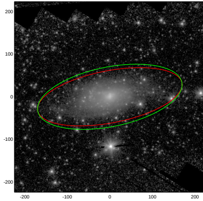
NGC7059
