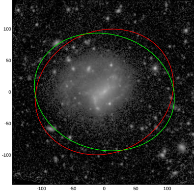
NGC7154
