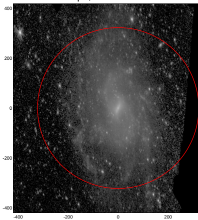
LEDA: pa,inc= 999.0 57.5
