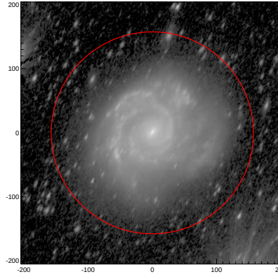
LEDA: pa,inc= 63.2 62.5
