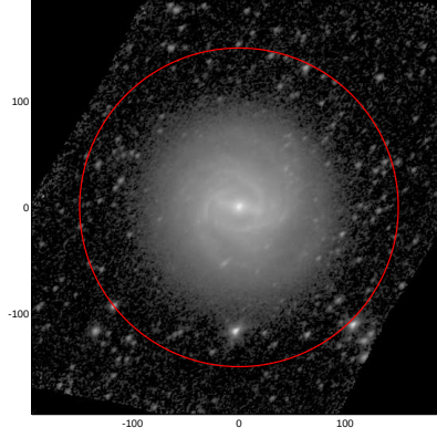
LEDA: pa,inc= 41.5 45.1
