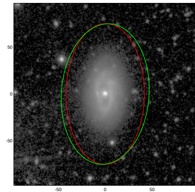
NGC7378
