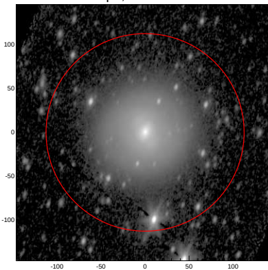
LEDA: pa,inc= 76.7 51.4
