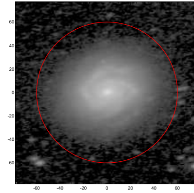
LEDA: pa,inc= 6.3 58.5
