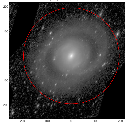
LEDA: pa,inc= 61.9 59.2
