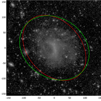
NGC7162A
