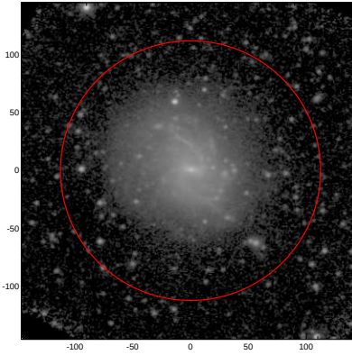
LEDA: pa,inc= 178.0 30.3
