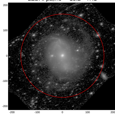
LEDA: pa,inc= 18.2 47.1
