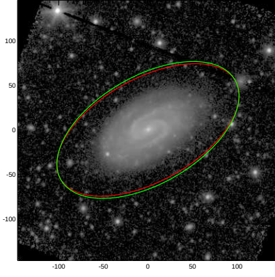
NGC7171
