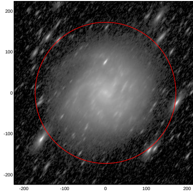
LEDA: pa,inc= 55.2 70.8
