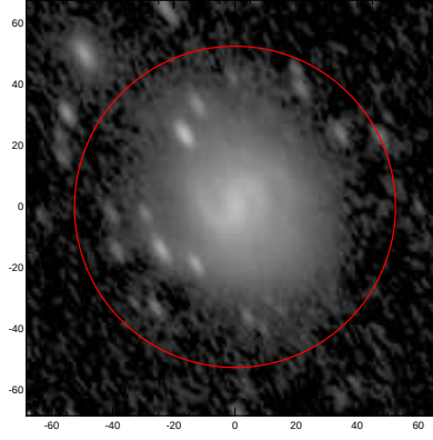
LEDA: pa,inc= 121.7 60.6
