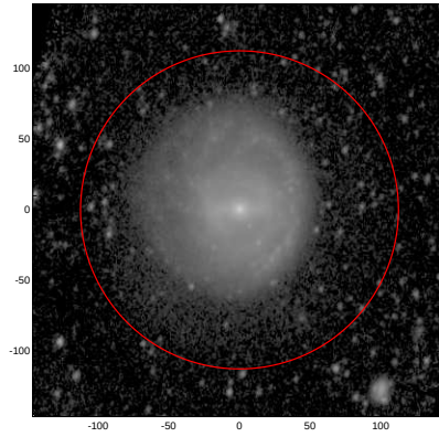
LEDA: pa,inc= 84.6 35.1
