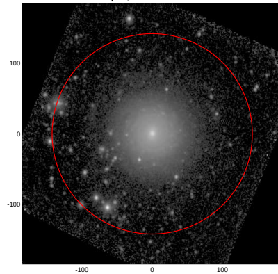
LEDA: pa,inc= 999.0 23.3
