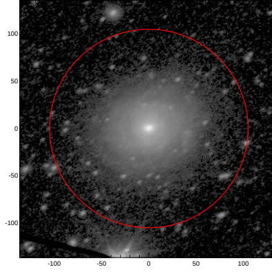
LEDA: pa,inc= 30.4 46.2
