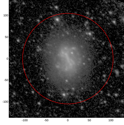
LEDA: pa,inc= 133.8 42.2
