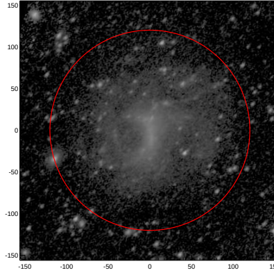
LEDA: pa,inc= 41.9 43.7
