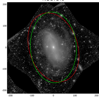
NGC7140
