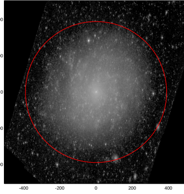
LEDA: pa,inc= 89.5 54.5
