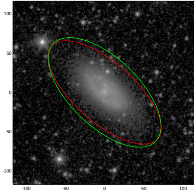
NGC7188
