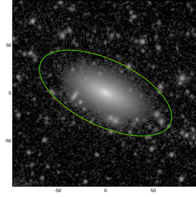
NGC7180
