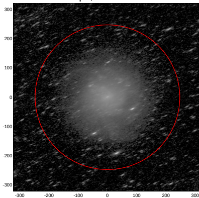
LEDA: pa,inc= 22.4 70.0
