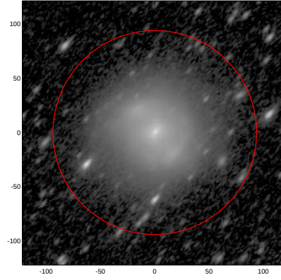
LEDA: pa,inc= 48.5 60.7
