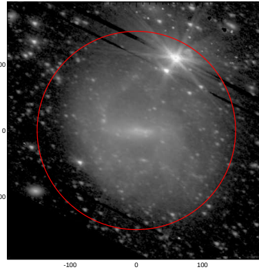
LEDA: pa,inc= 153.5 49.1
