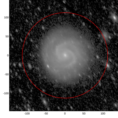
LEDA: pa,inc= 119.0 59.1
