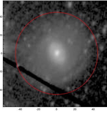
LEDA: pa,inc= 75.0 42.4
