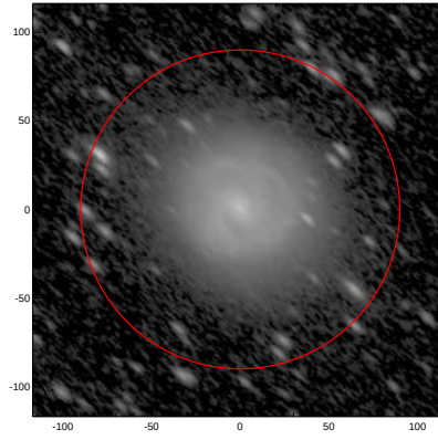
LEDA: pa,inc= 137.5 66.7
