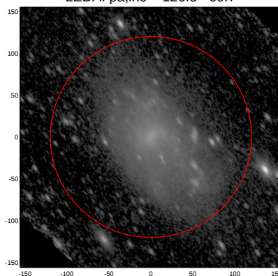
LEDA: pa,inc= 126.5 60.7
