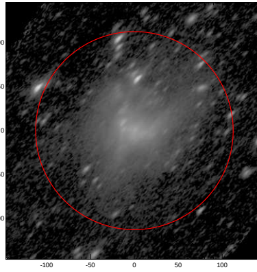
LEDA: pa,inc= 45.1 65.5
