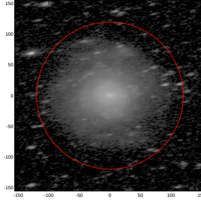
LEDA: pa,inc= 9.5 68.8
