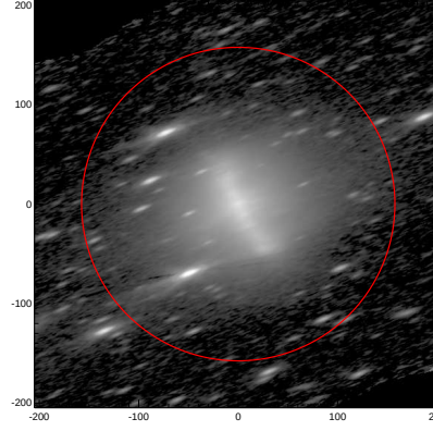
LEDA: pa,inc= 21.7 74.9
