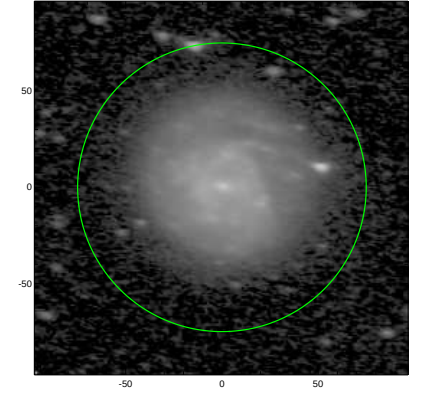
S4G: pa,inc= -9.0 60.2
