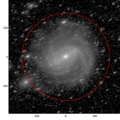
LEDA: pa,inc= 26.6 52.1
