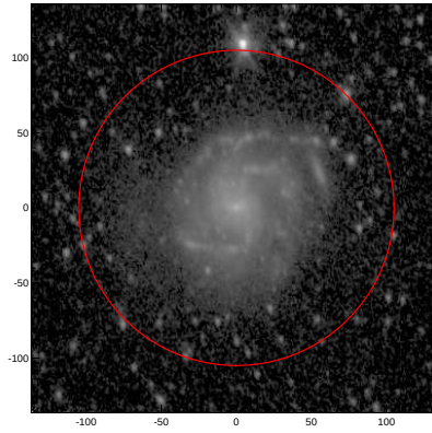
LEDA: pa,inc= 103.4 42.9
