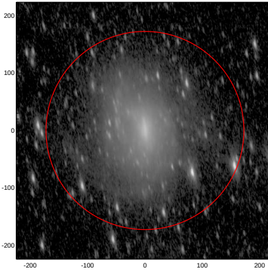
LEDA: pa,inc= 100.9 69.2
