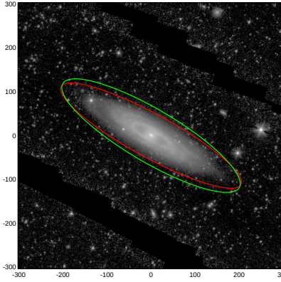
NGC7184
