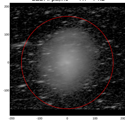
LEDA: pa,inc= 7.7 74.2
