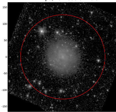
LEDA: pa,inc= 999.0 16.8
