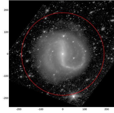
LEDA: pa,inc= 26.6 41.7
