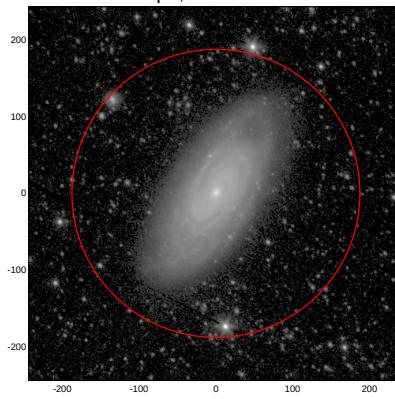
LEDA: pa,inc= 131.2 31.9
