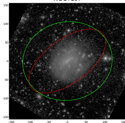
NGC7107
