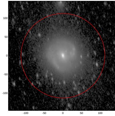
LEDA: pa,inc= 101.0 61.4
