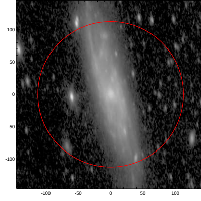
LEDA: pa,inc= 999.0 65.3
