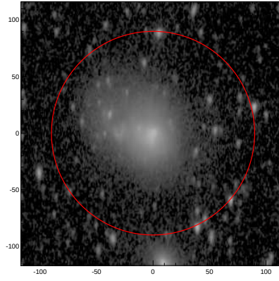
LEDA: pa,inc= 89.3 56.9
