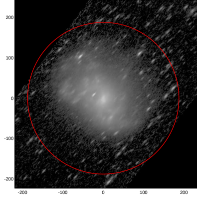
LEDA: pa,inc= 44.3 69.4
