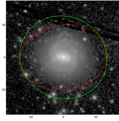
NGC7051
