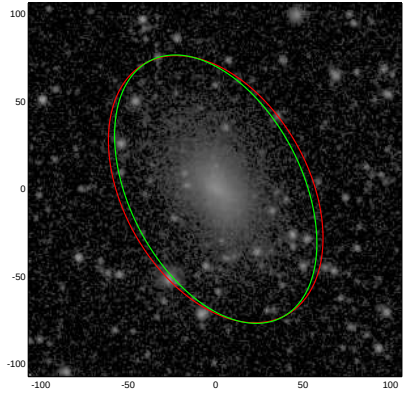
PGC042068
