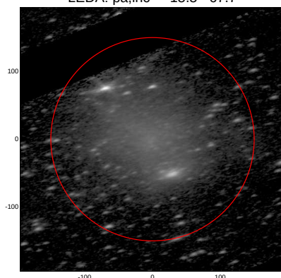
LEDA: pa,inc= 15.5 67.7
