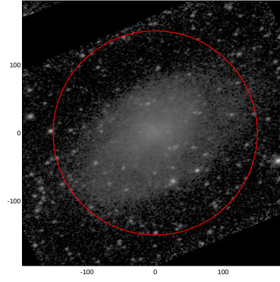
LEDA: pa,inc= 19.5 45.5
