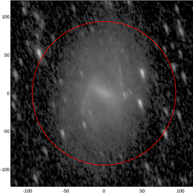
LEDA: pa,inc= 109.3 65.6
