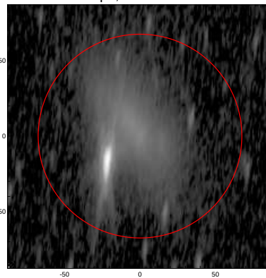
LEDA: pa,inc= 84.2 75.8
