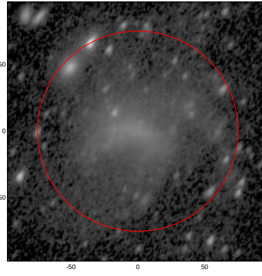
LEDA: pa,inc= 60.0 53.6
