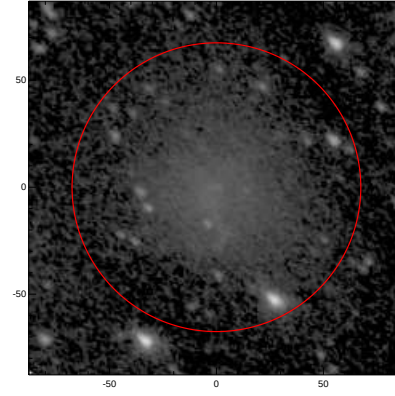
LEDA: pa,inc= 142.0 46.1
