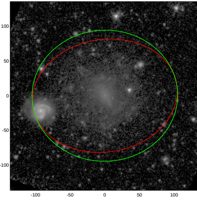
PGC006626
