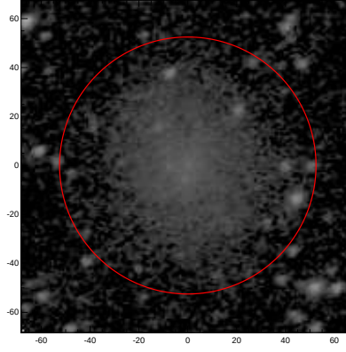
LEDA: pa,inc= 15.0 38.4
