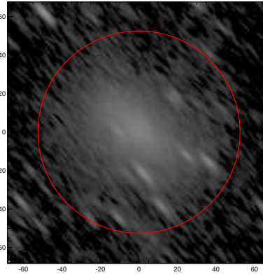
LEDA: pa,inc= 131.5 74.1
