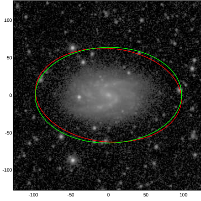
PGC069448
