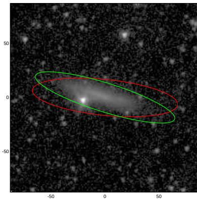
PGC003855
