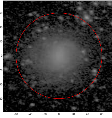
LEDA: pa,inc= 171.3 48.1
