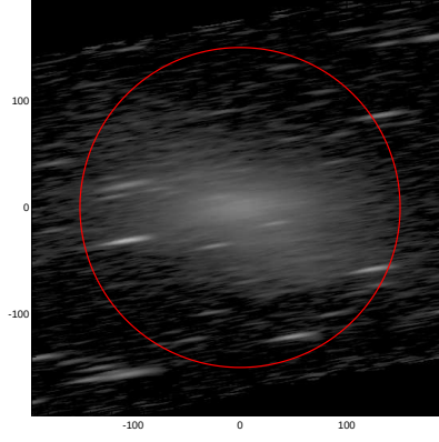
LEDA: pa,inc= 9.3 83.9
