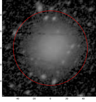
LEDA: pa,inc= 41.7 43.9
