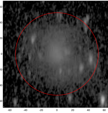
LEDA: pa,inc= 86.9 65.4
