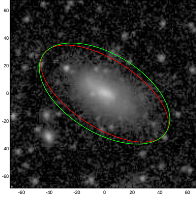
PGC011744
