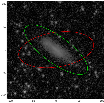
PGC072006
