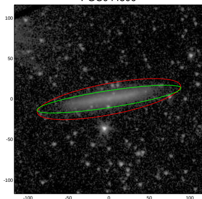
PGC044506
