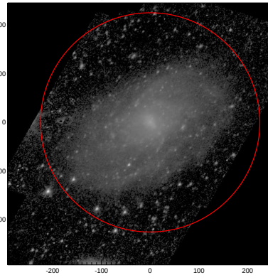
LEDA: pa,inc= 45.0 42.6
