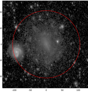
LEDA: pa,inc= 999.0 39.4
