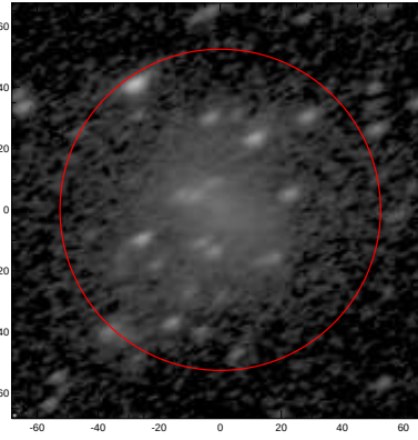
LEDA: pa,inc= 25.5 56.7
