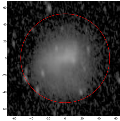
LEDA: pa,inc= 96.4 59.8
