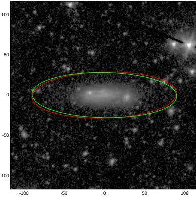
PGC009354
