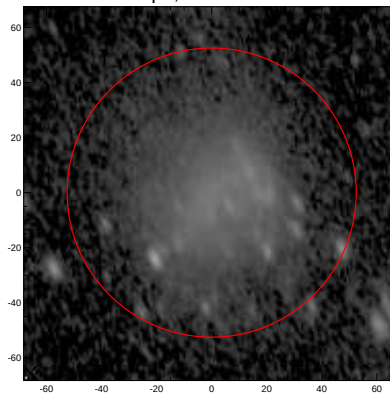
LEDA: pa,inc= 110.8 55.8
