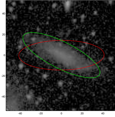
PGC006898
