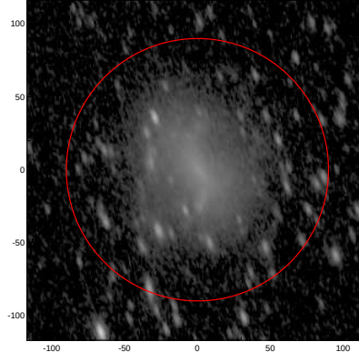
LEDA: pa,inc= 107.8 63.0
