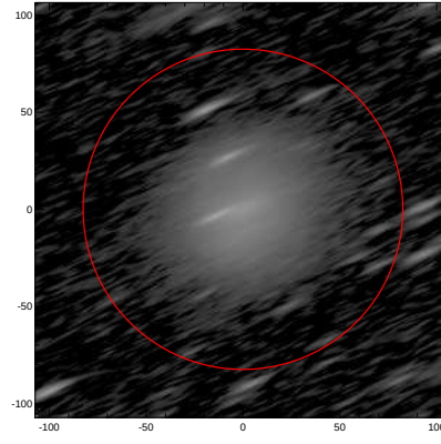
LEDA: pa,inc= 24.5 80.0
