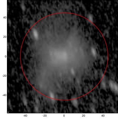
LEDA: pa,inc= 105.3 63.5
