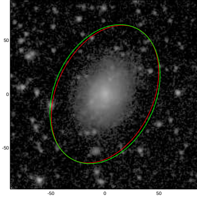
PGC052460
