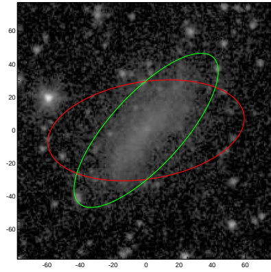
PGC043341
