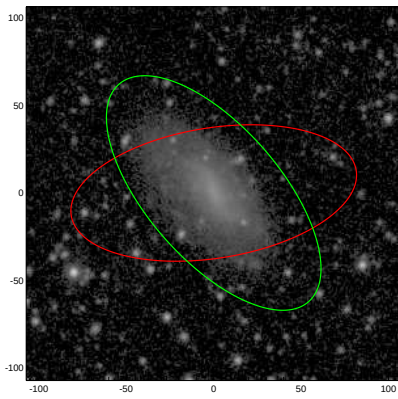
PGC06242
