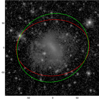
PGC012068
