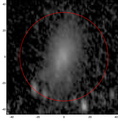
LEDA: pa,inc= 999.0 56.8
