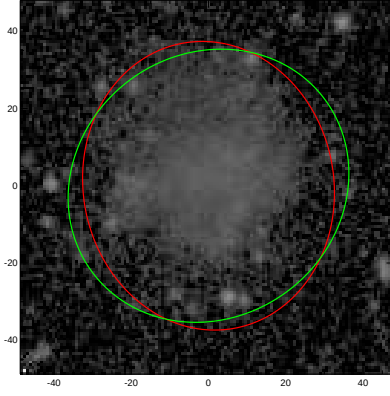
PGC069339
