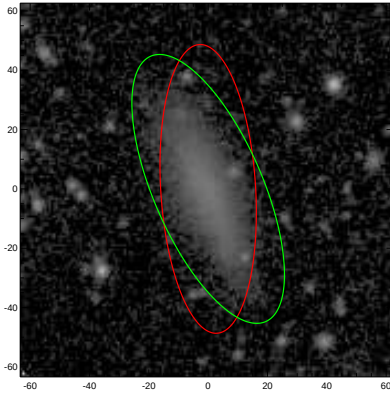
PGC003062
