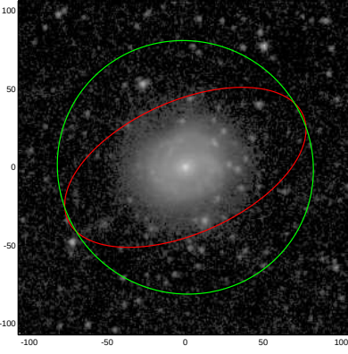
PGC012633
