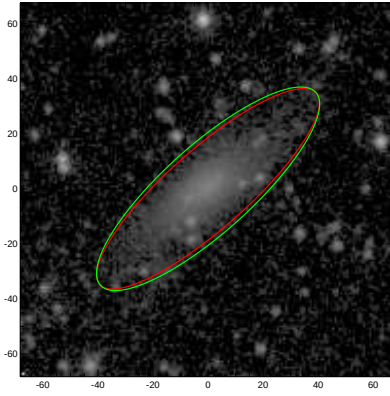
PGC069114
