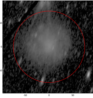
LEDA: pa,inc= 73.6 68.7
