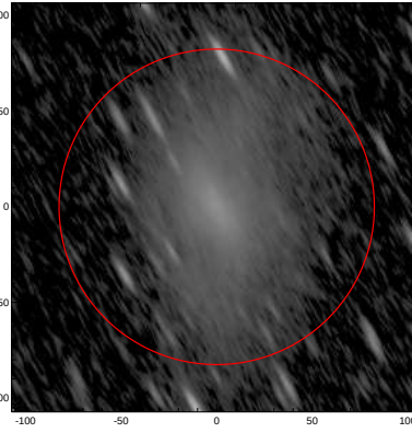
LEDA: pa,inc= 119.6 77.2
