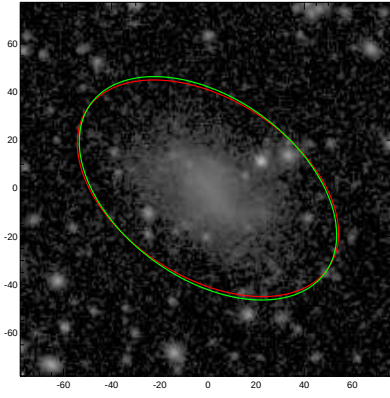
PGC035705
