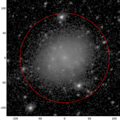
LEDA: pa,inc= 18.8 31.9
