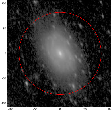
LEDA: pa,inc= 114.0 59.1
