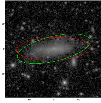
PGC037238
