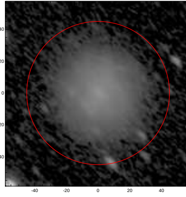
LEDA: pa,inc= 136.0 62.0
