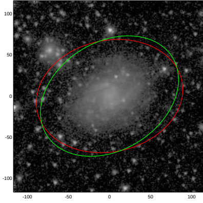
PGC052853
