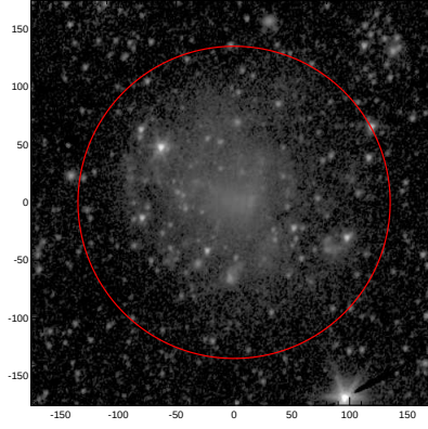
LEDA: pa,inc= 63.2 33.7
