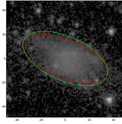
PGC006244
