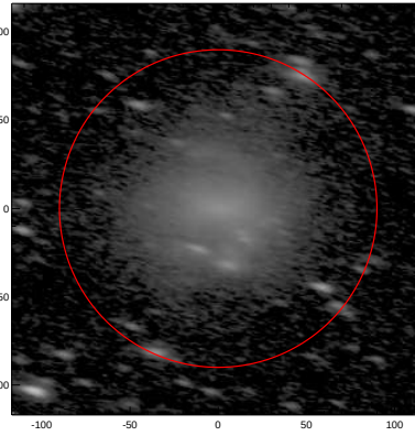
LEDA: pa,inc= 166.2 69.6
