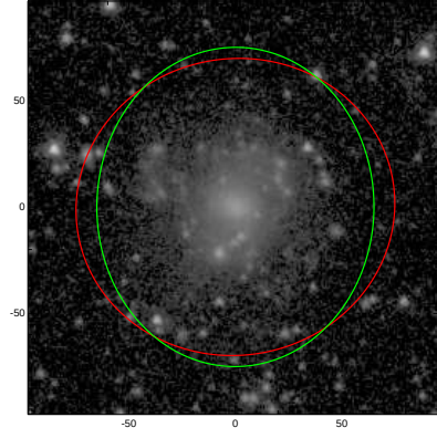
PGC031979
