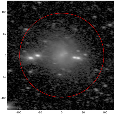
LEDA: pa,inc= 174.4 60.3
