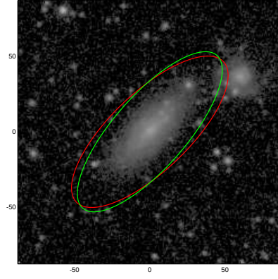
PGC043236
