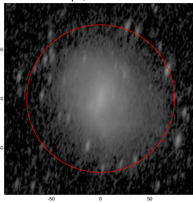
LEDA: pa,inc= 77.4 67.7
