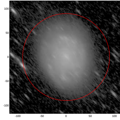
LEDA: pa,inc= 133.9 72.8
