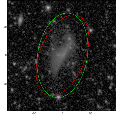
PGC044906
