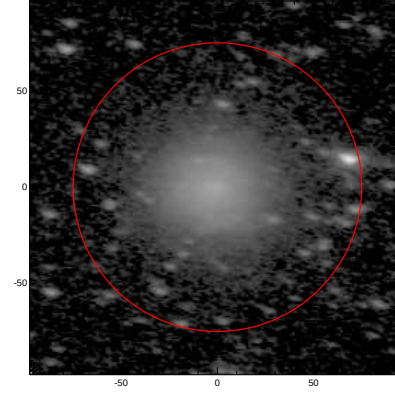
LEDA: pa,inc= 169.7 58.7
