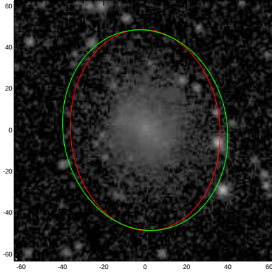
PGC1063216
