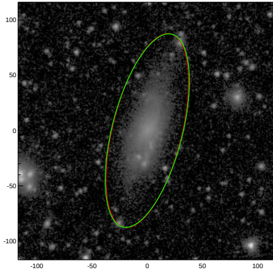
PGC014768
