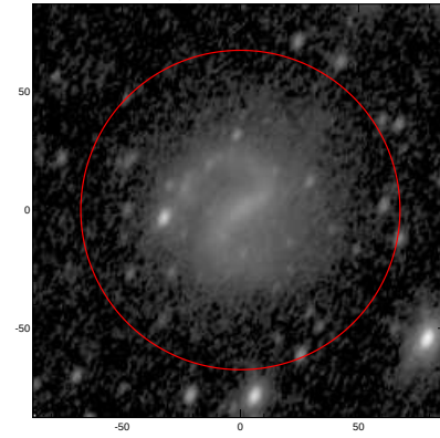
LEDA: pa,inc= 63.8 52.0
