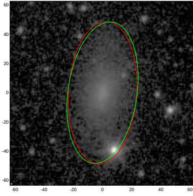
PGC004143
