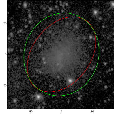
PGC047846
