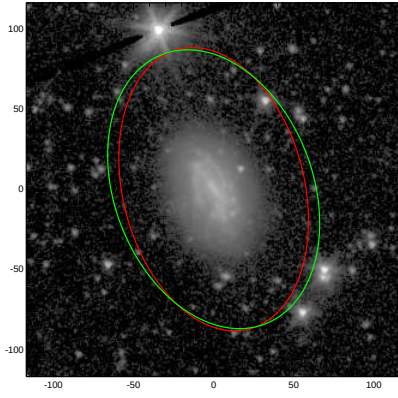
PGC054944
