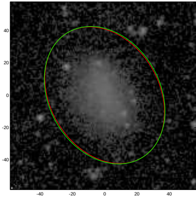
PGC007654
