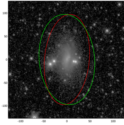
PGC037373
