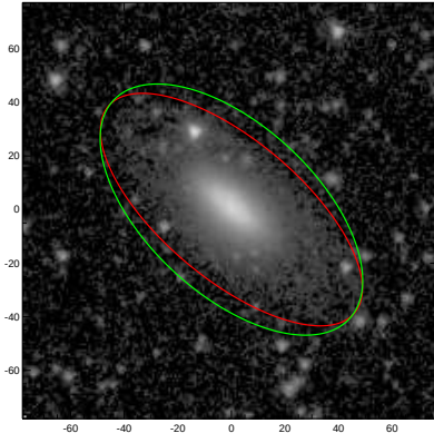
PGC053415
