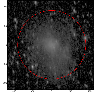
LEDA: pa,inc= 98.2 55.8
