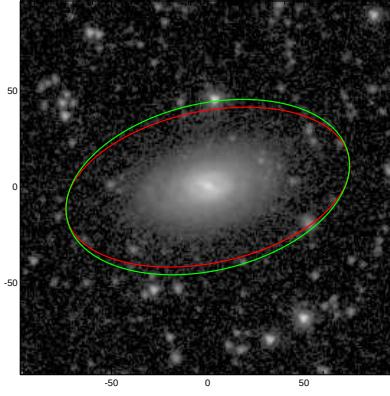
PGC053093
