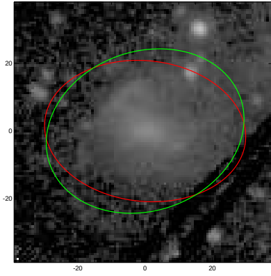
PGC038250
