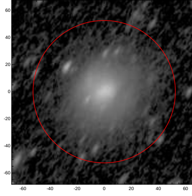
LEDA: pa,inc= 57.2 62.3
