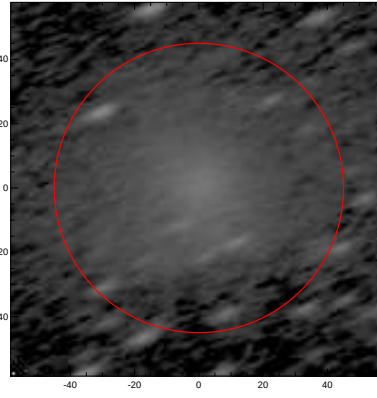
LEDA: pa,inc= 22.0 69.2
