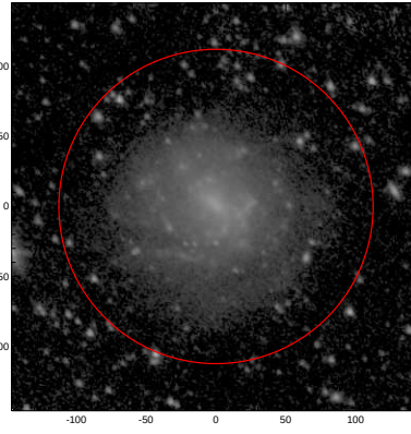
LEDA: pa,inc= 131.2 37.4
