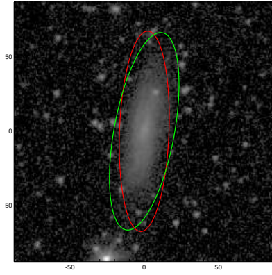
PGC006190
