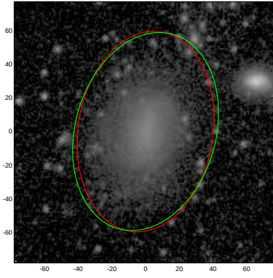
PGC002492
