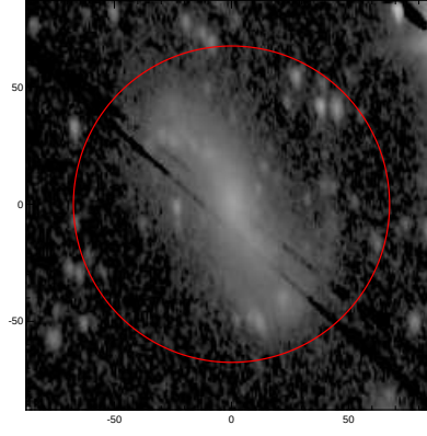
LEDA: pa,inc= 999.0 57.1
