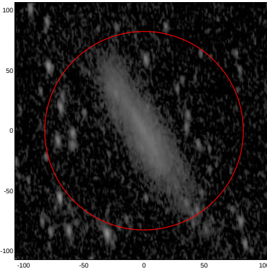
LEDA: pa,inc= 999.0 62.7
