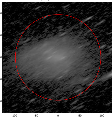
LEDA: pa,inc= 28.6 77.0
