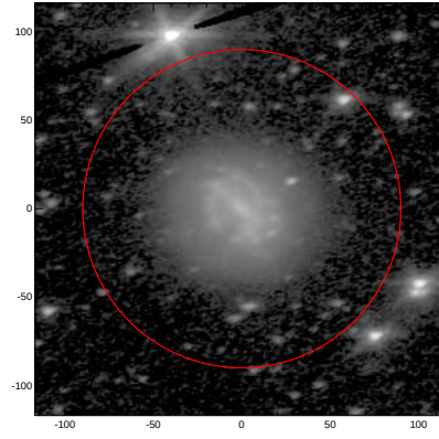
LEDA: pa,inc= 14.1 51.0
