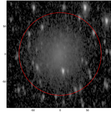
LEDA: pa,inc= 92.0 62.0
