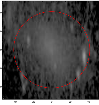
LEDA: pa,inc= 92.0 69.7
