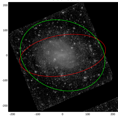
PGC043345
