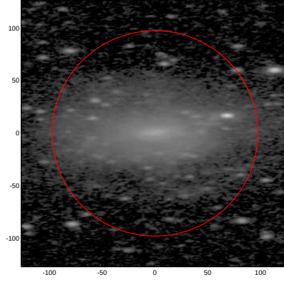
LEDA: pa,inc= 2.0 67.1
