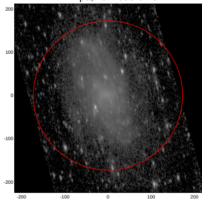
LEDA: pa,inc= 999.0 62.1
