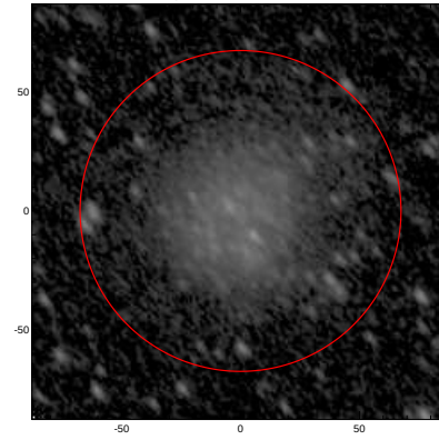
LEDA: pa,inc= 128.7 56.9
