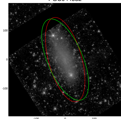
PGC044532
