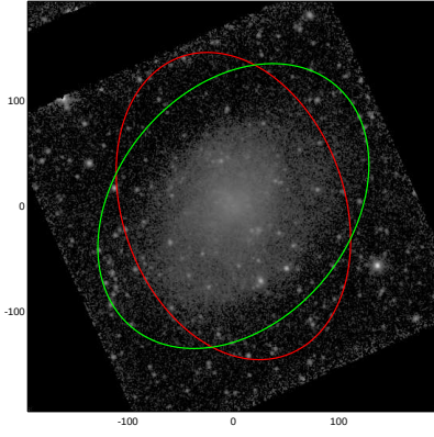
PGC043020
