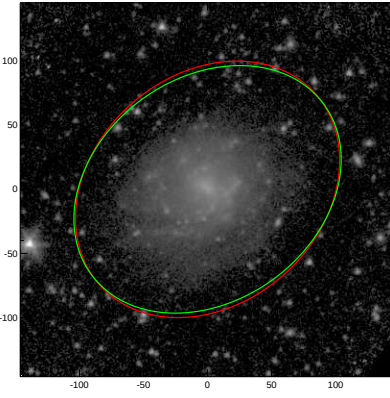
PGC006667
