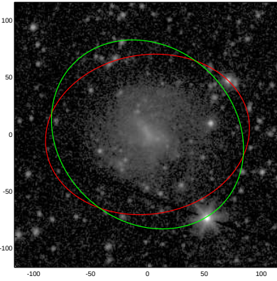
PGC068771
