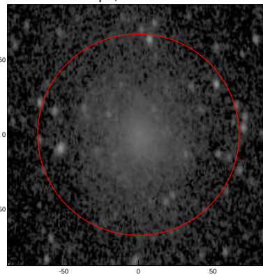
LEDA: pa,inc= 95.0 47.6
