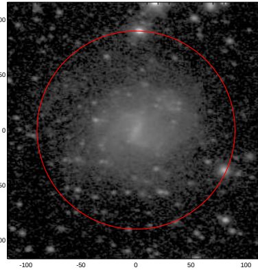
LEDA: pa,inc= 174.9 41.4
