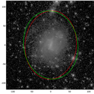
PGC036217
