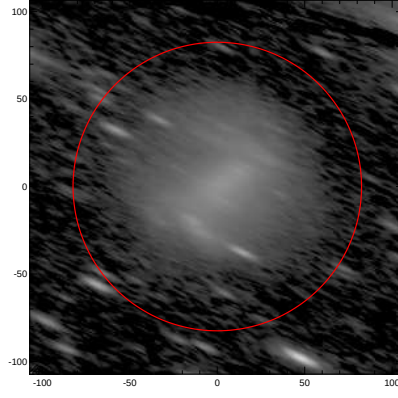
LEDA: pa,inc= 155.4 75.9
