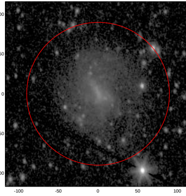
LEDA: pa,inc= 999.0 38.9
