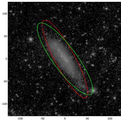
PGC008295
