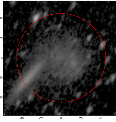
LEDA: pa,inc= 62.8 56.7
