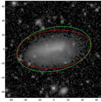
PGC051523
