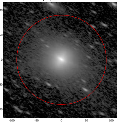
LEDA: pa,inc= 149.7 67.6
