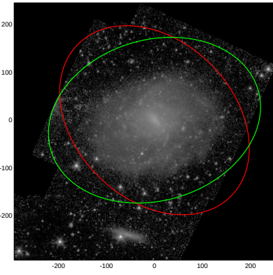
PGC003853
