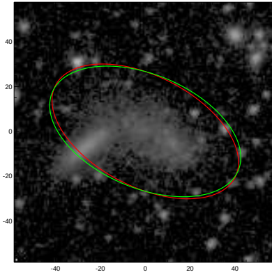
PGC016389
