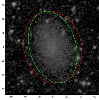
PGC006706
