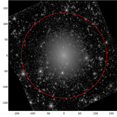
LEDA: pa,inc= 999.0 24.2
