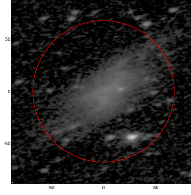
LEDA: pa,inc= 12.9 61.0
