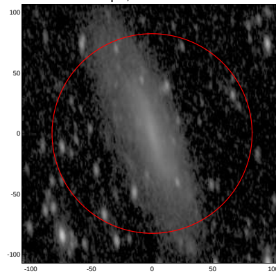
LEDA: pa,inc= 999.0 63.1
