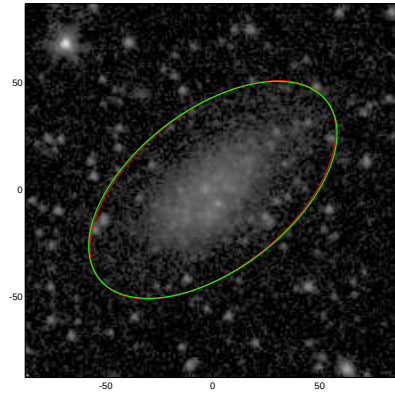
PGC035684
