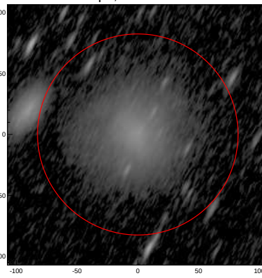
LEDA: pa,inc= 62.5 73.6
