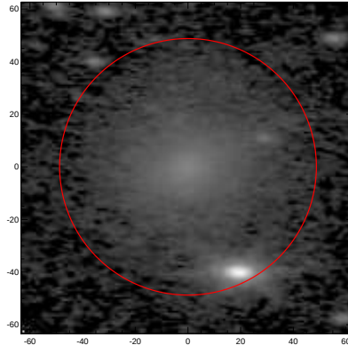
LEDA: pa,inc= 176.3 61.3
