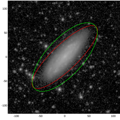
PGC013716
