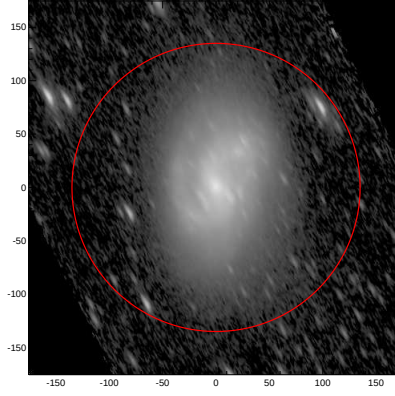
LEDA: pa,inc= 117.6 72.3
