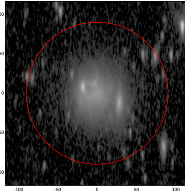
LEDA: pa,inc= 91.4 71.6
