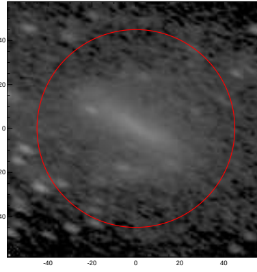
LEDA: pa,inc= 157.2 60.7
