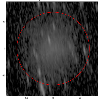
LEDA: pa,inc= 98.0 77.1
