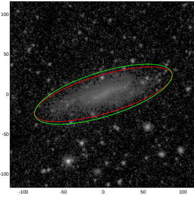
PGC009272
