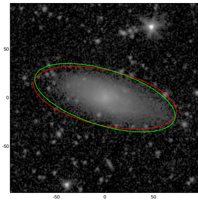
PGC006228
