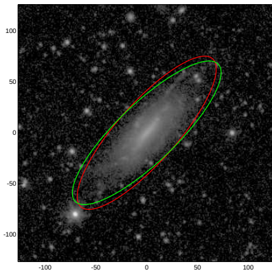
PGC036643
