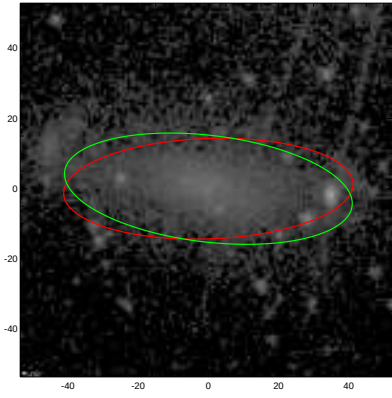
PGC005329
