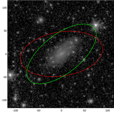
PGC045257
