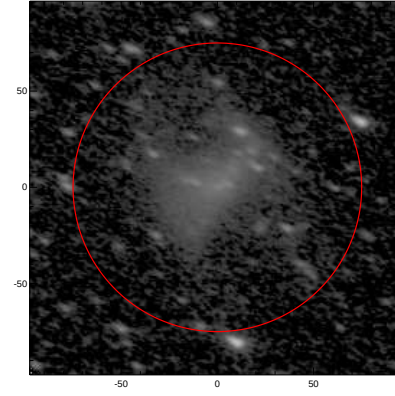
LEDA: pa,inc= 158.0 57.6
