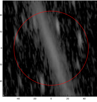
LEDA: pa,inc= 999.0 76.9
