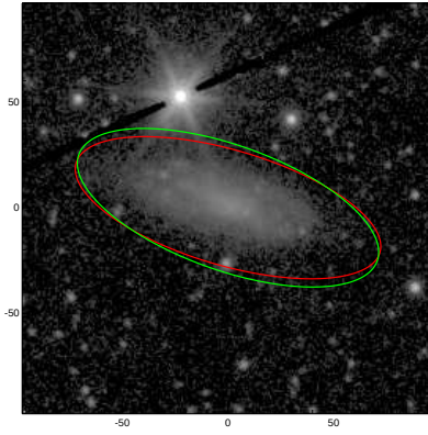
PGC036551
