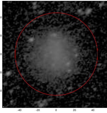
LEDA: pa,inc= 31.0 41.6
