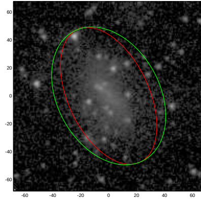
PGC015214
