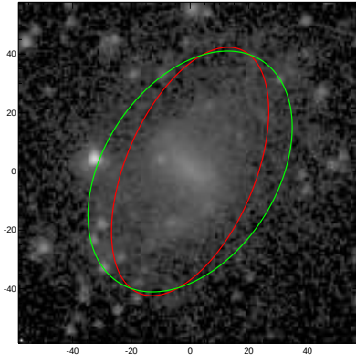
PGC067871
