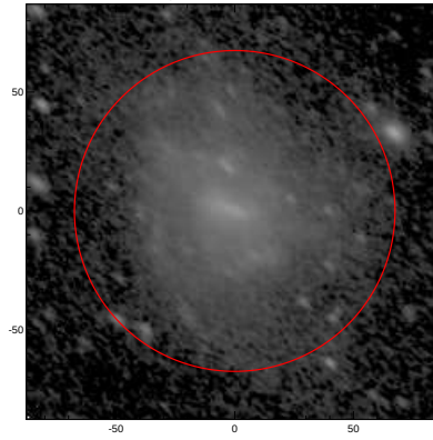
LEDA: pa,inc= 140.4 55.1
