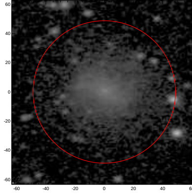
LEDA: pa,inc= 4.0 42.2
