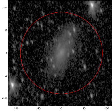
LEDA: pa,inc= 999.0 57.9
