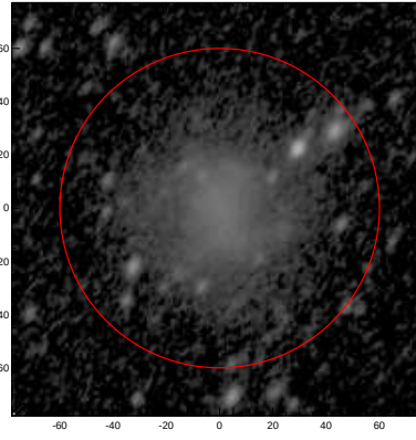
LEDA: pa,inc= 57.2 51.9
