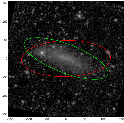
PGC007900
