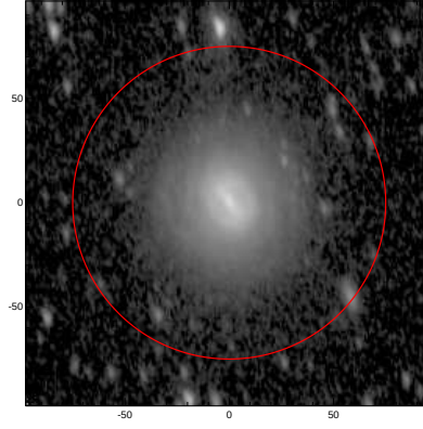
LEDA: pa,inc= 102.0 58.3
