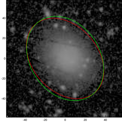
PGC007109
