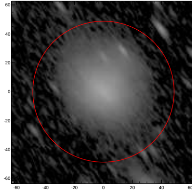
LEDA: pa,inc= 126.7 71.0
