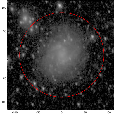
LEDA: pa,inc= 102.0 41.1
