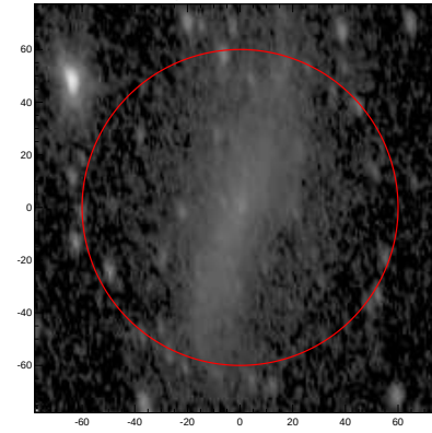
LEDA: pa,inc= 999.0 60.7
