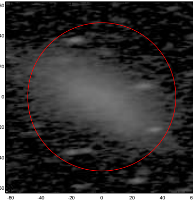
LEDA: pa,inc= 3.5 70.8
