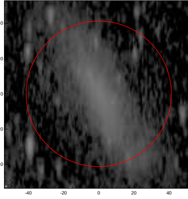
LEDA: pa,inc= 90.5 69.7
