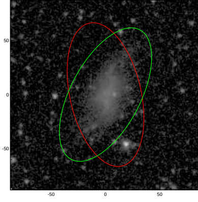
PGC049521
