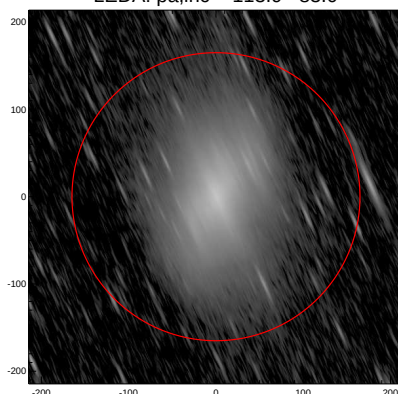
LEDA: pa,inc= 113.9 83.0
