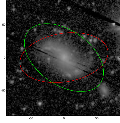
PGC072252
