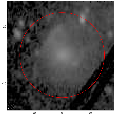
LEDA: pa,inc= 84.1 46.0
