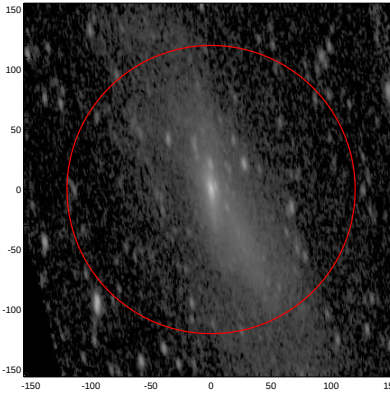
LEDA: pa,inc= 999.0 66.7
