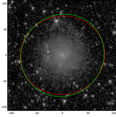
PGC048087
