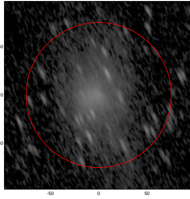
LEDA: pa,inc= 114.8 72.0
