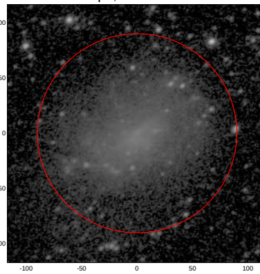
LEDA: pa,inc= 25.0 34.3
