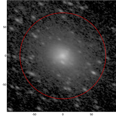
LEDA: pa,inc= 151.5 58.7
