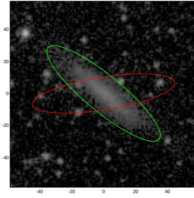
PGC008962
