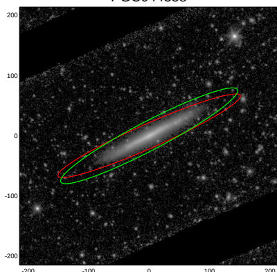
PGC044358
