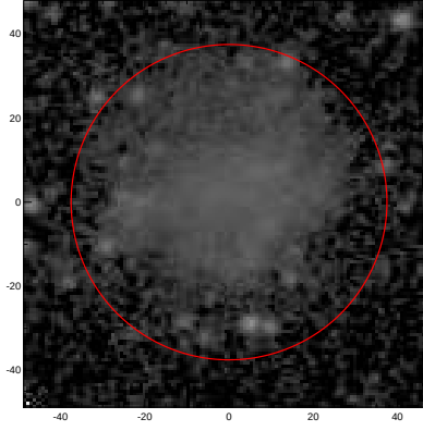
LEDA: pa,inc= 10.0 30.1
