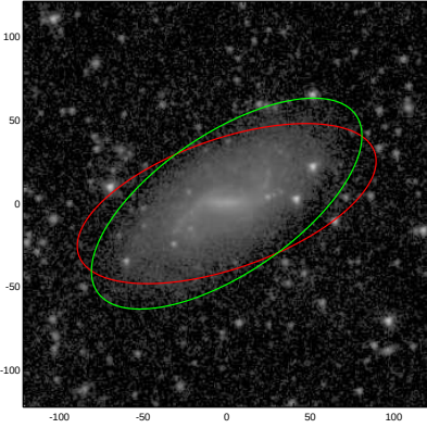
PGC011248
