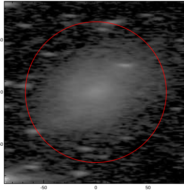
LEDA: pa,inc= 177.9 75.7
