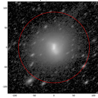
LEDA: pa,inc= 40.0 58.4
