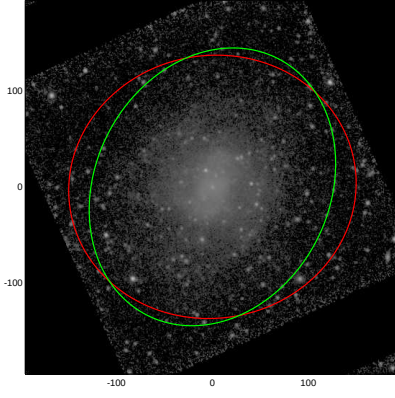
PGC042868
