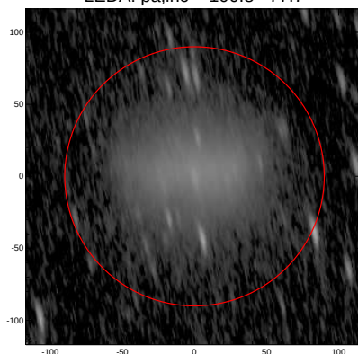
LEDA: pa,inc= 100.8 77.7
