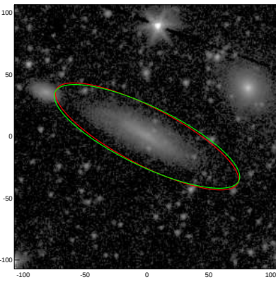
PGC006703
