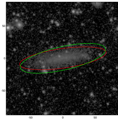
PGC039317
