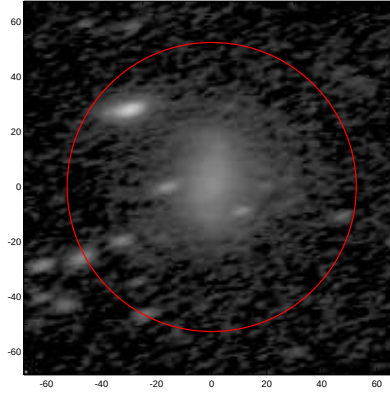
LEDA: pa,inc= 15.5 64.1
