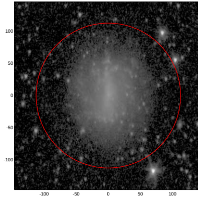
LEDA: pa,inc= 87.5 41.1
