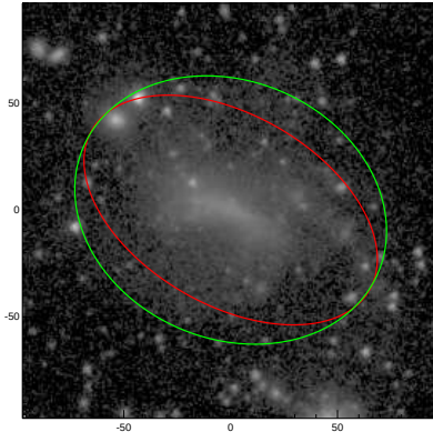
PGC016784
