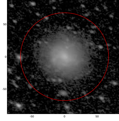
LEDA: pa,inc= 154.1 48.8
