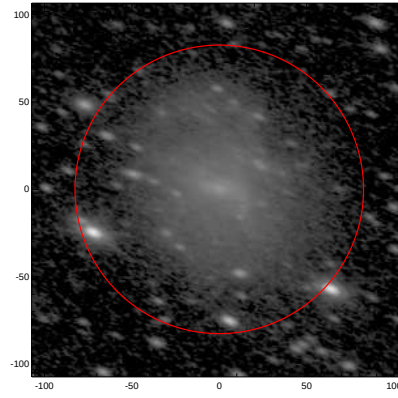
LEDA: pa,inc= 157.8 59.9
