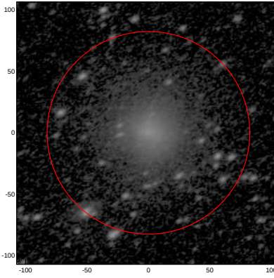
LEDA: pa,inc= 29.4 50.1
