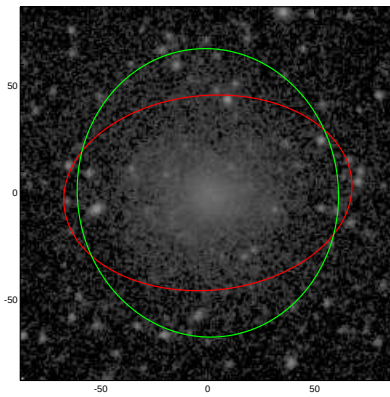
PGC009559
