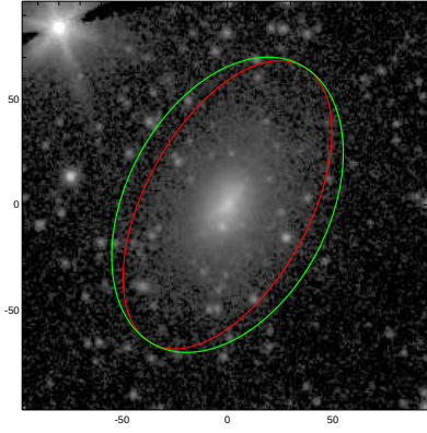
PGC050229
