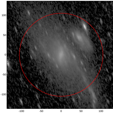
LEDA: pa,inc= 111.9 69.7
