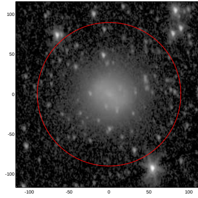
LEDA: pa,inc= 97.5 45.3
