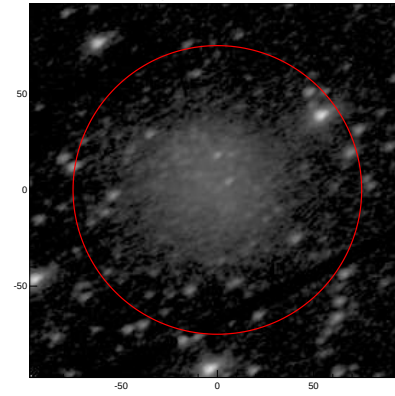
LEDA: pa,inc= 29.4 52.3
