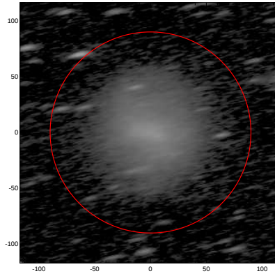
LEDA: pa,inc= 12.0 76.0
