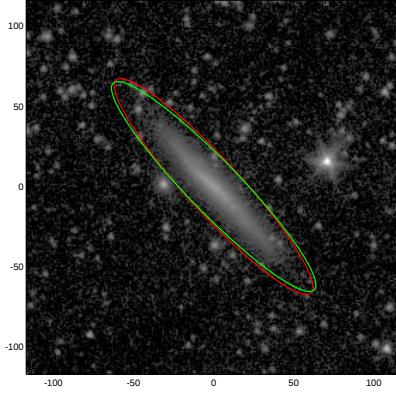
UGC05524
