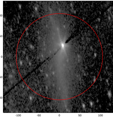
LEDA: pa,inc= 999.0 58.4
