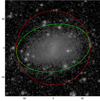
UGC10791
