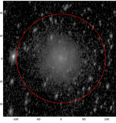
LEDA: pa,inc= 79.9 56.0
