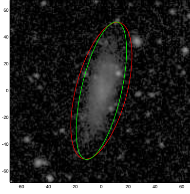
UGC08449
