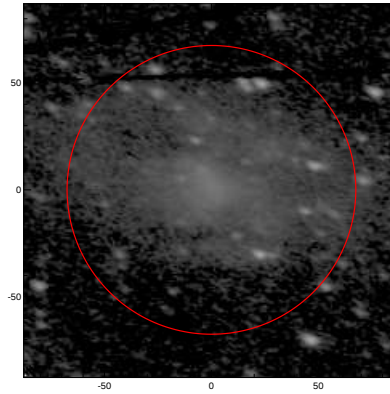
LEDA: pa,inc= 164.0 53.9
