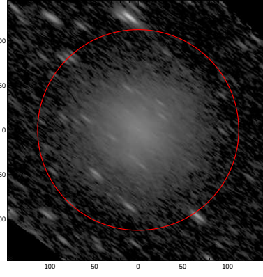
LEDA: pa,inc= 140.9 74.9
