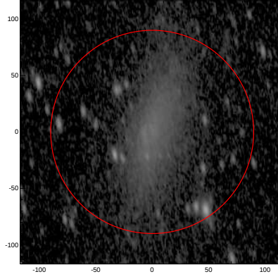
LEDA: pa,inc= 999.0 65.1
