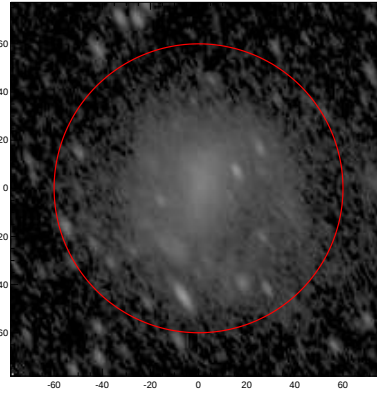
LEDA: pa,inc= 117.0 57.9
