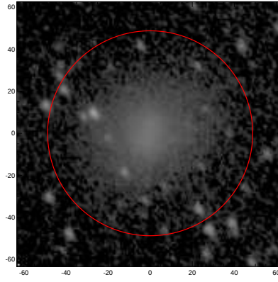
LEDA: pa,inc= 124.9 42.4
