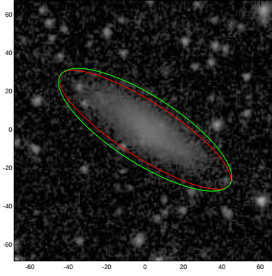
UGC00866
