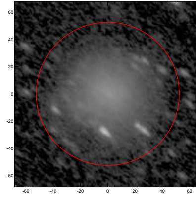
LEDA: pa,inc= 138.9 60.9
