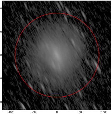
LEDA: pa,inc= 117.0 78.0
