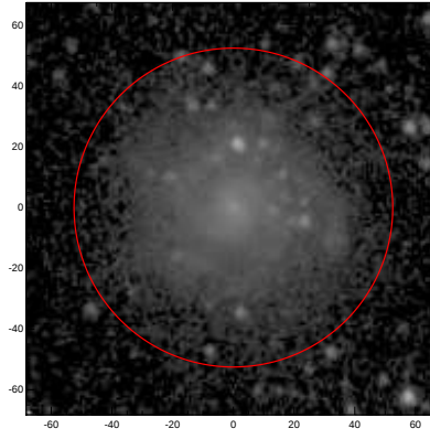
LEDA: pa,inc= 999.0 21.1
