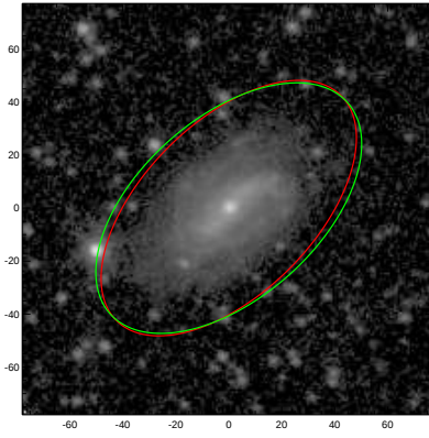
UGC05841
