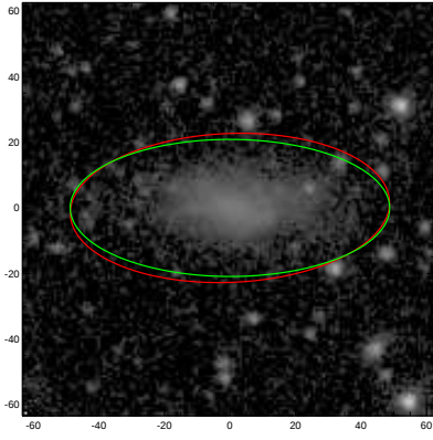
UGC10854
