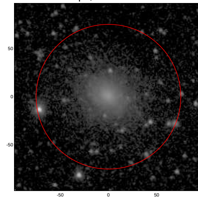
LEDA: pa,inc= 999.0 13.4
