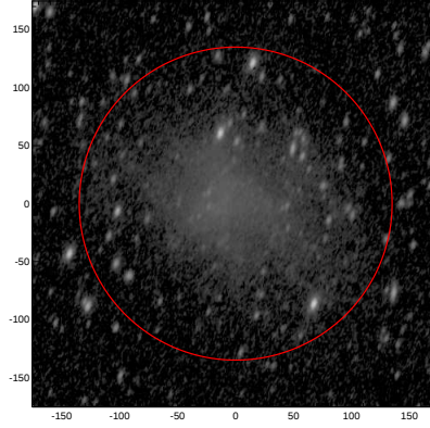
LEDA: pa,inc= 70.0 58.9
