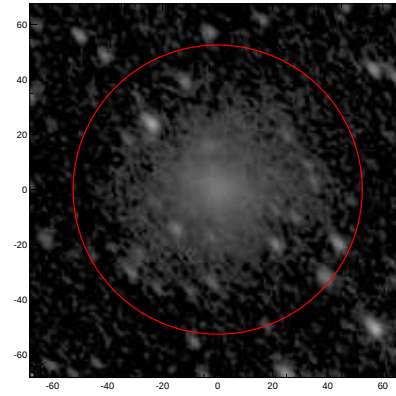
LEDA: pa,inc= 130.0 52.8
