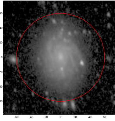
LEDA: pa,inc= 103.0 44.9
