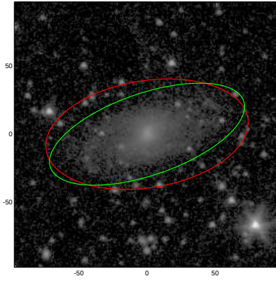
UGC04701
