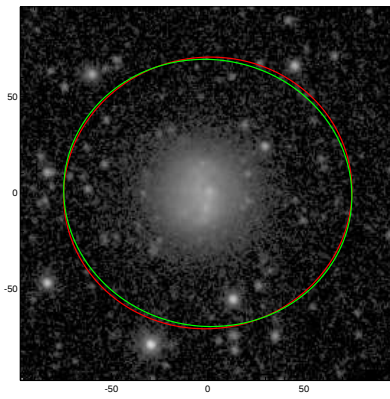
UGC06320
