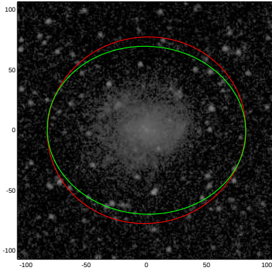
UGC06849
