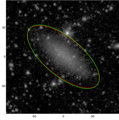
UGC07267
