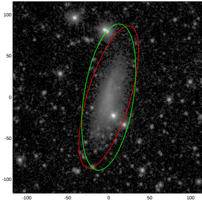
UGC09310
