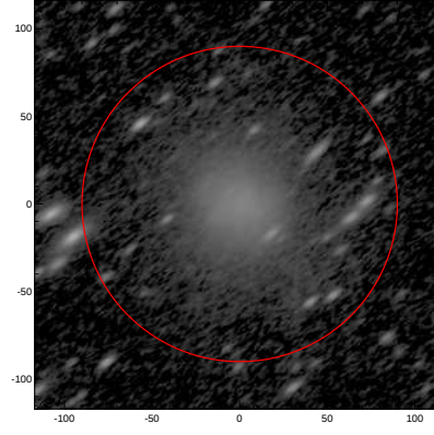
LEDA: pa,inc= 38.3 66.3
