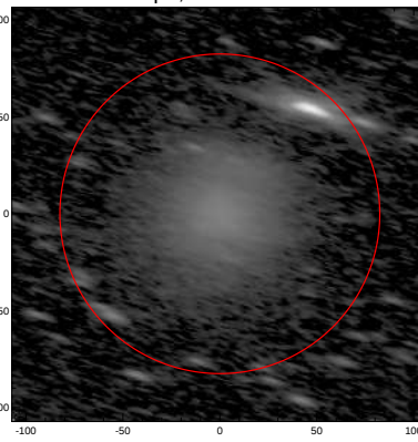
LEDA: pa,inc= 163.0 74.2
