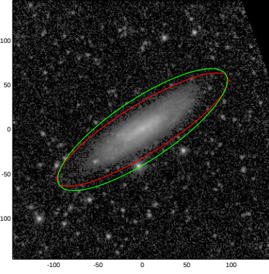
UGC05228
