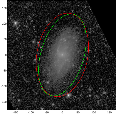
UGC08041
