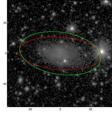
UGC07019
