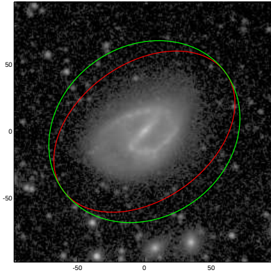
UGC06309
