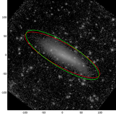
UGC06534
