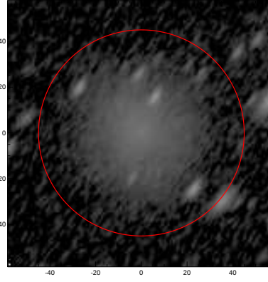
LEDA: pa,inc= 56.1 63.8
