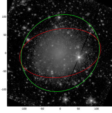
UGC07490
