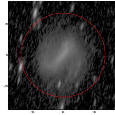
LEDA: pa,inc= 76.0 70.9
