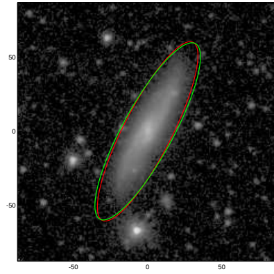
UGC08052
