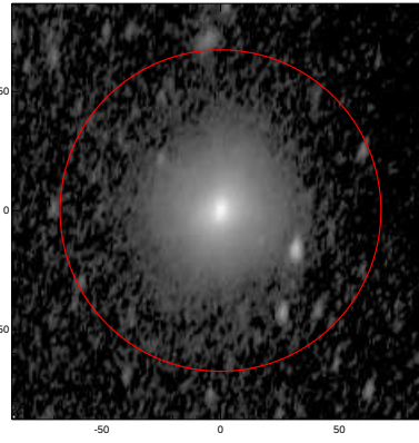
LEDA: pa,inc= 77.9 61.8
