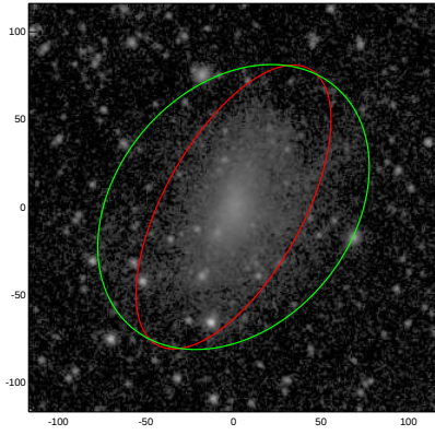
UGC04499
