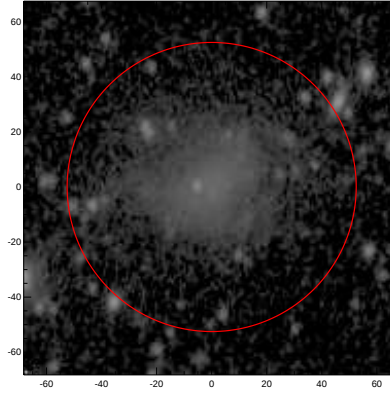
LEDA: pa,inc= 85.0 38.8
