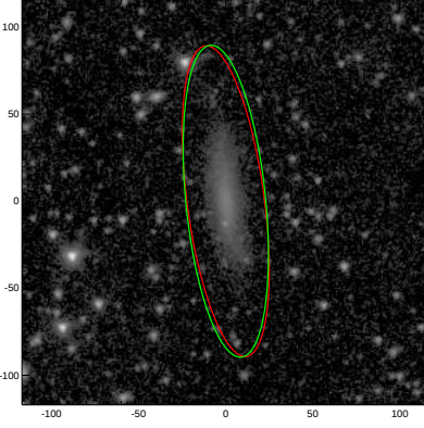
UGC09815
