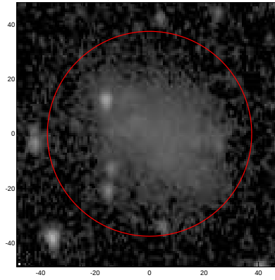
LEDA: pa,inc= 999.0 42.7
