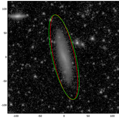
UGC06610
