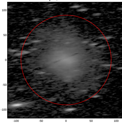
LEDA: pa,inc= 6.4 75.7
