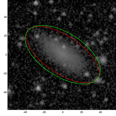
UGC05575
