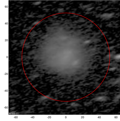
LEDA: pa,inc= 16.0 66.8
