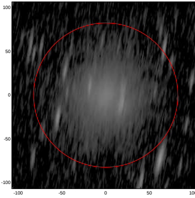
LEDA: pa,inc= 81.5 80.6
