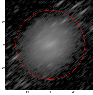
LEDA: pa,inc= 38.1 77.9
