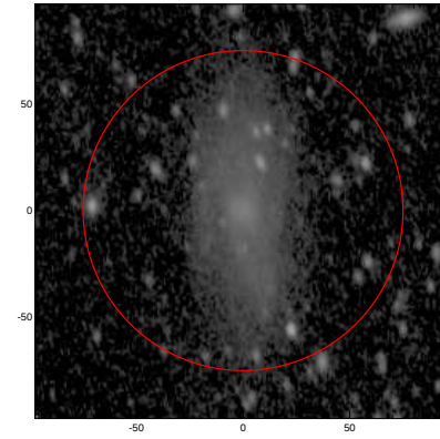
LEDA: pa,inc= 999.0 49.6
