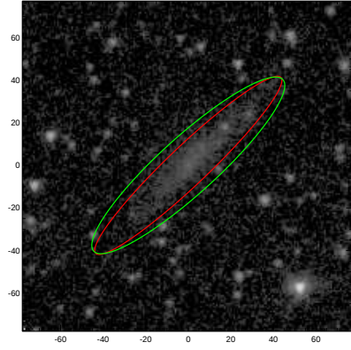
UGC00290
