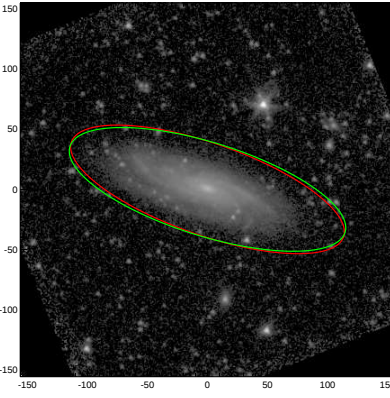
UGC05897
