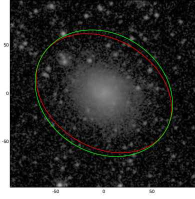
UGC08909
