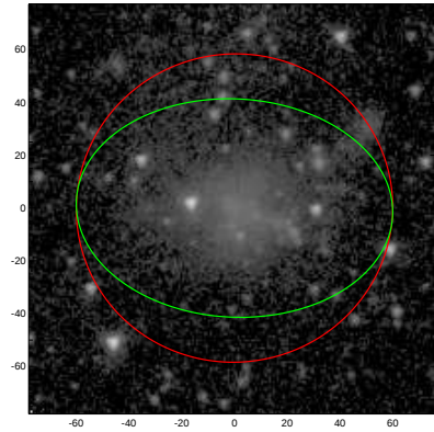
UGC01547
