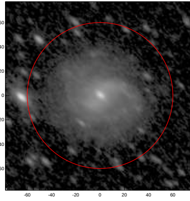
LEDA: pa,inc= 135.0 57.3
