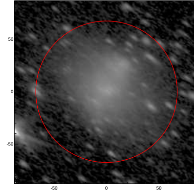
LEDA: pa,inc= 144.9 63.3
