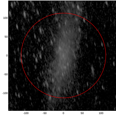
LEDA: pa,inc= 999.0 69.8
