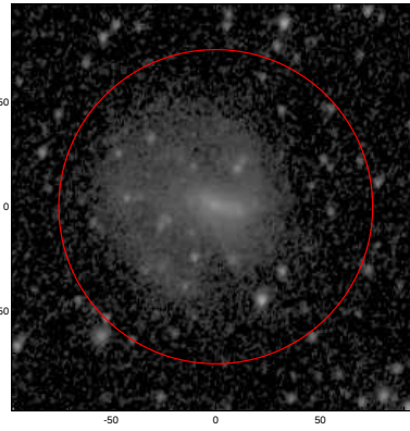
LEDA: pa,inc= 72.6 35.3
