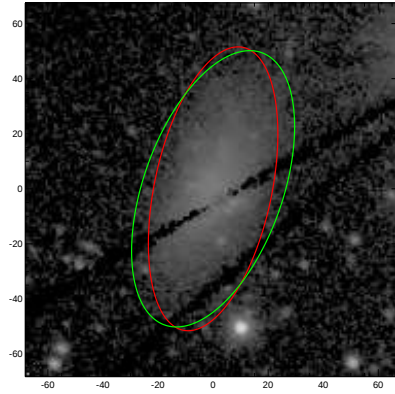
UGC06773
