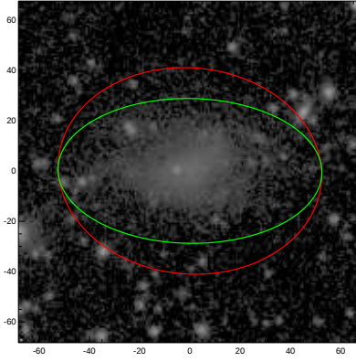
UGC00882
