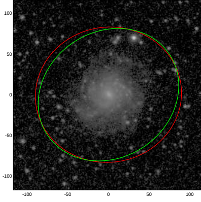
UGC09837
