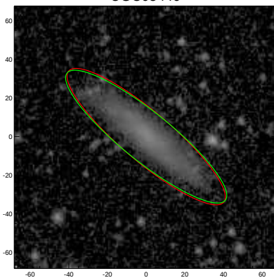
UGC05446
