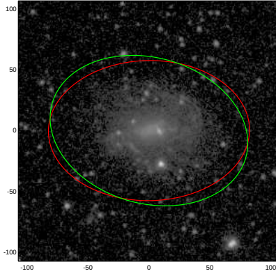
UGC07700
