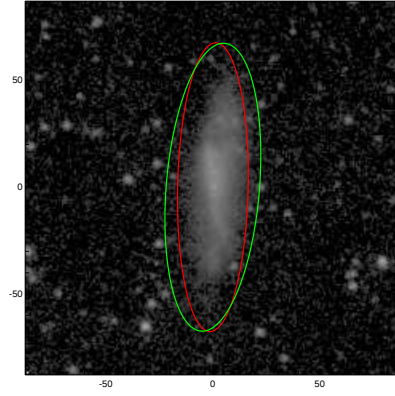
UGC07009
