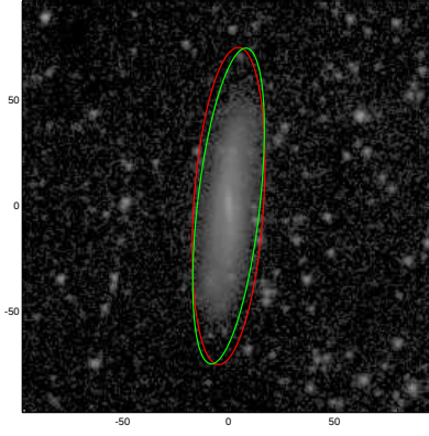
UGC01110
