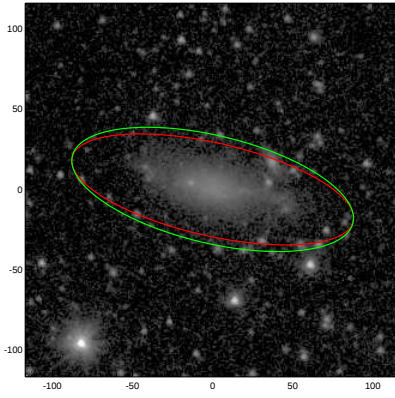
UGC06818
