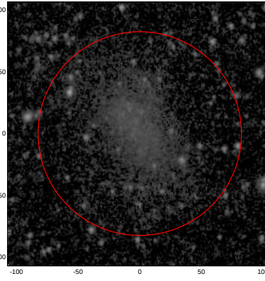
LEDA: pa,inc= 999.0 24.5
