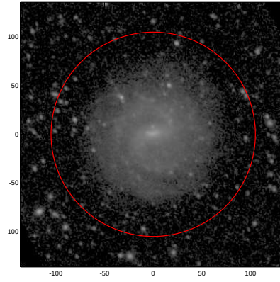
LEDA: pa,inc= 126.4 28.0
