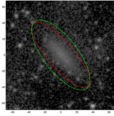
UGC08629
