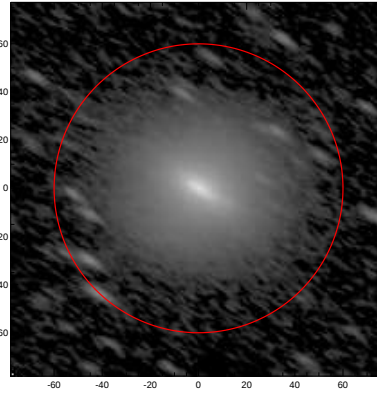
LEDA: pa,inc= 149.0 69.3
