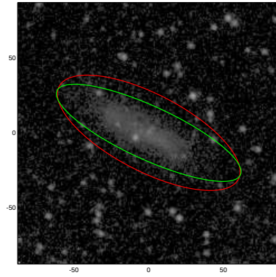
UGC07249
