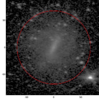
LEDA: pa,inc= 175.0 48.5
