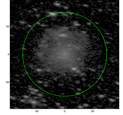
S4G: pa,inc= -9.2 61.9
