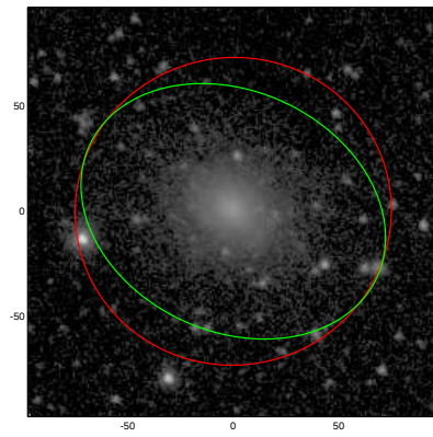
UGC06922
