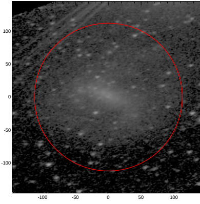
LEDA: pa,inc= 13.3 56.7
