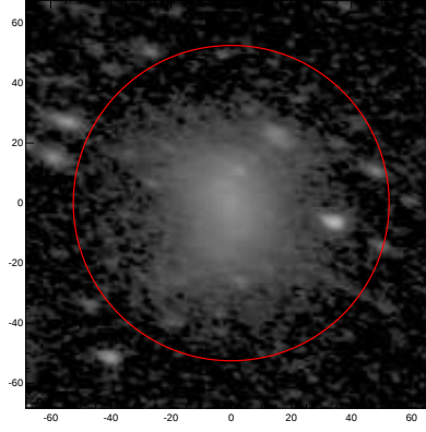
LEDA: pa,inc= 165.1 52.0
