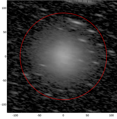
LEDA: pa,inc= 165.9 74.9
