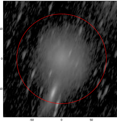
LEDA: pa,inc= 70.0 76.0
