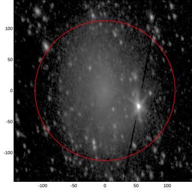
LEDA: pa,inc= 999.0 53.9
