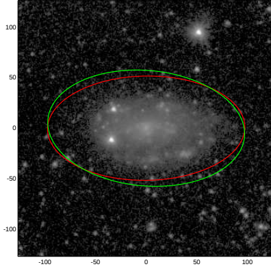
UGC06162
