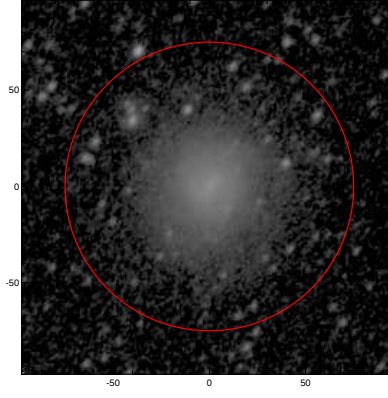
LEDA: pa,inc= 58.4 41.6
