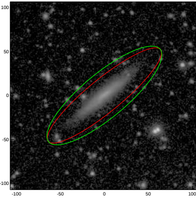
UGC05765
