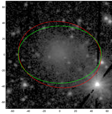
UGC05979
