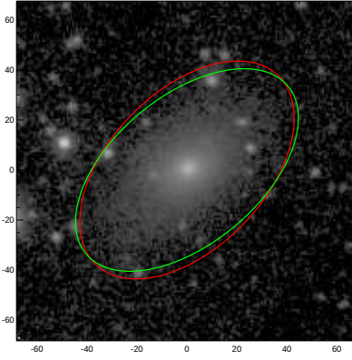
UGC05179
