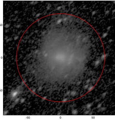
LEDA: pa,inc= 44.5 55.3
