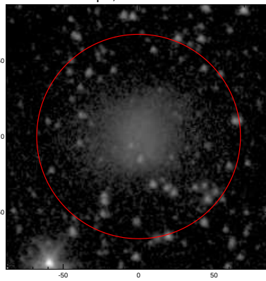
LEDA: pa,inc= 999.0 16.4
