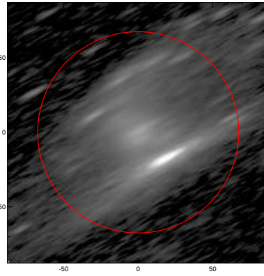
LEDA: pa,inc= 28.3 78.5
