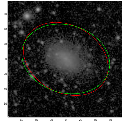
UGC04988
