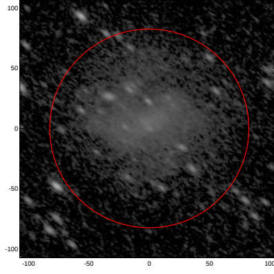
LEDA: pa,inc= 142.0 60.6
