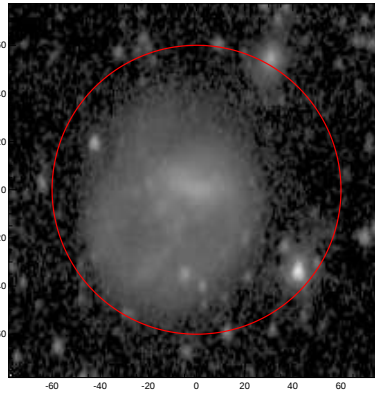
LEDA: pa,inc= 86.3 46.6
