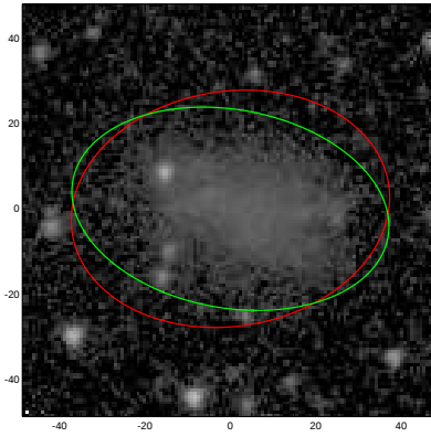
UGC00941
