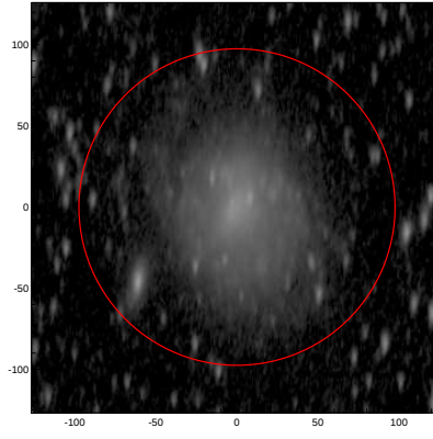
LEDA: pa,inc= 86.6 67.5
