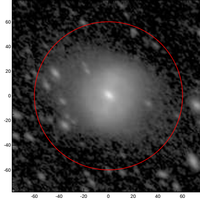
LEDA: pa,inc= 137.9 55.6
