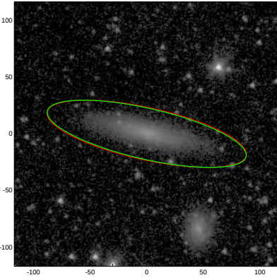
UGC05020
