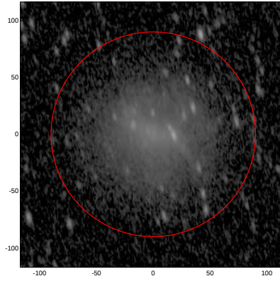
LEDA: pa,inc= 102.0 62.6
