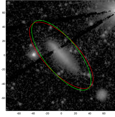
UGC05798
