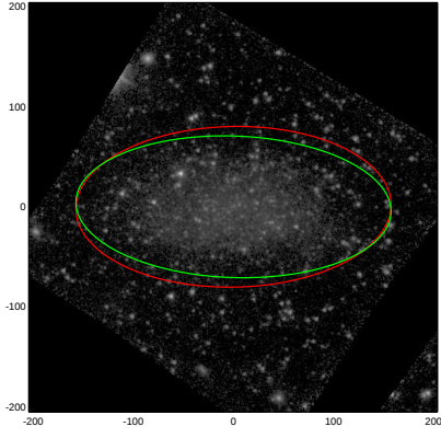
UGC08201
