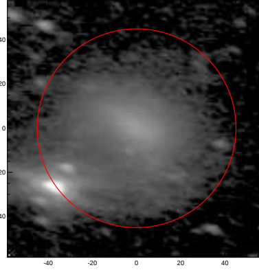
LEDA: pa,inc= 165.5 60.4
