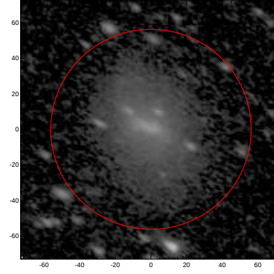
LEDA: pa,inc= 150.2 54.0
