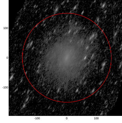
LEDA: pa,inc= 60.8 67.9
