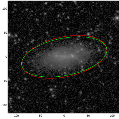
UGC08385
