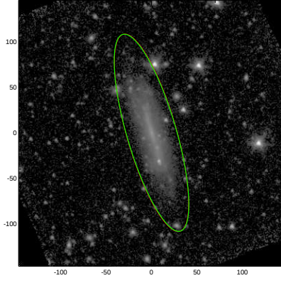
UGC05249
