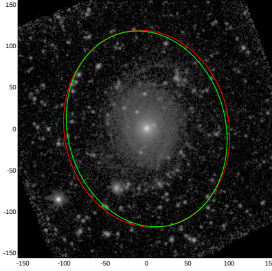
UGC08155
