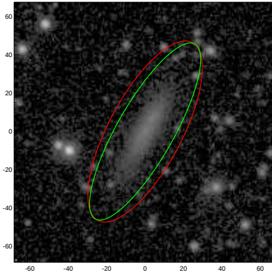
UGC06341
