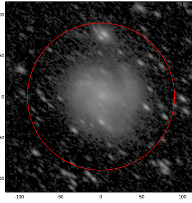
LEDA: pa,inc= 138.8 61.3
