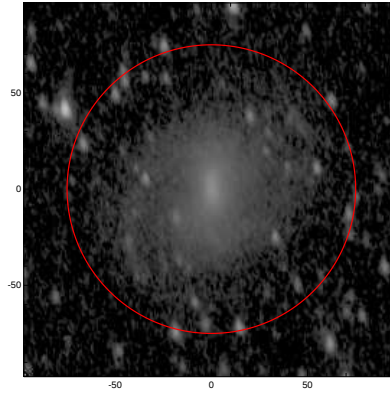
LEDA: pa,inc= 999.0 58.5
