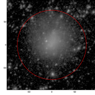
LEDA: pa,inc= 49.8 29.0
