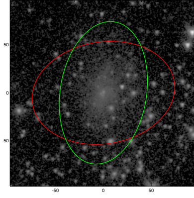
UGC00017
