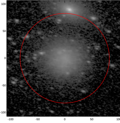
LEDA: pa,inc= 167.8 56.3
