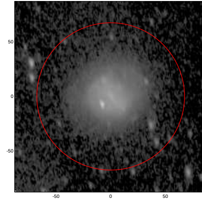
LEDA: pa,inc= 100.9 57.9
