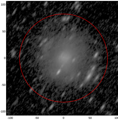
LEDA: pa,inc= 55.2 68.5
