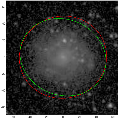
UGC06335
