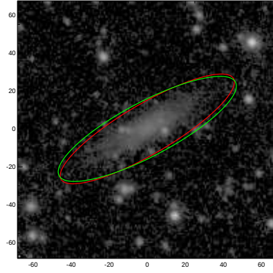
UGC04953
