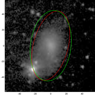
UGC03070
