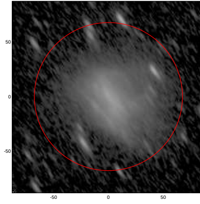
LEDA: pa,inc= 125.1 71.2
