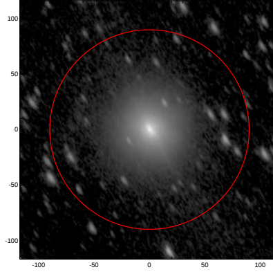
LEDA: pa,inc= 120.9 63.3
