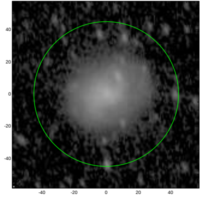
S4G: pa,inc= 100.1 54.4
