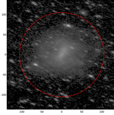
LEDA: pa,inc= 157.5 62.9
