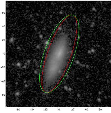
UGC06307
