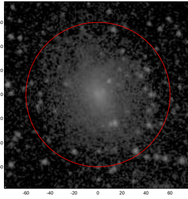
LEDA: pa,inc= 999.0 18.5
