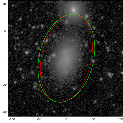
UGC01200
