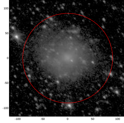
LEDA: pa,inc= 139.3 44.9
