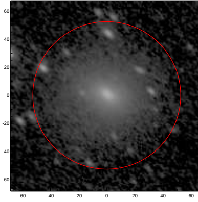
LEDA: pa,inc= 135.9 53.4
