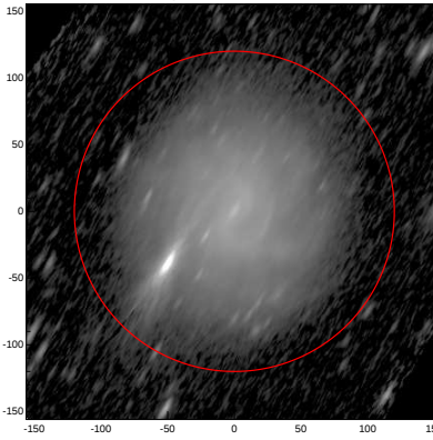
LEDA: pa,inc= 59.8 74.9
