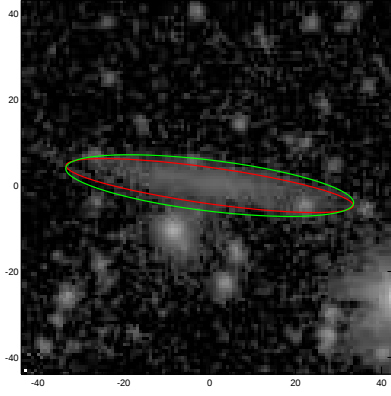
UGC10025
