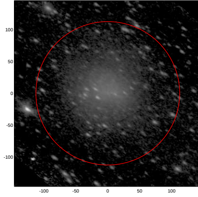
LEDA: pa,inc= 148.0 57.7
