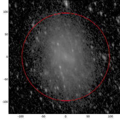
LEDA: pa,inc= 107.5 55.4
