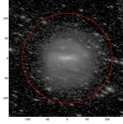
LEDA: pa,inc= 161.9 62.1
