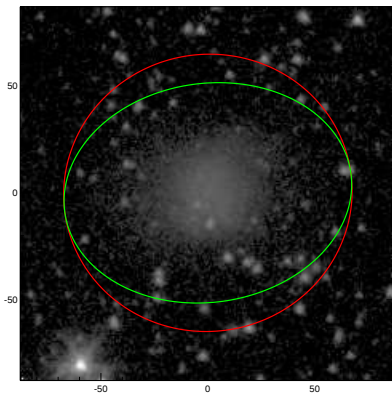
UGC05076
