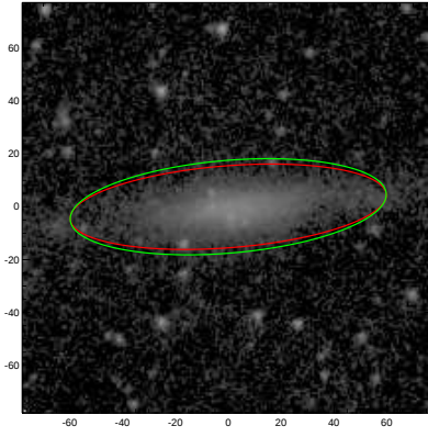
UGC01999
