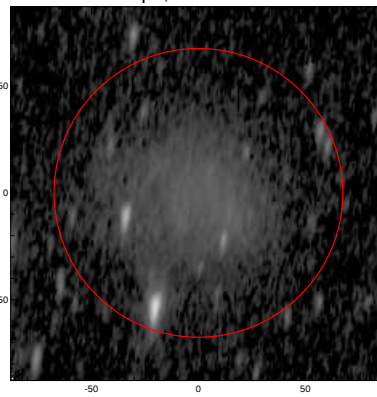
LEDA: pa,inc= 83.0 69.1
