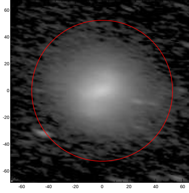
LEDA: pa,inc= 166.7 72.7
