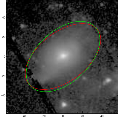
UGC05814
