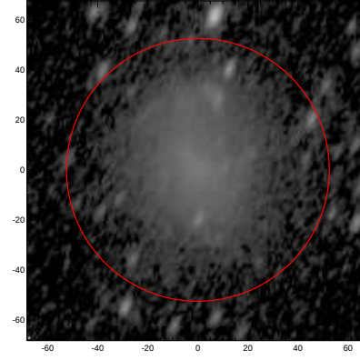
LEDA: pa,inc= 64.5 59.5
