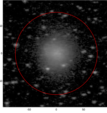
LEDA: pa,inc= 179.0 51.2
