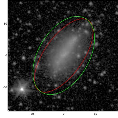
UGC05456
