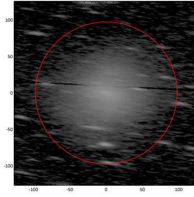
LEDA: pa,inc= 173.0 79.5
