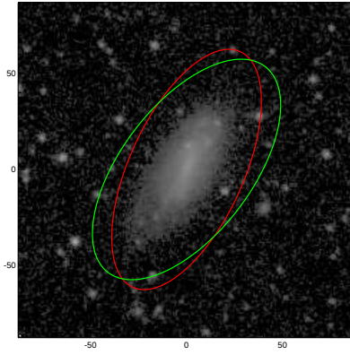
UGC07184
