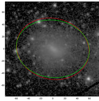
UGC04390
