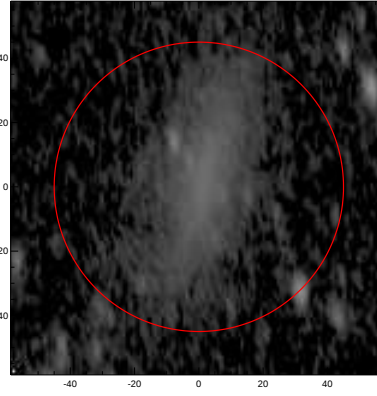
LEDA: pa,inc= 999.0 64.9
