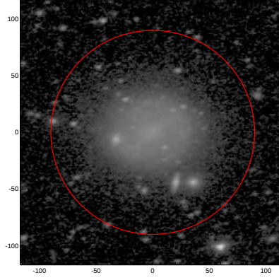
LEDA: pa,inc= 6.0 48.4
