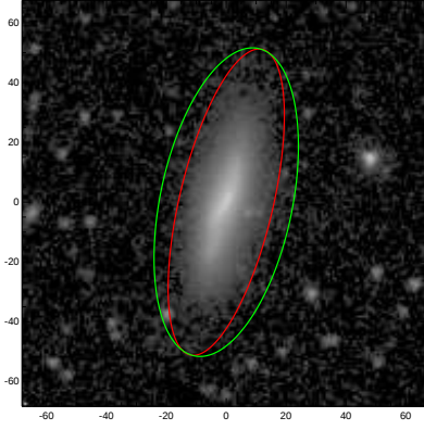
UGC09703
