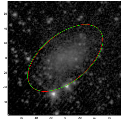
UGC07599
