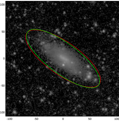
UGC05238
