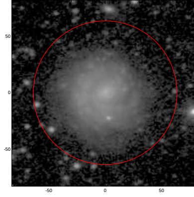
LEDA: pa,inc= 7.0 33.9
