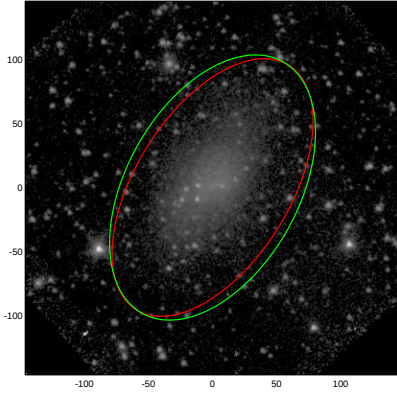
UGC07639
