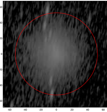
LEDA: pa,inc= 80.7 76.0
