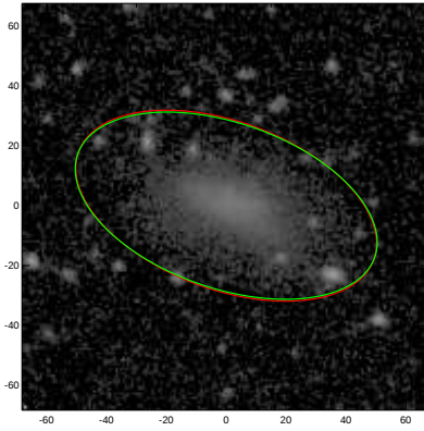
UGC06014
