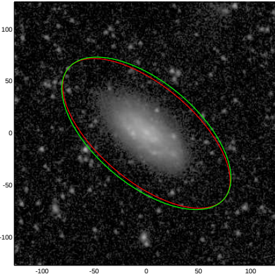
UGC06023
