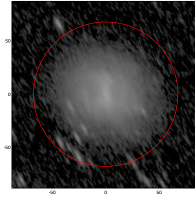
LEDA: pa,inc= 119.5 71.6
