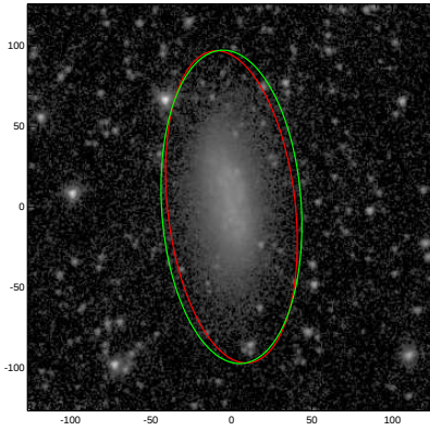
UGC01945
