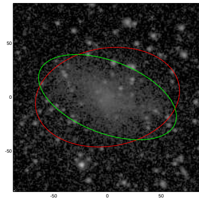
UGC08441
