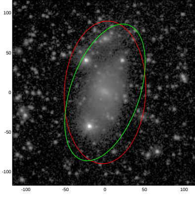
UGC07189
