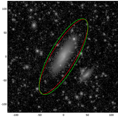
UGC07035
