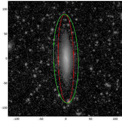
UGC06169
