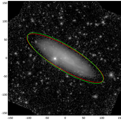
UGC04623
