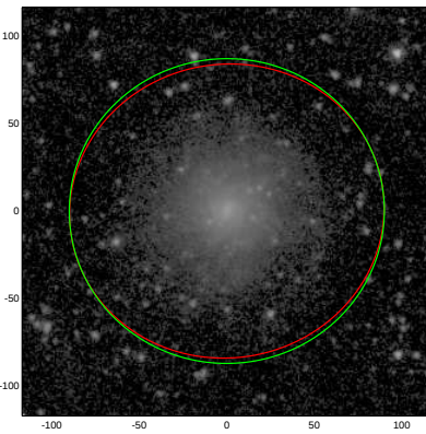
UGC10020
