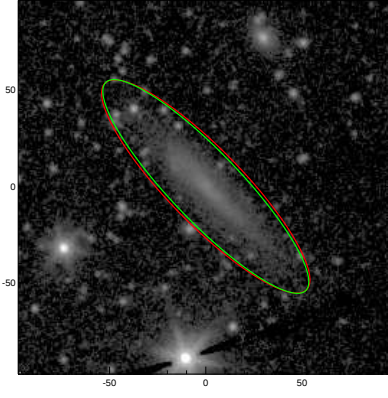
UGC05107
