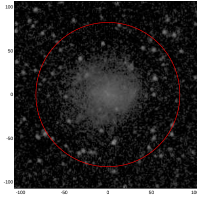
LEDA: pa,inc= 999.0 20.4
