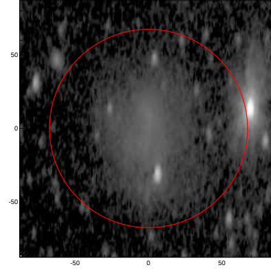
LEDA: pa,inc= 86.0 66.7
