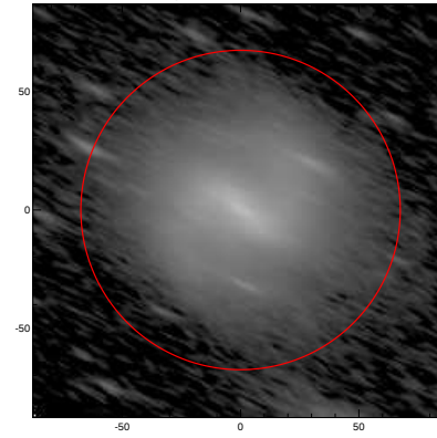
LEDA: pa,inc= 153.0 76.1
