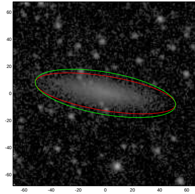
UGC08181
