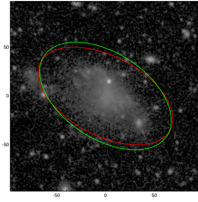
UGC06345
