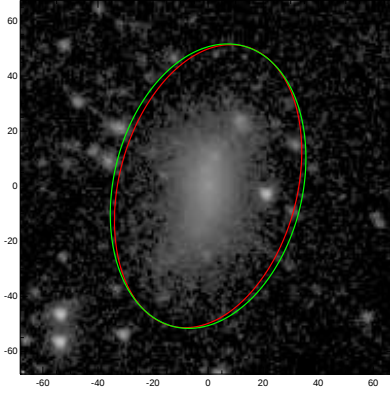
UGC07257
