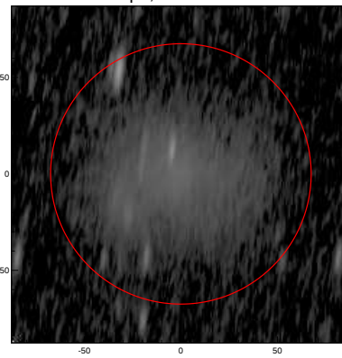
LEDA: pa,inc= 83.0 77.3
