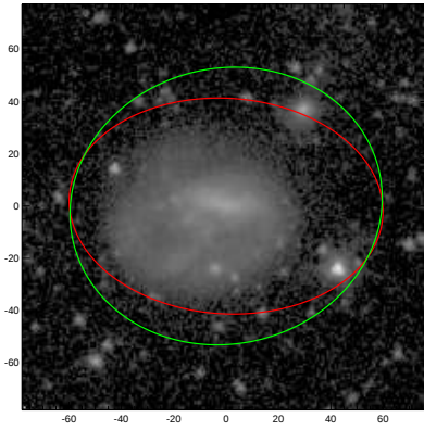
UGC05832
