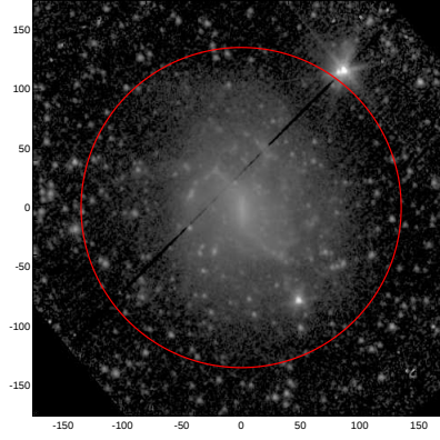
LEDA: pa,inc= 999.0 24.8
