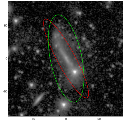
UGC10650
