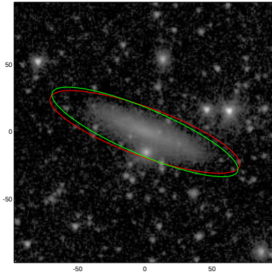
UGC09991
