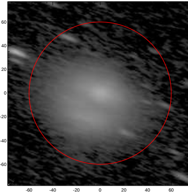
LEDA: pa,inc= 160.6 73.4
