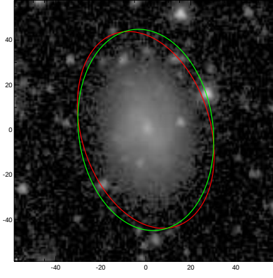
UGC05922
