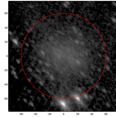
LEDA: pa,inc= 129.9 57.9
