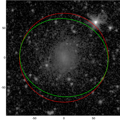
UGC00099
