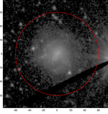
LEDA: pa,inc= 999.0 15.0
