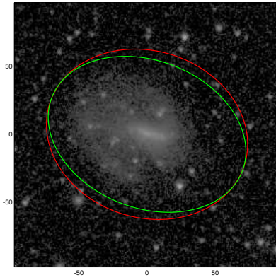
UGC08084
