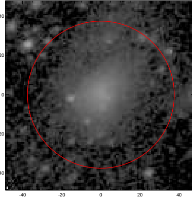
LEDA: pa,inc= 32.8 31.7
