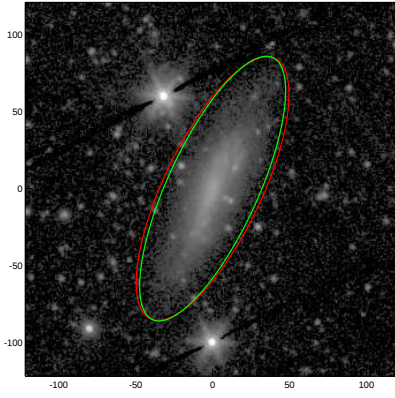
UGC06670
