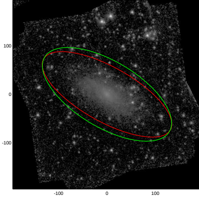
UGC04922
