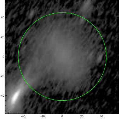
S4G: pa,inc= 60.5 70.2
