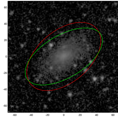
UGC09951
