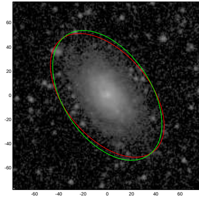
UGC06517
