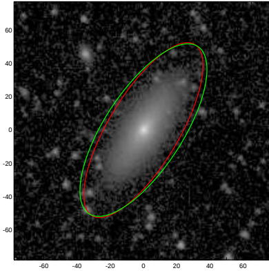
UGC05833
