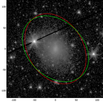
UGC07943
