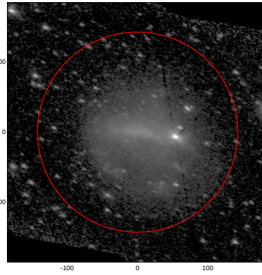
LEDA: pa,inc= 154.0 51.3
