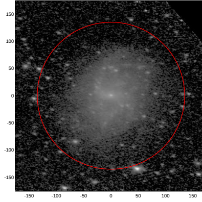
LEDA: pa,inc= 169.2 53.0
