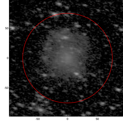
LEDA: pa,inc= 167.0 57.2
