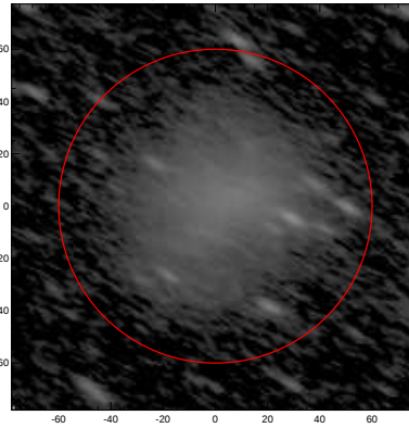
LEDA: pa,inc= 151.5 69.3
