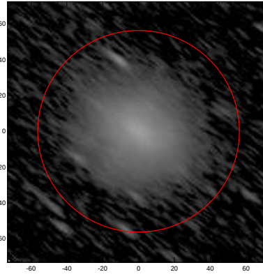
LEDA: pa,inc= 142.0 74.9
