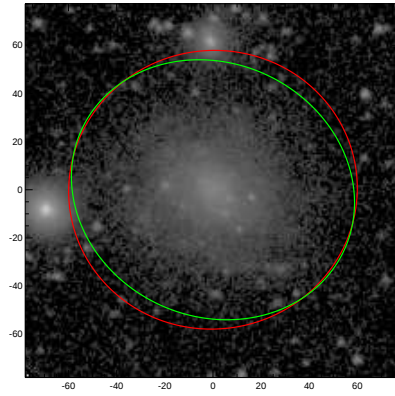
UGC06249
