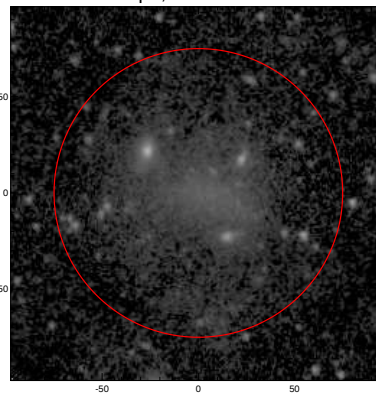
LEDA: pa,inc= 999.0 18.1
