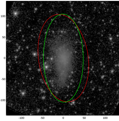
UGC00156
