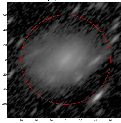
LEDA: pa,inc= 45.4 74.1
