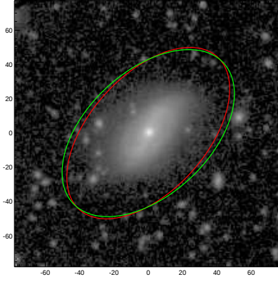
UGC04621
