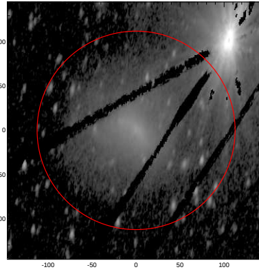
LEDA: pa,inc= 79.7 66.0
