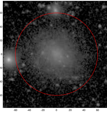
LEDA: pa,inc= 999.0 15.5
