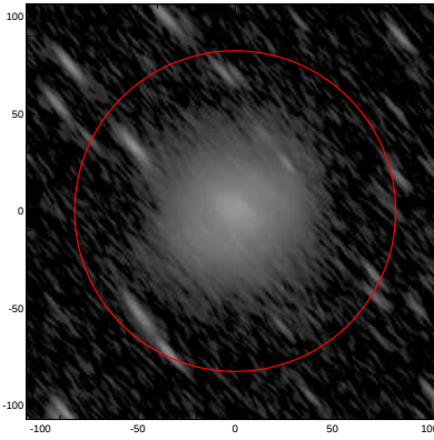
LEDA: pa,inc= 129.2 76.8
