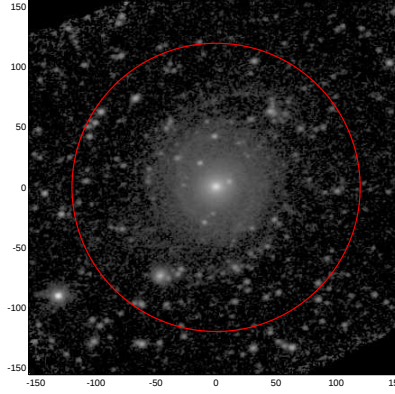
LEDA: pa,inc= 11.6 33.7
