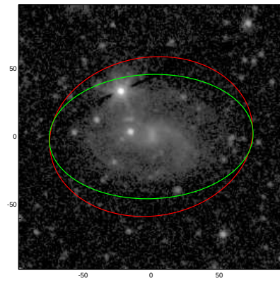
UGC04867
