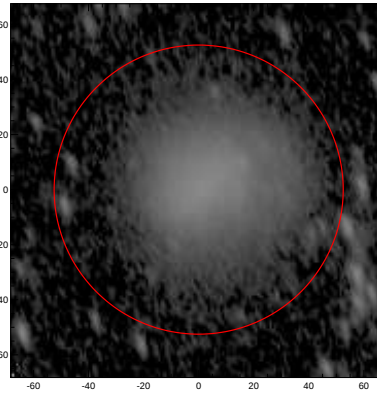
LEDA: pa,inc= 108.5 63.3
