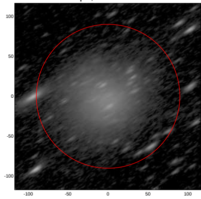
LEDA: pa,inc= 32.7 72.6
