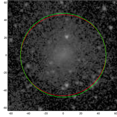
UGC09875
