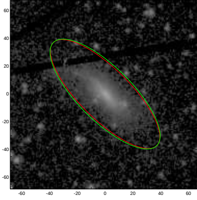
UGC05791
