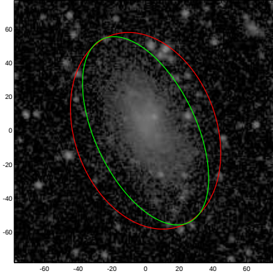
UGC08053
