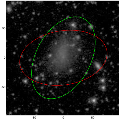
UGC09992
