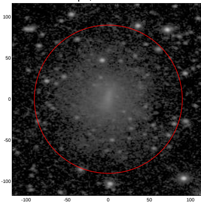
LEDA: pa,inc= 176.1 45.3
