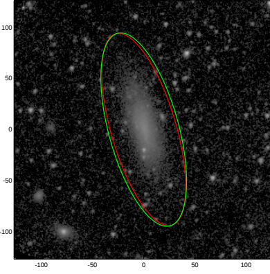
UGC00132
