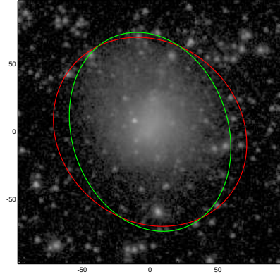
UGC07690
