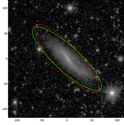
UGC09389
