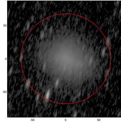
LEDA: pa,inc= 75.2 72.4
