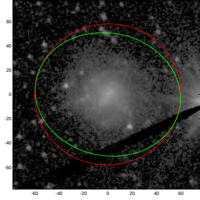
UGC06194
