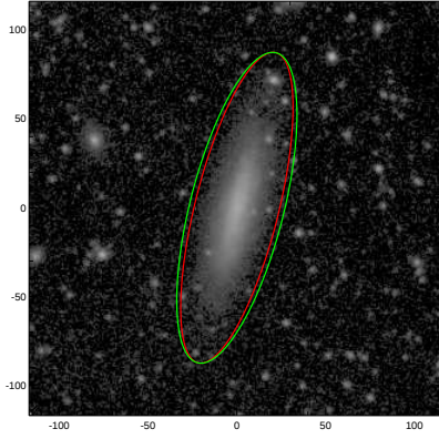
UGC05646
