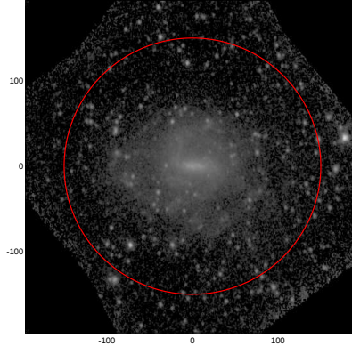
LEDA: pa,inc= 95.2 36.7
