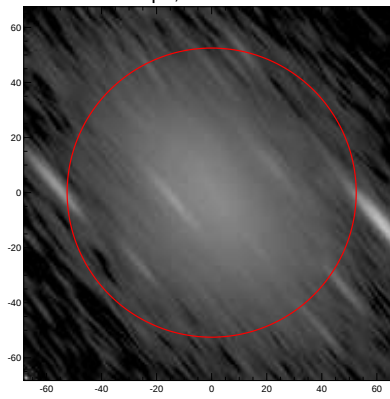
LEDA: pa,inc= 129.5 81.5
