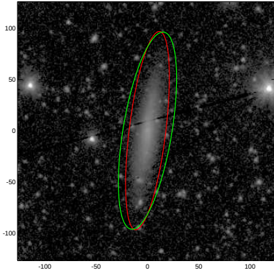
UGC06792
