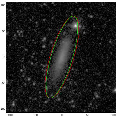
UGC05921
