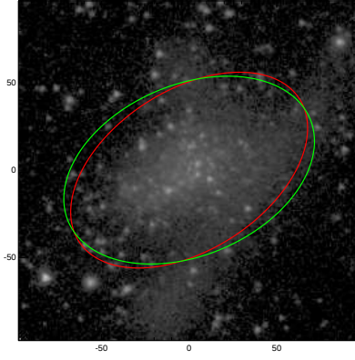
UGC08508
