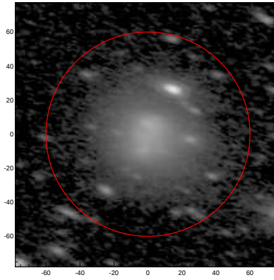
LEDA: pa,inc= 164.0 61.0
