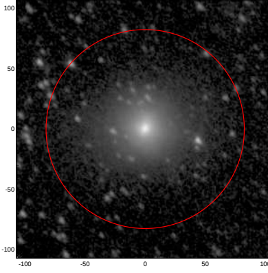
LEDA: pa,inc= 129.3 41.4
