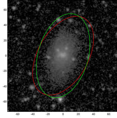
UGC08042
