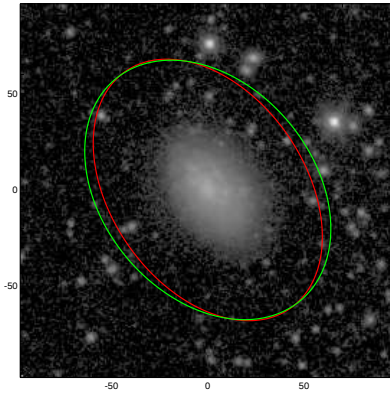
UGC08516
