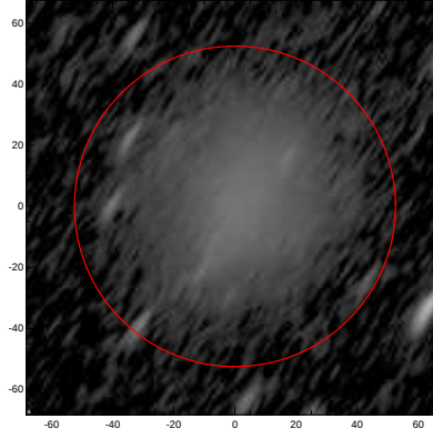
LEDA: pa,inc= 57.1 74.2
