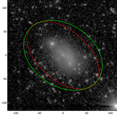
UGC09274
