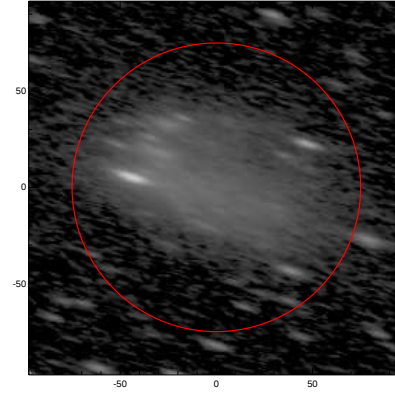
LEDA: pa,inc= 164.1 73.2
