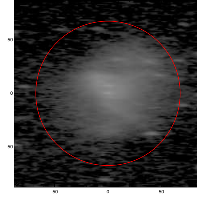
LEDA: pa,inc= 178.8 75.9
