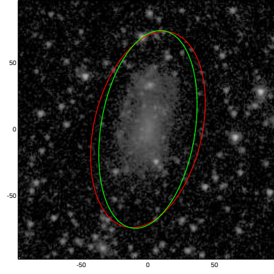
UGC09936
