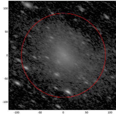
LEDA: pa,inc= 151.0 63.9
