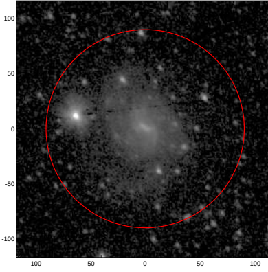
LEDA: pa,inc= 123.4 31.4
