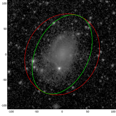
UGC00191
