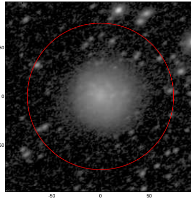
LEDA: pa,inc= 34.8 47.8
