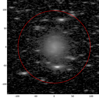
LEDA: pa,inc= 1.2 68.5
