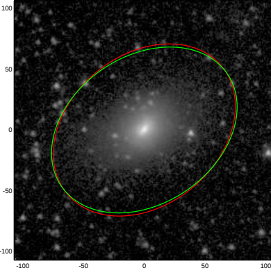
UGC05720
