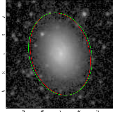
UGC10803
