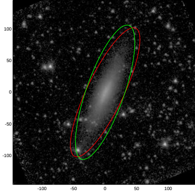
UGC05672
