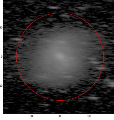
LEDA: pa,inc= 176.3 77.3
