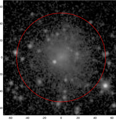
LEDA: pa,inc= 999.0 10.3
