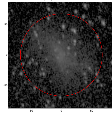
LEDA: pa,inc= 999.0 47.6
