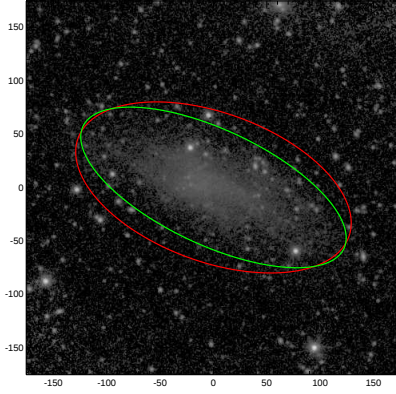
UGC06955
