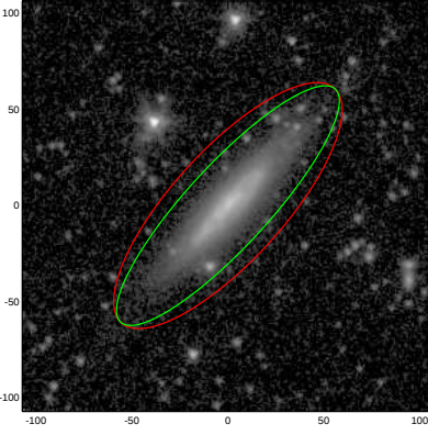
UGC08067
