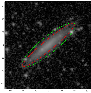
UGC06390
