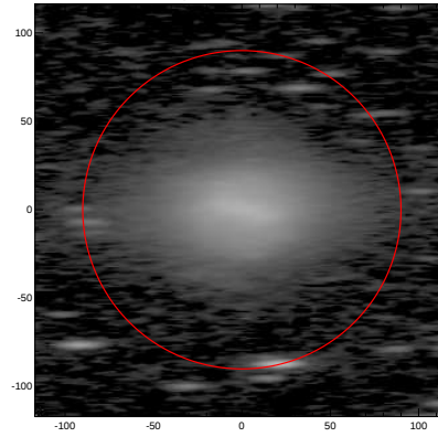
LEDA: pa,inc= 1.4 79.9
