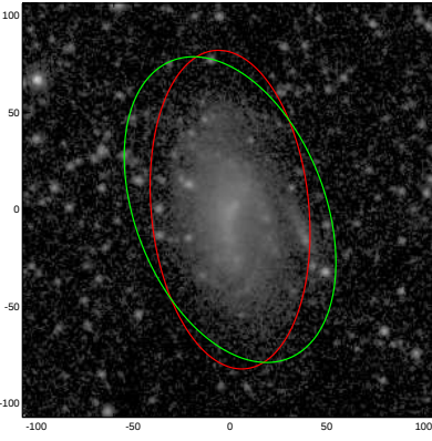
UGC08733
