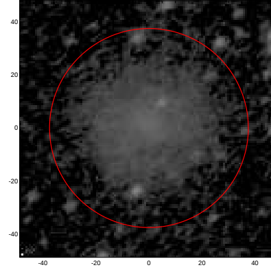
LEDA: pa,inc= 34.3 45.5
