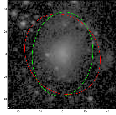
UGC10437
