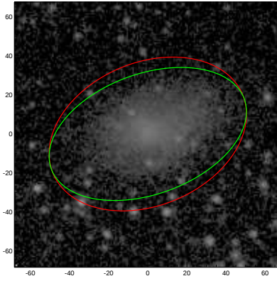
UGC05427
