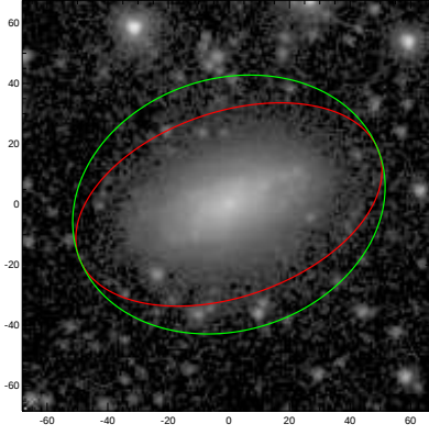
UGC10721
