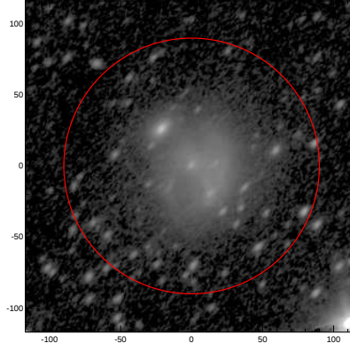
LEDA: pa,inc= 48.6 54.3
