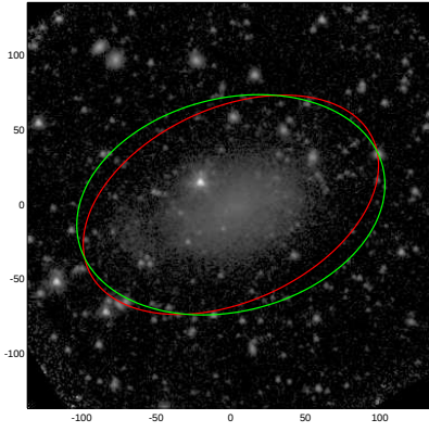
UGC06900
