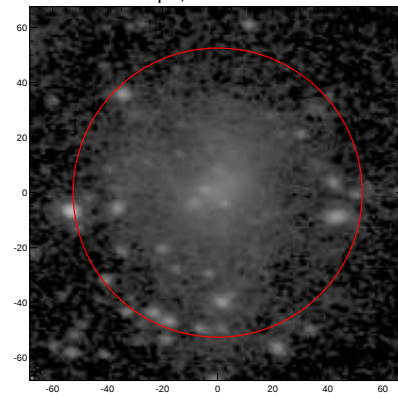
LEDA: pa,inc= 173.9 40.2
