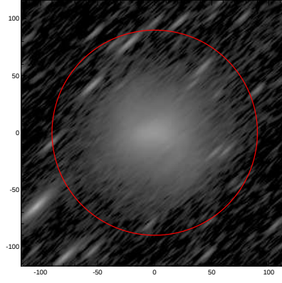
LEDA: pa,inc= 42.5 79.4
