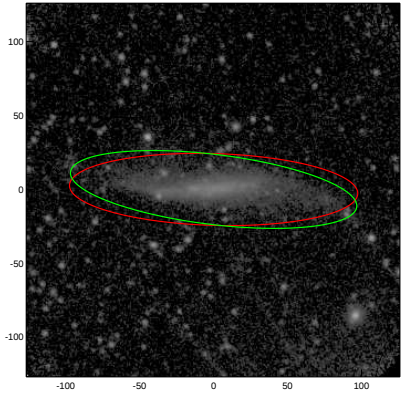
UGC08246
