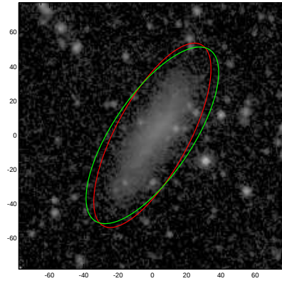
UGC06969
