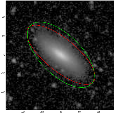
UGC06271
