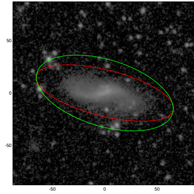
UGC05358
