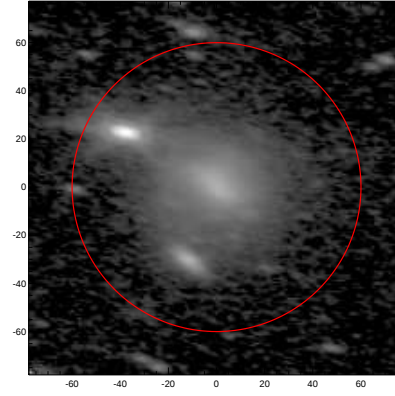
LEDA: pa,inc= 170.5 63.9
