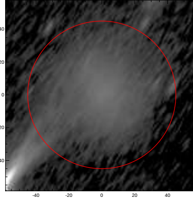
LEDA: pa,inc= 57.2 73.6
