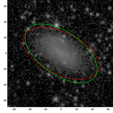
UGC09470
