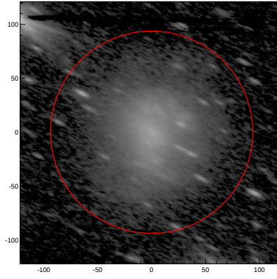
LEDA: pa,inc= 154.3 70.2
