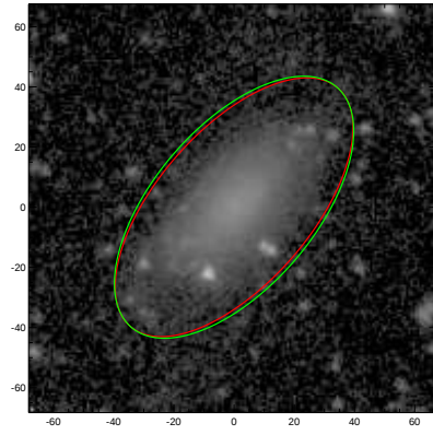
UGC05522
