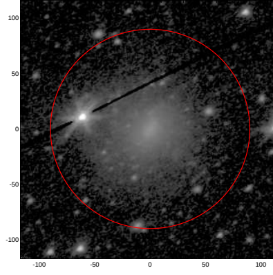
LEDA: pa,inc= 32.0 43.2
