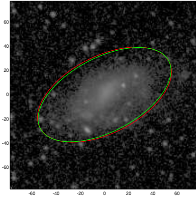
UGC05393
