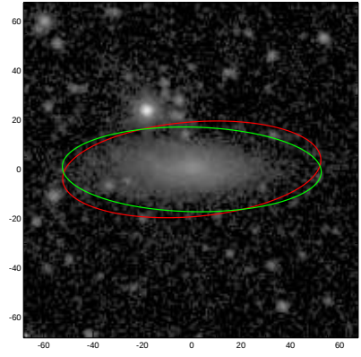
UGC08282
