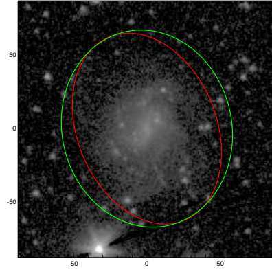
UGC06157
