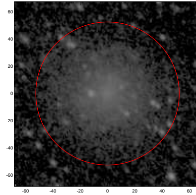
LEDA: pa,inc= 126.0 37.8
