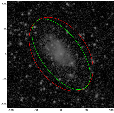
UGC00634
