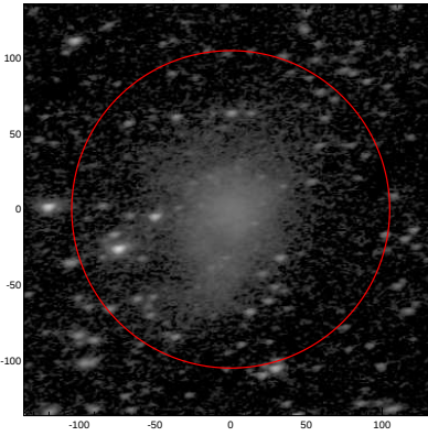
LEDA: pa,inc= 8.5 55.7
