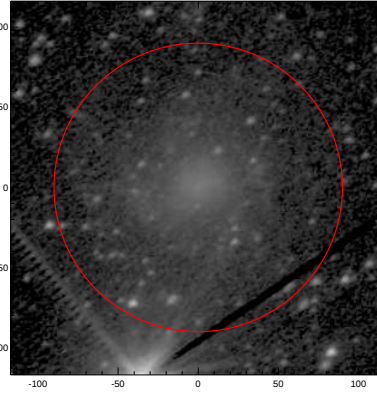
LEDA: pa,inc= 28.9 43.4
