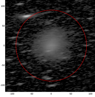
LEDA: pa,inc= 7.6 75.8
