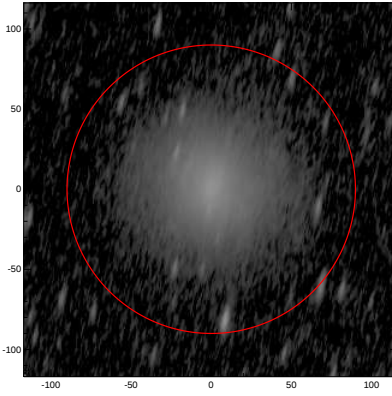
LEDA: pa,inc= 77.6 75.2
