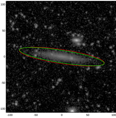
UGC07301
