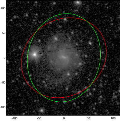
UGC05707
