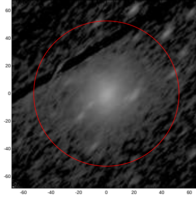
LEDA: pa,inc= 45.2 69.8
