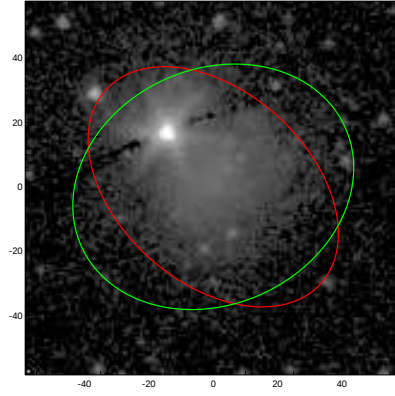
UGC06181
