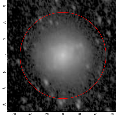
LEDA: pa,inc= 109.3 54.5
