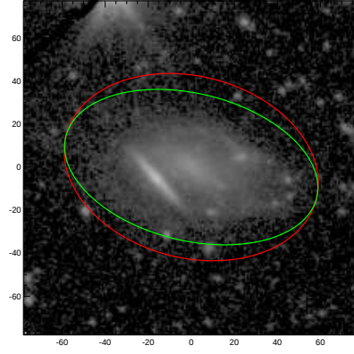
UGC05354
