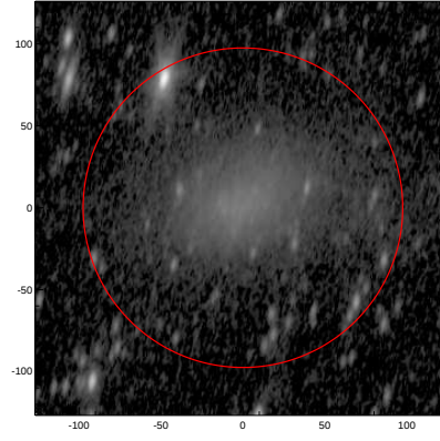
LEDA: pa,inc= 78.8 65.4
