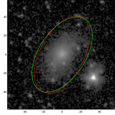
UGC06512
