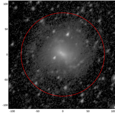
LEDA: pa,inc= 51.0 48.5
