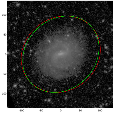
UGC06903
