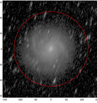
LEDA: pa,inc= 70.7 71.4
