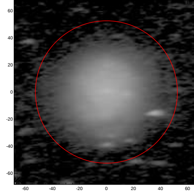
LEDA: pa,inc= 4.5 70.6
