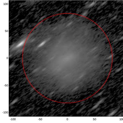
LEDA: pa,inc= 37.5 74.3
