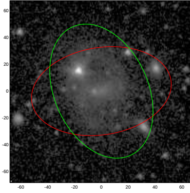
UGC05934
