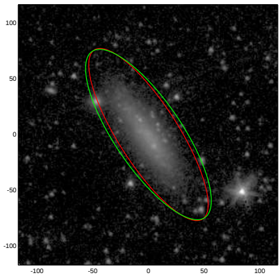
UGC08313
