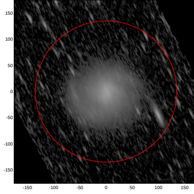
LEDA: pa,inc= 115.8 76.0
