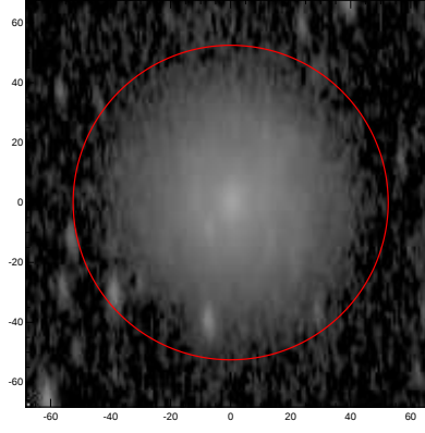
LEDA: pa,inc= 93.3 69.2
