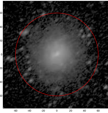
LEDA: pa,inc= 40.0 54.5
