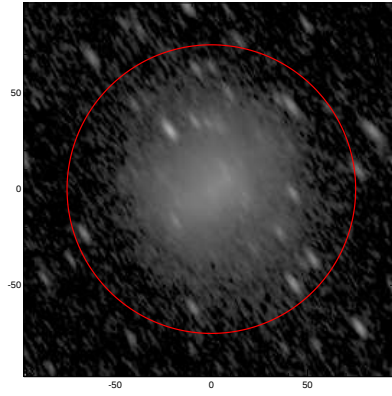
LEDA: pa,inc= 124.7 68.0
