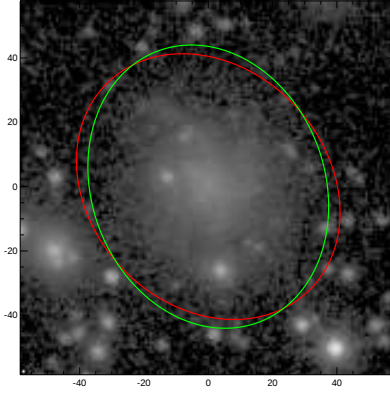
UGC05976
