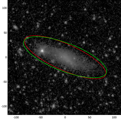
UGC06171
