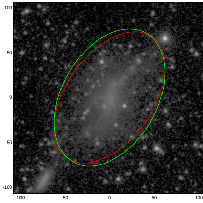
UGC05688
