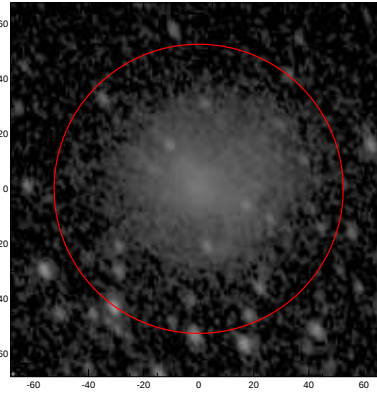
LEDA: pa,inc= 112.7 45.8
