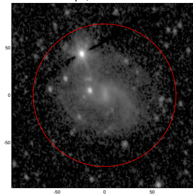
LEDA: pa,inc= 999.0 39.1
