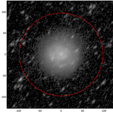
LEDA: pa,inc= 50.0 61.9
