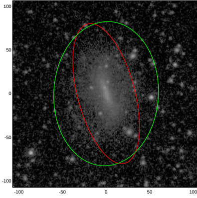
UGC09245
