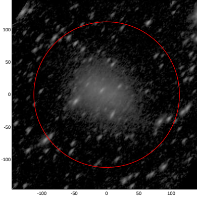
LEDA: pa,inc= 47.0 61.3
