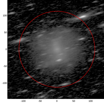
LEDA: pa,inc= 16.2 76.0
