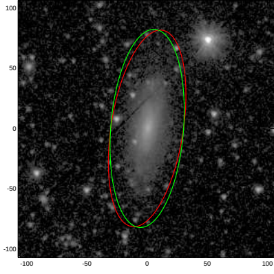
UGC10413
