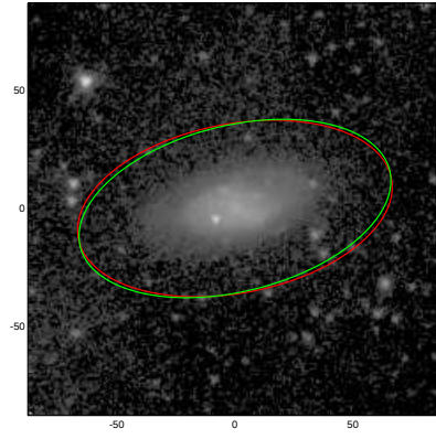
UGC09356
