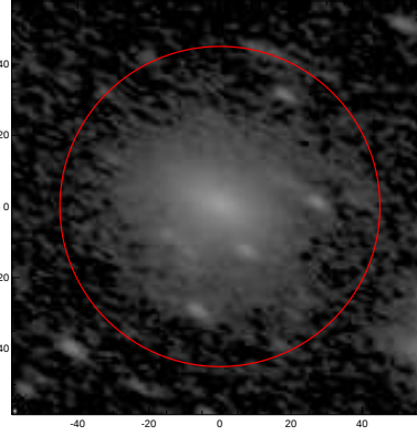
LEDA: pa,inc= 151.7 58.6
