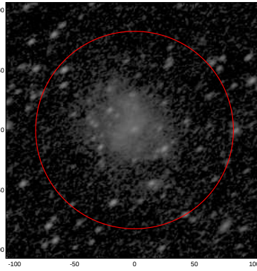
LEDA: pa,inc= 35.0 50.8
