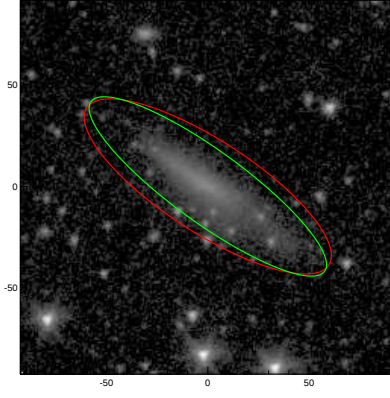
UGC01197
