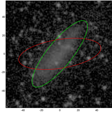
UGC09979
