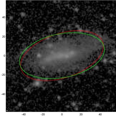
UGC08489
