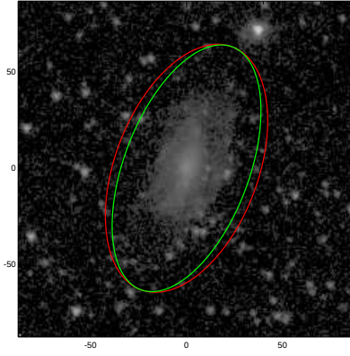
UGC08056
