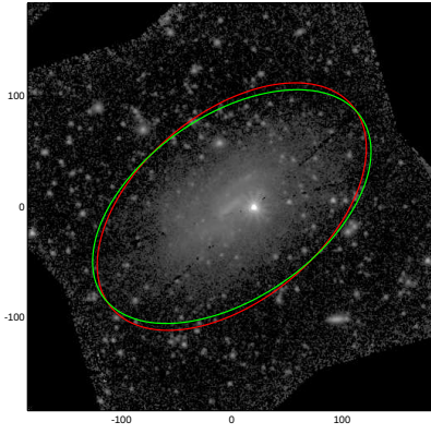
UGC06917
