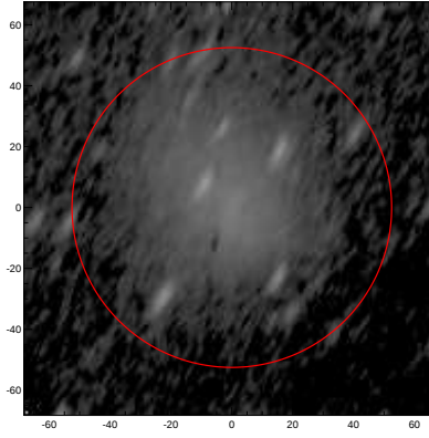
LEDA: pa,inc= 62.7 68.4
