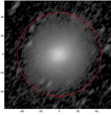
LEDA: pa,inc= 50.3 67.7
