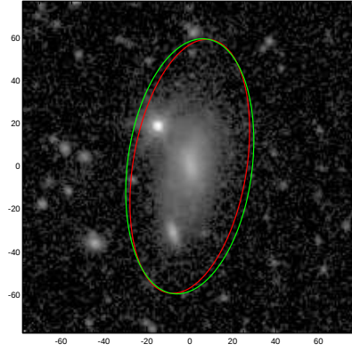
UGC07590
