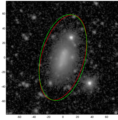
UGC09206
