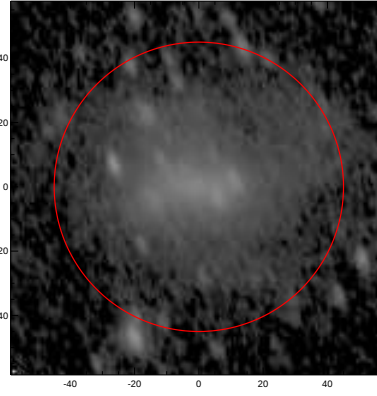
LEDA: pa,inc= 108.2 59.1
