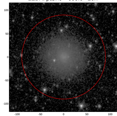
LEDA: pa,inc= 999.0 26.7
