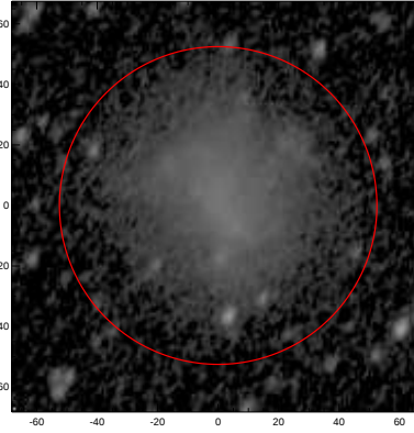
LEDA: pa,inc= 67.7 49.9
