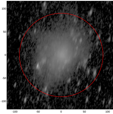
LEDA: pa,inc= 77.0 69.7
