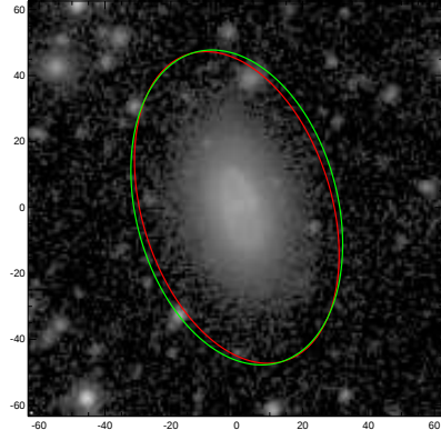
UGC00313
