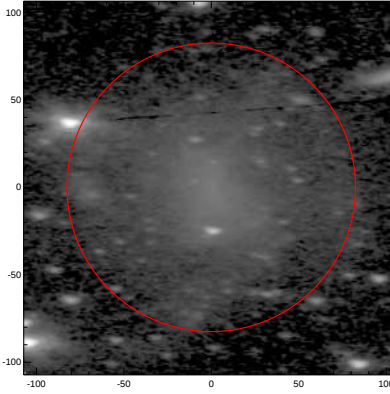
LEDA: pa,inc= 177.0 61.6
