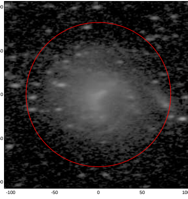
LEDA: pa,inc= 5.5 60.5
