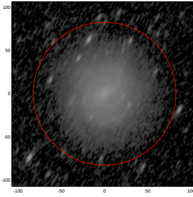
LEDA: pa,inc= 61.0 66.7
