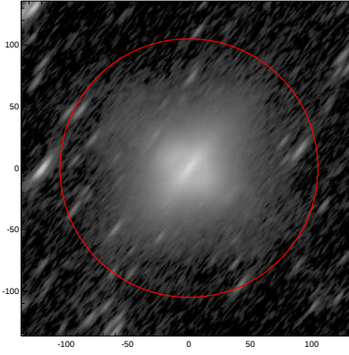
LEDA: pa,inc= 50.7 77.0
