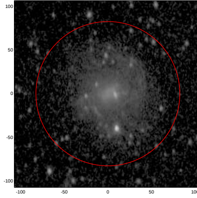
LEDA: pa,inc= 90.8 45.8
