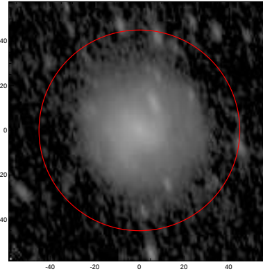
LEDA: pa,inc= 105.5 63.4
