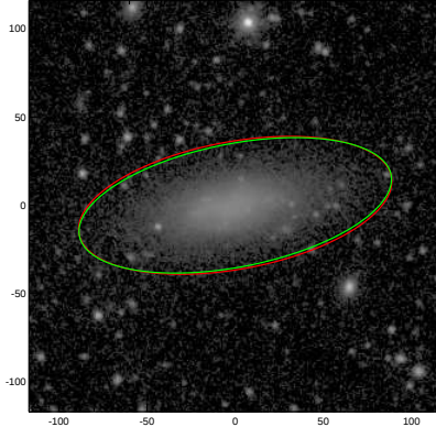
UGC05451
