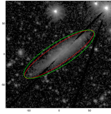
UGC08726
