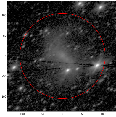
LEDA: pa,inc= 35.0 53.0
