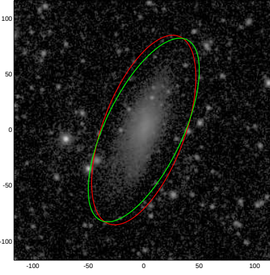
UGC07271
