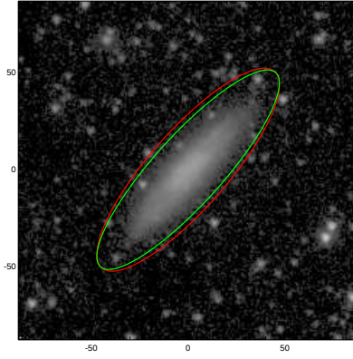
UGC09746
