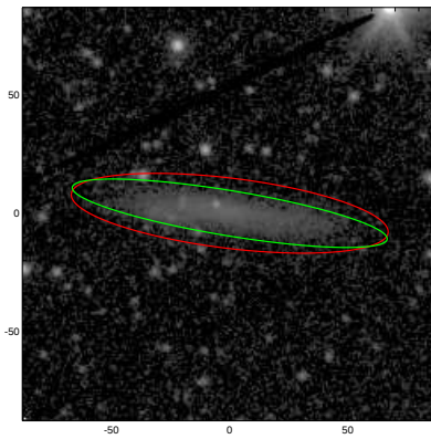
UGC07186
