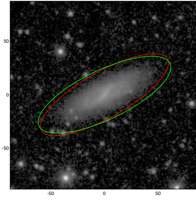
UGC04800
