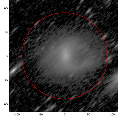
LEDA: pa,inc= 43.3 73.6
