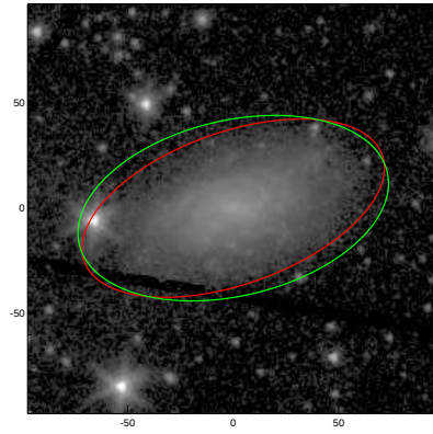
UGC09291
