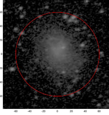
LEDA: pa,inc= 20.1 45.5
