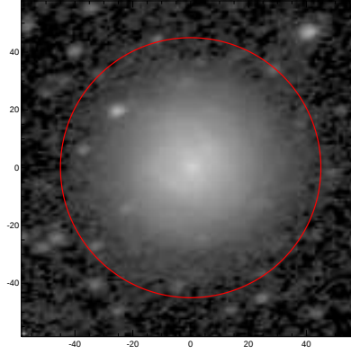
LEDA: pa,inc= 15.0 46.0
