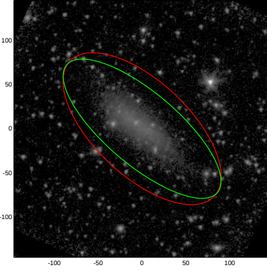
UGC00891
