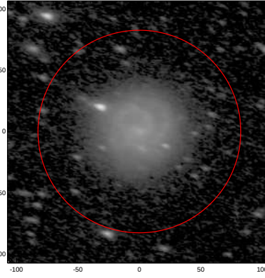
LEDA: pa,inc= 163.2 60.6
