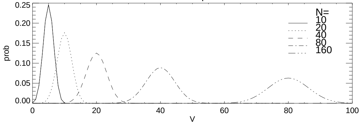
Binomial p=0.5
