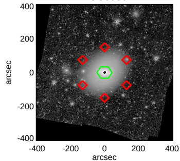
NGC0936
