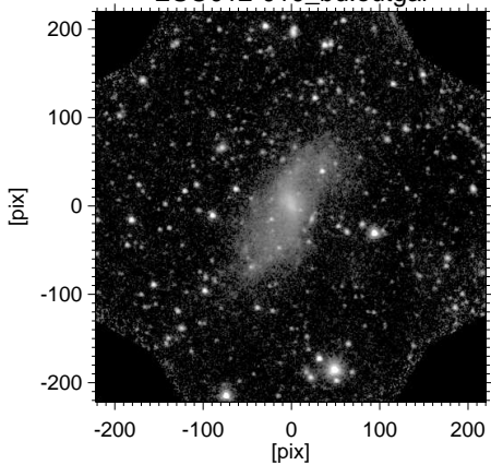
model (20&lt;mag&lt;26)
