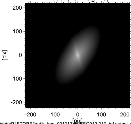
model (20&lt;mag&lt;26)
