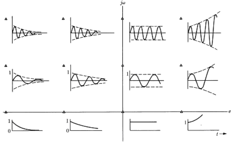
Figure 1: Navat ja impulssivasteet.
