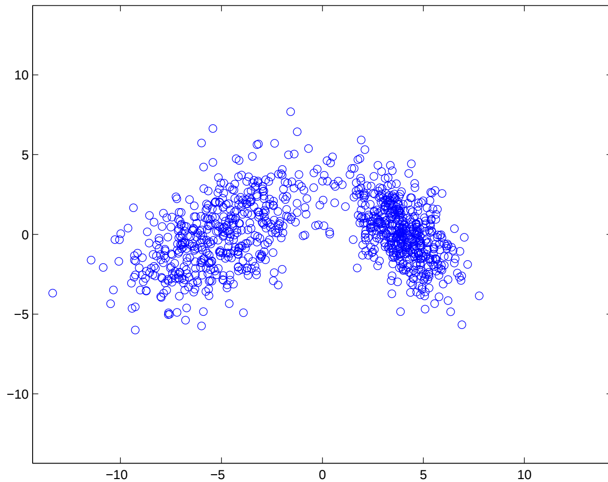
Harjoitus 4, tehtävä 5, osa 2 alkuperäiset jakaumat
