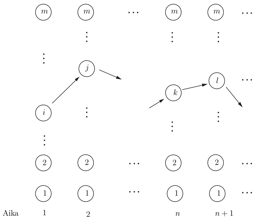
Kuva 3.6: Markovin ketju.
