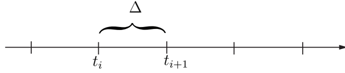
Kuva 6.3: Reaaliakselin osiinjako.
